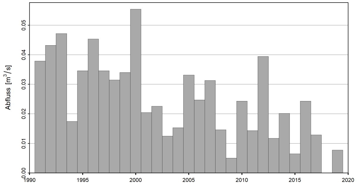
Abbildung 6: Zeitreihe der NM7Q [ m^3/s ] (01.03.1990 - 28.02.2020)
