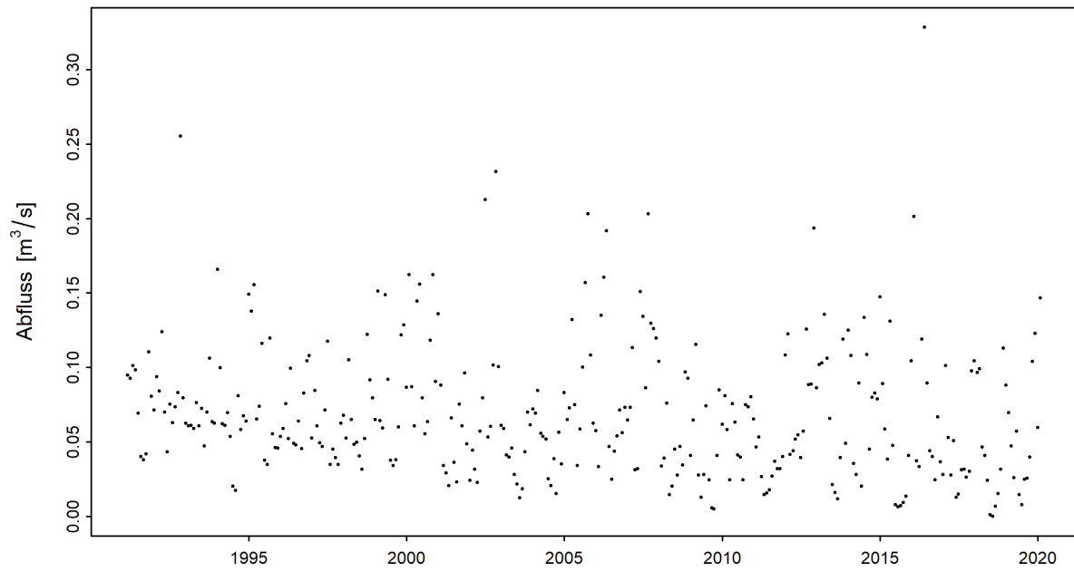
Abbildung 3: Zeitreihe der monatlichen Minima der M7Q [m³/s] (01.03.1990 - 28.02.2020)
