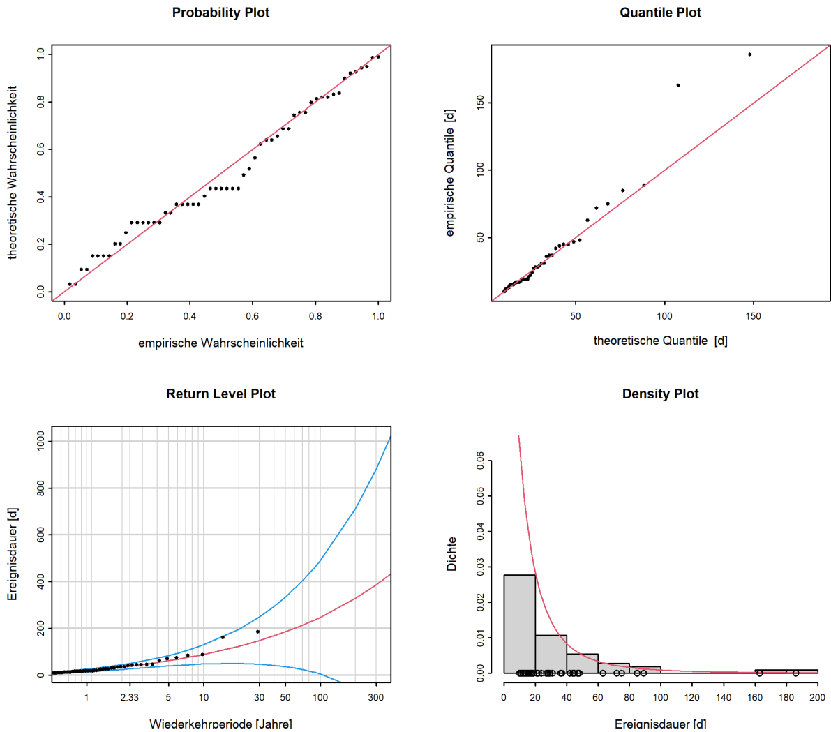
Abbildung 12: Diagnostikplots der Modellvariante "stat" des POT-Ansatzes (01.03.1991 - 29.02.2020)
