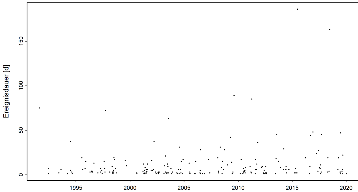
Abbildung 4: Zeitreihe der Niedrigwasserdauern [d] (01.03.1990 - 28.02.2020)
