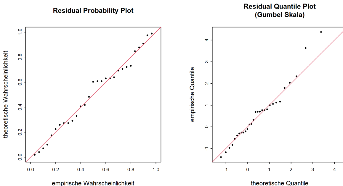
Abbildung 7: Diagnostikplots der Modellvariante “mujump2001” des BLOCK-Ansatzes (01.03.1991 - 29.02.2020)
