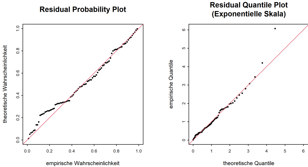
Abbildung 9: Diagnostikplots der Modellvariante “sigjump2001” des POT-Ansatzes (01.03.1991 - 29.02.2020)
