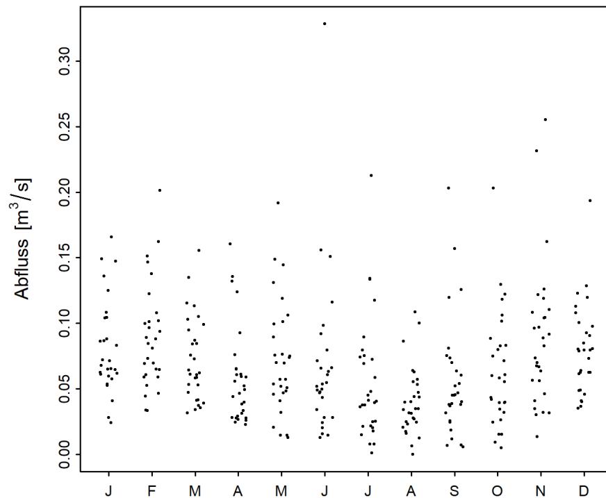
Abbildung 2: Saisonaler Verlauf der monatlichen Minima der M7Q [ \text{m}^3/\text{s} ] (01.03.1990 - 28.02.2020)
