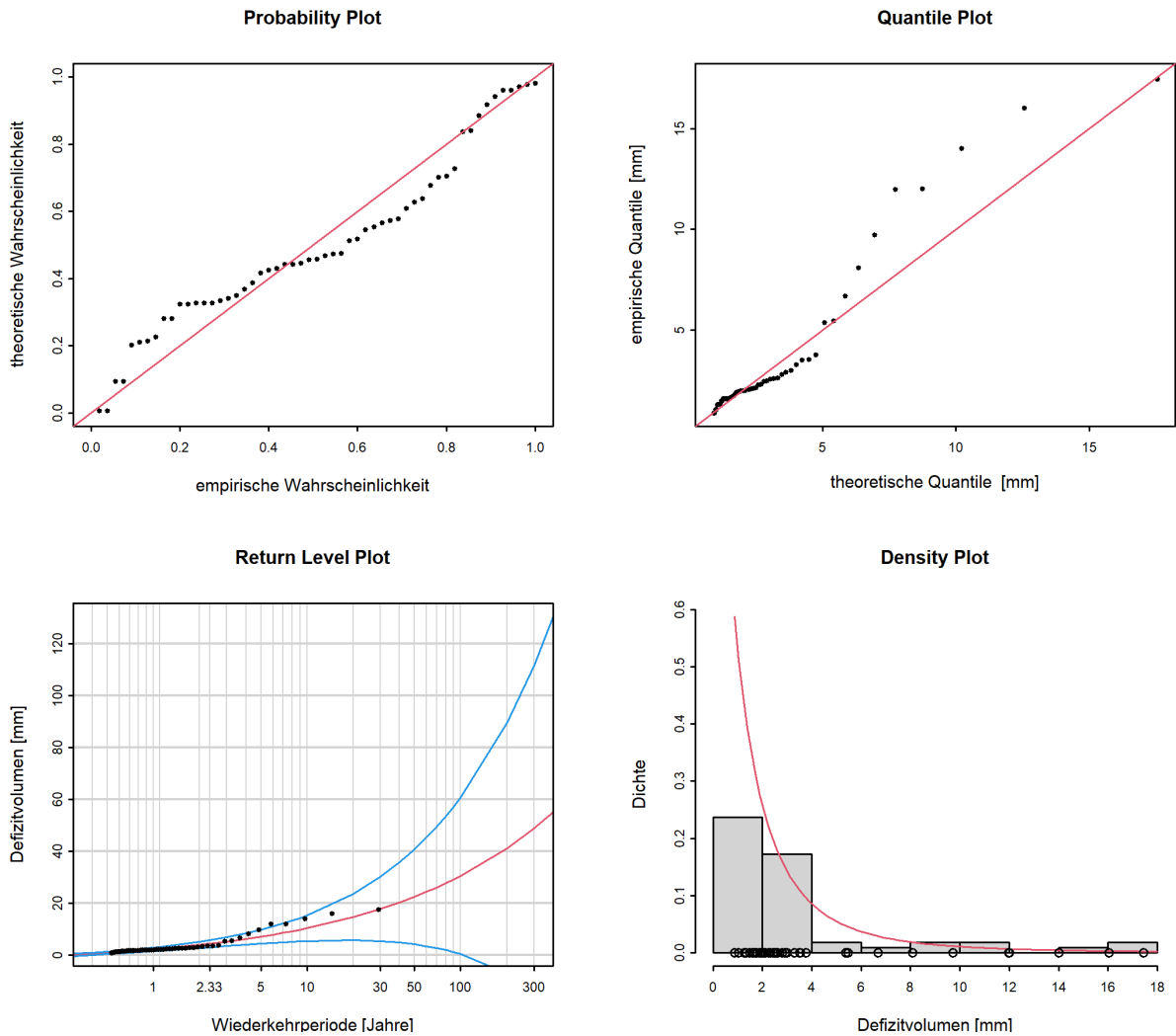
Abbildung 14: Diagnostikplots der Modellvariante “stat” des POT-Ansatzes (01.03.1991 - 29.02.2020)
