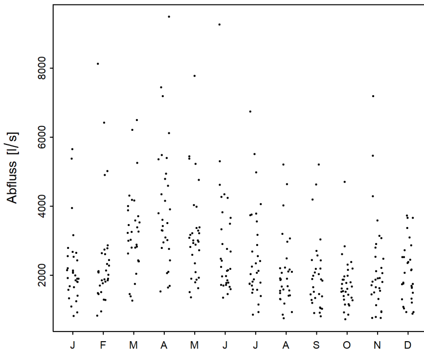
Abbildung 2: Saisonaler Verlauf der monatlichen Minima der M7Q [l/s] (01.04.1989 - 31.03.2020)
