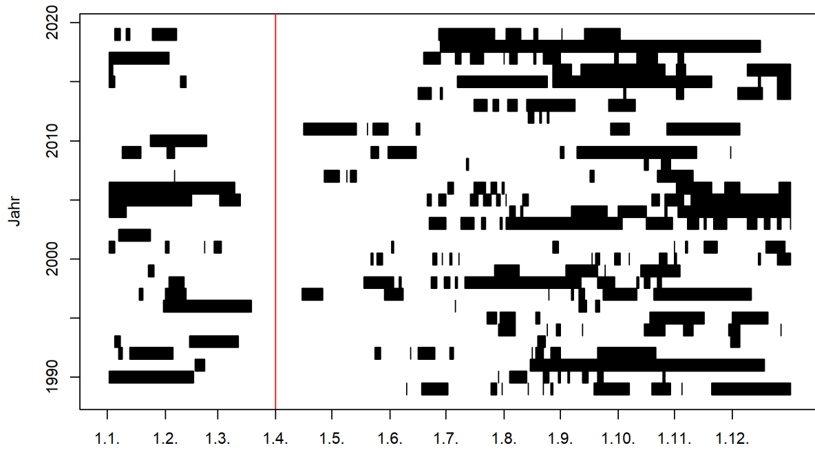
Abbildung 1: Zeitliches Auftreten der Niedrigwasserperioden im Jahresverlauf (01.04.1989 - 31.03.2020) und Startmonat des Niedrigwasserjahres (rote Linie) 1
