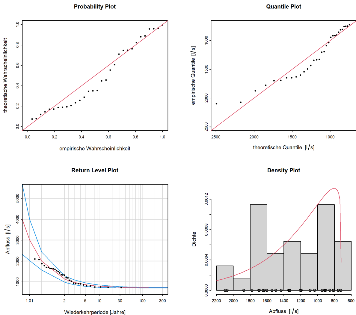
Abbildung 7: Diagnostikplots der Modellvariante “stat” des BLOCK-Ansatzes (01.04.1989 - 31.03.2020)
