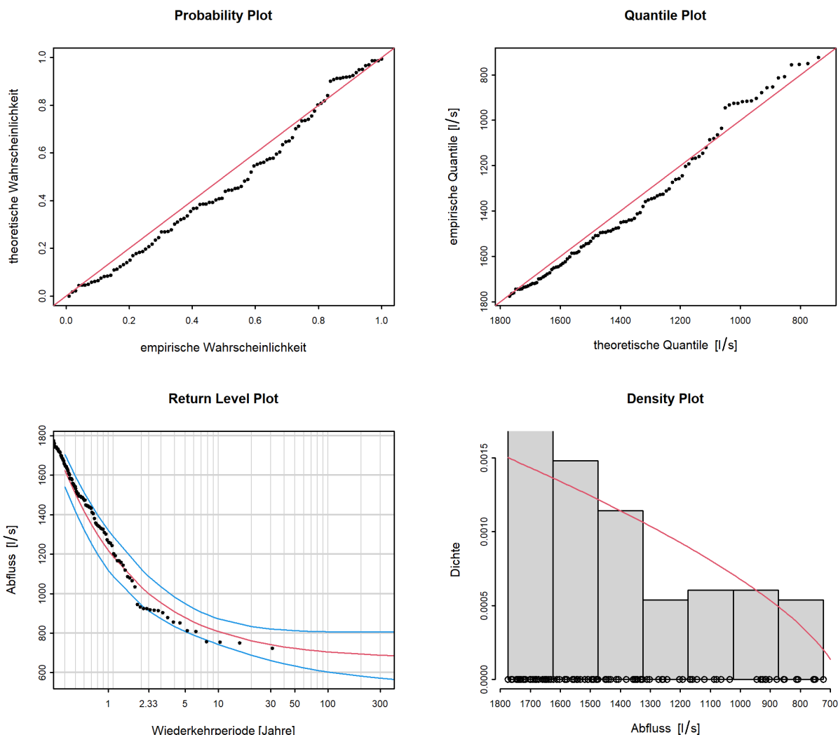
Abbildung 9: Diagnostikplots der Modellvariante "stat" des POT-Ansatzes (01.04.1989 - 31.03.2020)
