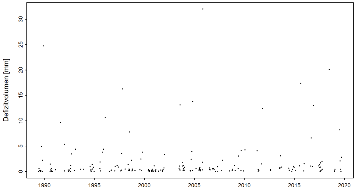
Abbildung 5: Zeitreihe der Defizitvolumen [mm] (01.04.1989 - 31.03.2020)
