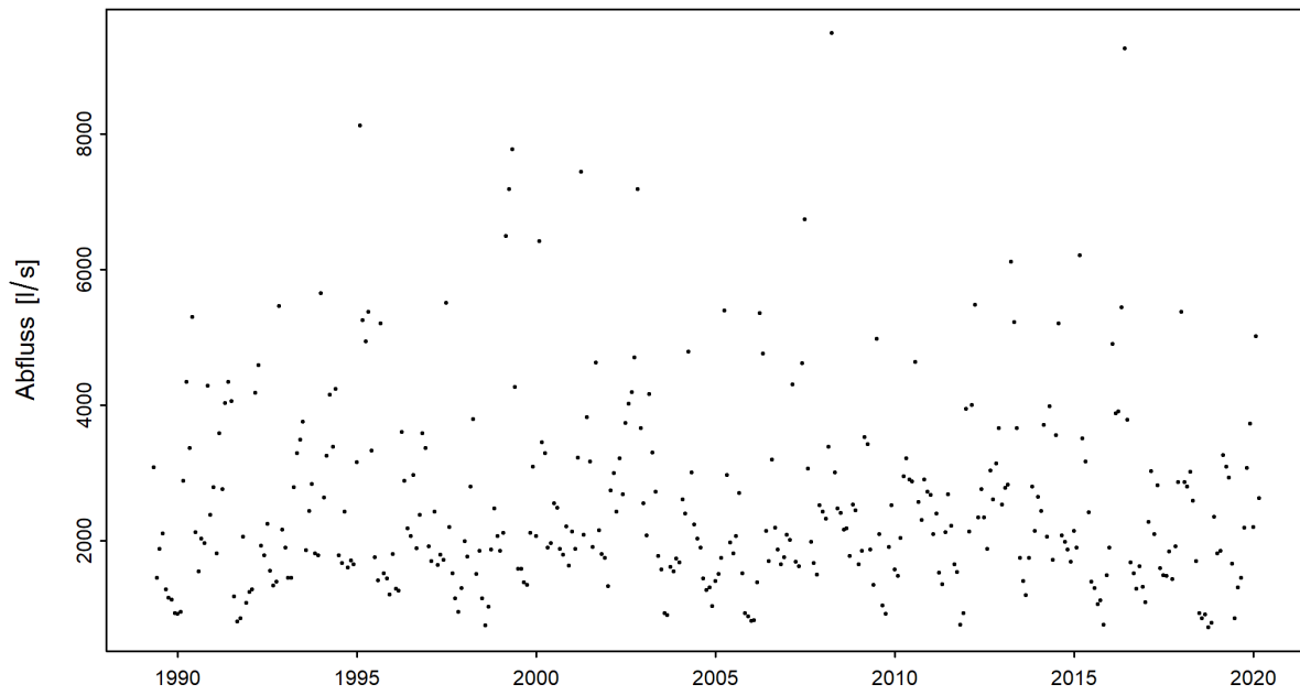
Abbildung 3: Zeitreihe der monatlichen Minima der M7Q [l/s] (01.04.1989 - 31.03.2020)
