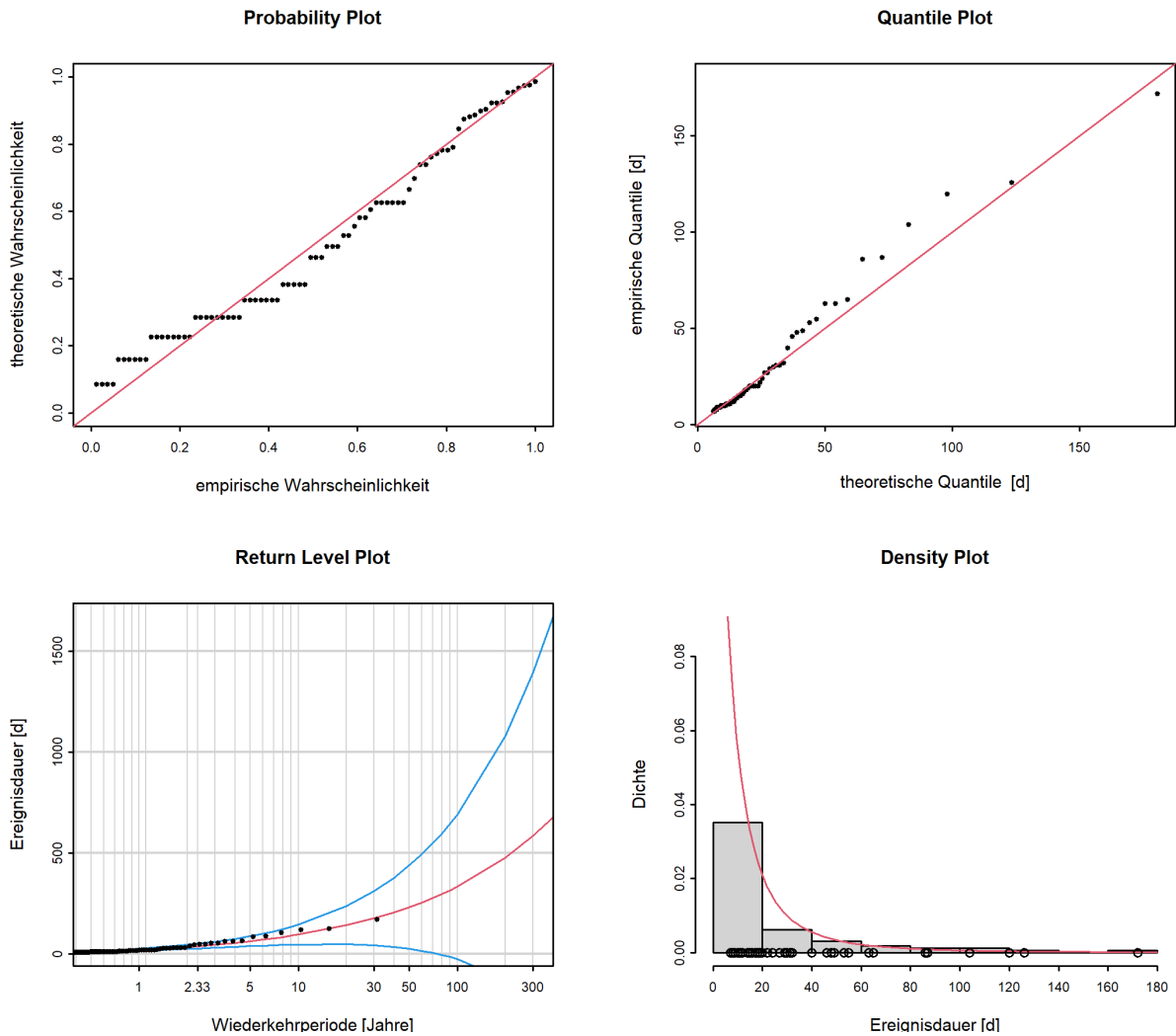
Abbildung 12: Diagnostikplots der Modellvariante “stat” des POT-Ansatzes (01.04.1989 - 31.03.2020)
