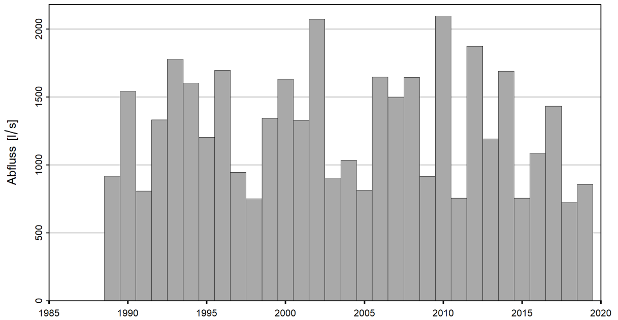
Abbildung 6: Zeitreihe der NM7Q [l/s] (01.04.1989 - 31.03.2020)
