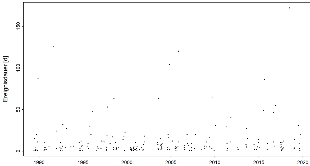
Abbildung 4: Zeitreihe der Niedrigwasserdauern [d] (01.04.1989 - 31.03.2020)
