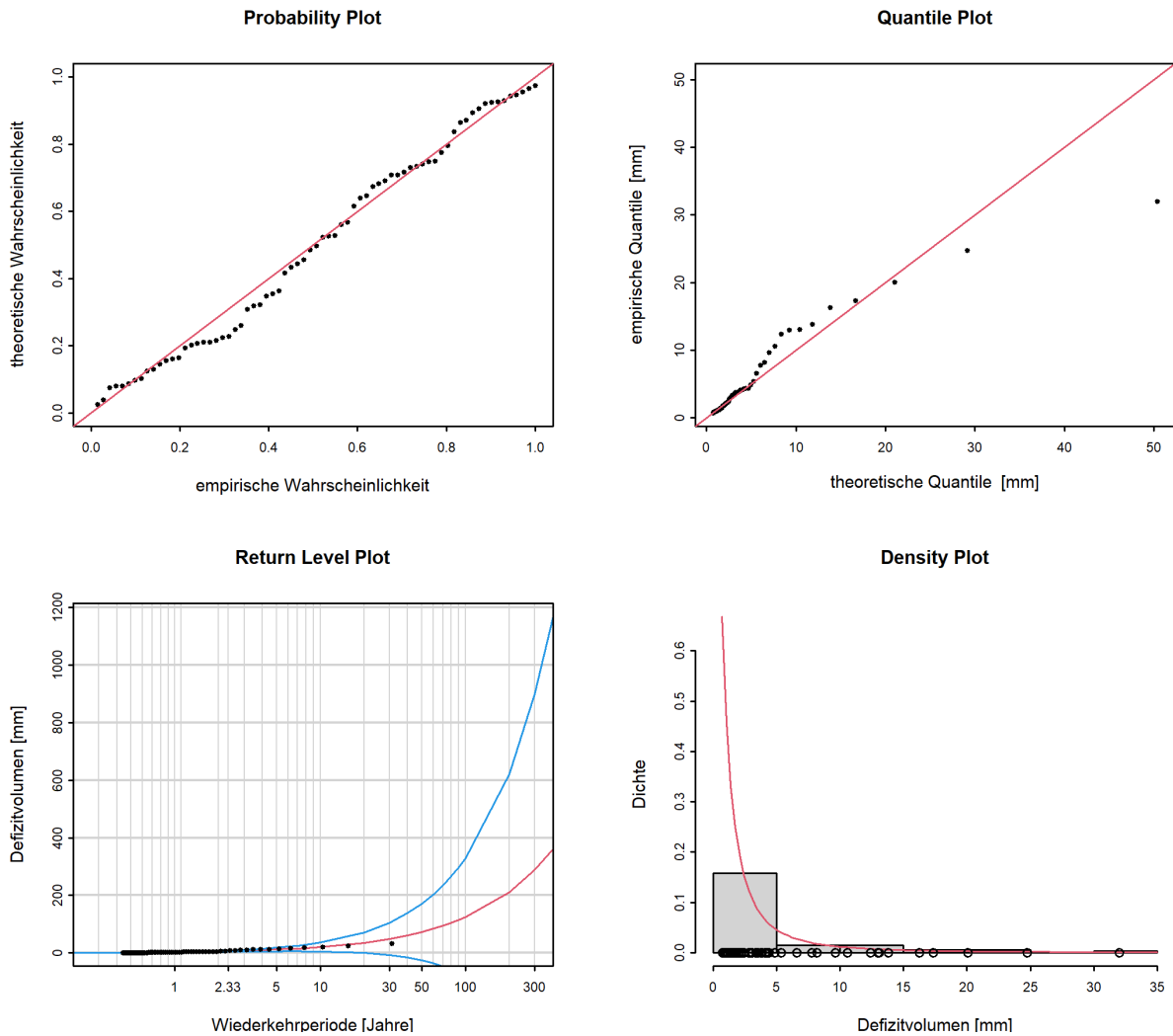
Abbildung 14: Diagnostikplots der Modellvariante “stat” des POT-Ansatzes (01.04.1989 - 31.03.2020)
