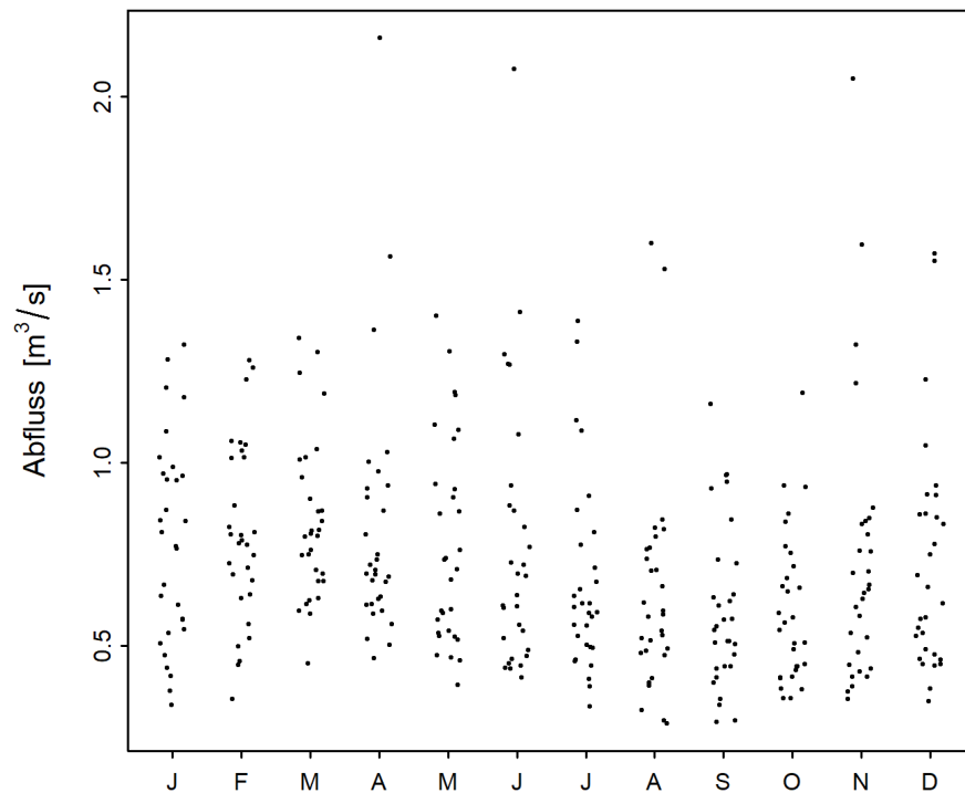
Abbildung 2: Saisonaler Verlauf der monatlichen Minima der M7Q [ \text{m}^3/\text{s} ] (01.04.1988 - 31.03.2019)
