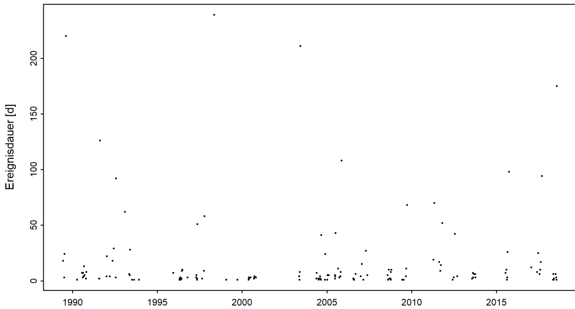
Abbildung 4: Zeitreihe der Niedrigwasserdauern [d] (01.04.1988 - 31.03.2019)
