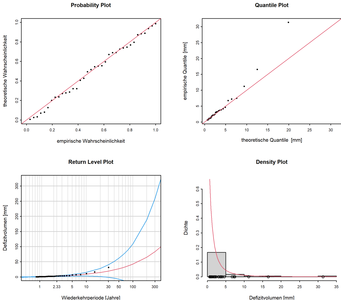
Abbildung 14: Diagnostikplots der Modellvariante "stat" des POT-Ansatzes (01.04.1989 - 31.03.2019)
