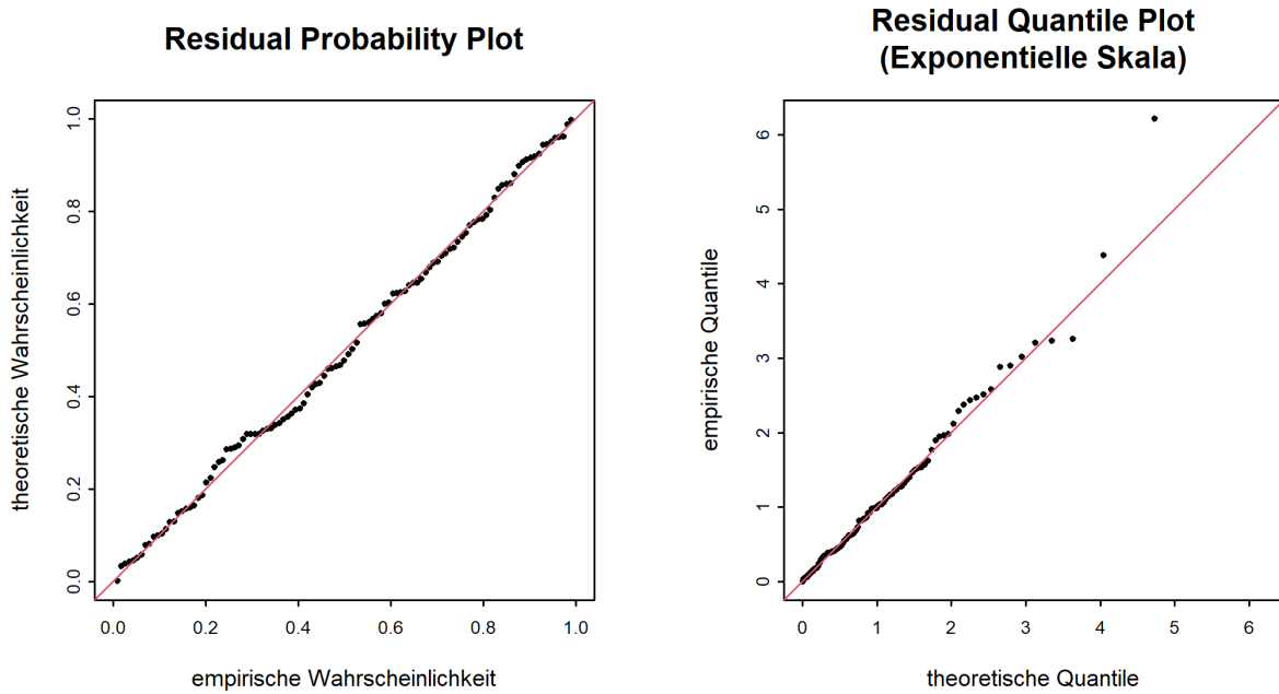
Abbildung 9: Diagnostikplots der Modellvariante “sigl” des POT-Ansatzes (01.04.1989 - 31.03.2019)
