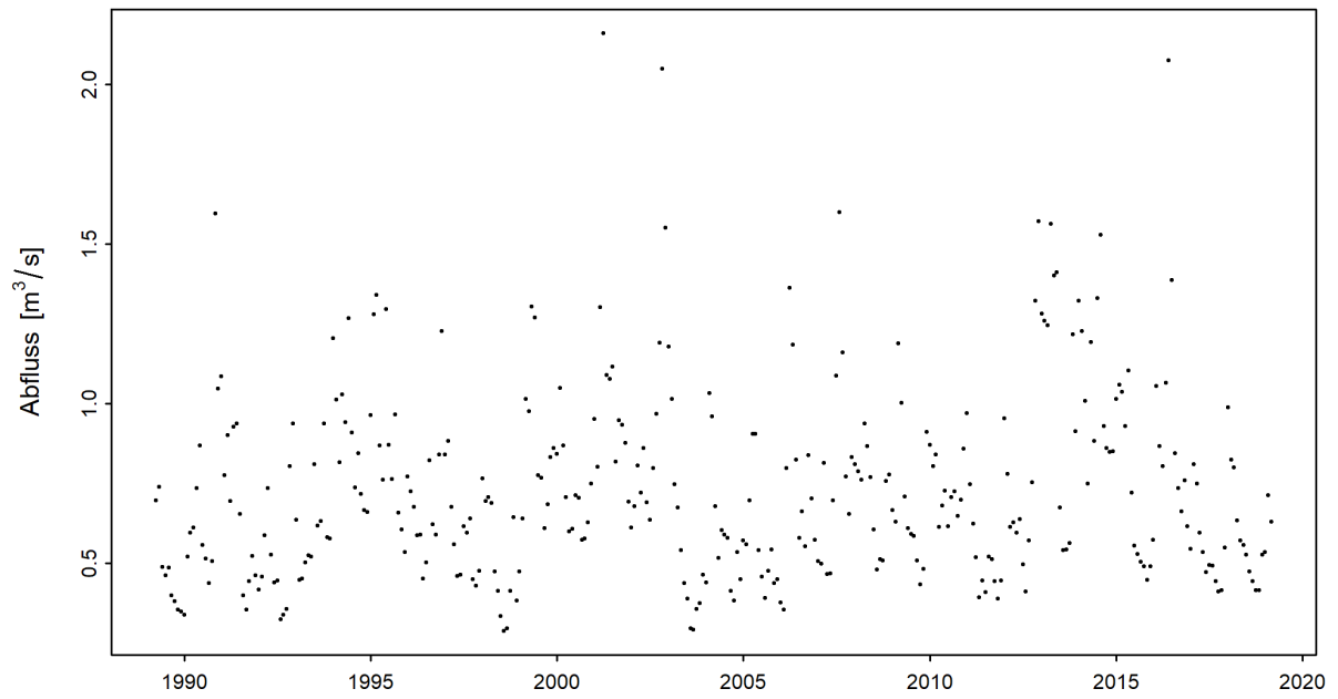
Abbildung 3: Zeitreihe der monatlichen Minima der M7Q [m³/s] (01.04.1988 - 31.03.2019)
