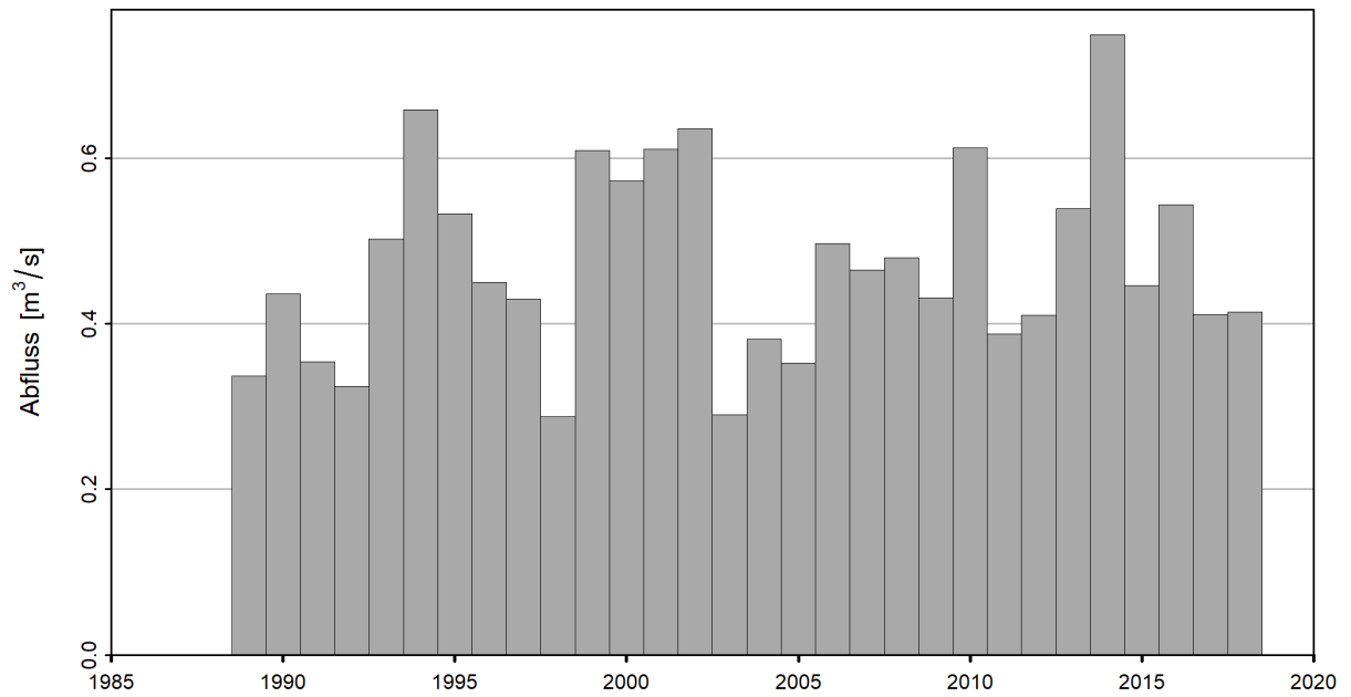
Abbildung 6: Zeitreihe der NM7Q [ \text{m}^3/\text{s} ] (01.04.1988 - 31.03.2019)
