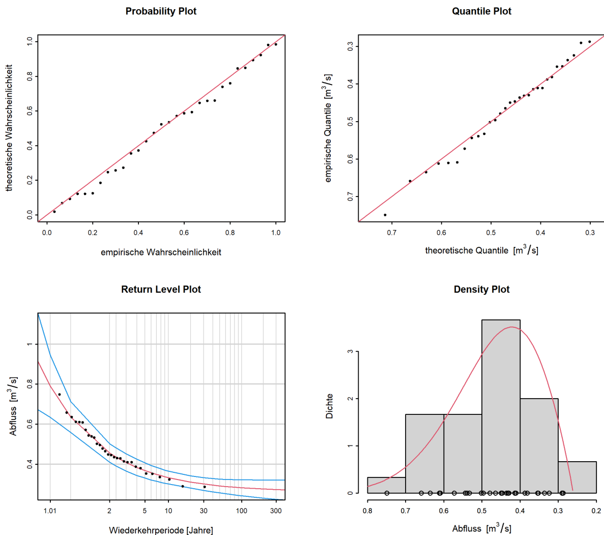
Abbildung 7: Diagnostikplots der Modellvariante “stat” des BLOCK-Ansatzes (01.04.1989 - 31.03.2019)
