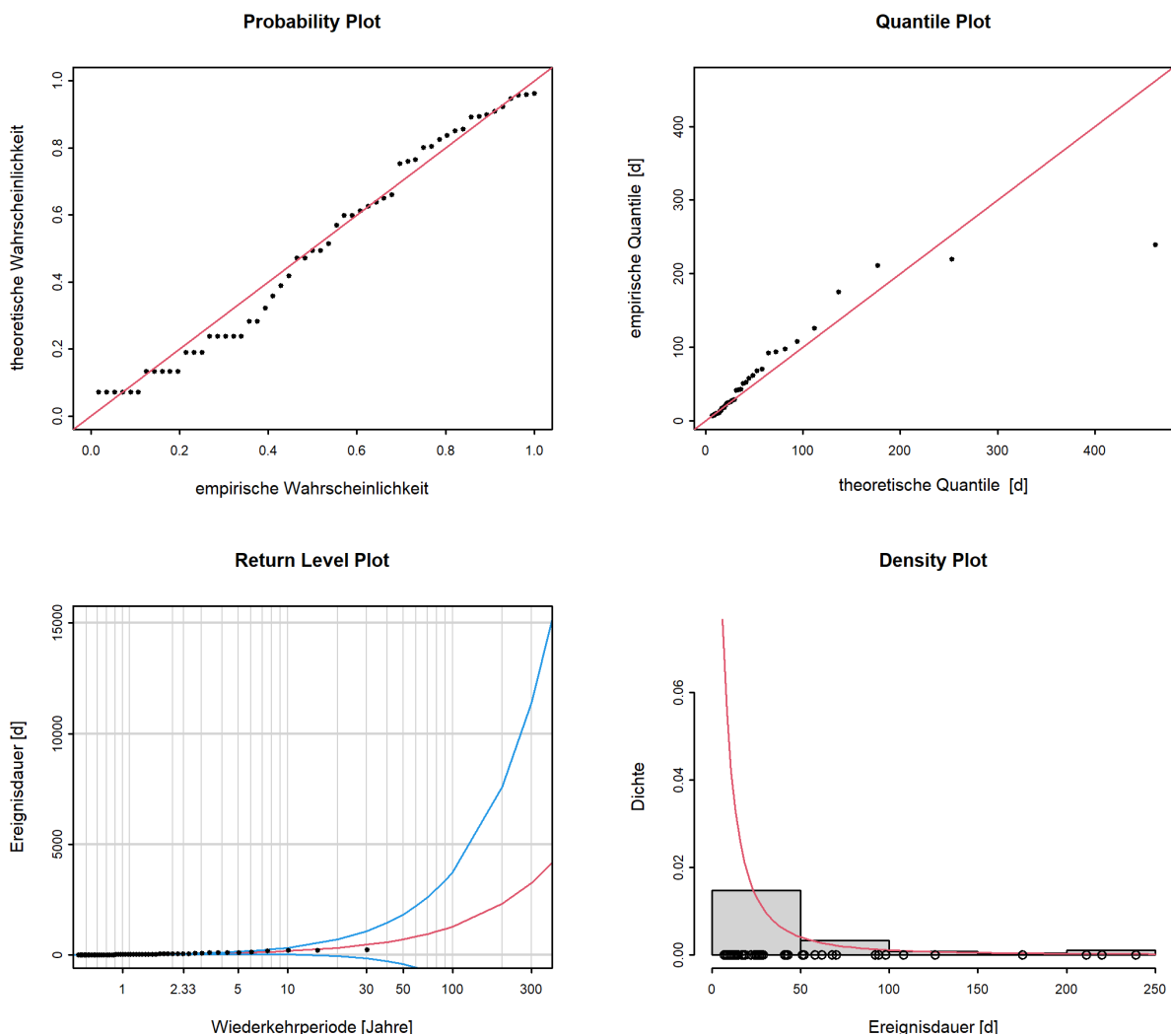
Abbildung 12: Diagnostikplots der Modellvariante “stat” des POT-Ansatzes (01.04.1989 - 31.03.2019)
