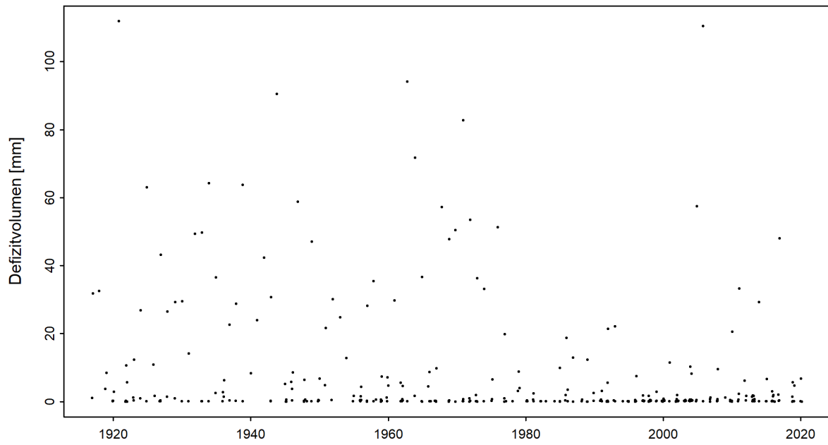
Abbildung 5: Zeitreihe der Defizitvolumen [mm] (01.06.1916 - 31.05.2020)
