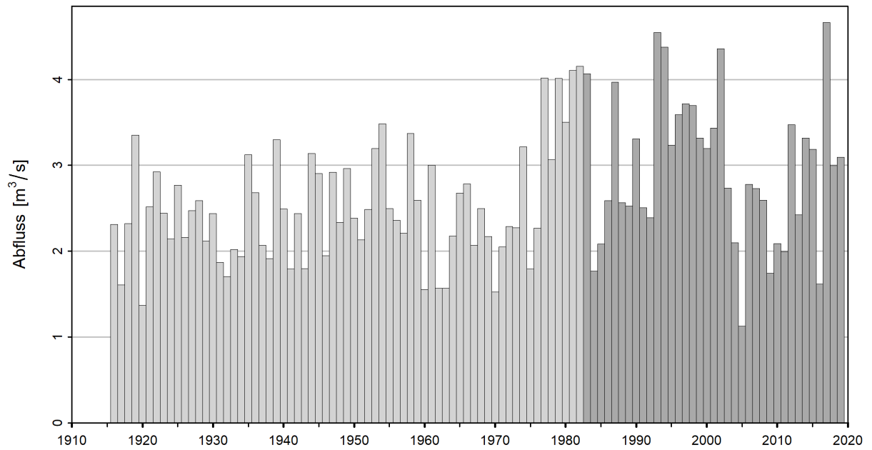
Abbildung 6: Zeitreihe der NM7Q [ \text{m}^3/\text{s} ] (01.06.1916 - 31.05.2020), hellgrau: nicht verwendete NM7Q, dunkelgrau: verwendete NM7Q
