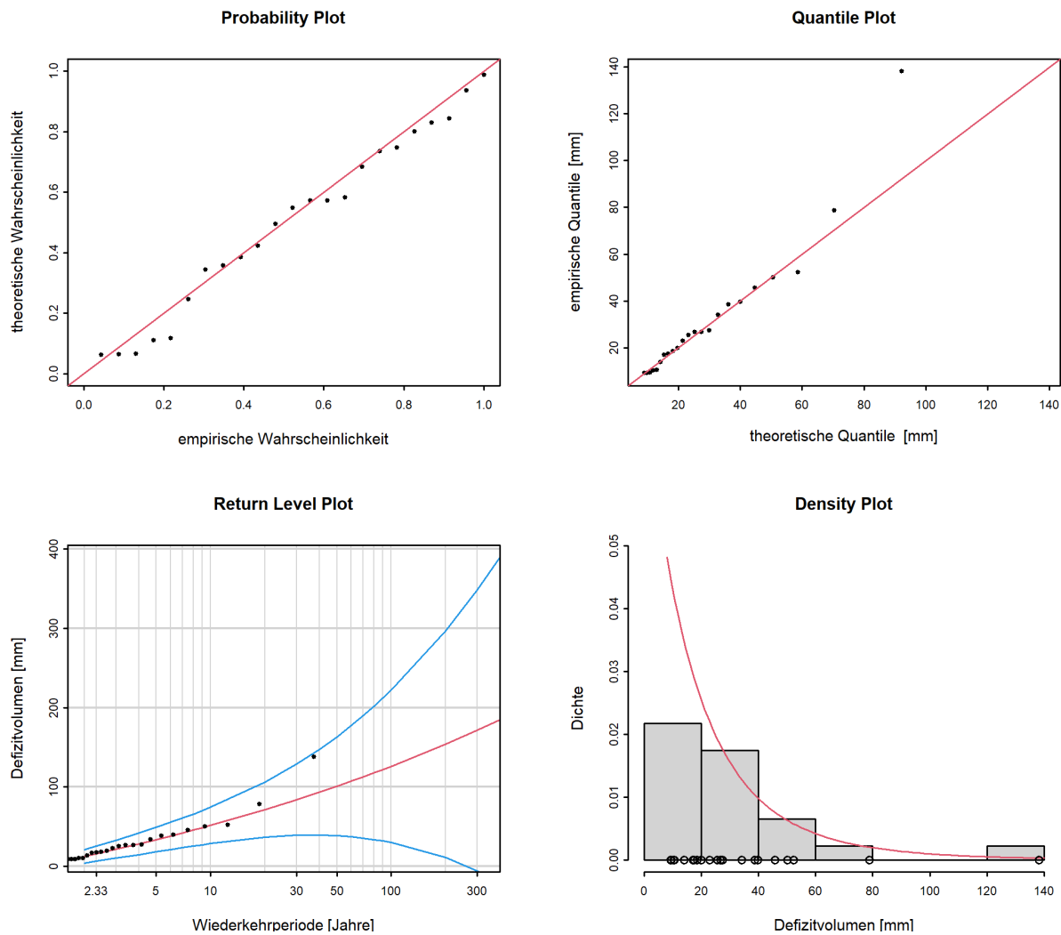
Abbildung 14: Diagnostikplots der Modellvariante “stat” des POT-Ansatzes (01.06.1983 - 31.05.2020)
