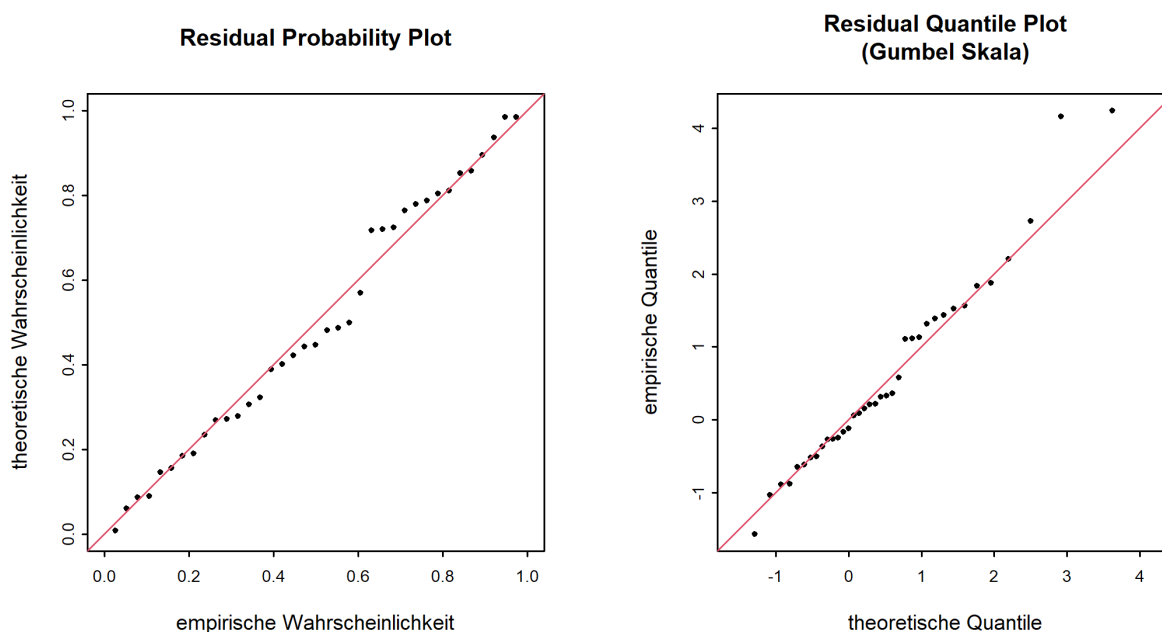
Abbildung 7: Diagnostikplots der Modellvariante "mujump2004" des BLOCK-Ansatzes (01.06.1983 - 31.05.2020)
