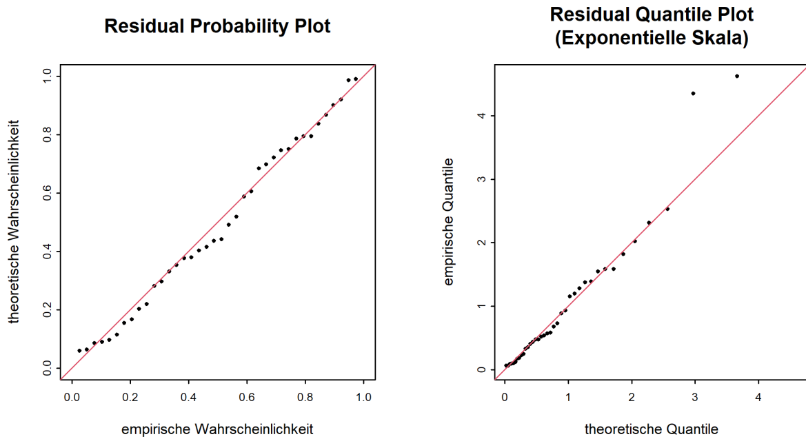
Abbildung 9: Diagnostikplots der Modellvariante "sigjump2004" des POT-Ansatzes (01.06.1983 - 31.05.2020)
