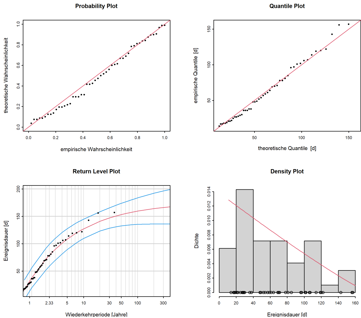
Abbildung 12: Diagnostikplots der Modellvariante “stat” des POT-Ansatzes (01.06.1983 - 31.05.2020)
