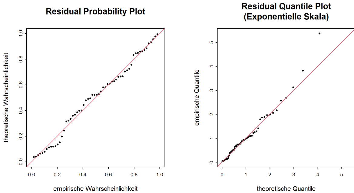
Abbildung 9: Diagnostikplots der Modellvariante “sigjump2009” des POT-Ansatzes (01.04.1983 - 31.03.2020)
