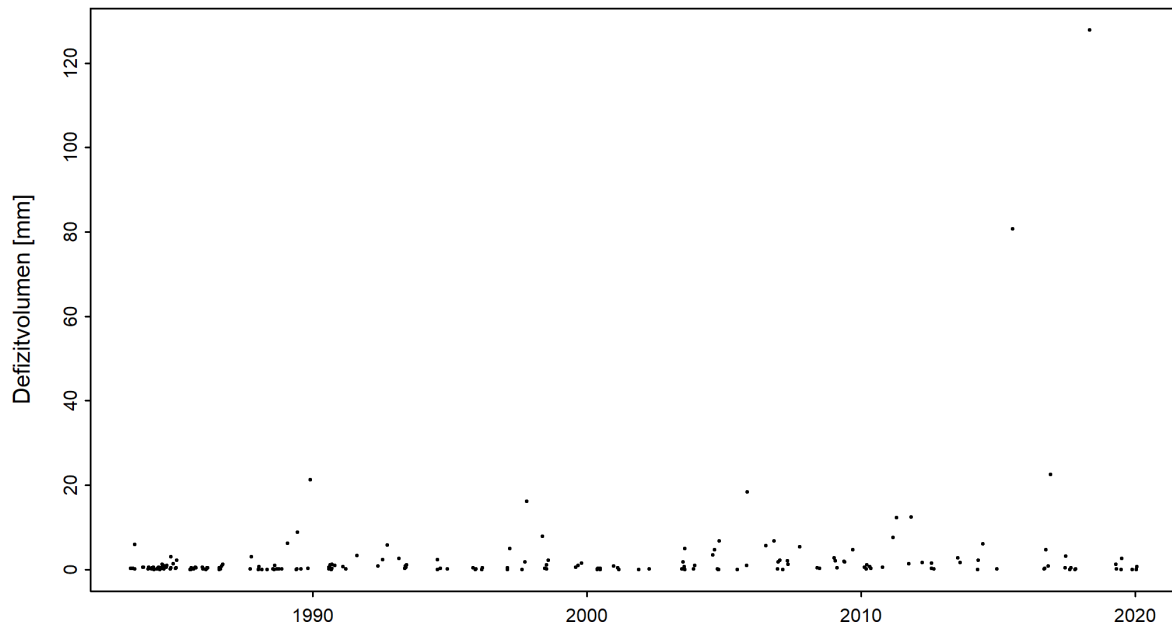
Abbildung 5: Zeitreihe der Defizitvolumen [mm] (01.04.1982 - 31.03.2020)
