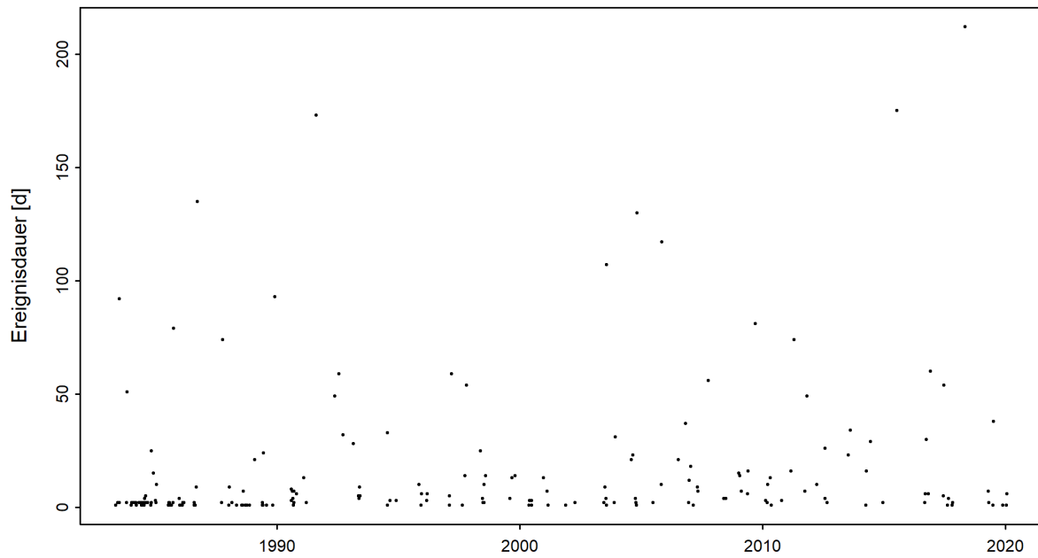
Abbildung 4: Zeitreihe der Niedrigwasserdauern [d] (01.04.1982 - 31.03.2020)
