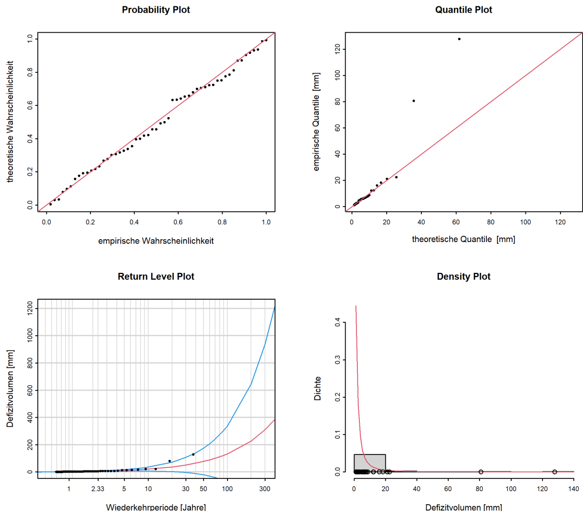
Abbildung 14: Diagnostikplots der Modellvariante “stat” des POT-Ansatzes (01.04.1983 - 31.03.2020)
