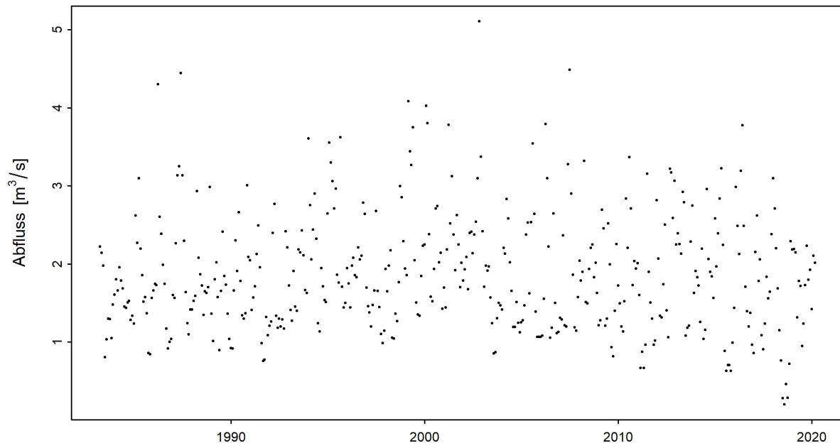
Abbildung 3: Zeitreihe der monatlichen Minima der M7Q [ \text{m}^3/\text{s} ] (01.04.1982 - 31.03.2020)
