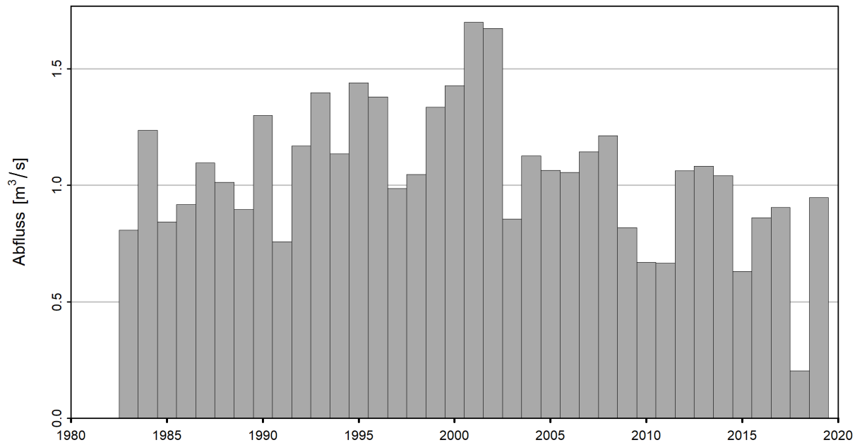
Abbildung 6: Zeitreihe der NM7Q [m³/s] (01.04.1982 - 31.03.2020)
