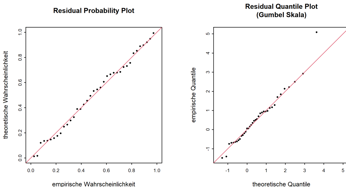
Abbildung 7: Diagnostikplots der Modellvariante “mujump2009” des BLOCK-Ansatzes (01.04.1983 - 31.03.2020)
