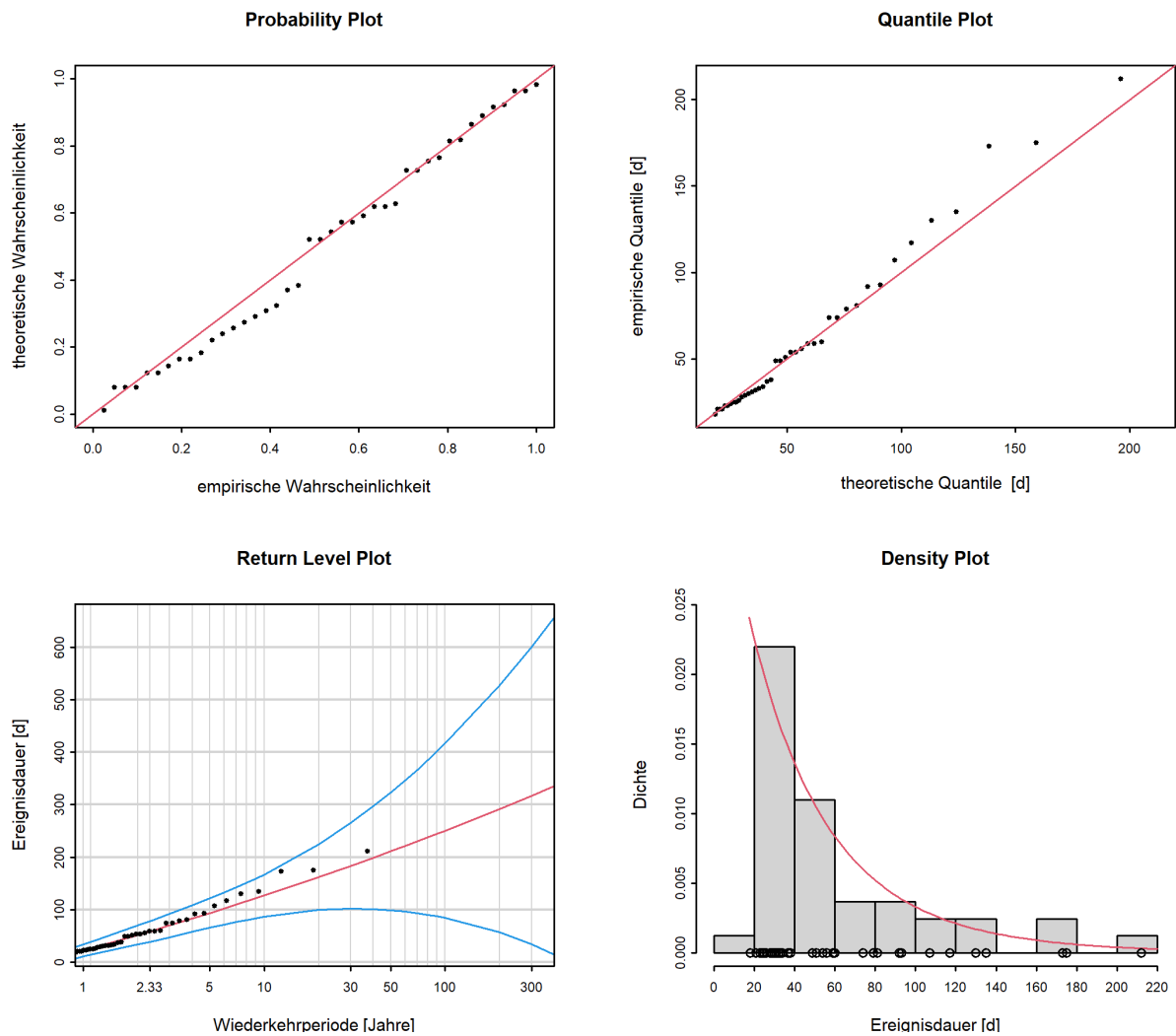
Abbildung 12: Diagnostikplots der Modellvariante “stat” des POT-Ansatzes (01.04.1983 - 31.03.2020)
