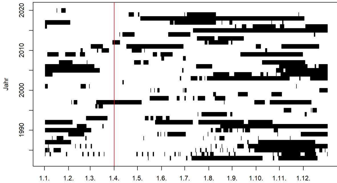
Abbildung 1: Zeitliches Auftreten der Niedrigwasserperioden im Jahresverlauf (01.04.1982 - 31.03.2020) und Startmonat des Niedrigwasserjahres (rote Linie) 1
