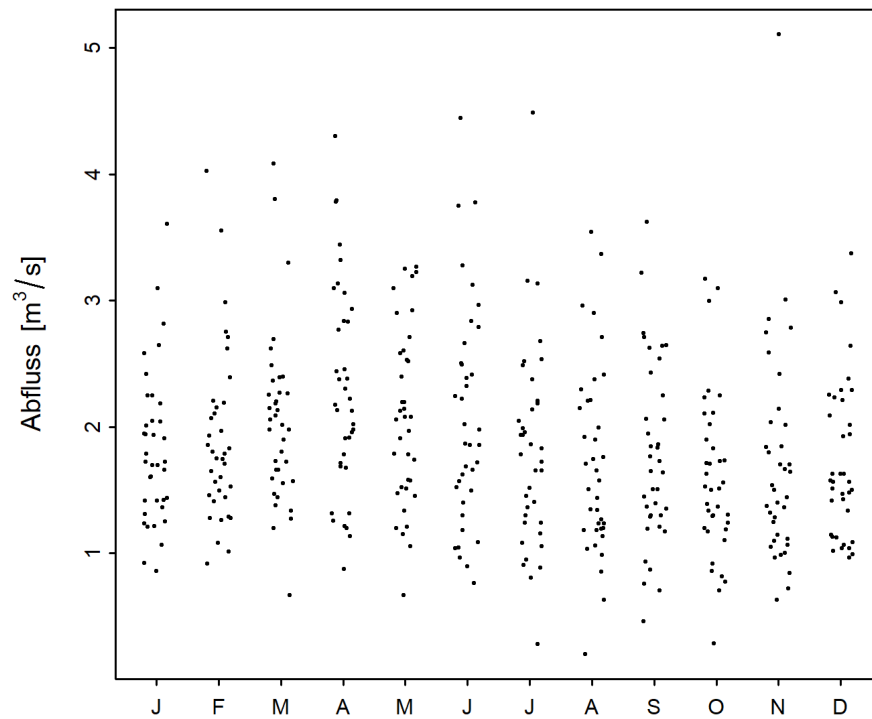
Abbildung 2: Saisonaler Verlauf der monatlichen Minima der M7Q [m³/s] (01.04.1982 - 31.03.2020)
