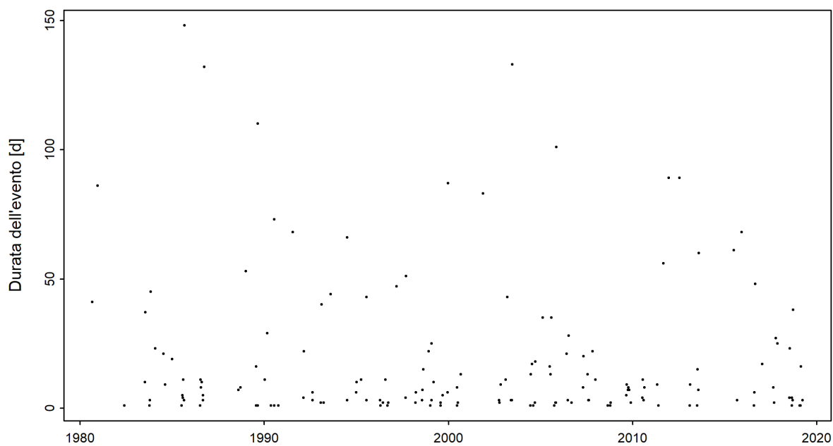
Figura 4: Serie temporale della durata di magra [d] (01.06.1980 - 31.05.2019)
