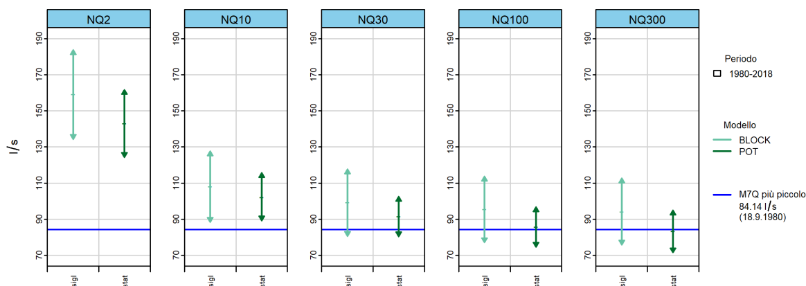
Figura 10: NQ_T [l/s] incl. intervallo di confidenza 95%, calcolato con la variante di modello più adatta degli approcci BLOCK e POT
