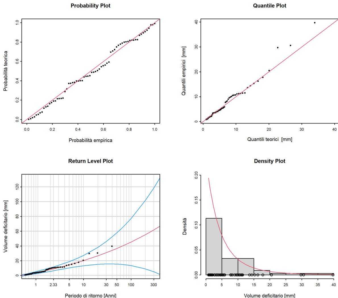
Figura 14: Plot diagnostici della variante di modello "stat" dell'approccio POT (01.06.1980 - 31.05.2019)
