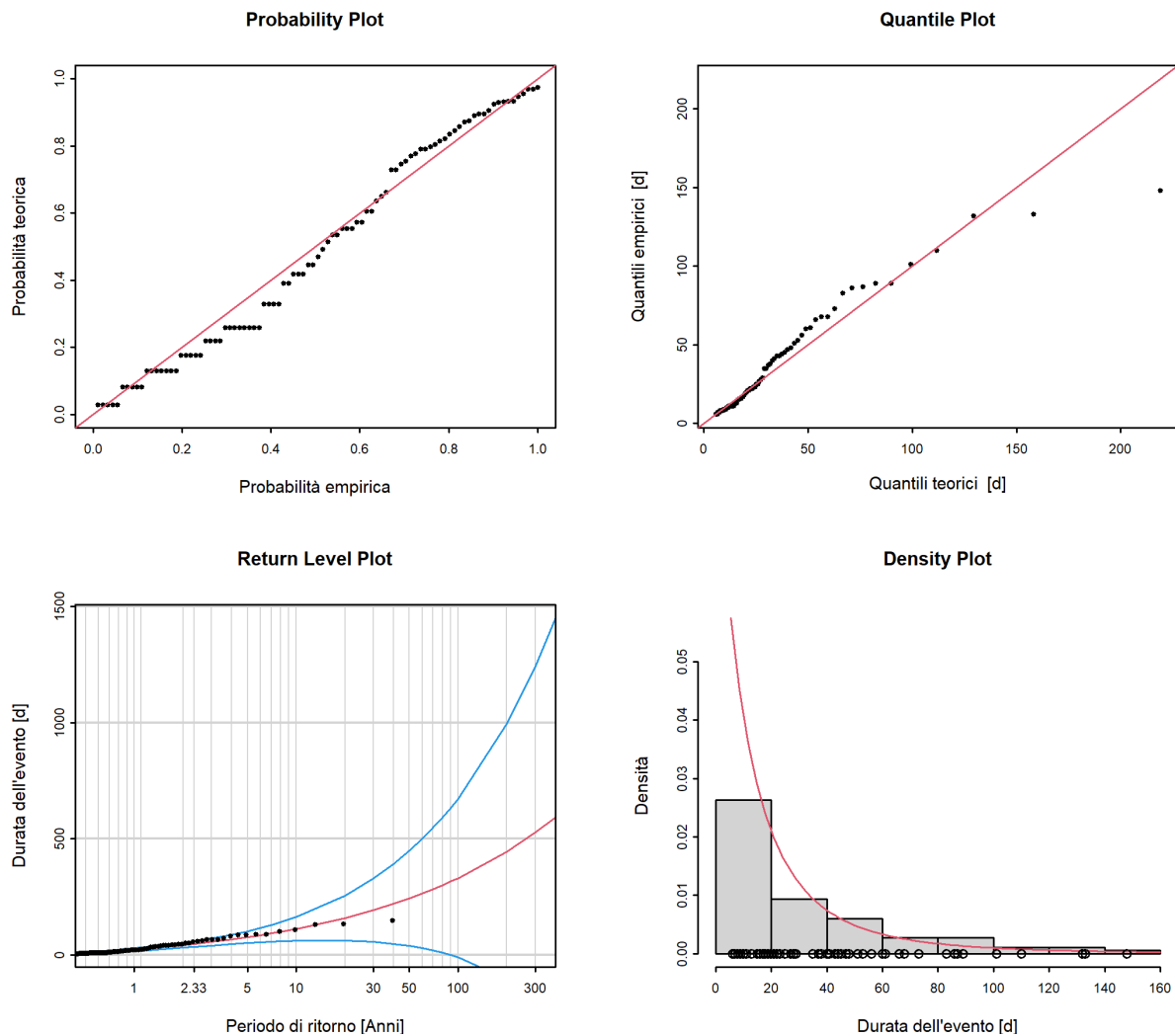
Figura 12: Plot diagnostici della variante di modello "stat" dell'approccio POT (01.06.1980 - 31.05.2019)
