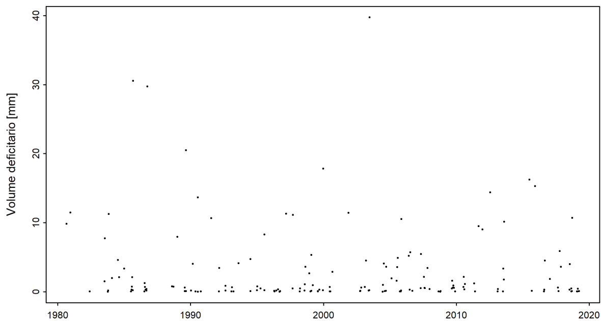
Figura 5: Serie temporale del volume deficitario [mm] (01.06.1980 - 31.05.2019)
