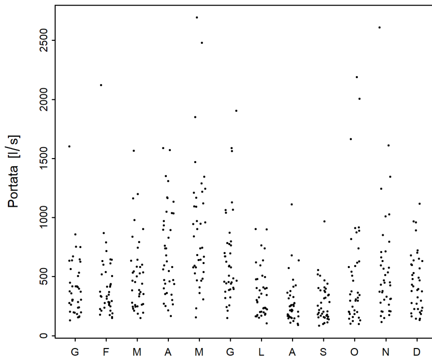
Figura 2: Sviluppo stagionale del minimo mensile di M7Q [l/s] (01.06.1980 - 31.05.2019)
