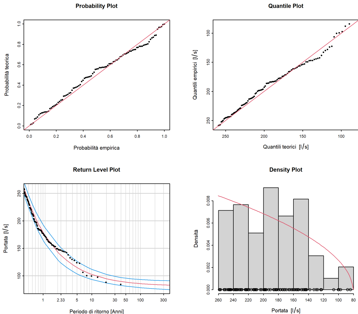
Figura 9: Plot diagnostici della variante di modello "stat" dell'approccio POT (01.06.1980 - 31.05.2019)
