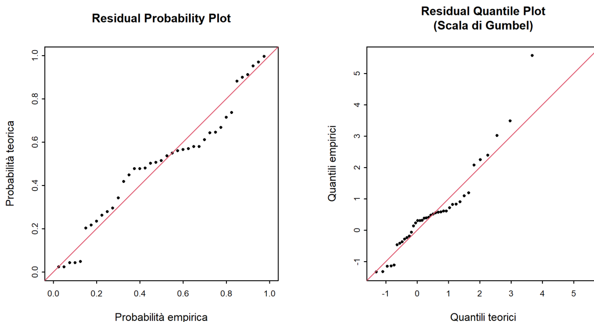
Figura 7: Plot diagnostici della variante di modello "sigl" dell'approccio BLOCK (01.06.1980 - 31.05.2019)
