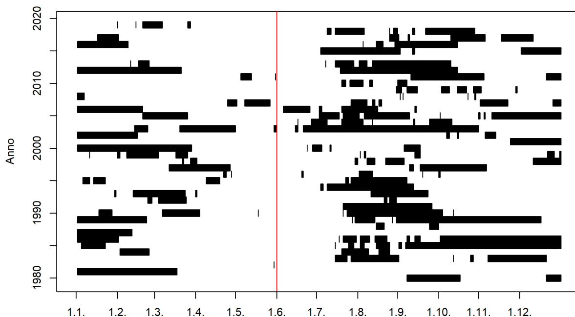
Figura 1: Apparizione temporale dei periodi di magra durante l'anno (01.06.1980 - 31.05.2019) e mese iniziale dell'anno di magra (linea rossa) 1
