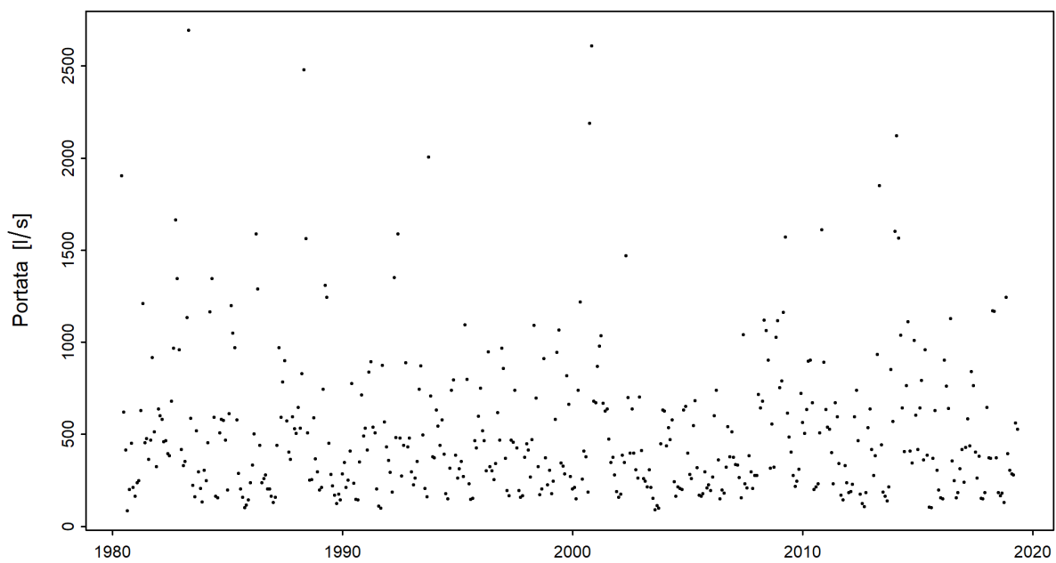
Figura 3: Serie temporale del minimo mensile di M7Q [l/s] (01.06.1980 - 31.05.2019)
