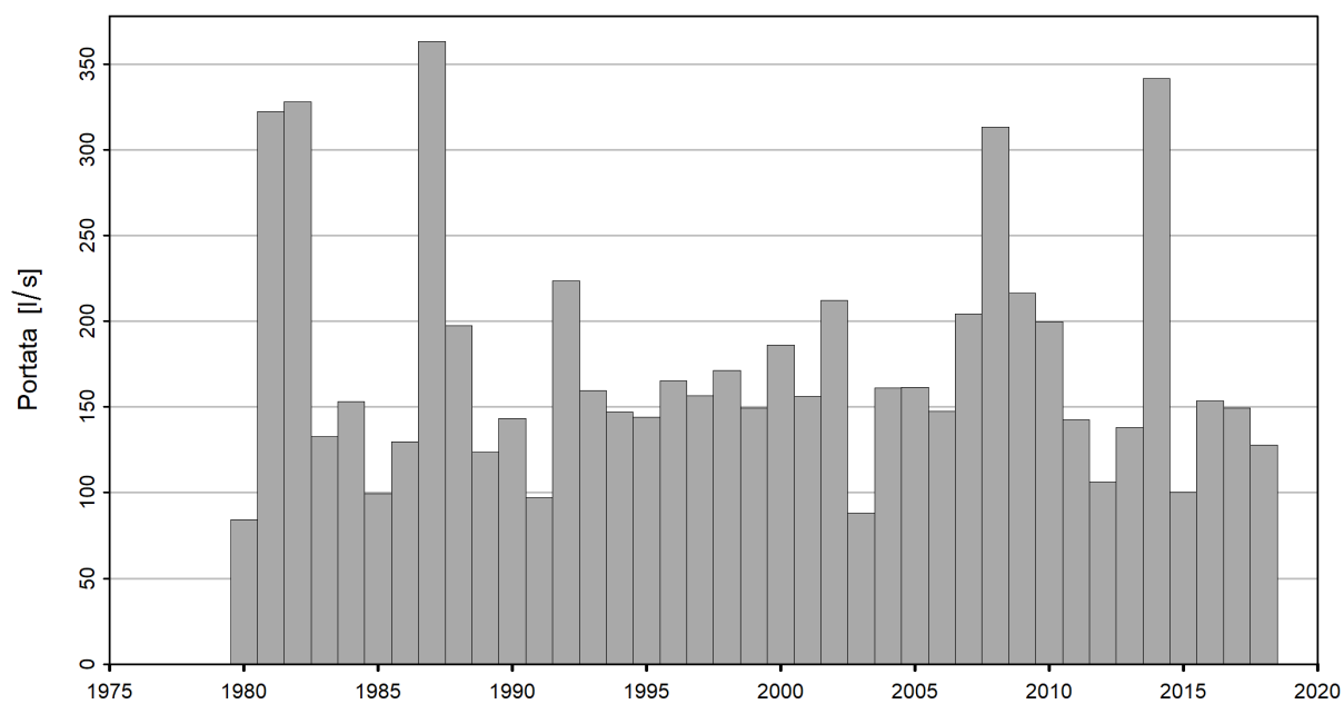
Figura 6: Serie temporale di NM7Q [l/s] (01.06.1980 - 31.05.2019)
