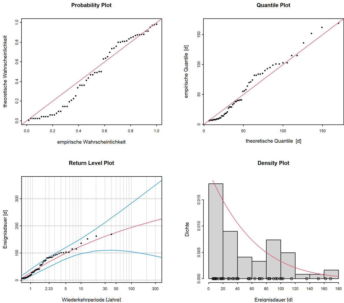
Abbildung 12: Diagnostikplots der Modellvariante “stat” des POT-Ansatzes (01.06.1980 - 31.05.2020)
