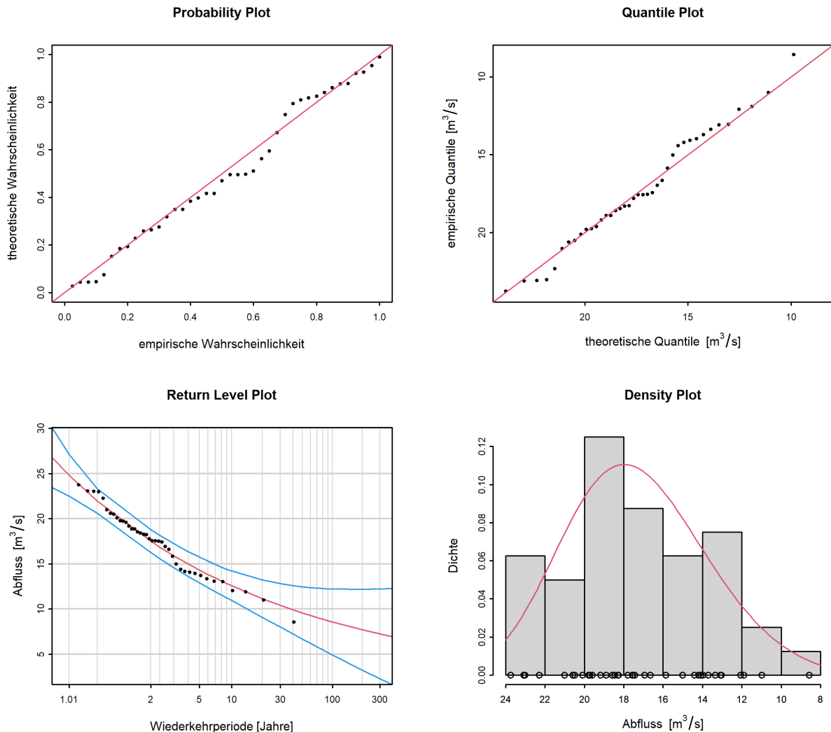
Abbildung 7: Diagnostikplots der Modellvariante "stat" des BLOCK-Ansatzes (01.06.1980 - 31.05.2020)
