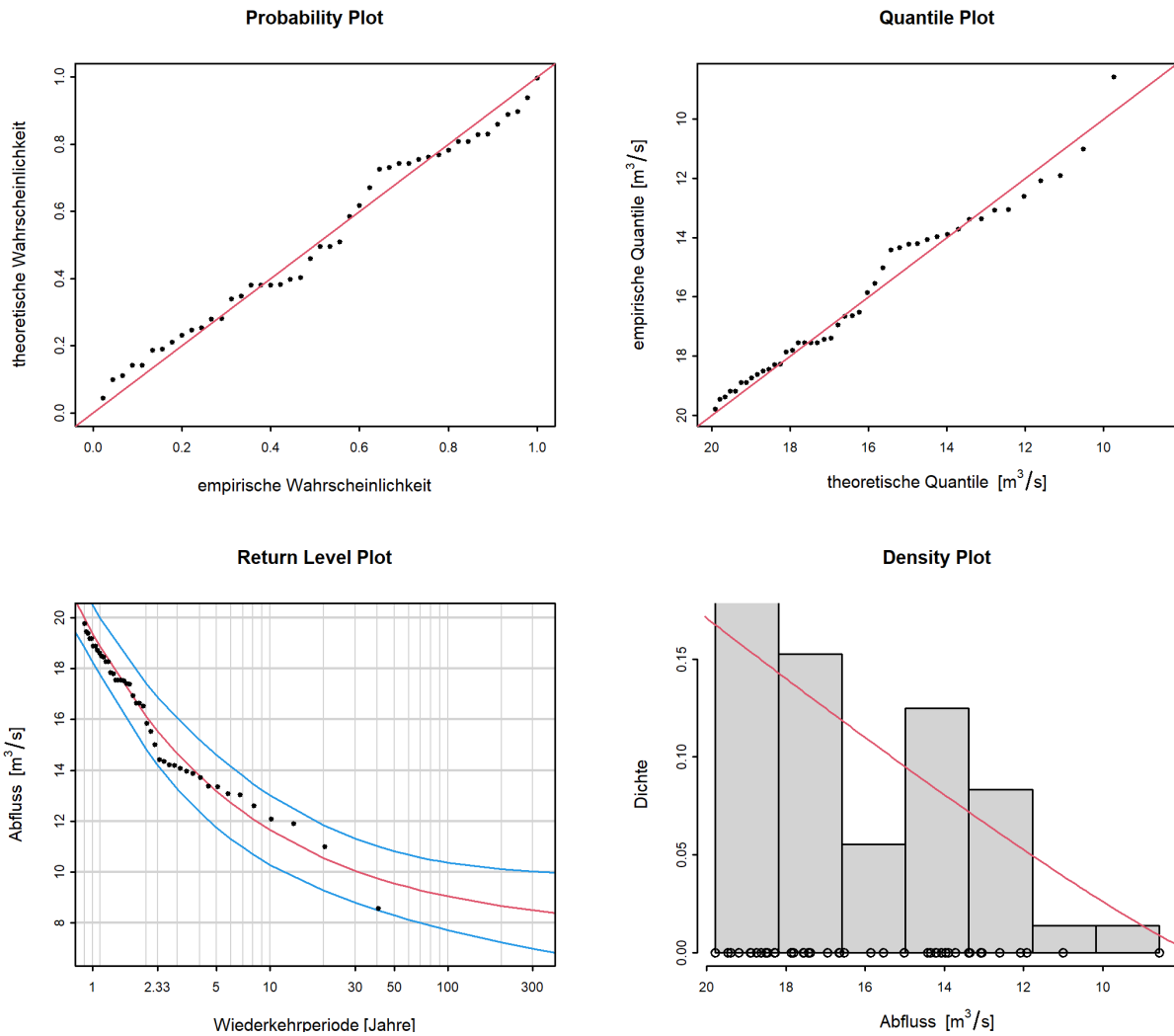
Abbildung 9: Diagnostikplots der Modellvariante "stat" des POT-Ansatzes (01.06.1980 - 31.05.2020)
