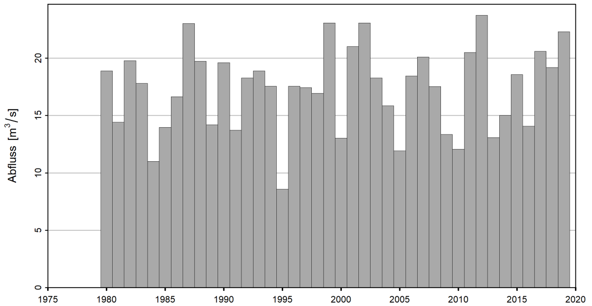
Abbildung 6: Zeitreihe der NM7Q [ \text{m}^3/\text{s} ] (01.06.1980 - 31.05.2020)
