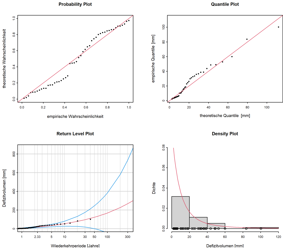
Abbildung 14: Diagnostikplots der Modellvariante “stat” des POT-Ansatzes (01.06.1980 - 31.05.2020)
