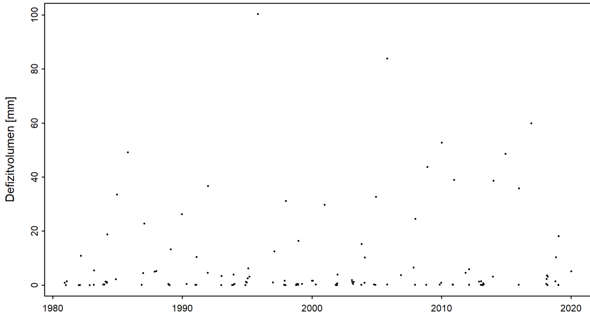
Abbildung 5: Zeitreihe der Defizitvolumen [mm] (01.06.1980 - 31.05.2020)
