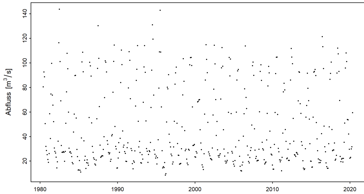
Abbildung 3: Zeitreihe der monatlichen Minima der M7Q [m³/s] (01.06.1980 - 31.05.2020)
