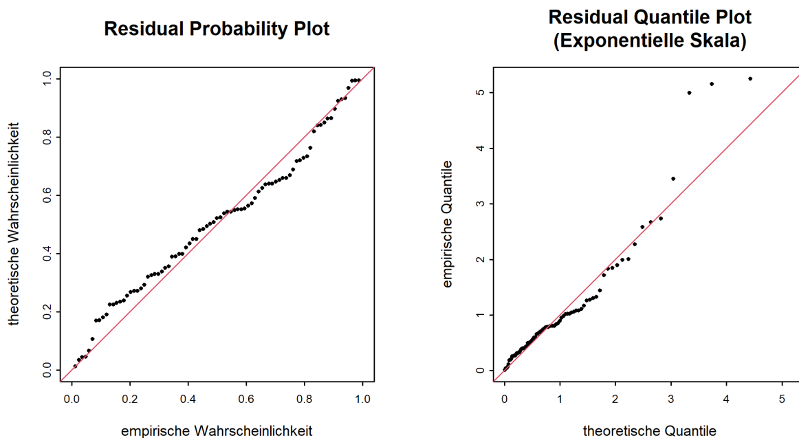
Abbildung 9: Diagnostikplots der Modellvariante “sigjump2003” des POT-Ansatzes (01.04.1979 - 31.03.2020)
