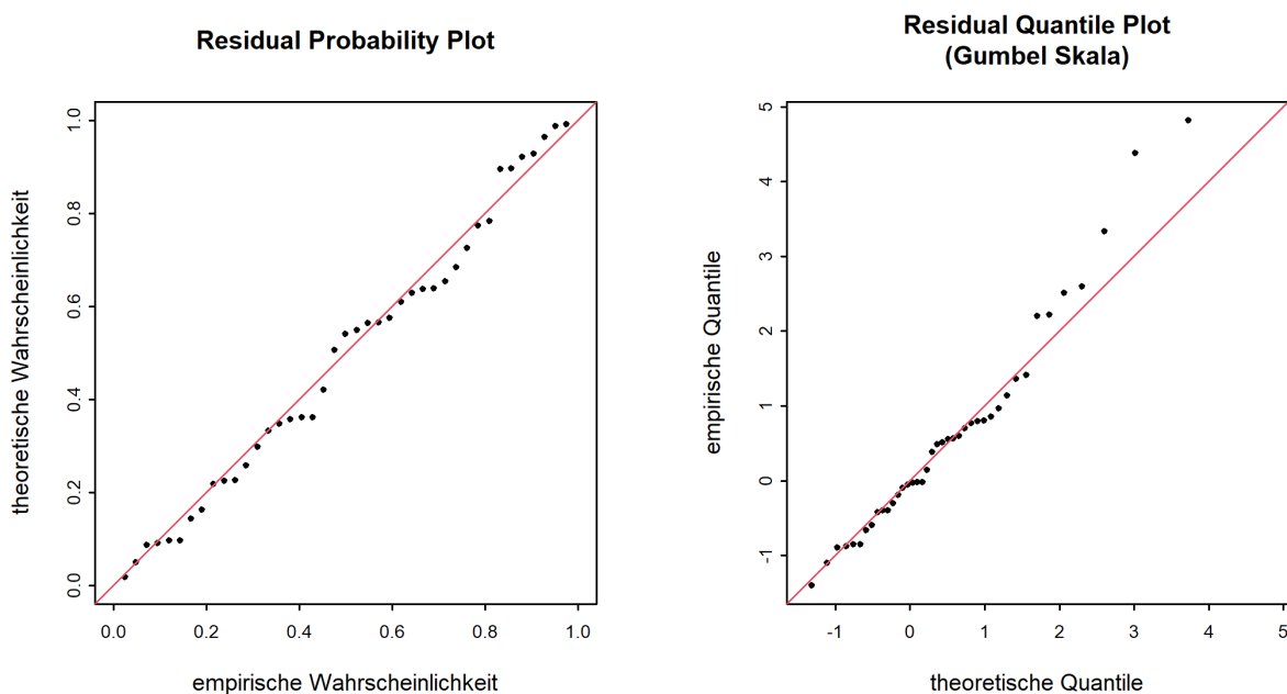
Abbildung 7: Diagnostikplots der Modellvariante "mujump2003" des BLOCK-Ansatzes (01.04.1979 - 31.03.2020)
