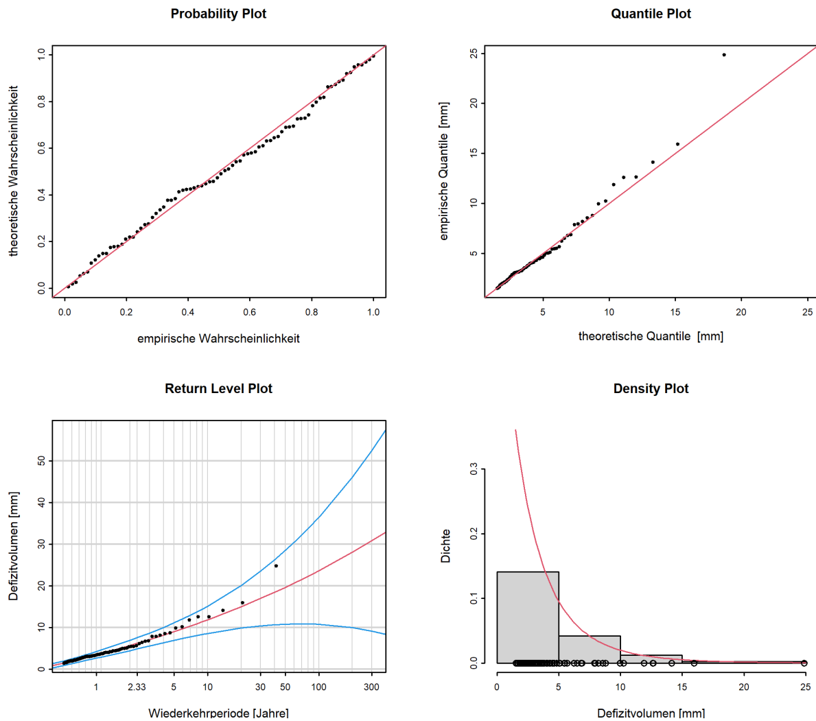
Abbildung 14: Diagnostikplots der Modellvariante “stat” des POT-Ansatzes (01.04.1979 - 31.03.2020)
