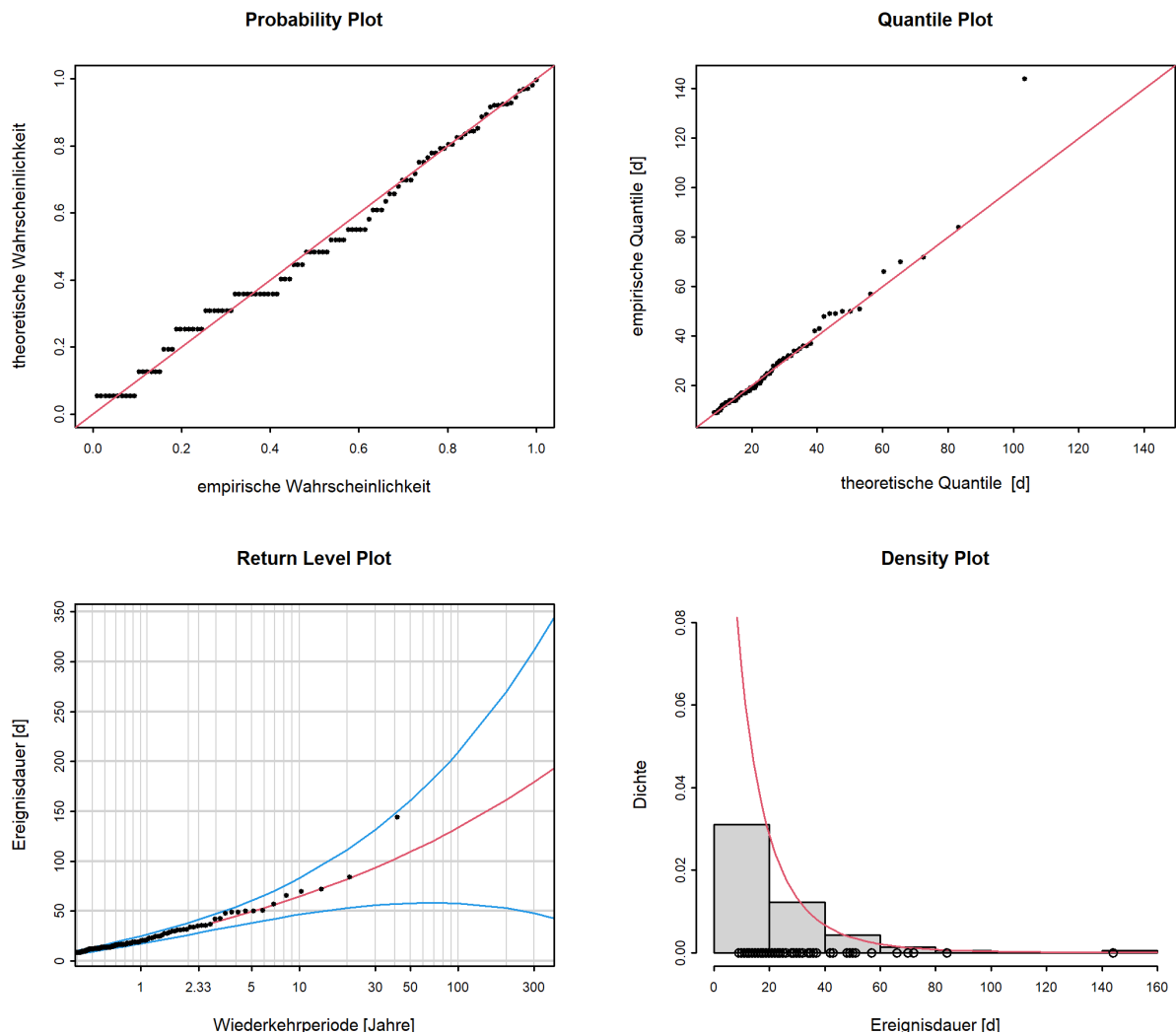
Abbildung 12: Diagnostikplots der Modellvariante “stat” des POT-Ansatzes (01.04.1979 - 31.03.2020)
