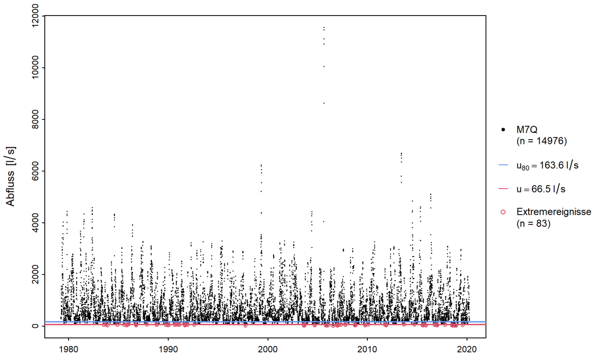
Abbildung 8: Auswahl der für den POT-Ansatz verwendeten Extremereignisse
