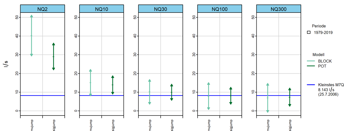
Abbildung 10: NQ_T [l/s] inkl. 95%-Konfidenzintervalle, berechnet mit den jeweils bestangepassten Modellvarianten des BLOCK- und POT-Ansatzes
