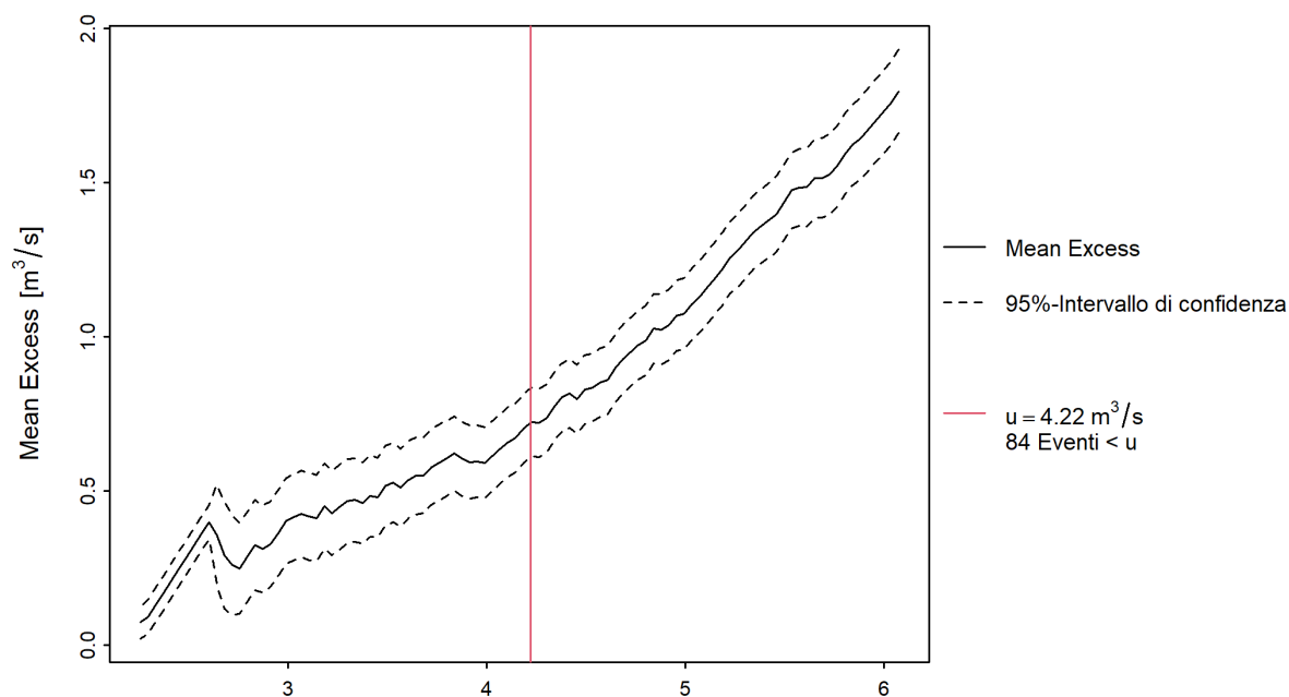
Figura 15: "mean residual life plot" per la portata di magra
