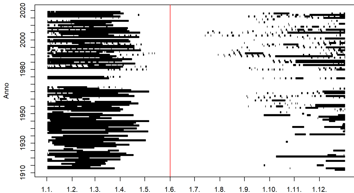
Figura 1: Apparizione temporale dei periodi di magra durante l'anno (01.06.1912 - 31.05.2019) e mese iniziale dell'anno di magra (linea rossa) 1
