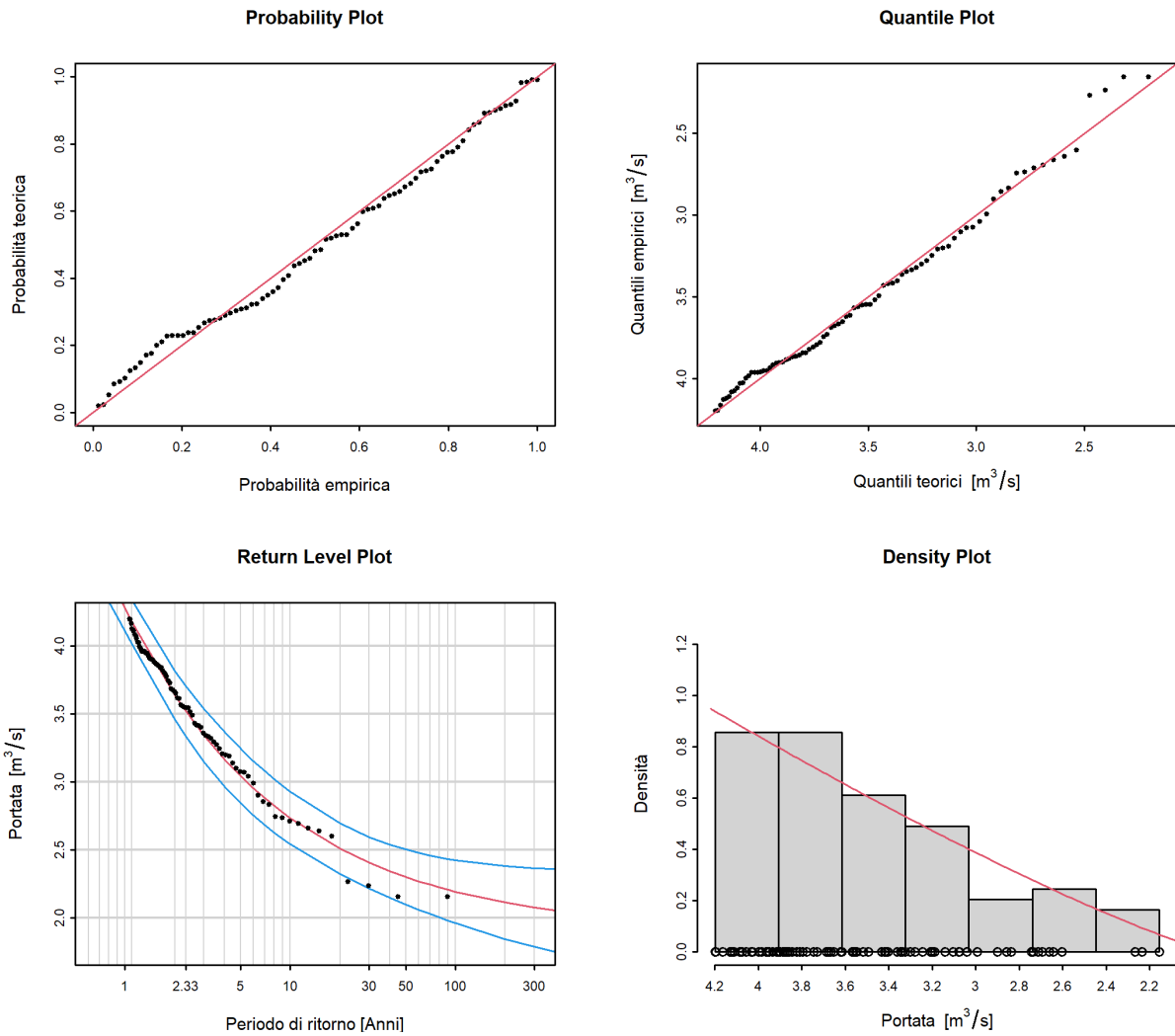
Figura 9: Plot diagnostici della variante di modello "stat" dell'approccio POT (01.06.1921 - 31.05.2019)
