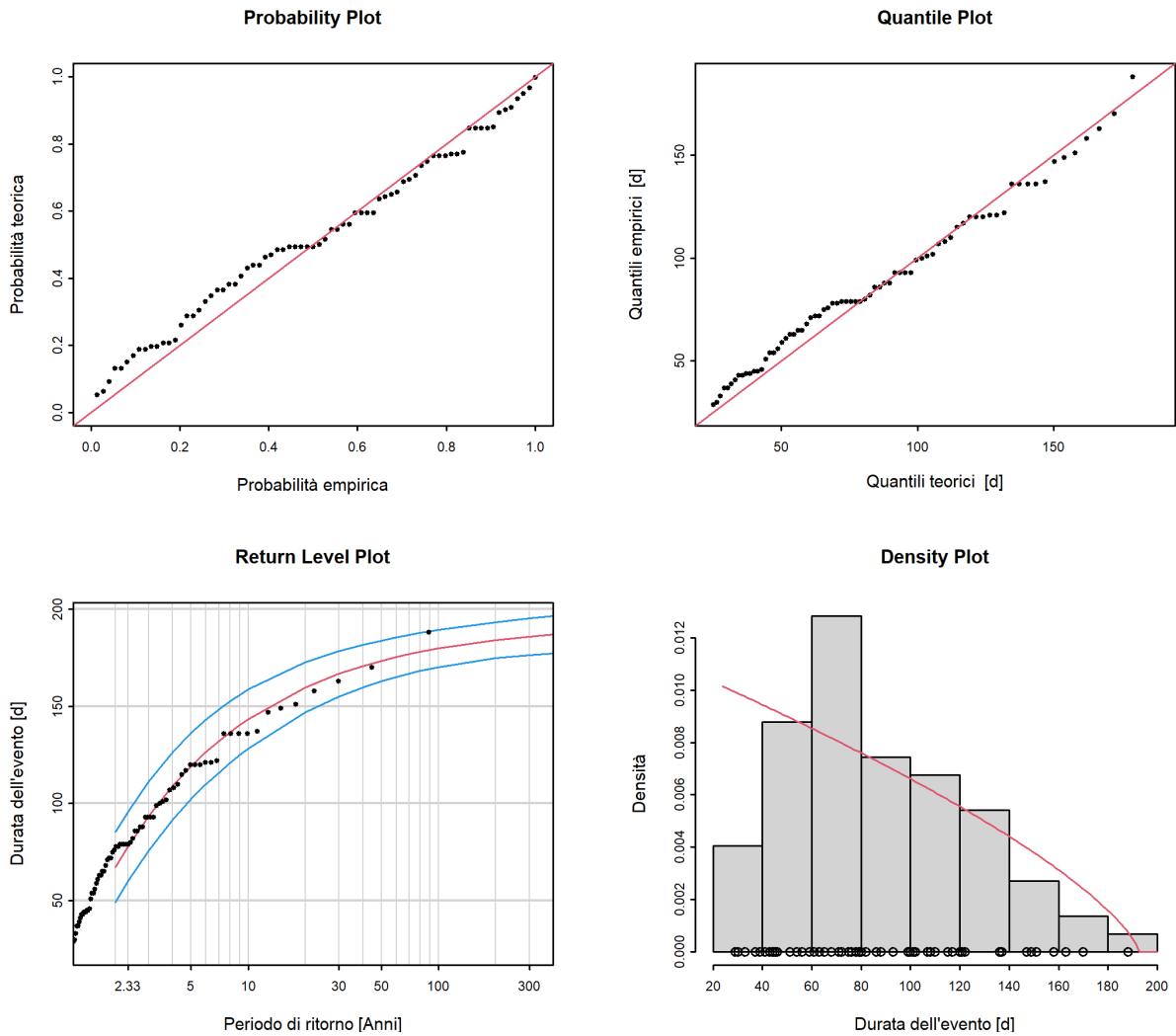
Figura 12: Plot diagnostici della variante di modello "stat" dell'approccio POT (01.06.1921 - 31.05.2019)
