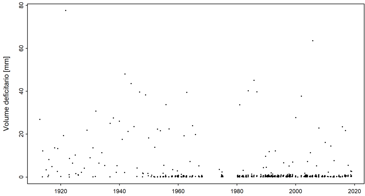
Figura 5: Serie temporale del volume deficitario [mm] (01.06.1912 - 31.05.2019)
