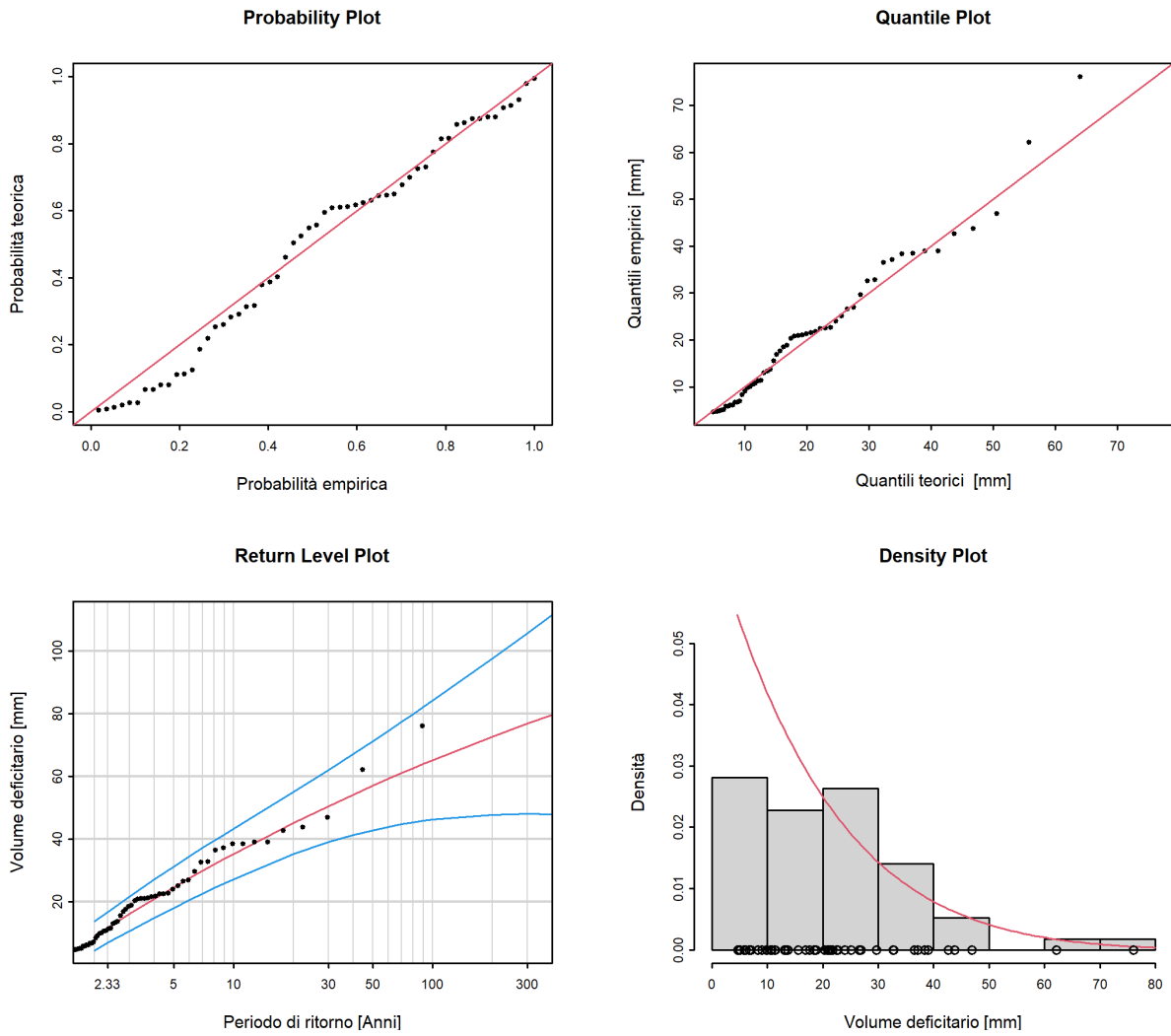
Figura 14: Plot diagnostici della variante di modello "stat" dell'approccio POT (01.06.1921 - 31.05.2019)
