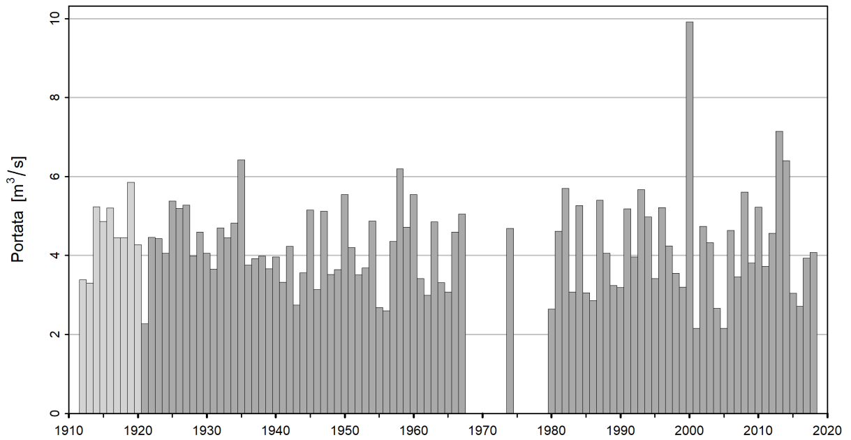
Figura 6: Serie temporale di NM7Q [ \text{m}^3/\text{s} ] (01.06.1912 - 31.05.2019), grigio chiaro: NM7Q non utilizzati, grigio scuro: NM7Q utilizzati
