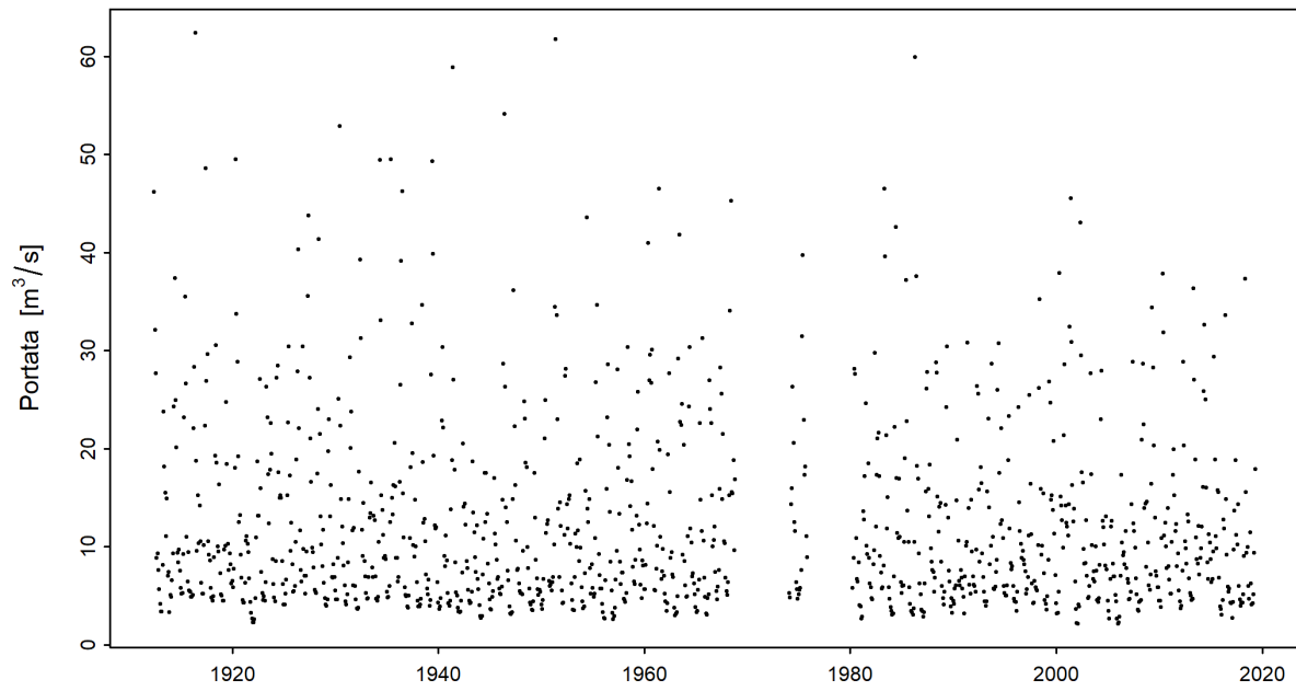
Figura 3: Serie temporale del minimo mensile di M7Q [ \text{m}^3/\text{s} ] (01.06.1912 - 31.05.2019)
