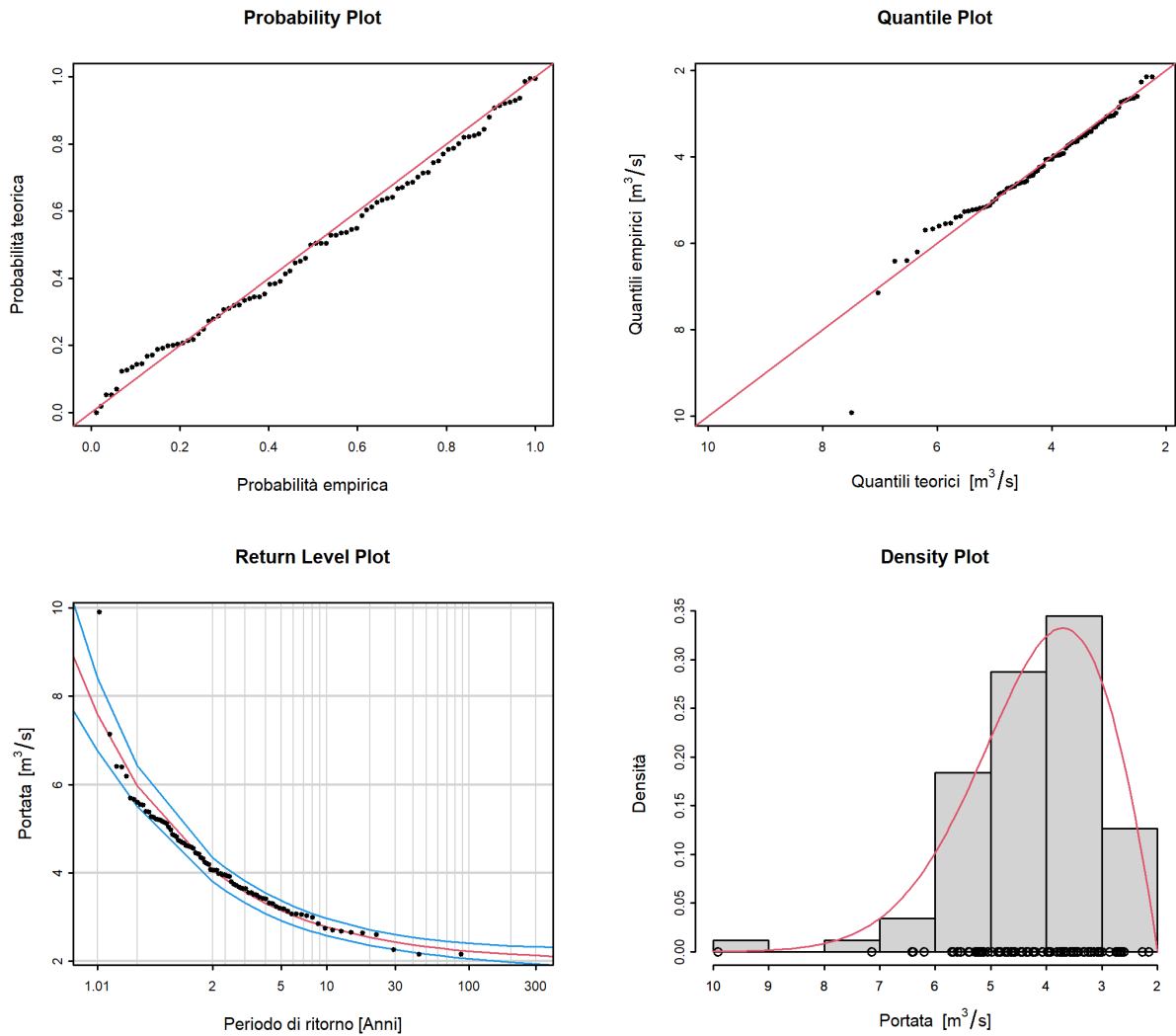
Figura 7: Plot diagnostici della variante di modello "stat" dell'approccio BLOCK (01.06.1921 - 31.05.2019)
