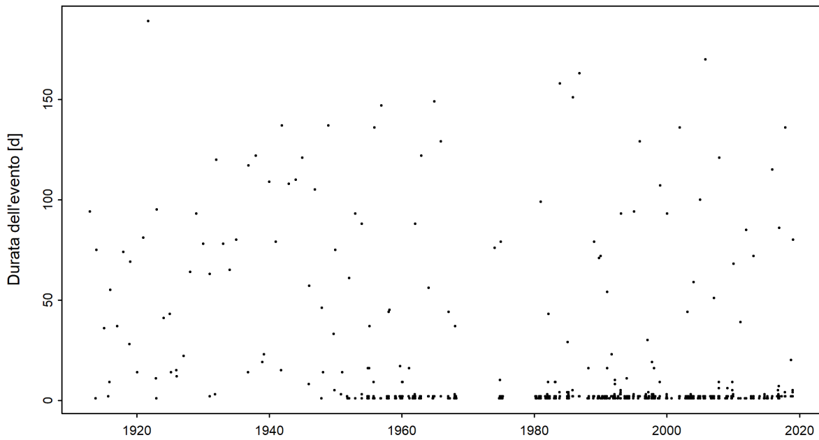
Figura 4: Serie temporale della durata di magra [d] (01.06.1912 - 31.05.2019)
