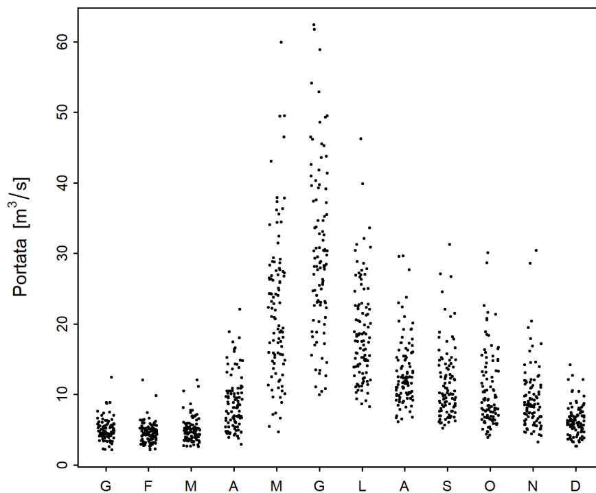
Figura 2: Sviluppo stagionale del minimo mensile di M7Q [ \text{m}^3/\text{s} ] (01.06.1912 - 31.05.2019)
