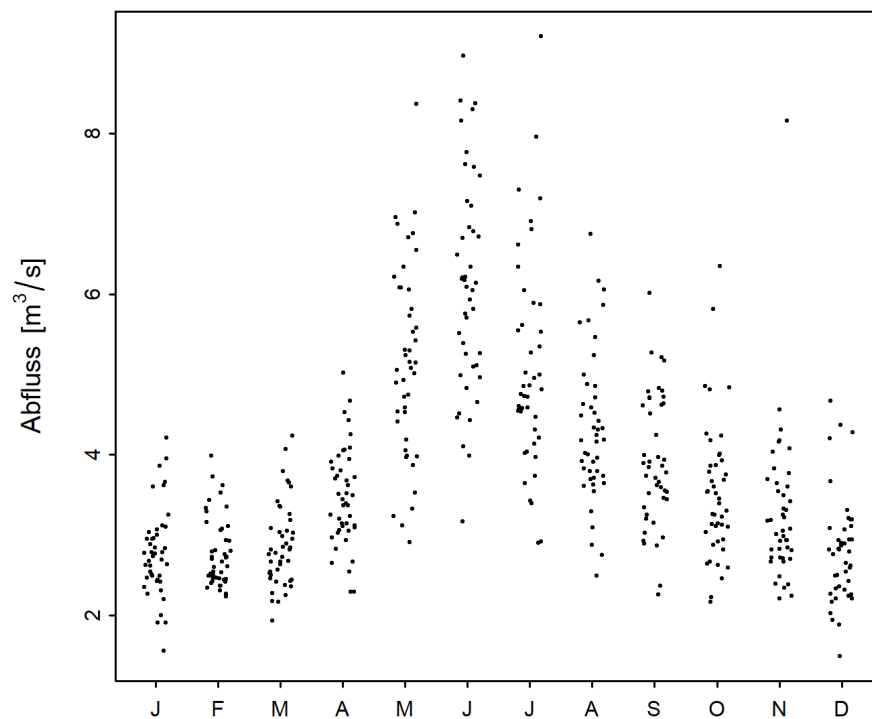
Abbildung 2: Saisonaler Verlauf der monatlichen Minima der M7Q [ \text{m}^3/\text{s} ] (01.06.1975 - 31.05.2019)
