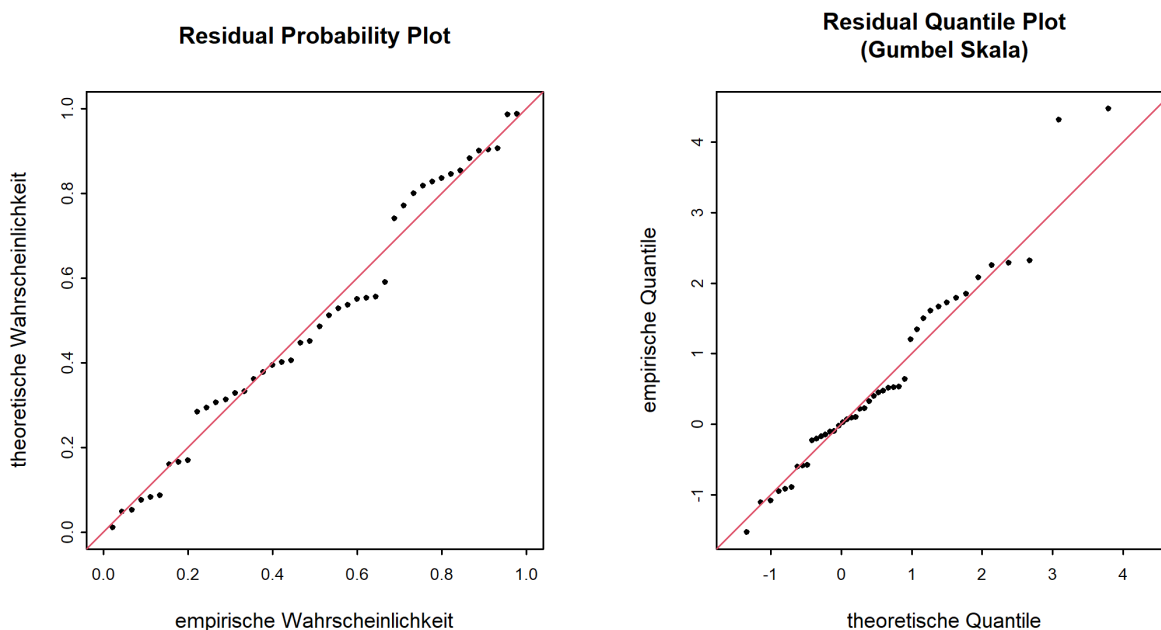
Abbildung 7: Diagnostikplots der Modellvariante "mujump2003" des BLOCK-Ansatzes (01.06.1975 - 31.05.2019)
