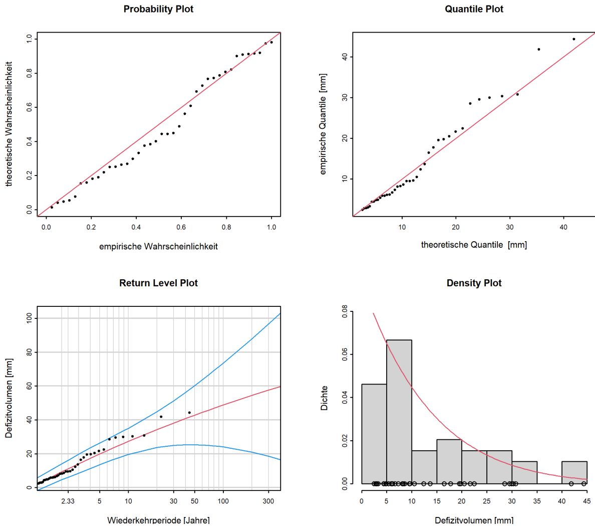
Abbildung 14: Diagnostikplots der Modellvariante "stat" des POT-Ansatzes (01.06.1975 - 31.05.2019)
