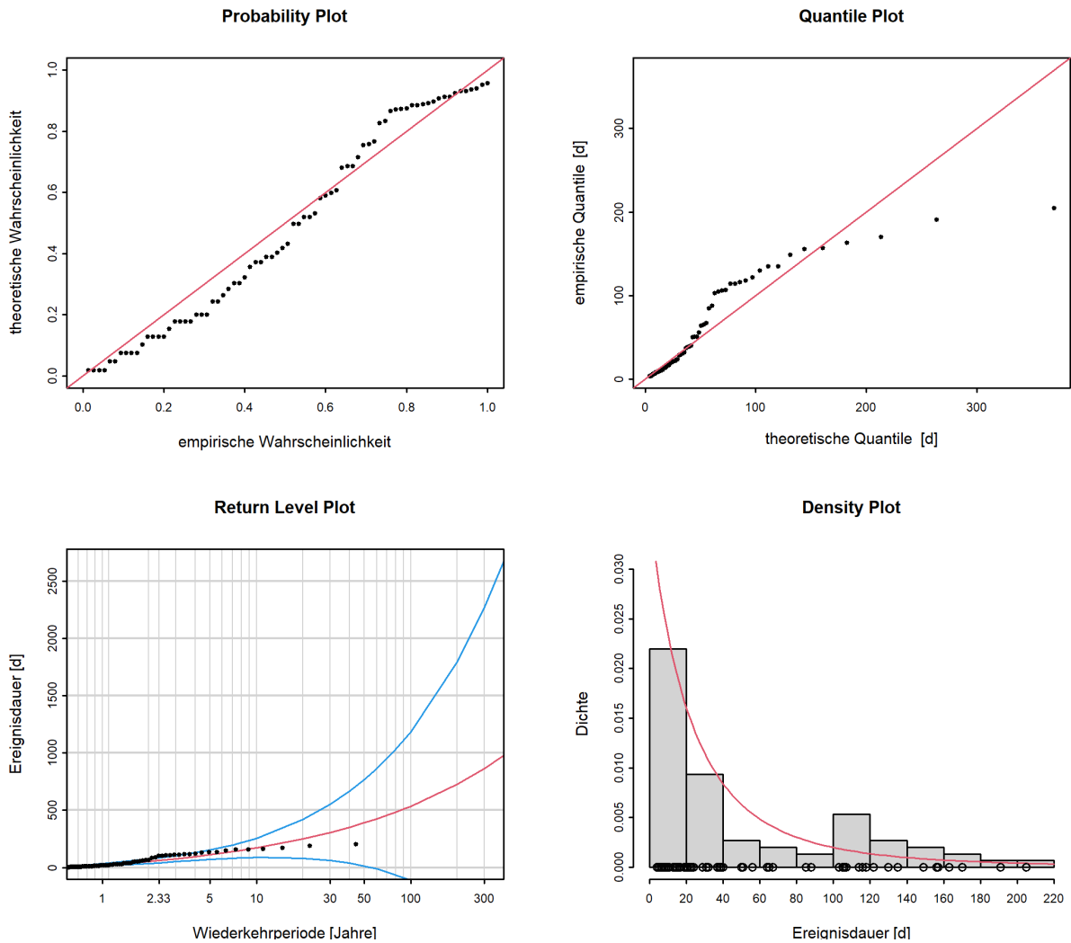
Abbildung 12: Diagnostikplots der Modellvariante “stat” des POT-Ansatzes (01.06.1975 - 31.05.2019)
