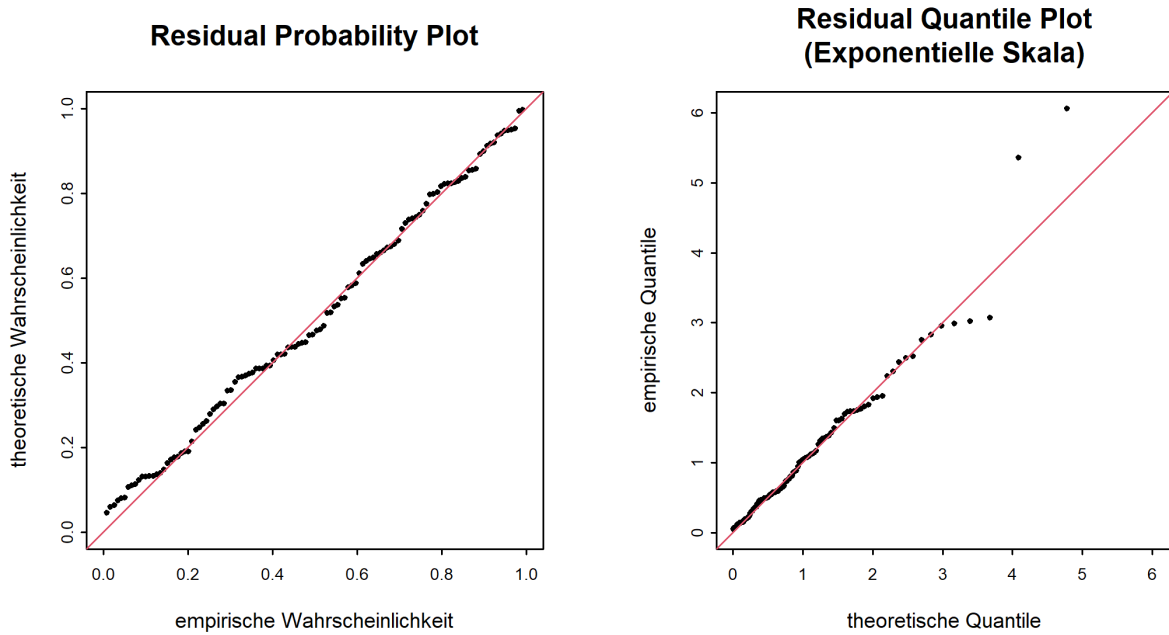
Abbildung 9: Diagnostikplots der Modellvariante “sigjump2003” des POT-Ansatzes (01.06.1975 - 31.05.2019)
