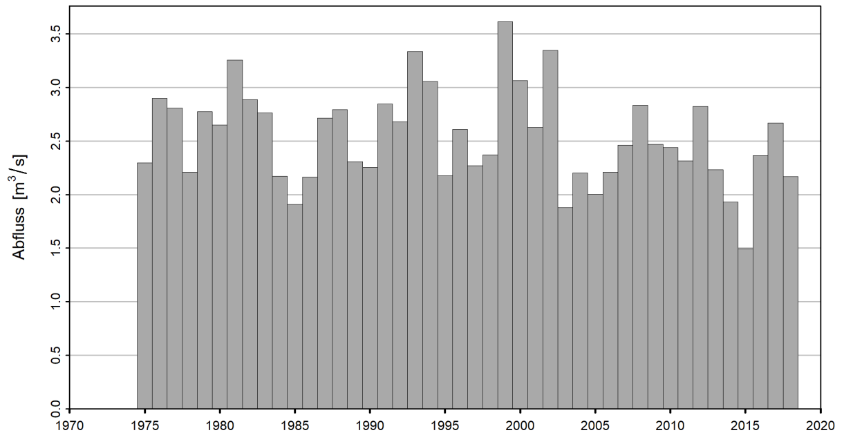
Abbildung 6: Zeitreihe der NM7Q [ m^3/s ] (01.06.1975 - 31.05.2019)
