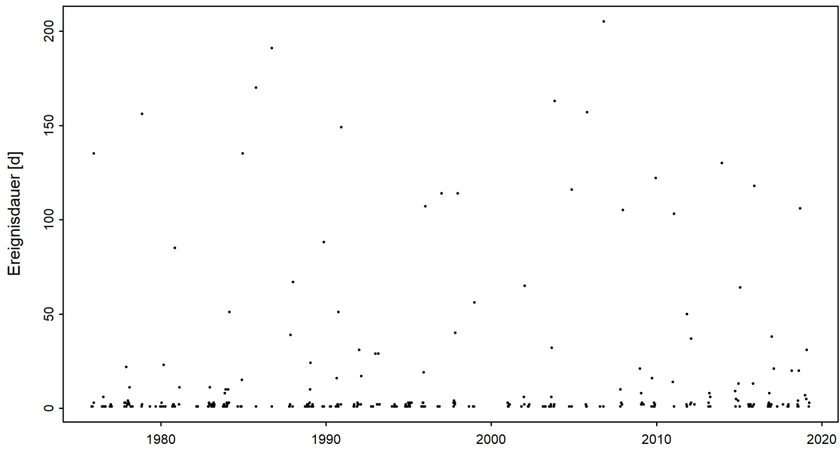
Abbildung 4: Zeitreihe der Niedrigwasserdauern [d] (01.06.1975 - 31.05.2019)
