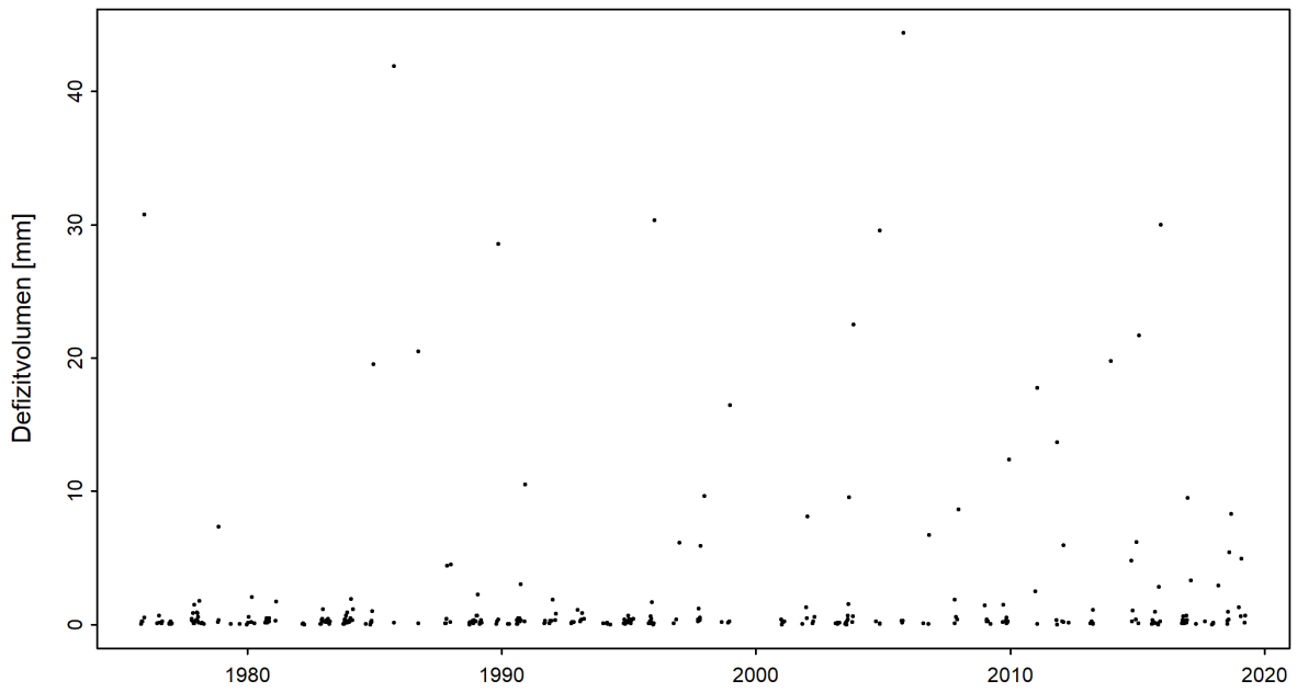
Abbildung 5: Zeitreihe der Defizitvolumen [mm] (01.06.1975 - 31.05.2019)
