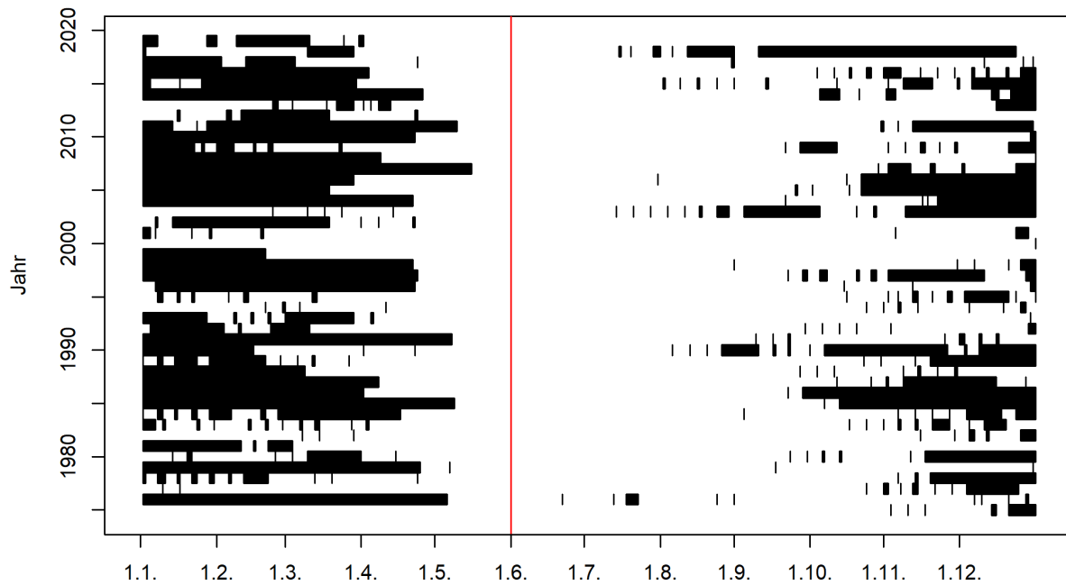
Abbildung 1: Zeitliches Auftreten der Niedrigwasserperioden im Jahresverlauf (01.06.1975 - 31.05.2019) und Startmonat des Niedrigwasserjahres (rote Linie) 1
