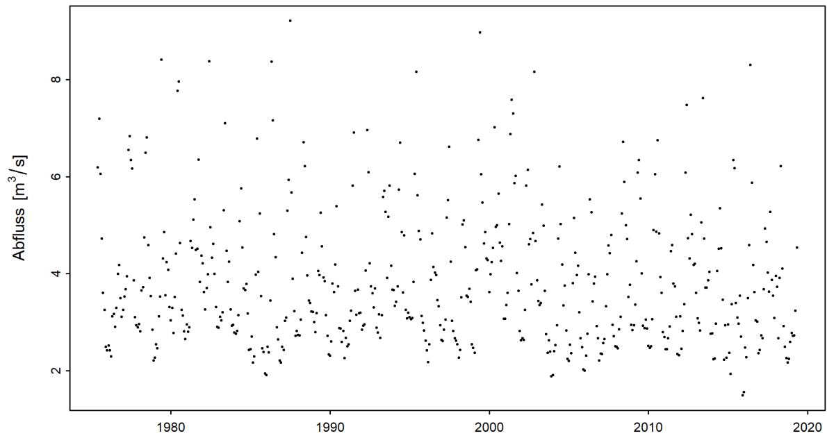
Abbildung 3: Zeitreihe der monatlichen Minima der M7Q [ \text{m}^3/\text{s} ] (01.06.1975 - 31.05.2019)
