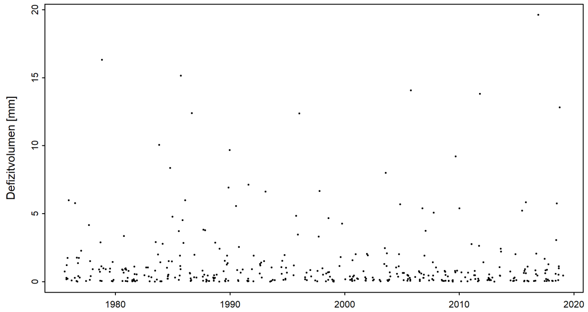
Abbildung 5: Zeitreihe der Defizitvolumen [mm] (01.04.1975 - 31.03.2019)
