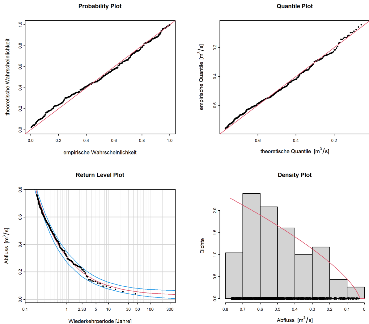
Abbildung 9: Diagnostikplots der Modellvariante “stat” des POT-Ansatzes (01.04.1975 - 31.03.2019)
