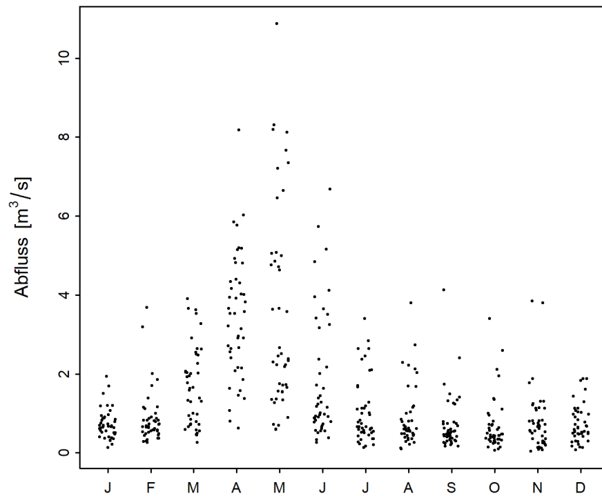
Abbildung 2: Saisonaler Verlauf der monatlichen Minima der M7Q [m³/s] (01.04.1975 - 31.03.2019)
