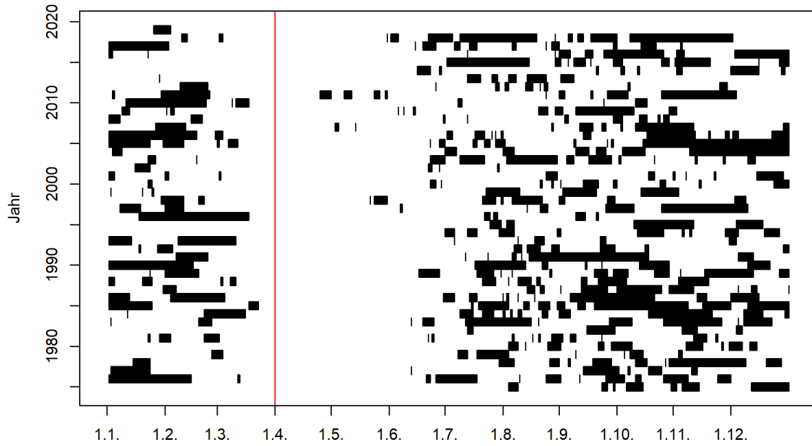
Abbildung 1: Zeitliches Auftreten der Niedrigwasserperioden im Jahresverlauf (01.04.1975 - 31.03.2019) und Startmonat des Niedrigwasserjahres (rote Linie) 1
