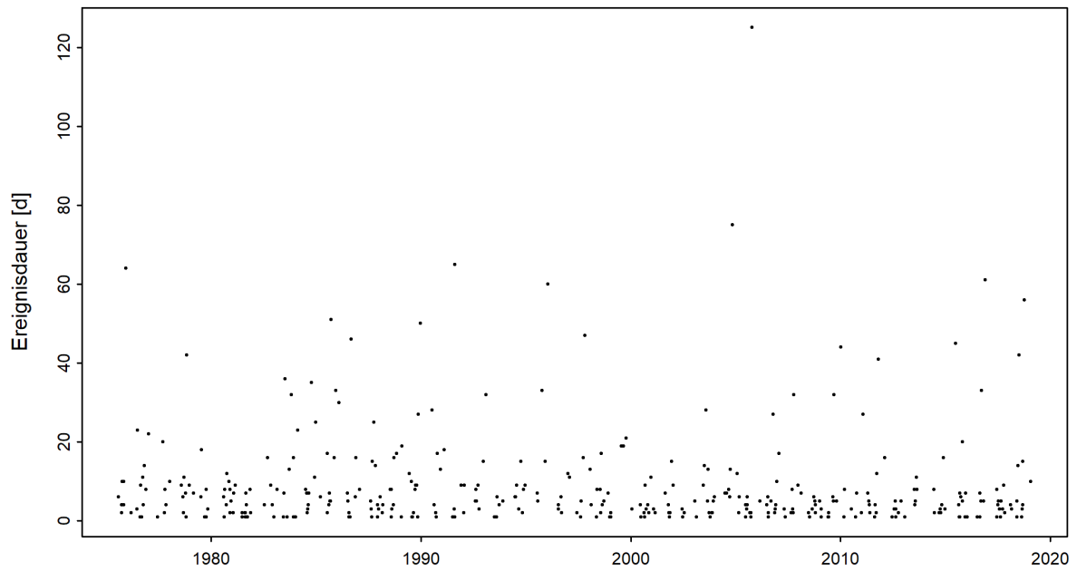
Abbildung 4: Zeitreihe der Niedrigwasserdauern [d] (01.04.1975 - 31.03.2019)
