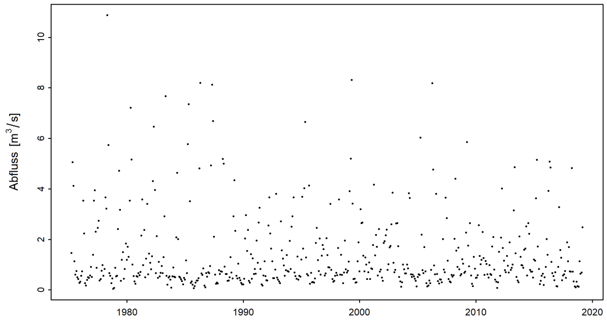
Abbildung 3: Zeitreihe der monatlichen Minima der M7Q [ \text{m}^3/\text{s} ] (01.04.1975 - 31.03.2019)
