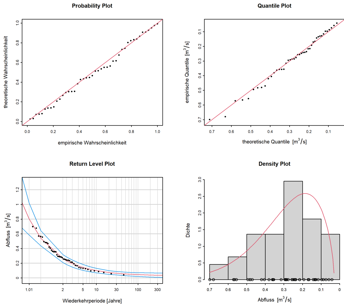
Abbildung 7: Diagnostikplots der Modellvariante "stat" des BLOCK-Ansatzes (01.04.1975 - 31.03.2019)
