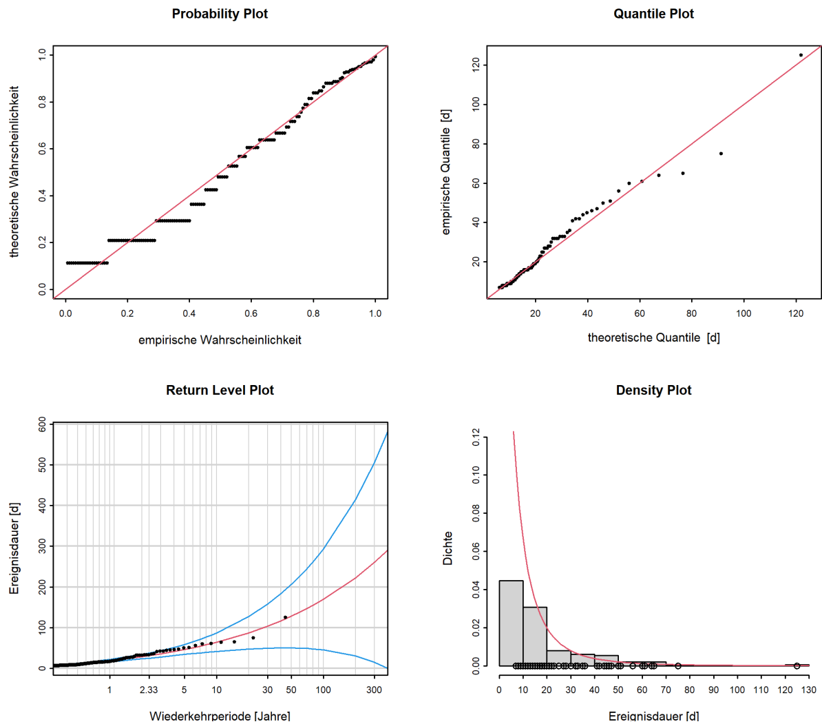
Abbildung 12: Diagnostikplots der Modellvariante "stat" des POT-Ansatzes (01.04.1975 - 31.03.2019)
