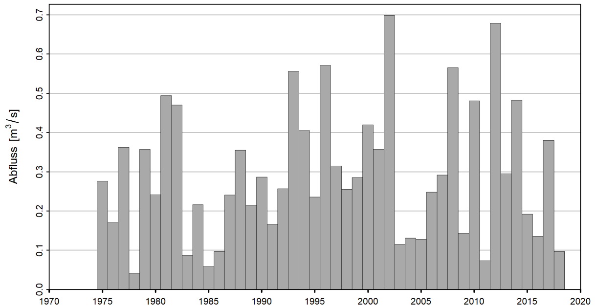
Abbildung 6: Zeitreihe der NM7Q [m³/s] (01.04.1975 - 31.03.2019)
