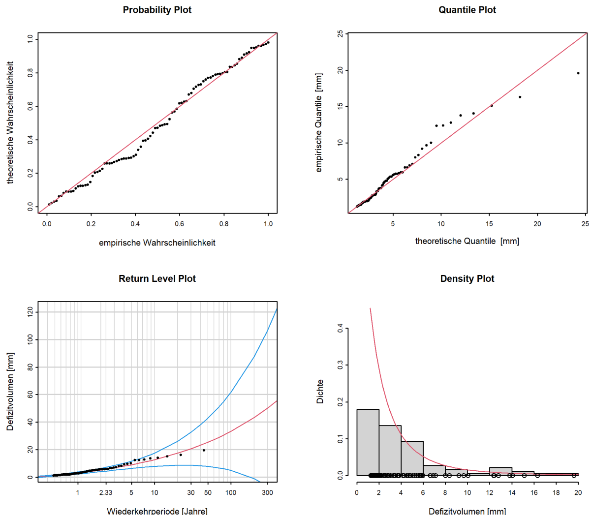
Abbildung 14: Diagnostikplots der Modellvariante "stat" des POT-Ansatzes (01.04.1975 - 31.03.2019)
