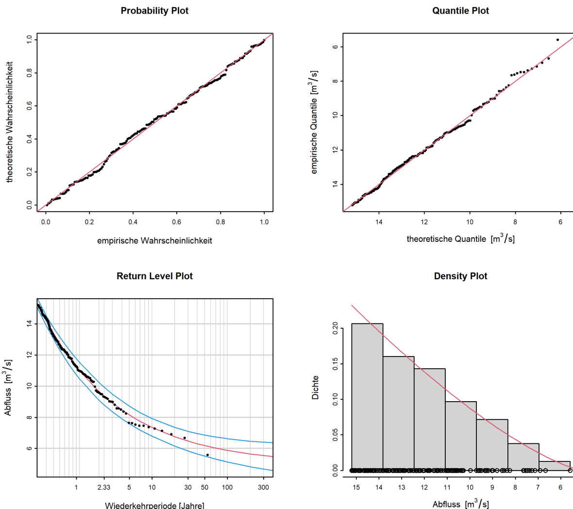
Abbildung 9: Diagnostikplots der Modellvariante “stat” des POT-Ansatzes (01.06.1965 - 31.05.2019)
