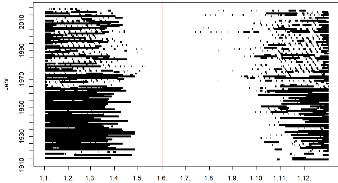
Abbildung 1: Zeitliches Auftreten der Niedrigwasserperioden im Jahresverlauf (01.06.1914 - 31.05.2019) und Startmonat des Niedrigwasserjahres (rote Linie) 1
