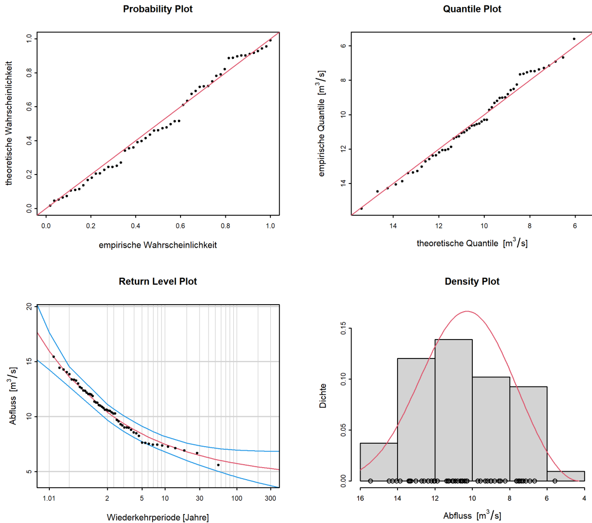
Abbildung 7: Diagnostikplots der Modellvariante "stat" des BLOCK-Ansatzes (01.06.1965 - 31.05.2019)
