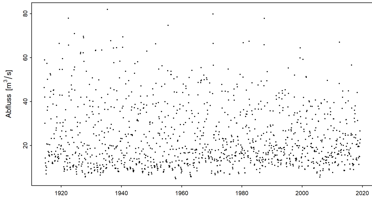
Abbildung 3: Zeitreihe der monatlichen Minima der M7Q [ \text{m}^3/\text{s} ] (01.06.1914 - 31.05.2019)
