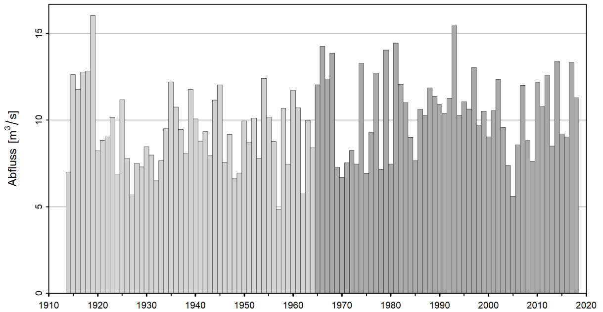
Abbildung 6: Zeitreihe der NM7Q [ \text{m}^3/\text{s} ] (01.06.1914 - 31.05.2019), hellgrau: nicht verwendete NM7Q, dunkelgrau: verwendete NM7Q
