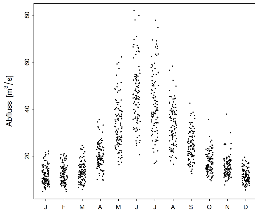
Abbildung 2: Saisonaler Verlauf der monatlichen Minima der M7Q [ \text{m}^3/\text{s} ] (01.06.1914 - 31.05.2019)
