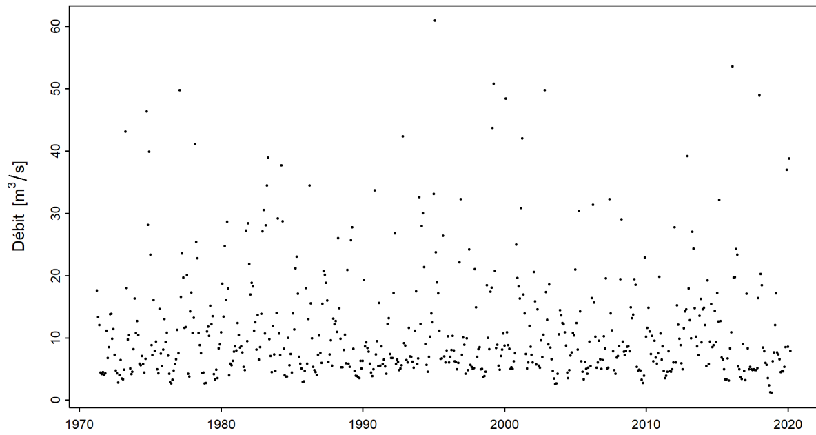
FIGURE 3 – Série temporelle du minimum mensuel de M7Q [ \text{m}^3/\text{s} ] (01.04.1971 - 31.03.2020)
