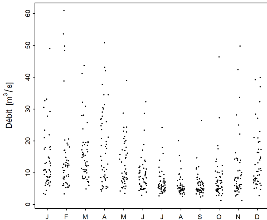
FIGURE 2 – Évolution saisonnière du minimum mensuel de M7Q [ \text{m}^3/\text{s} ] (01.04.1971 - 31.03.2020)
