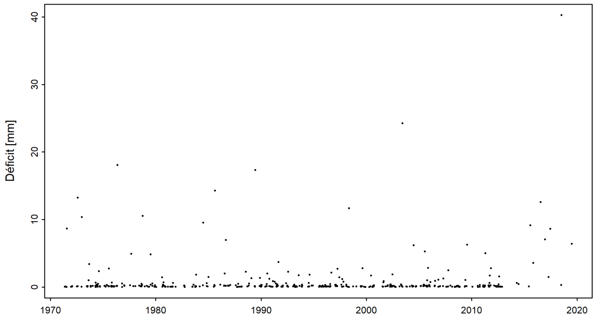
FIGURE 5 – Série temporelle du volume déficitaire [mm] (01.04.1971 - 31.03.2020)
