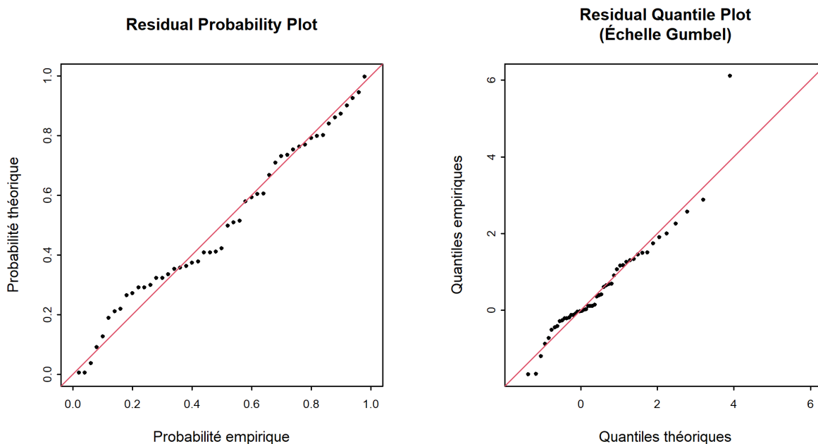
FIGURE 7 – Graphiques diagnostiques de la variante du modèle " mujump1981 " de la méthode BLOCK (01.04.1971 - 31.03.2020)
