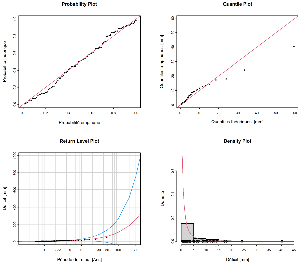
FIGURE 14 – Graphiques diagnostiques de la variante du modèle “ stat ” de la méthode POT (01.04.1971 - 31.03.2020)
