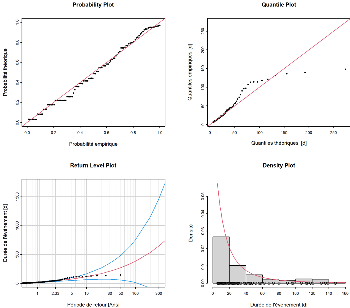
FIGURE 12 – Graphiques diagnostiques de la variante du modèle “ stat ” de la méthode POT (01.04.1971 - 31.03.2020)
