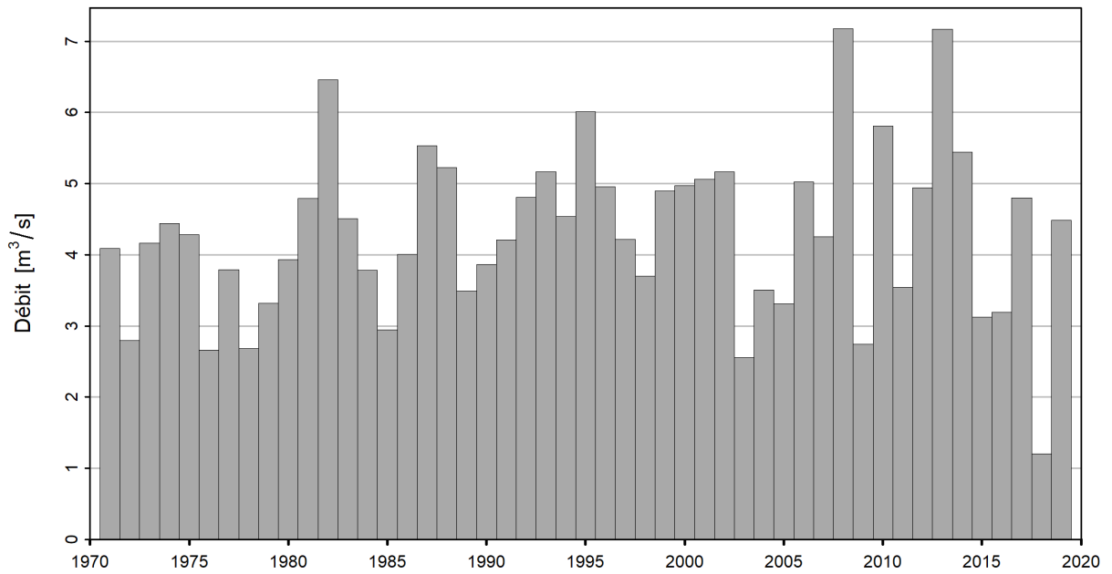
FIGURE 6 – Série temporelle de NM7Q [m 3 /s] (01.04.1971 - 31.03.2020)
