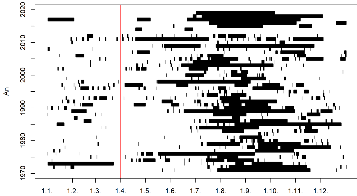
FIGURE 1 – Apparition temporelle des périodes d’étéage pendant l’année (01.04.1971 - 31.03.2020) et mois de début de l’année d’étéage (ligne rouge) 1
