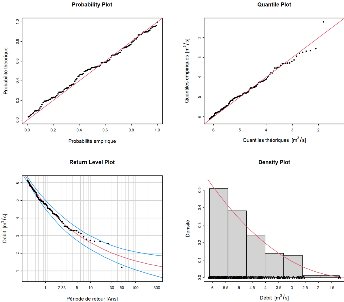
FIGURE 9 – Graphiques diagnostiques de la variante du modèle “ stat ” de la méthode POT (01.04.1971 - 31.03.2020)
