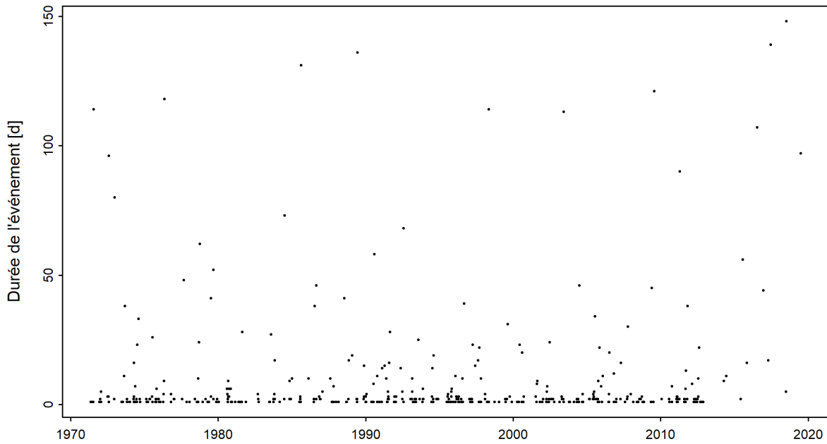
FIGURE 4 – Série temporelle des durées d'étiage [d] (01.04.1971 - 31.03.2020)
