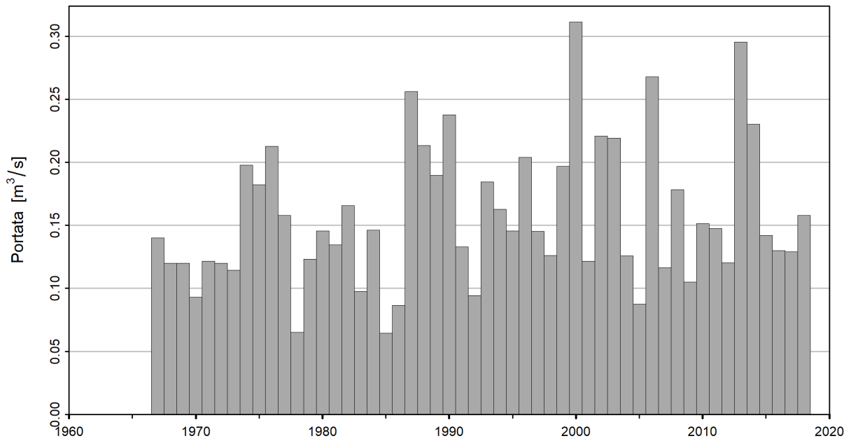
Figura 6: Serie temporale di NM7Q [ \text{m}^3/\text{s} ] (01.06.1967 - 31.05.2019)
