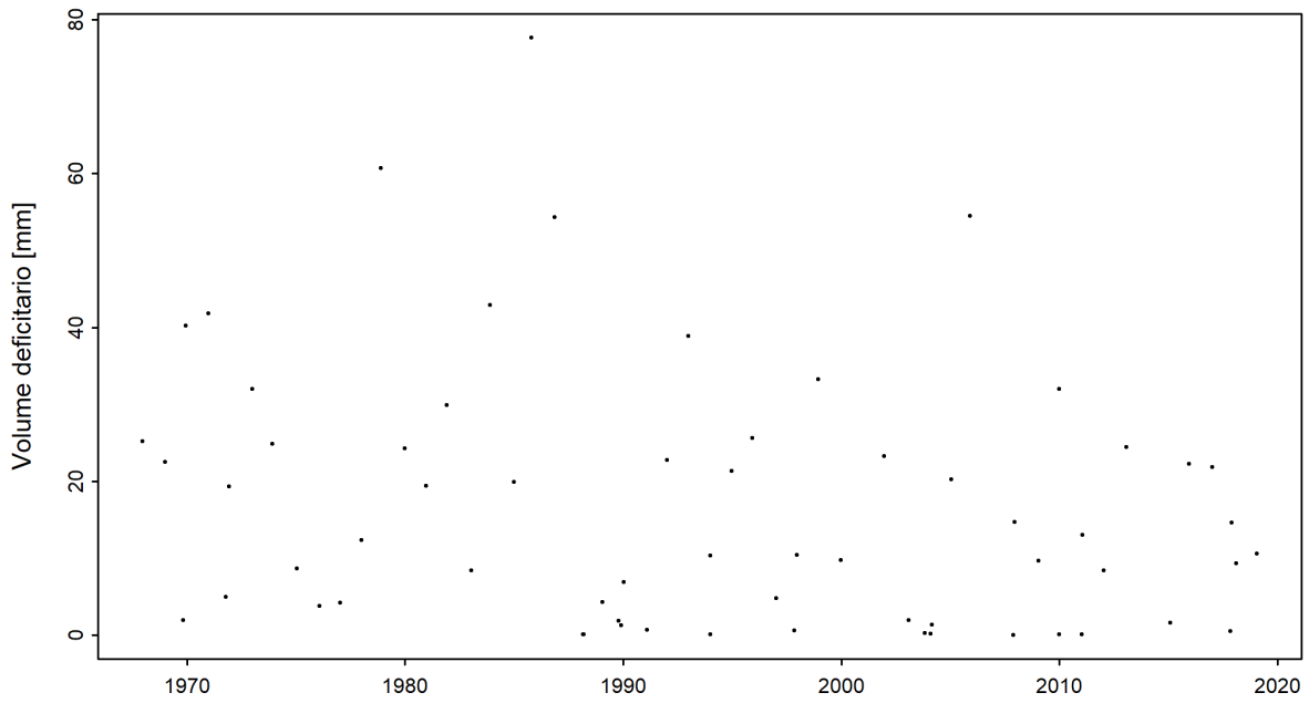
Figura 5: Serie temporale del volume deficitario [mm] (01.06.1967 - 31.05.2019)
