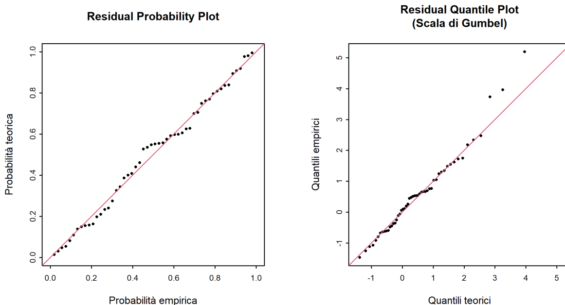
Figura 7: Plot diagnostici della variante di modello "mul" dell'approccio BLOCK (01.06.1967 - 31.05.2019)
