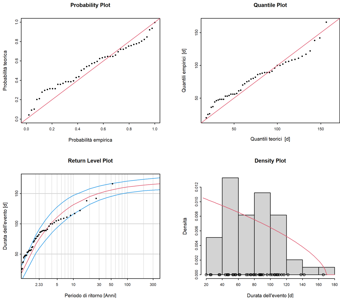
Figura 12: Plot diagnostici della variante di modello "stat" dell'approccio POT (01.06.1967 - 31.05.2019)
