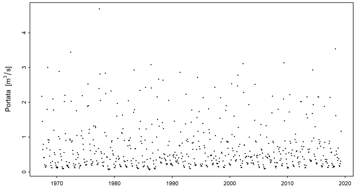
Figura 3: Serie temporale del minimo mensile di M7Q [m³/s] (01.06.1967 - 31.05.2019)
