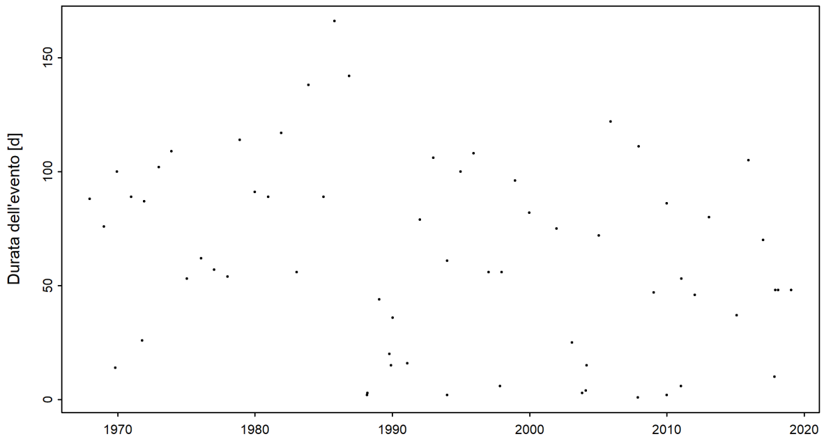
Figura 4: Serie temporale della durata di magra [d] (01.06.1967 - 31.05.2019)
