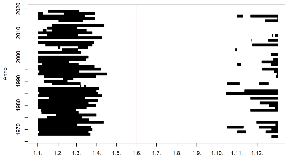
Figura 1: Apparizione temporale dei periodi di magra durante l'anno (01.06.1967 - 31.05.2019) e mese iniziale dell'anno di magra (linea rossa) 1
