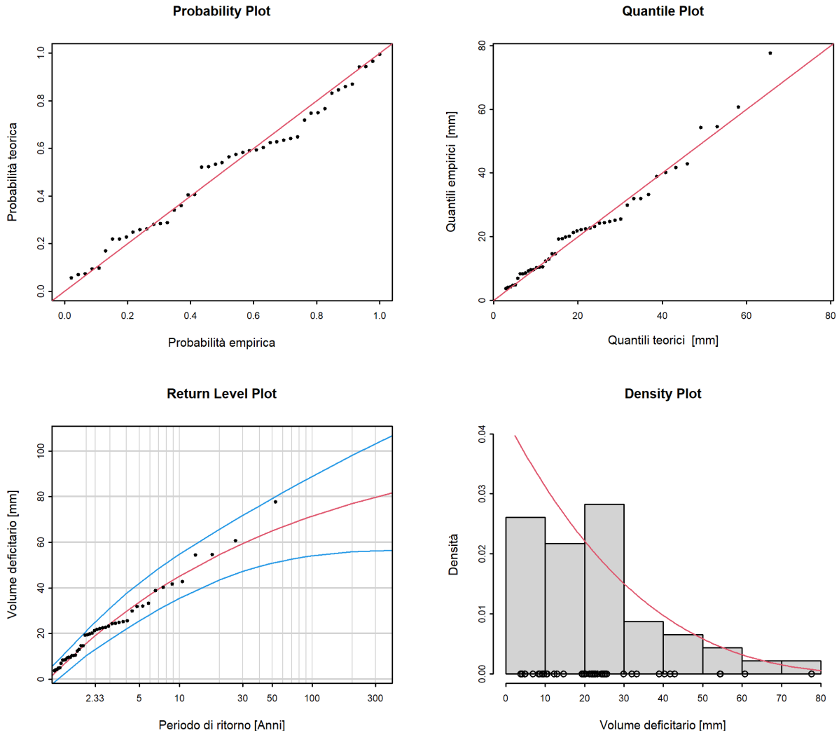
Figura 14: Plot diagnostici della variante di modello "stat" dell'approccio POT (01.06.1967 - 31.05.2019)
