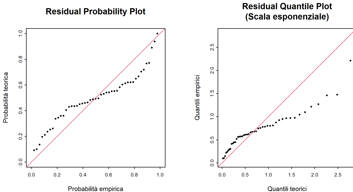
Figura 9: Plot diagnostici della variante di modello "sigl" dell'approccio POT (01.06.1967 - 31.05.2019)
