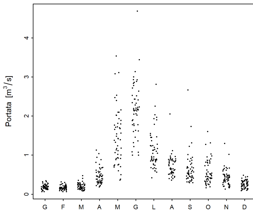
Figura 2: Sviluppo stagionale del minimo mensile di M7Q [ \text{m}^3/\text{s} ] (01.06.1967 - 31.05.2019)
