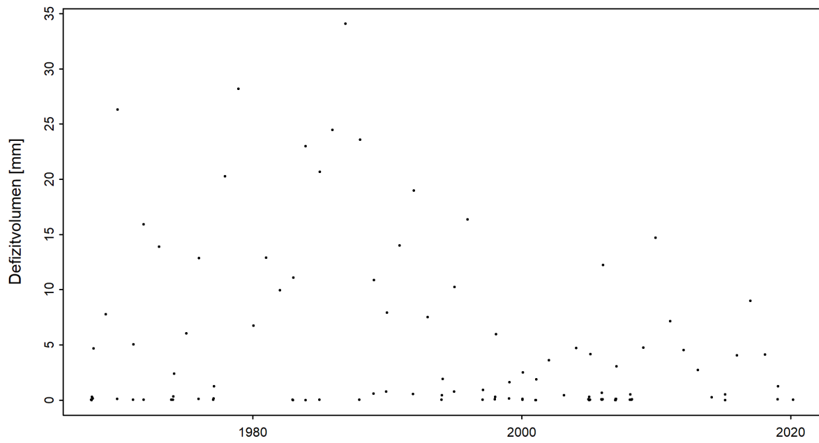
Abbildung 5: Zeitreihe der Defizitvolumen [mm] (01.06.1967 - 31.05.2020)
