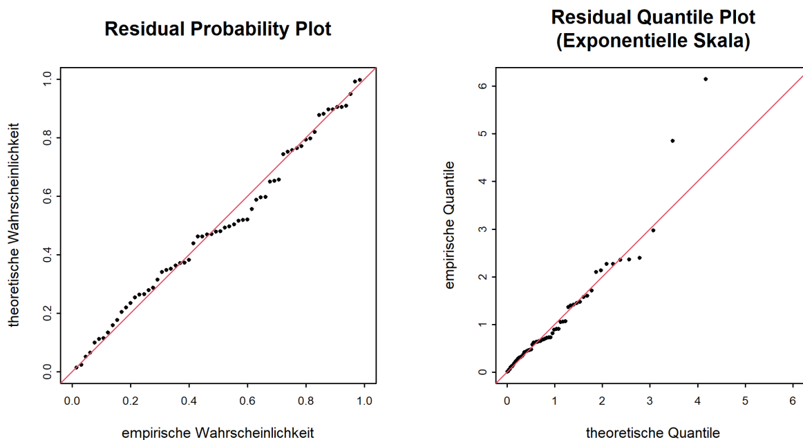
Abbildung 9: Diagnostikplots der Modellvariante “sigl” des POT-Ansatzes (01.06.1967 - 31.05.2020)
