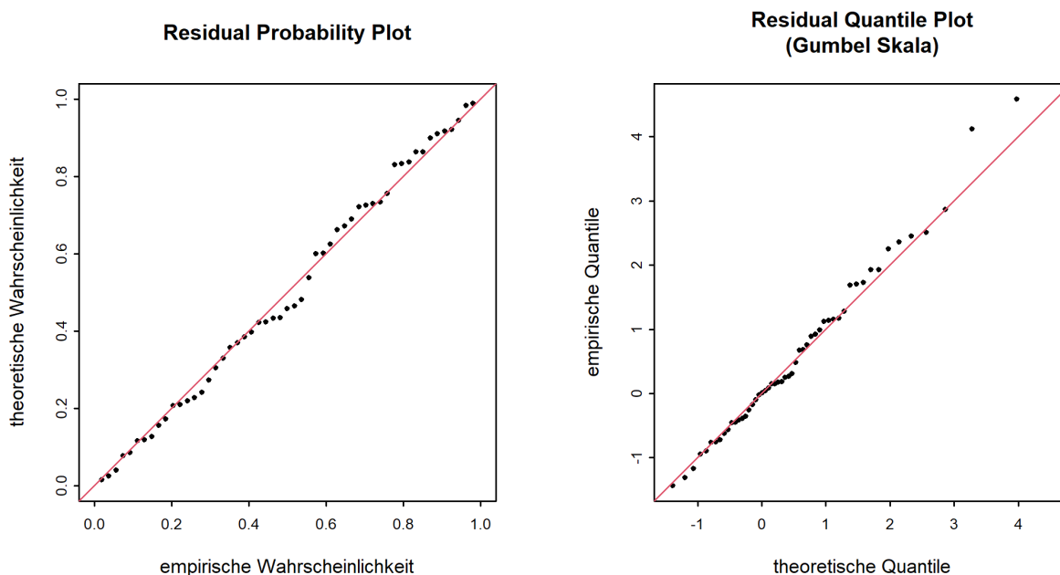
Abbildung 7: Diagnostikplots der Modellvariante “mujump1996” des BLOCK-Ansatzes (01.06.1967 - 31.05.2020)
