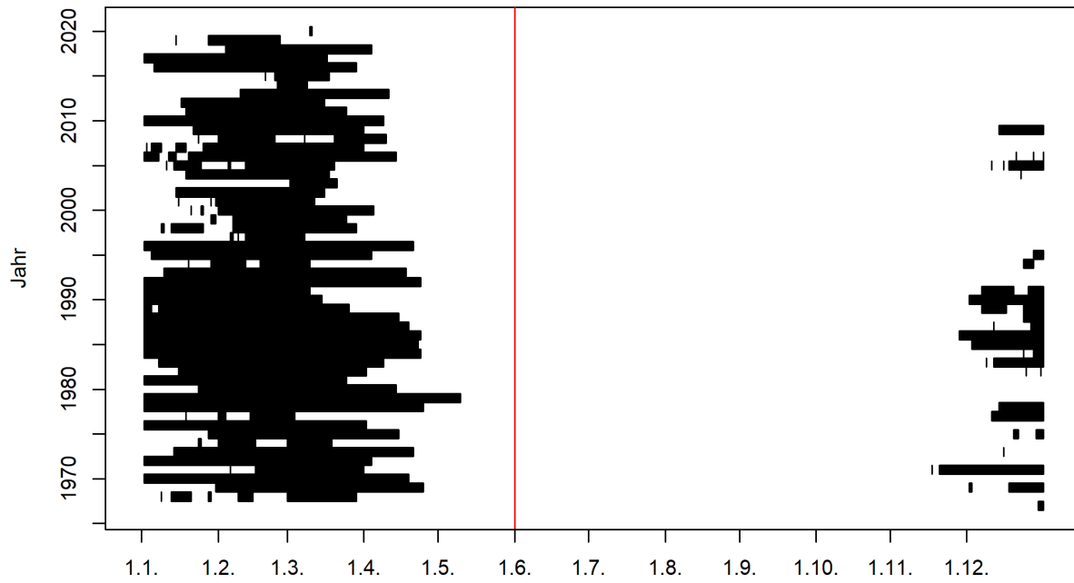
Abbildung 1: Zeitliches Auftreten der Niedrigwasserperioden im Jahresverlauf (01.06.1967 - 31.05.2020) und Startmonat des Niedrigwasserjahres (rote Linie) 1
