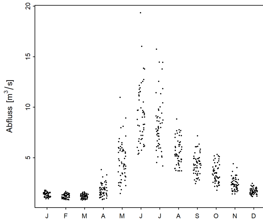
Abbildung 2: Saisonaler Verlauf der monatlichen Minima der M7Q [ \text{m}^3/\text{s} ] (01.06.1967 - 31.05.2020)
