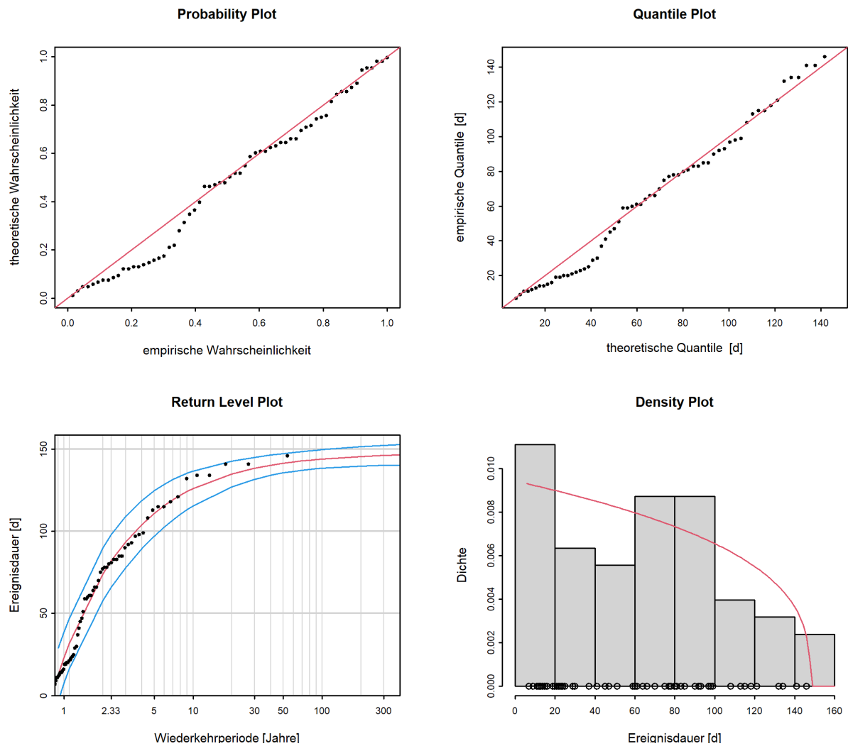
Abbildung 12: Diagnostikplots der Modellvariante “stat” des POT-Ansatzes (01.06.1967 - 31.05.2020)
