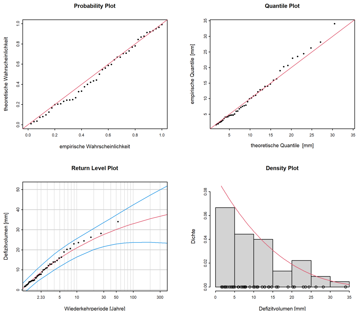
Abbildung 14: Diagnostikplots der Modellvariante “stat” des POT-Ansatzes (01.06.1967 - 31.05.2020)
