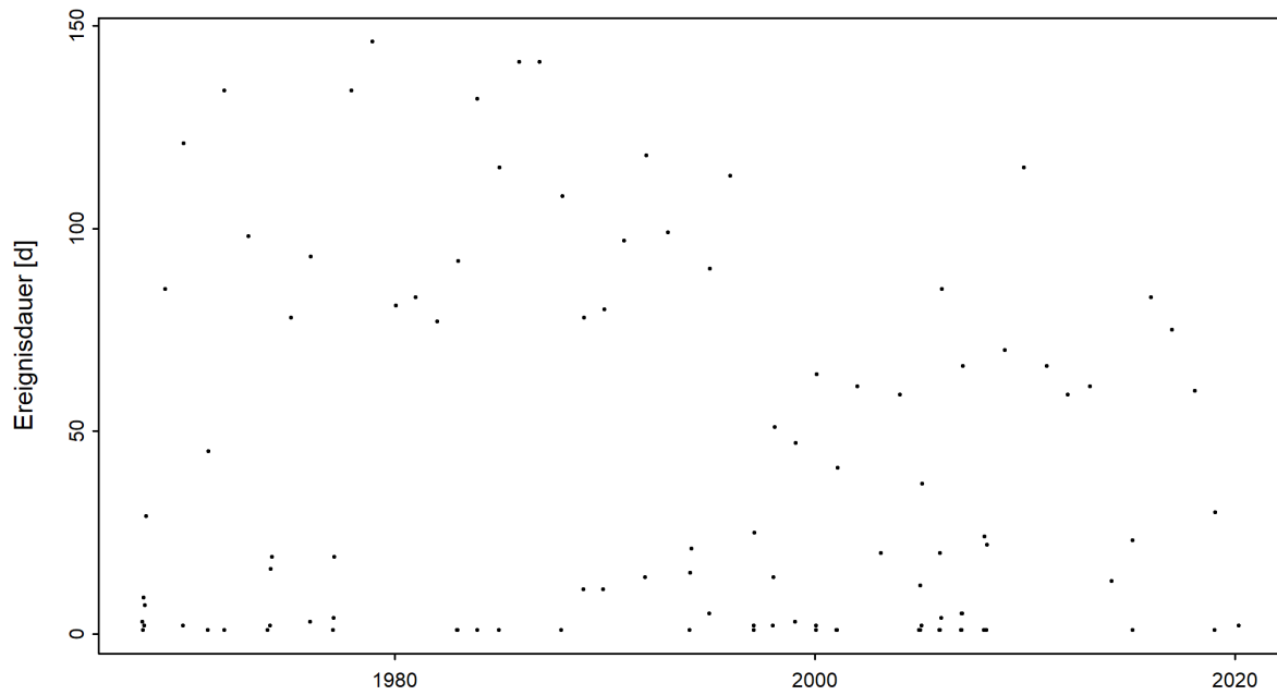
Abbildung 4: Zeitreihe der Niedrigwasserdauern [d] (01.06.1967 - 31.05.2020)
