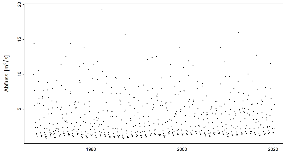
Abbildung 3: Zeitreihe der monatlichen Minima der M7Q [ \text{m}^3/\text{s} ] (01.06.1967 - 31.05.2020)
