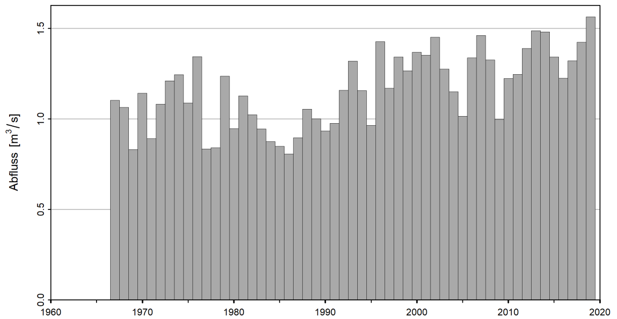
Abbildung 6: Zeitreihe der NM7Q [m³/s] (01.06.1967 - 31.05.2020)
