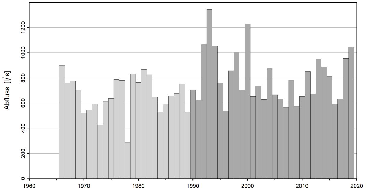
Abbildung 6: Zeitreihe der NM7Q [l/s] (01.06.1966 - 31.05.2020), hellgrau: nicht verwendete NM7Q, dunkelgrau: verwendete NM7Q
