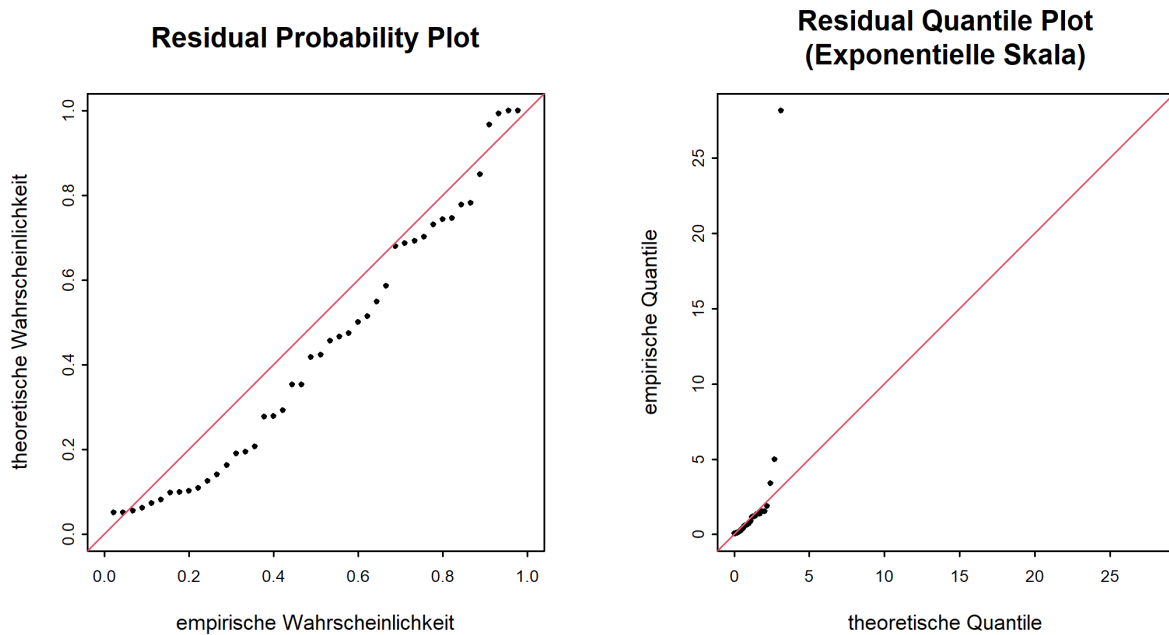
Abbildung 9: Diagnostikplots der Modellvariante “sigl” des POT-Ansatzes (01.06.1990 - 31.05.2020)
