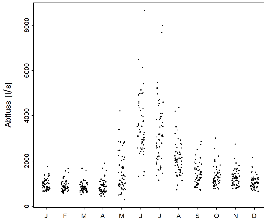
Abbildung 2: Saisonaler Verlauf der monatlichen Minima der M7Q [l/s] (01.06.1966 - 31.05.2020)
