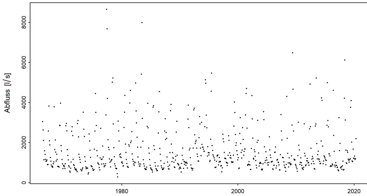
Abbildung 3: Zeitreihe der monatlichen Minima der M7Q [l/s] (01.06.1966 - 31.05.2020)
