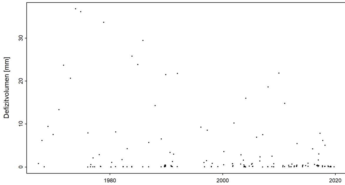
Abbildung 5: Zeitreihe der Defizitvolumen [mm] (01.06.1966 - 31.05.2020)
