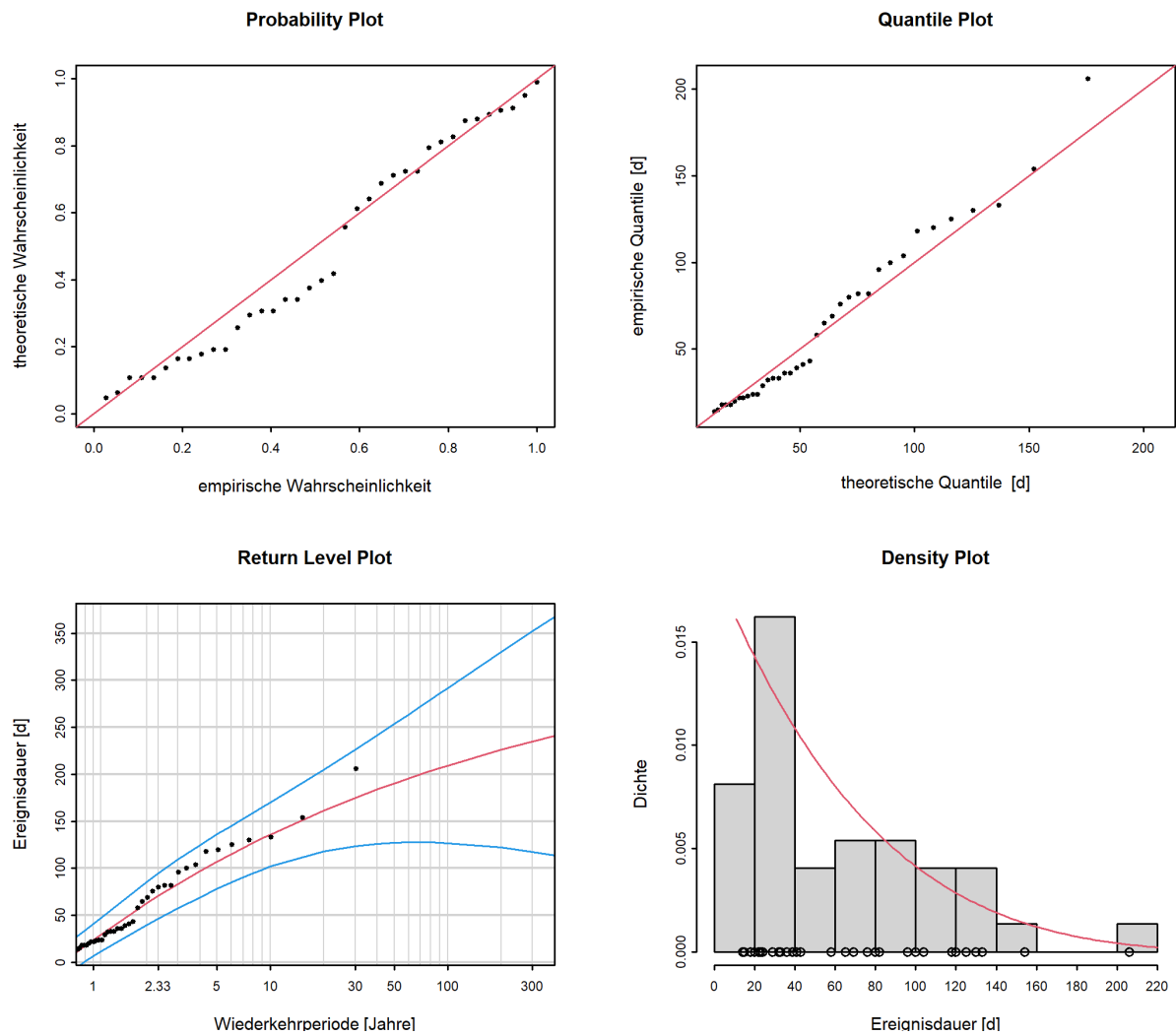
Abbildung 12: Diagnostikplots der Modellvariante “stat” des POT-Ansatzes (01.06.1990 - 31.05.2020)
