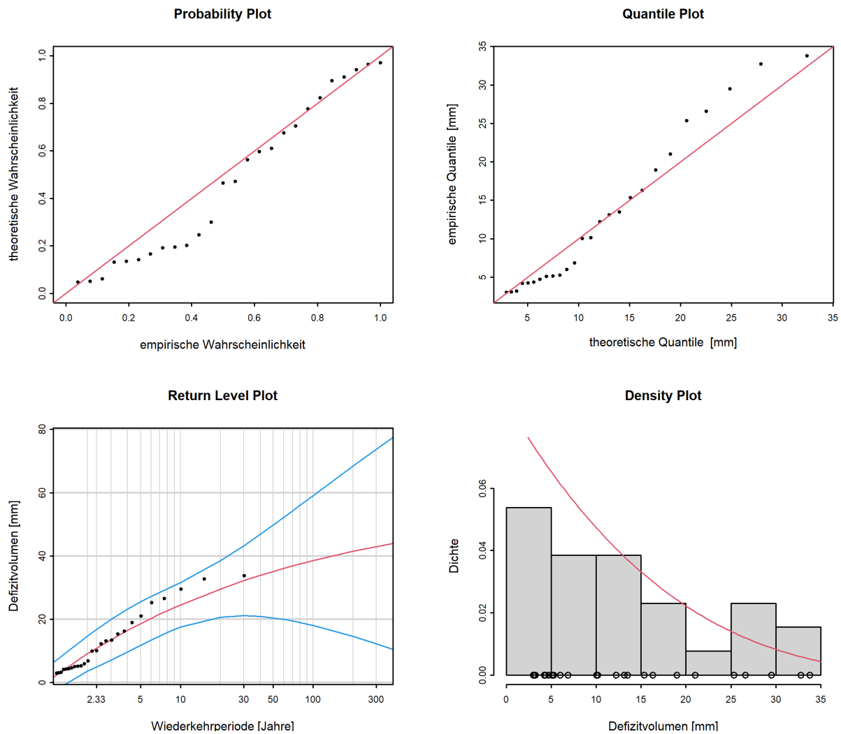
Abbildung 14: Diagnostikplots der Modellvariante "stat" des POT-Ansatzes (01.06.1990 - 31.05.2020)
