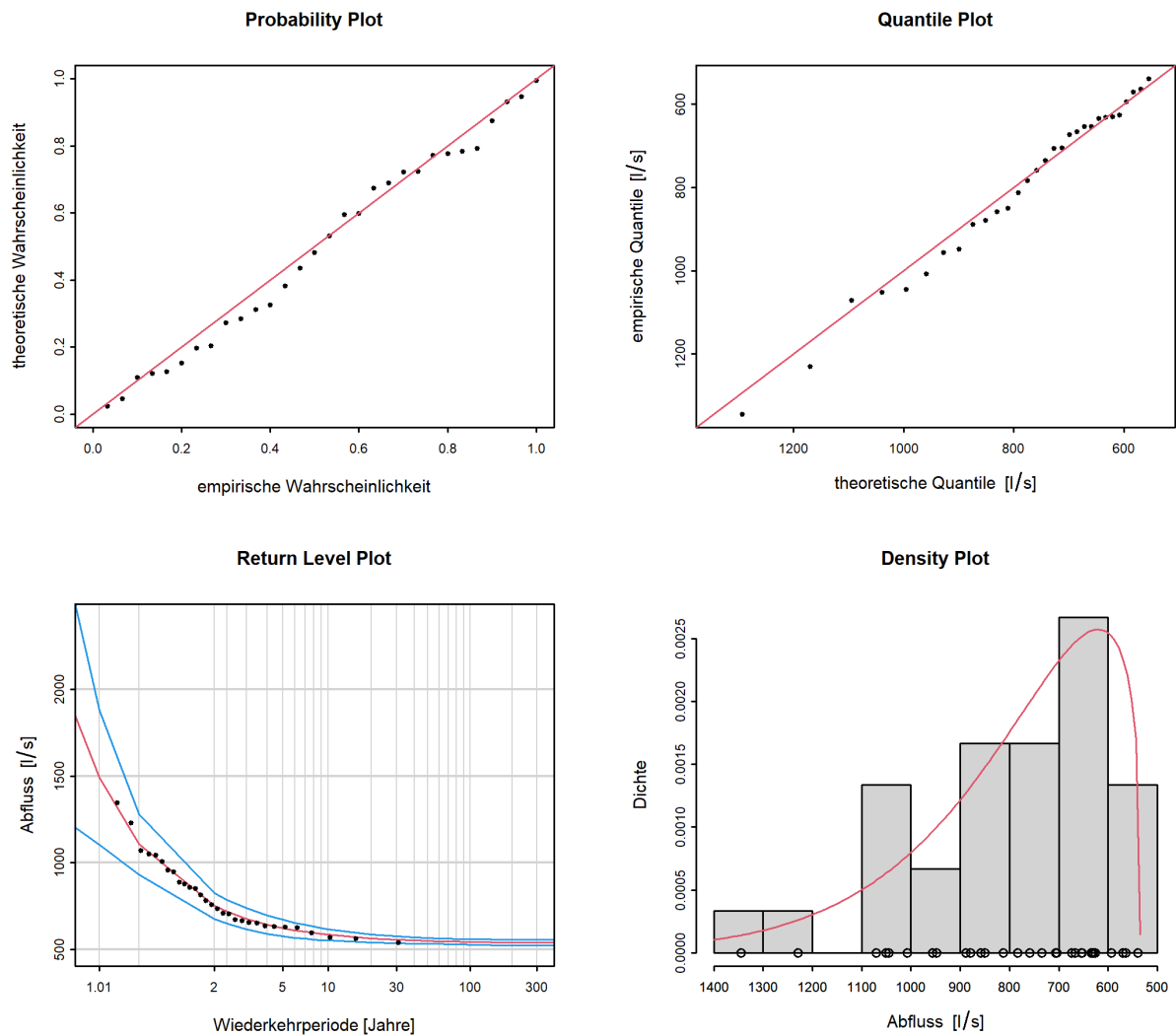
Abbildung 7: Diagnostikplots der Modellvariante “stat” des BLOCK-Ansatzes (01.06.1990 - 31.05.2020)
