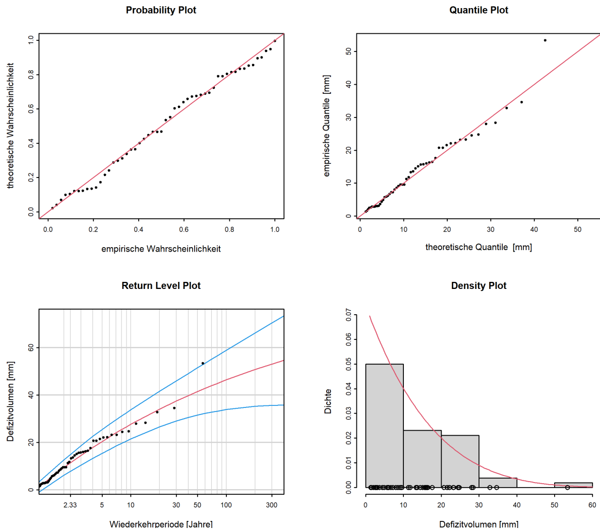
Abbildung 14: Diagnostikplots der Modellvariante “stat” des POT-Ansatzes (01.06.1964 - 31.05.2020)
