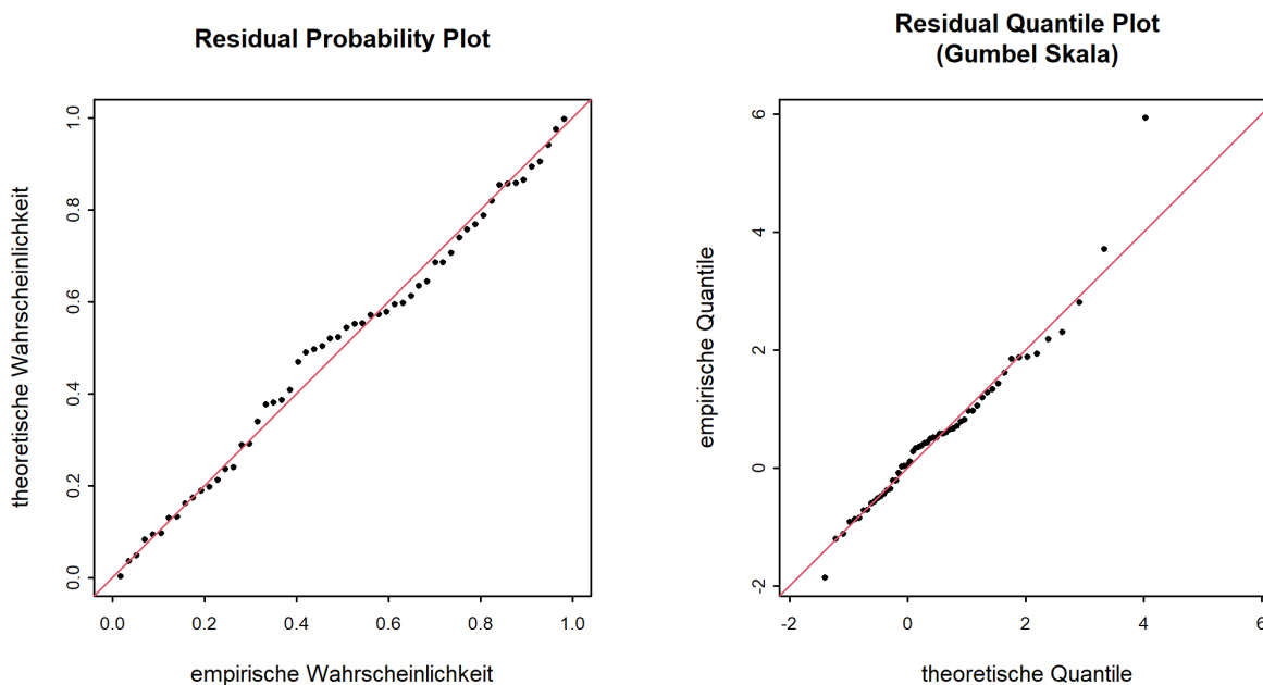
Abbildung 7: Diagnostikplots der Modellvariante “muq” des BLOCK-Ansatzes (01.06.1964 - 31.05.2020)
