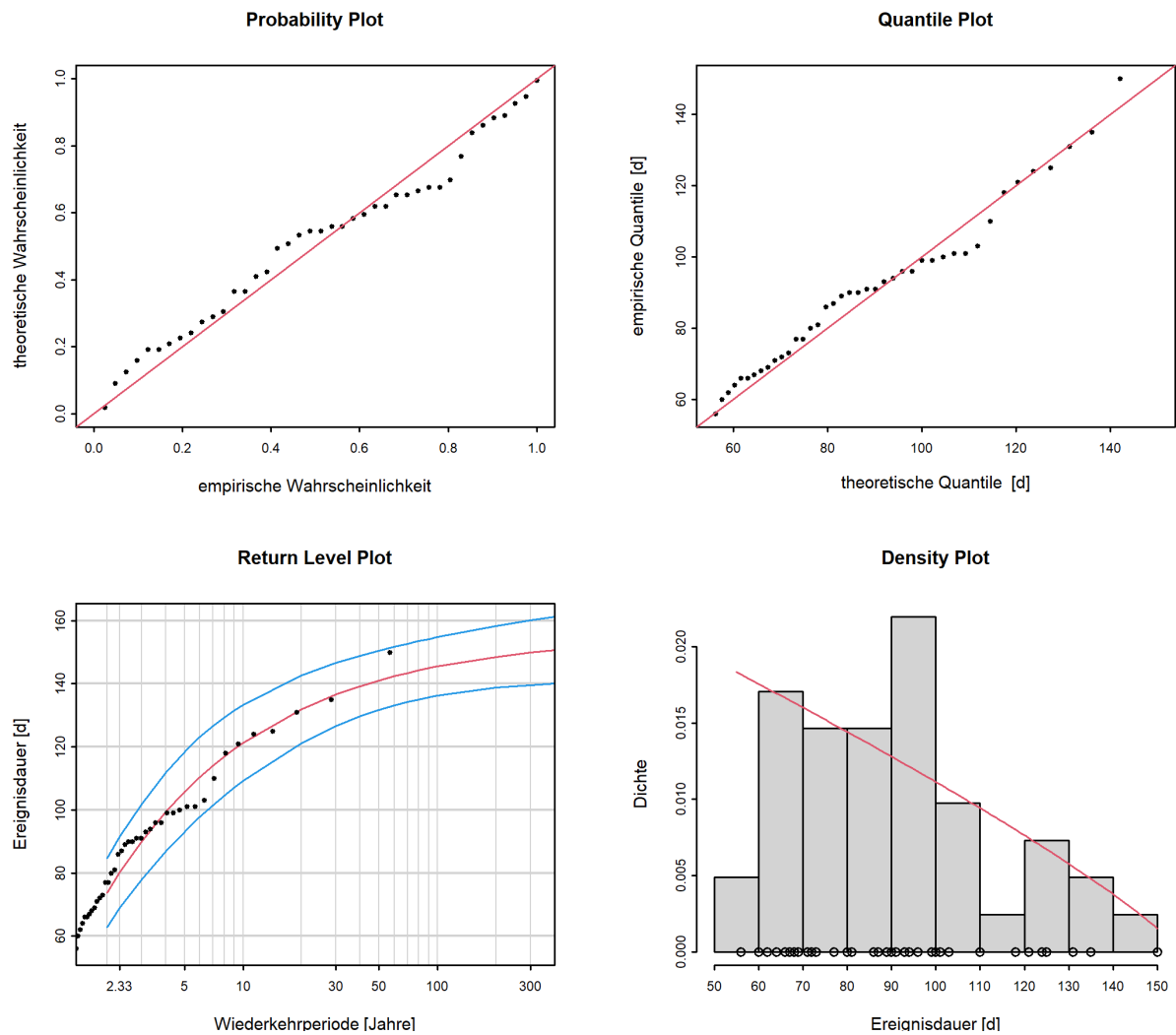
Abbildung 12: Diagnostikplots der Modellvariante “stat” des POT-Ansatzes (01.06.1964 - 31.05.2020)
