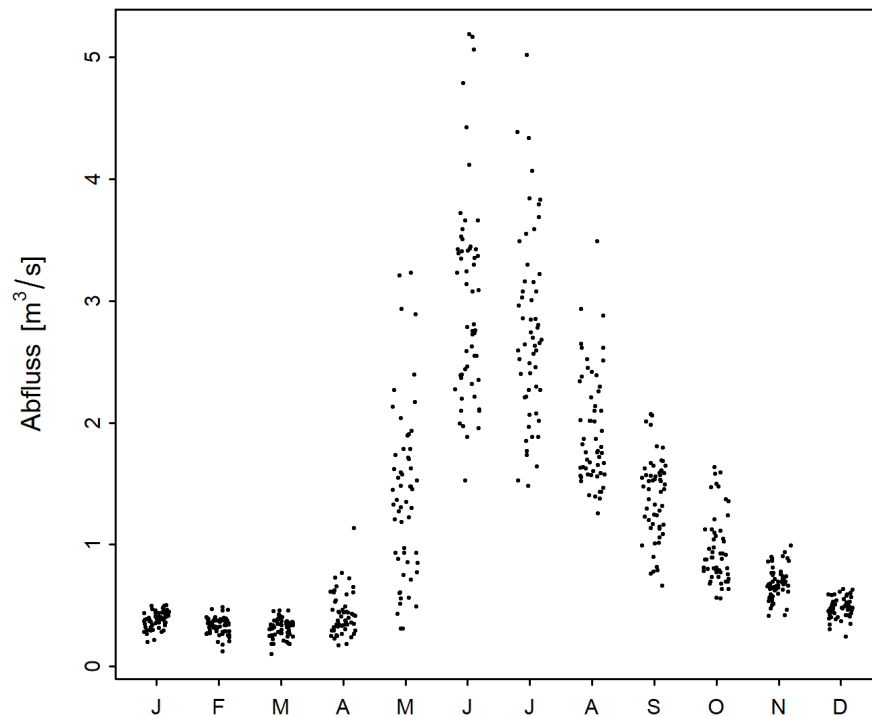
Abbildung 2: Saisonaler Verlauf der monatlichen Minima der M7Q [m³/s] (01.06.1963 - 31.05.2020)
