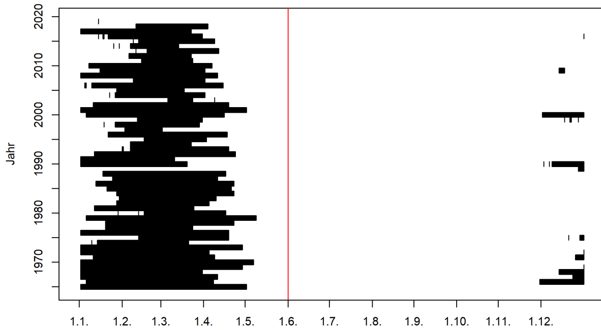
Abbildung 1: Zeitliches Auftreten der Niedrigwasserperioden im Jahresverlauf (01.06.1963 - 31.05.2020) und Startmonat des Niedrigwasserjahres (rote Linie) 1
