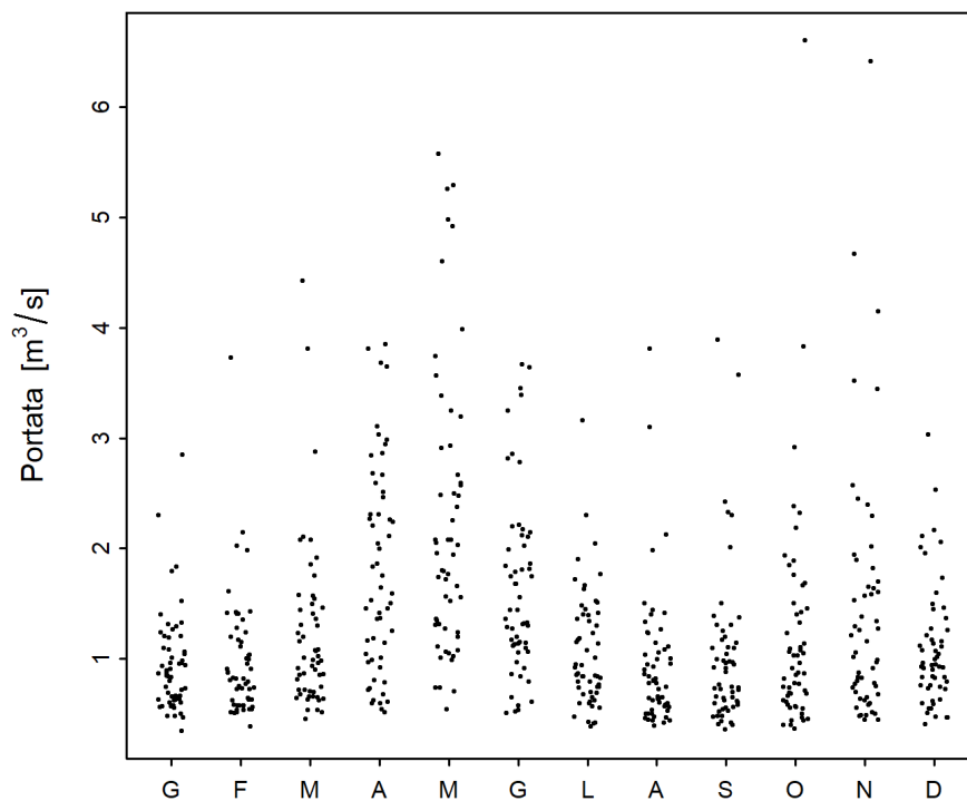
Figura 2: Sviluppo stagionale del minimo mensile di M7Q [ \text{m}^3/\text{s} ] (01.06.1963 - 31.05.2019)
