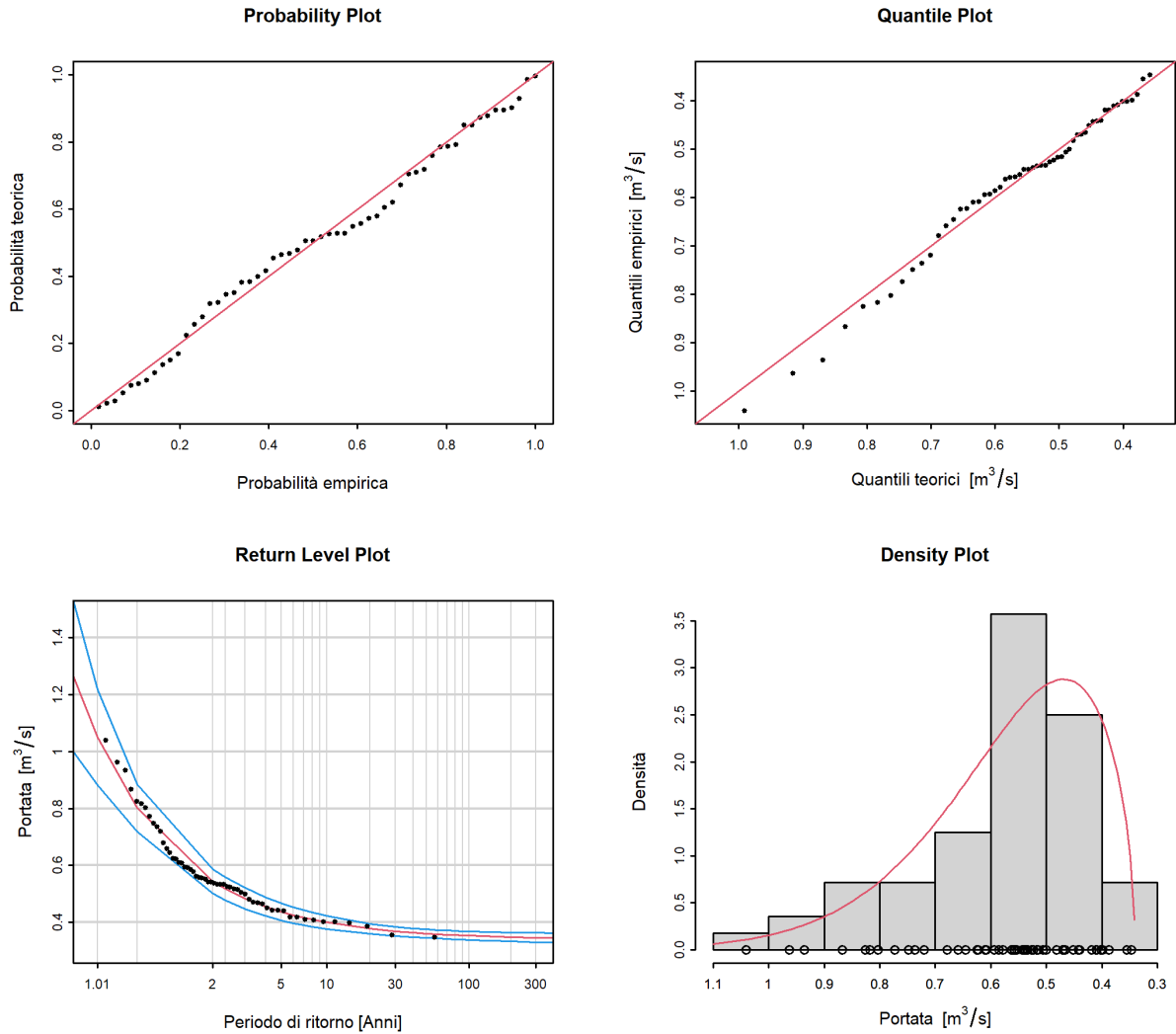
Figura 7: Plot diagnostici della variante di modello "stat" dell'approccio BLOCK (01.06.1963 - 31.05.2019)
