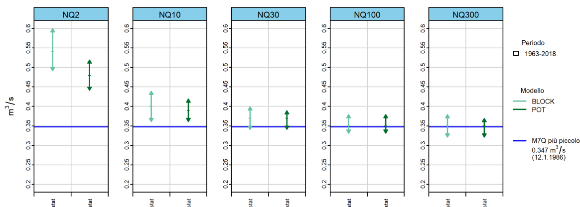
Figura 10: NQ_T [ m^3/s ] incl. intervallo di confidenza 95%, calcolato con la variante di modello più adatta degli approcci BLOCK e POT
