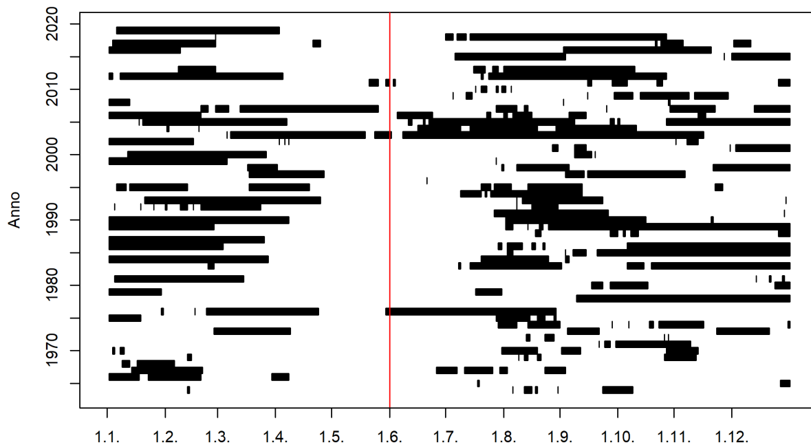
Figura 1: Apparizione temporale dei periodi di magra durante l'anno (01.06.1963 - 31.05.2019) e mese iniziale dell'anno di magra (linea rossa) 1
