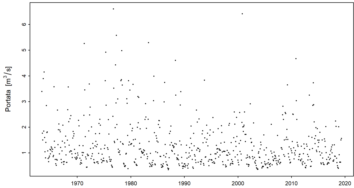
Figura 3: Serie temporale del minimo mensile di M7Q [m³/s] (01.06.1963 - 31.05.2019)
