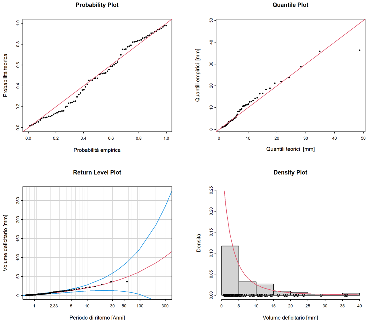
Figura 14: Plot diagnostici della variante di modello "stat" dell'approccio POT (01.06.1963 - 31.05.2019)
