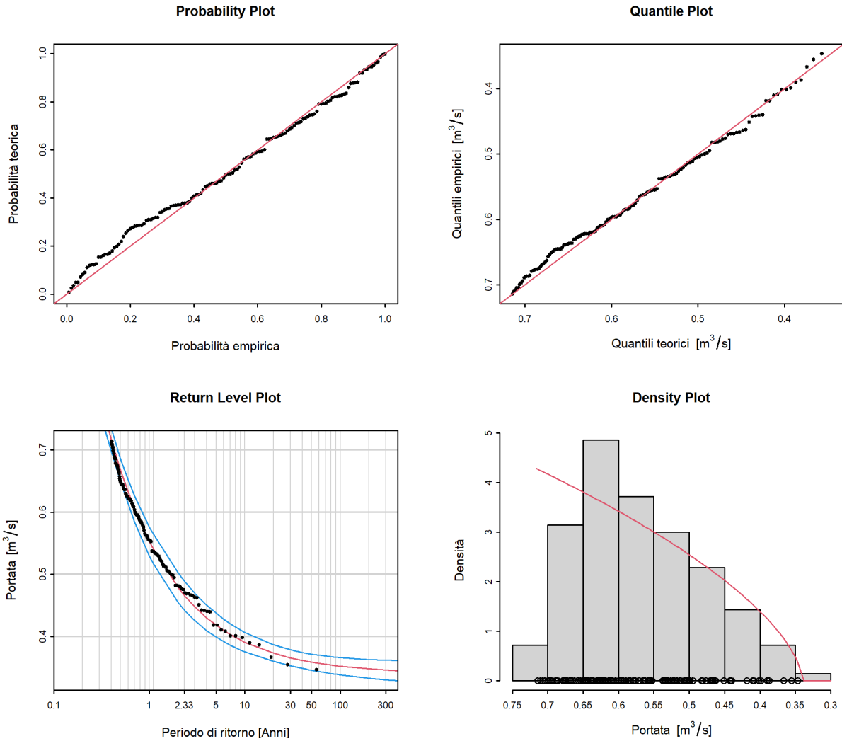
Figura 9: Plot diagnostici della variante di modello "stat" dell'approccio POT (01.06.1963 - 31.05.2019)
