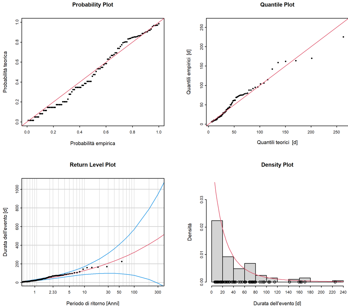
Figura 12: Plot diagnostici della variante di modello "stat" dell'approccio POT (01.06.1963 - 31.05.2019)
