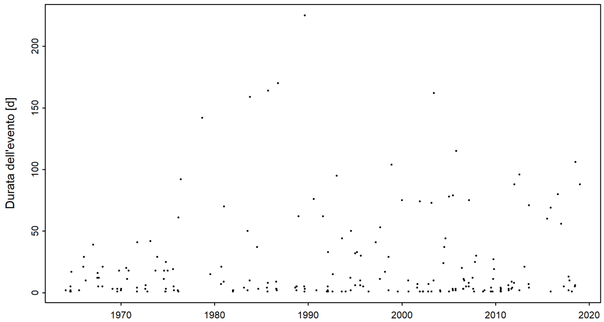
Figura 4: Serie temporale della durata di magra [d] (01.06.1963 - 31.05.2019)
