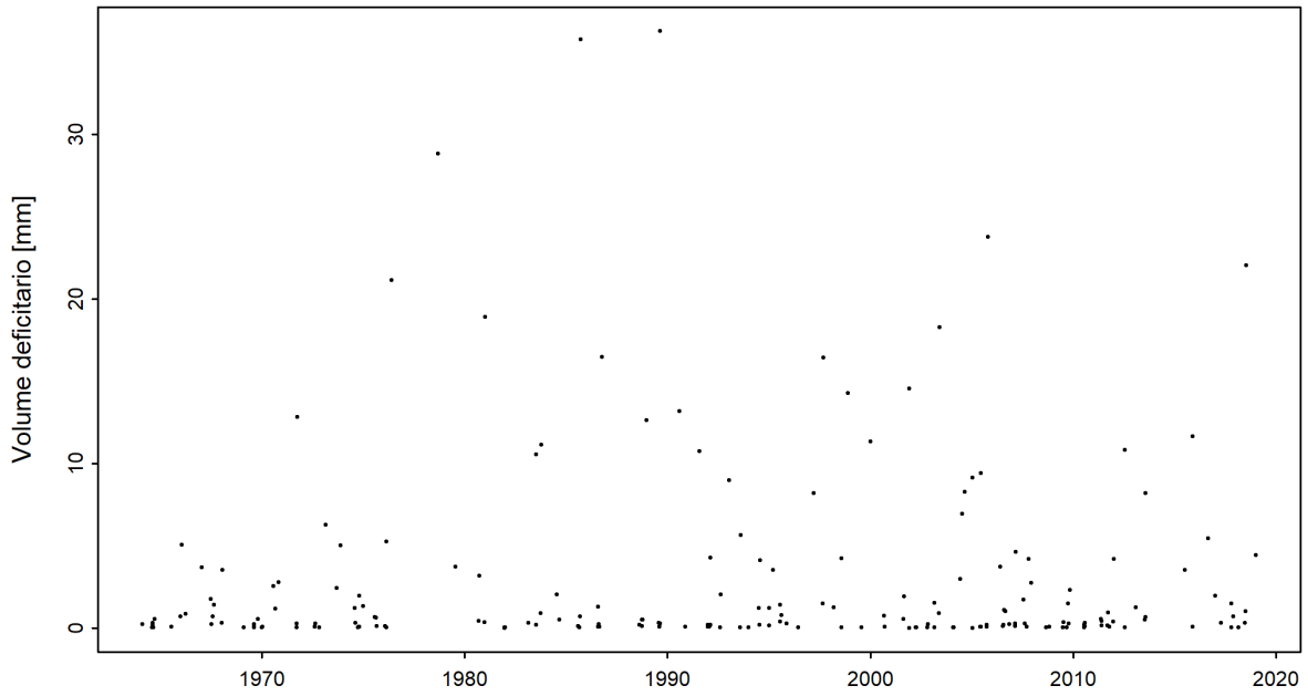
Figura 5: Serie temporale del volume deficitario [mm] (01.06.1963 - 31.05.2019)
