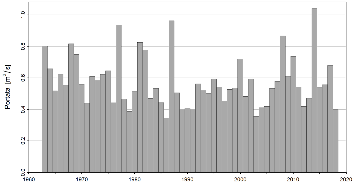
Figura 6: Serie temporale di NM7Q [ \text{m}^3/\text{s} ] (01.06.1963 - 31.05.2019)
