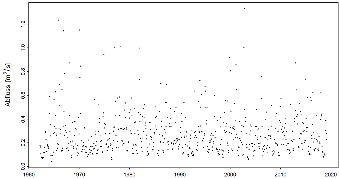
Abbildung 3: Zeitreihe der monatlichen Minima der M7Q [ \text{m}^3/\text{s} ] (01.04.1961 - 31.03.2019)
