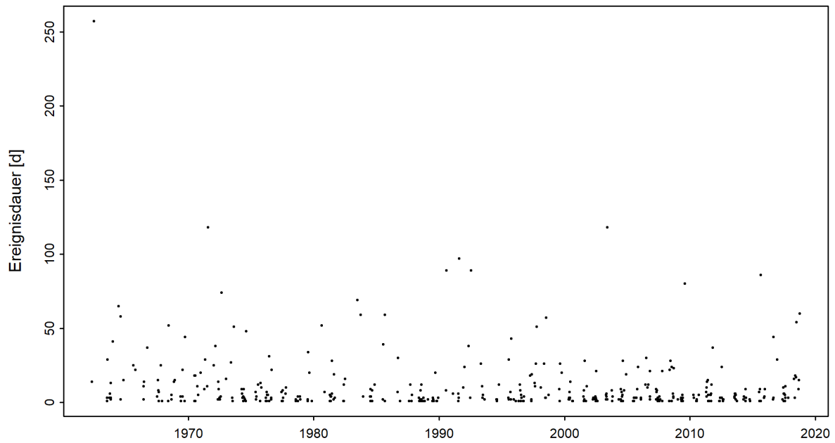
Abbildung 4: Zeitreihe der Niedrigwasserdauern [d] (01.04.1961 - 31.03.2019)
