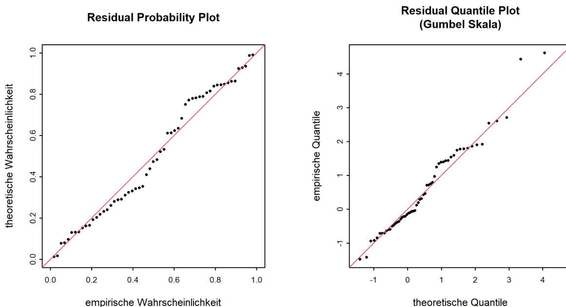
Abbildung 7: Diagnostikplots der Modellvariante “mujump1977” des BLOCK-Ansatzes (01.04.1962 - 31.03.2019)
