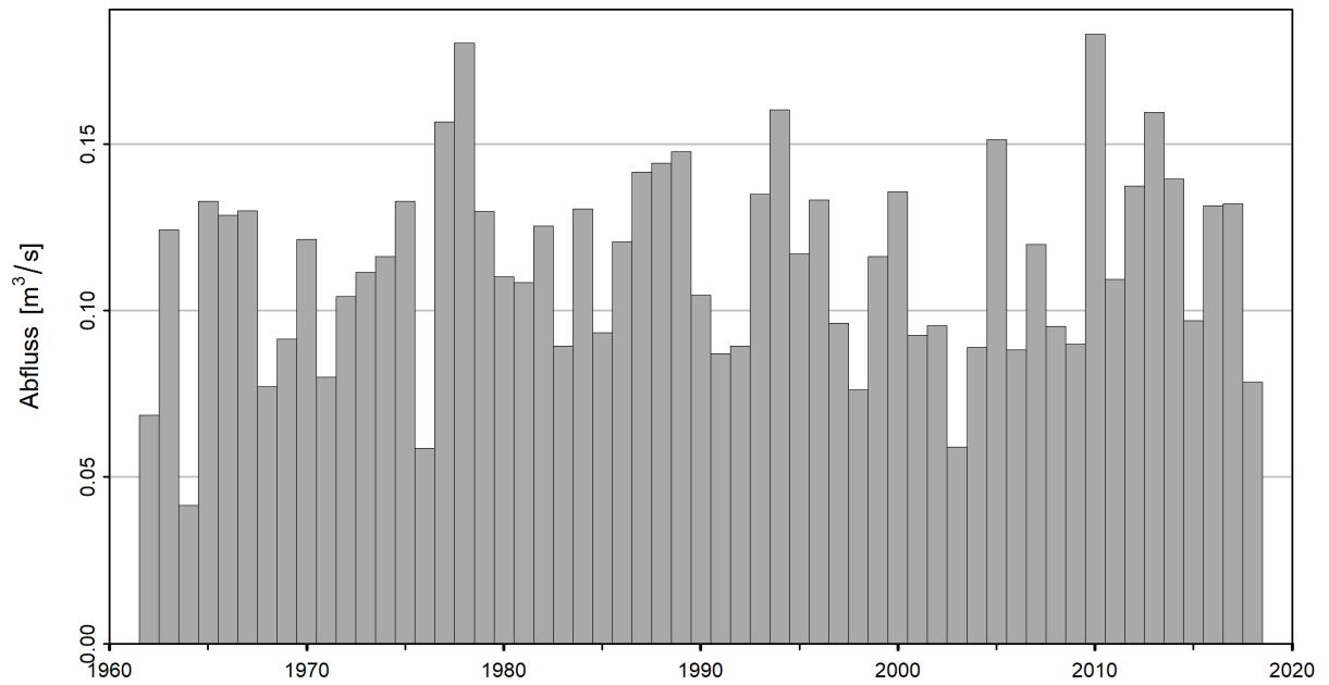
Abbildung 6: Zeitreihe der NM7Q [m³/s] (01.04.1961 - 31.03.2019)
