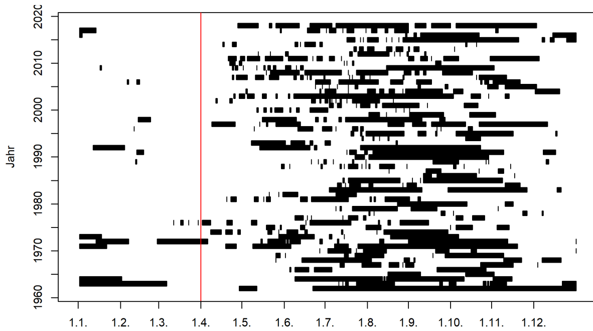
Abbildung 1: Zeitliches Auftreten der Niedrigwasserperioden im Jahresverlauf (01.04.1961 - 31.03.2019) und Startmonat des Niedrigwasserjahres (rote Linie) 1
