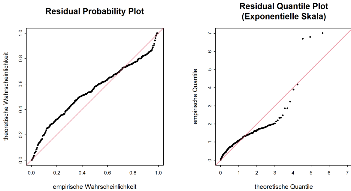
Abbildung 9: Diagnostikplots der Modellvariante “sigl” des POT-Ansatzes (01.04.1962 - 31.03.2019)
