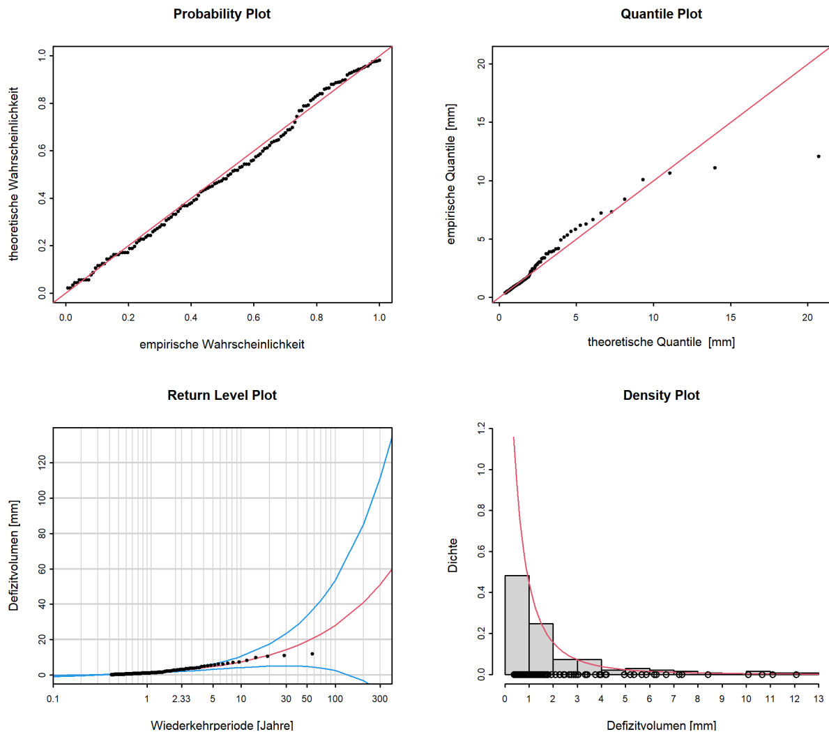
Abbildung 14: Diagnostikplots der Modellvariante “stat” des POT-Ansatzes (01.04.1962 - 31.03.2019)
