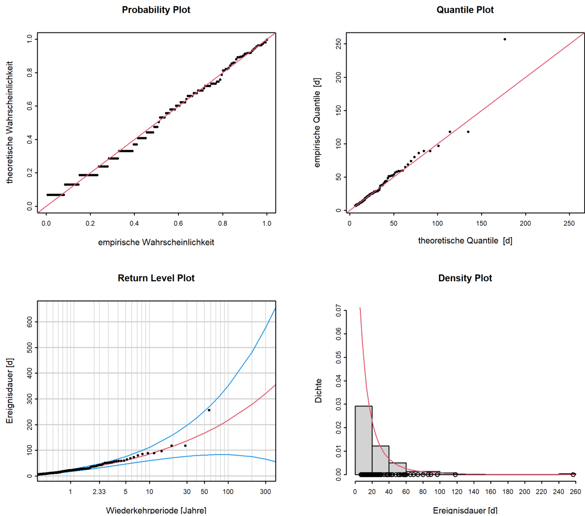
Abbildung 12: Diagnostikplots der Modellvariante “stat” des POT-Ansatzes (01.04.1962 - 31.03.2019)
