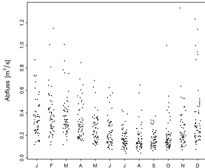
Abbildung 2: Saisonaler Verlauf der monatlichen Minima der M7Q [ \text{m}^3/\text{s} ] (01.04.1961 - 31.03.2019)
