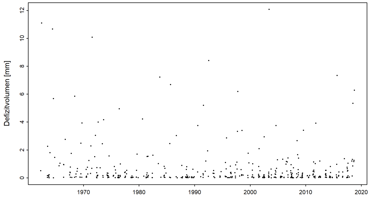
Abbildung 5: Zeitreihe der Defizitvolumen [mm] (01.04.1961 - 31.03.2019)
