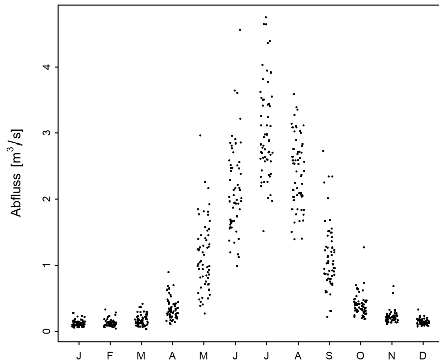
Abbildung 2: Saisonaler Verlauf der monatlichen Minima der M7Q [m³/s] (01.06.1960 - 31.05.2020)
