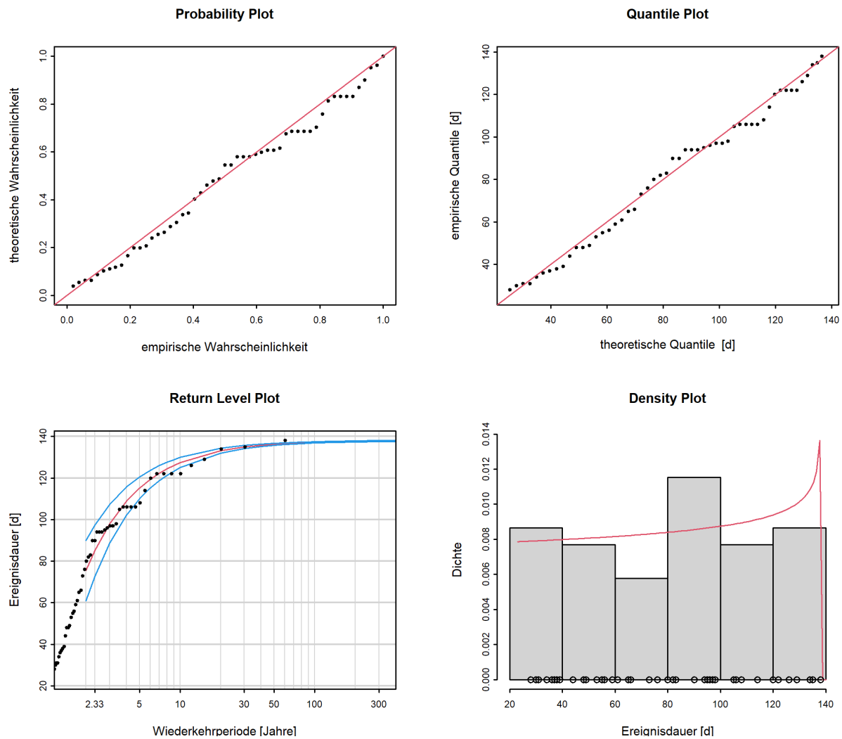
Abbildung 12: Diagnostikplots der Modellvariante “stat” des POT-Ansatzes (01.06.1960 - 31.05.2020)
