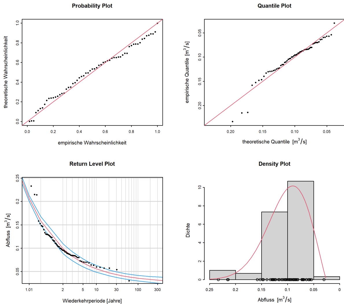
Abbildung 7: Diagnostikplots der Modellvariante “stat” des BLOCK-Ansatzes (01.06.1960 - 31.05.2020)
