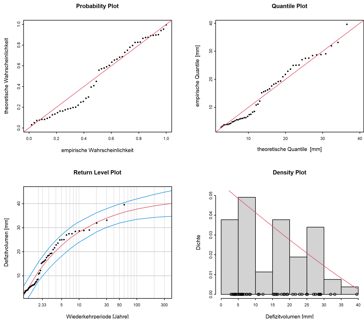
Abbildung 14: Diagnostikplots der Modellvariante “stat” des POT-Ansatzes (01.06.1960 - 31.05.2020)
