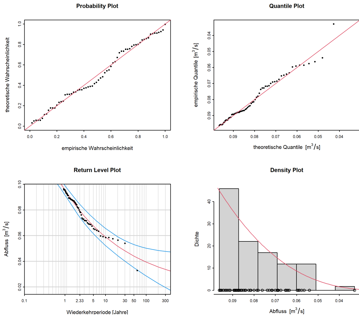
Abbildung 9: Diagnostikplots der Modellvariante "stat" des POT-Ansatzes (01.06.1960 - 31.05.2020)
