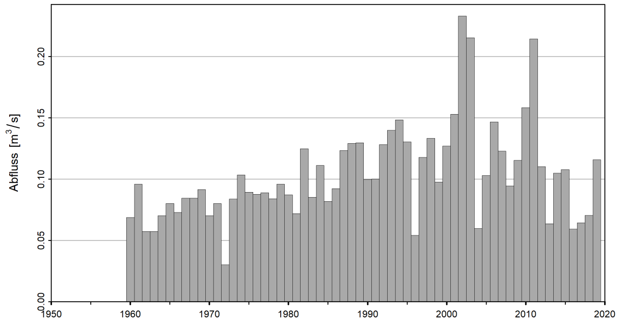
Abbildung 6: Zeitreihe der NM7Q [m³/s] (01.06.1960 - 31.05.2020)
