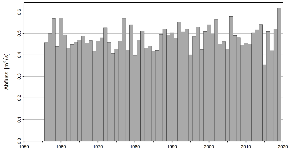
Abbildung 6: Zeitreihe der NM7Q [m³/s] (01.06.1956 - 31.05.2020)
