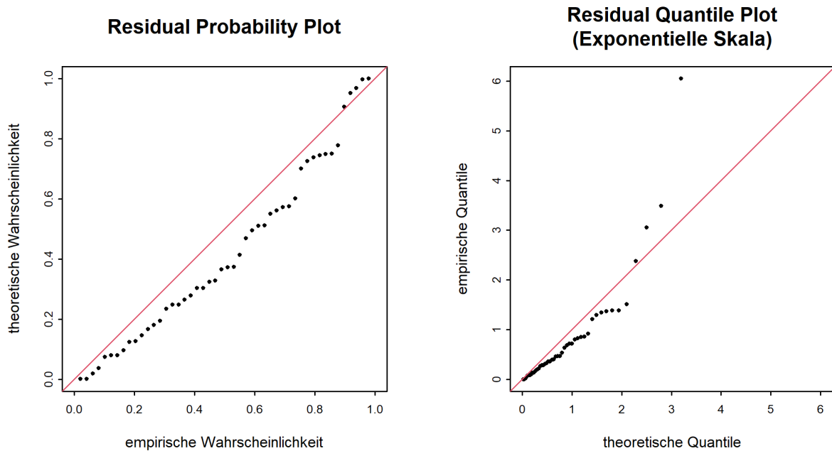
Abbildung 9: Diagnostikplots der Modellvariante “sigl” des POT-Ansatzes (01.06.1956 - 31.05.2020)
