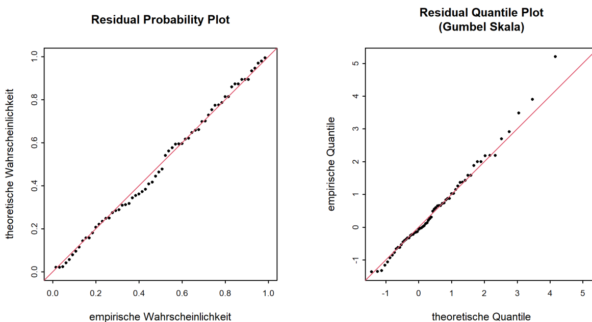
Abbildung 7: Diagnostikplots der Modellvariante “sigl” des BLOCK-Ansatzes (01.06.1956 - 31.05.2020)
