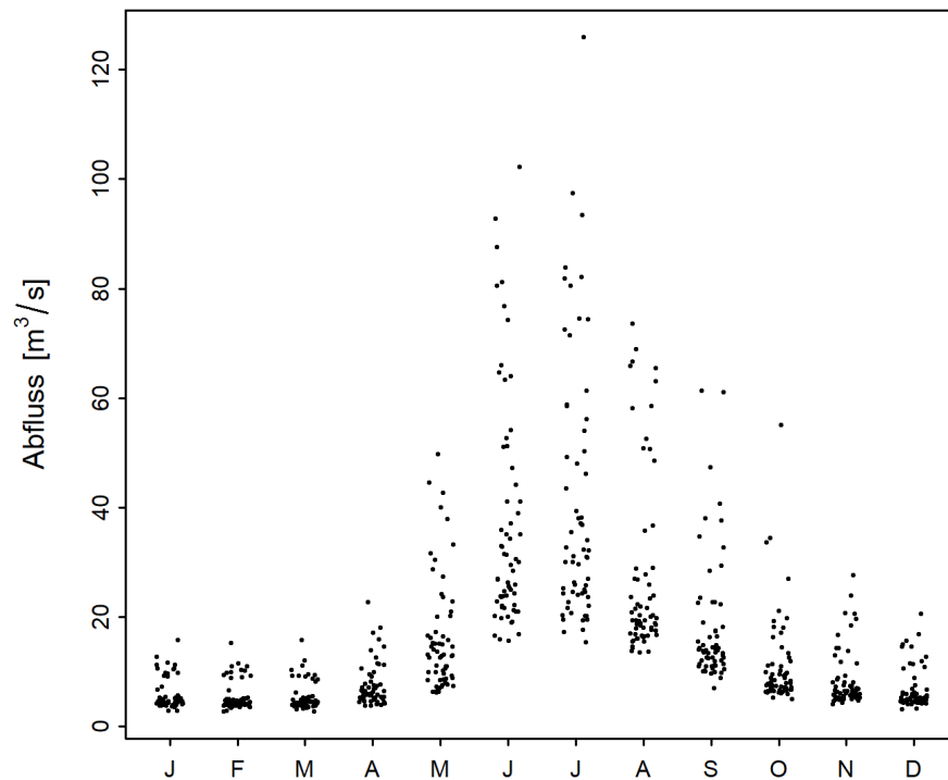
Abbildung 2: Saisonaler Verlauf der monatlichen Minima der M7Q [ \text{m}^3/\text{s} ] (01.06.1957 - 31.05.2020)
