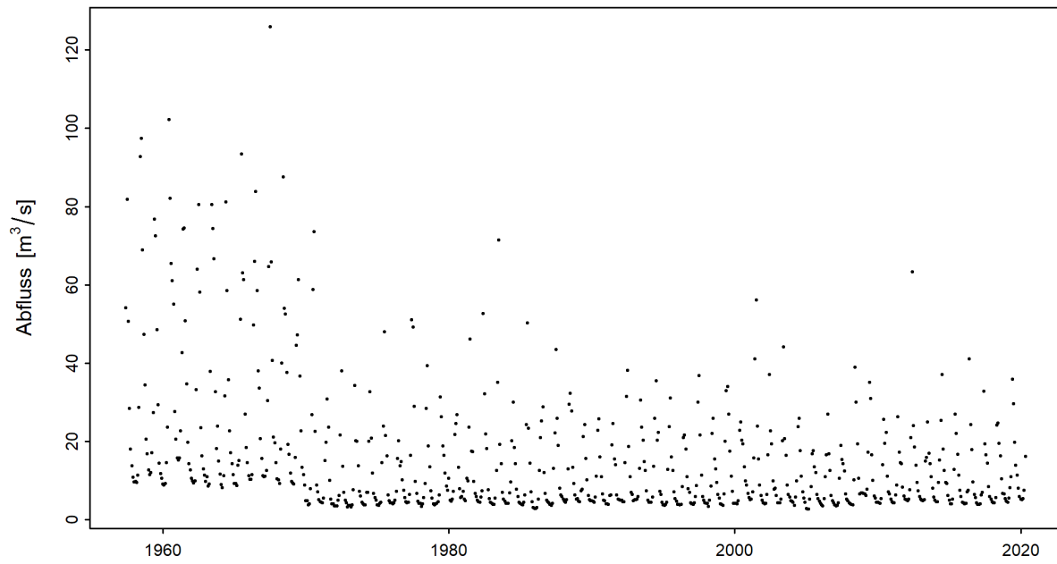
Abbildung 3: Zeitreihe der monatlichen Minima der M7Q [ \text{m}^3/\text{s} ] (01.06.1957 - 31.05.2020)
