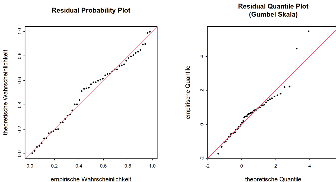
Abbildung 7: Diagnostikplots der Modellvariante “mujump2008” des BLOCK-Ansatzes (01.06.1969 - 31.05.2020)
