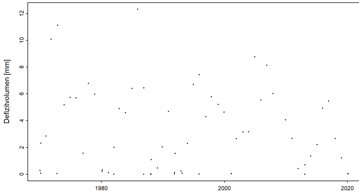
Abbildung 5: Zeitreihe der Defizitvolumen [mm] (01.06.1957 - 31.05.2020)
