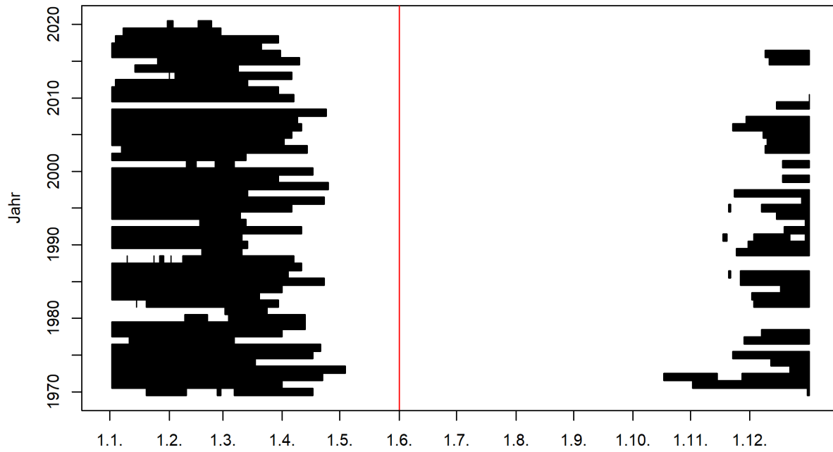
Abbildung 1: Zeitliches Auftreten der Niedrigwasserperioden im Jahresverlauf (01.06.1957 - 31.05.2020) und Startmonat des Niedrigwasserjahres (rote Linie) 1
