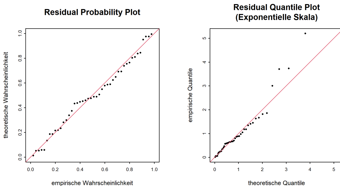
Abbildung 9: Diagnostikplots der Modellvariante “sigjump2008” des POT-Ansatzes (01.06.1969 - 31.05.2020)
