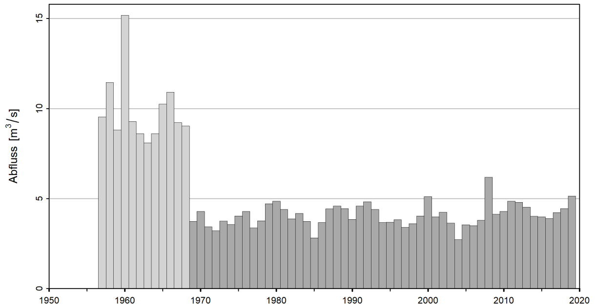
Abbildung 6: Zeitreihe der NM7Q [m³/s] (01.06.1957 - 31.05.2020), hellgrau: nicht verwendete NM7Q, dunkelgrau: verwendete NM7Q
