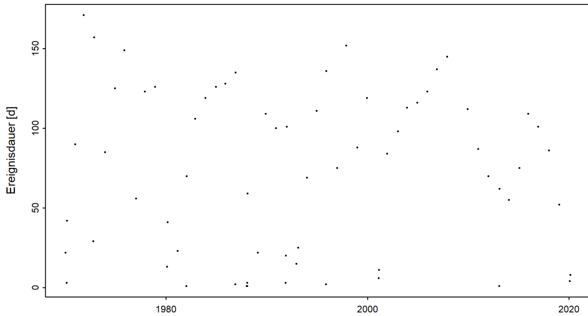
Abbildung 4: Zeitreihe der Niedrigwasserdauern [d] (01.06.1957 - 31.05.2020)
