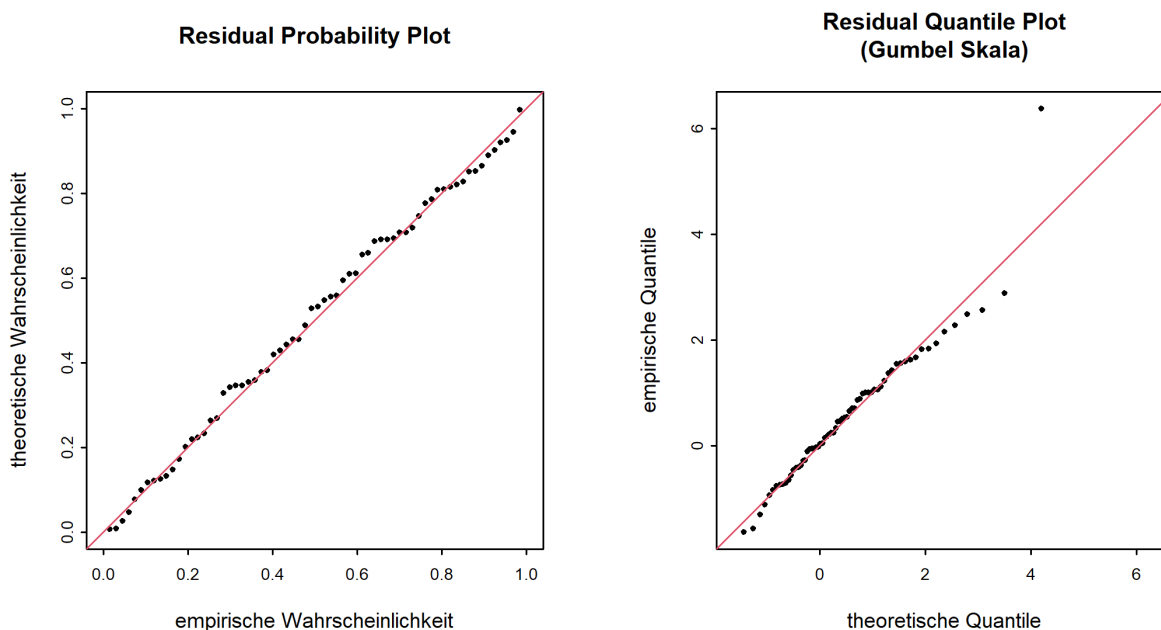
Abbildung 7: Diagnostikplots der Modellvariante “mujump2011” des BLOCK-Ansatzes (01.06.1954 - 31.05.2020)
