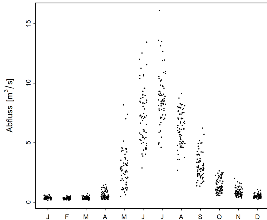
Abbildung 2: Saisonaler Verlauf der monatlichen Minima der M7Q [ \text{m}^3/\text{s} ] (01.06.1954 - 31.05.2020)
