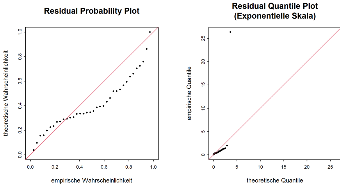
Abbildung 9: Diagnostikplots der Modellvariante “sigl” des POT-Ansatzes (01.06.1954 - 31.05.2020)
