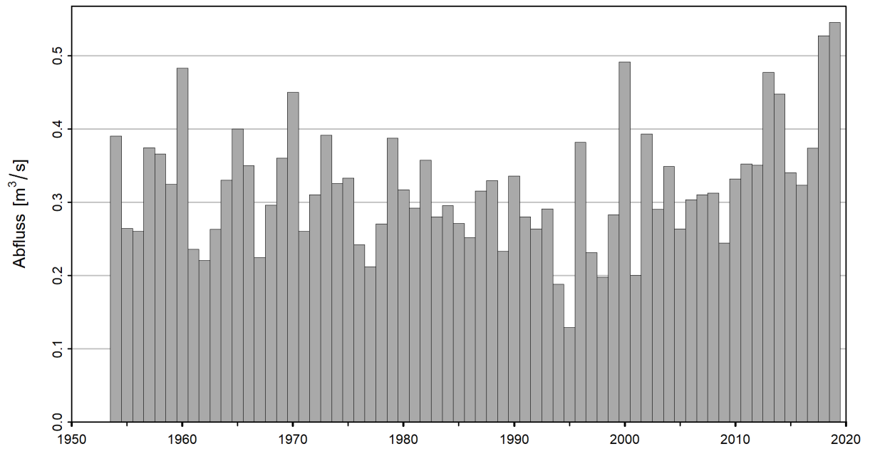
Abbildung 6: Zeitreihe der NM7Q [ \text{m}^3/\text{s} ] (01.06.1954 - 31.05.2020)
