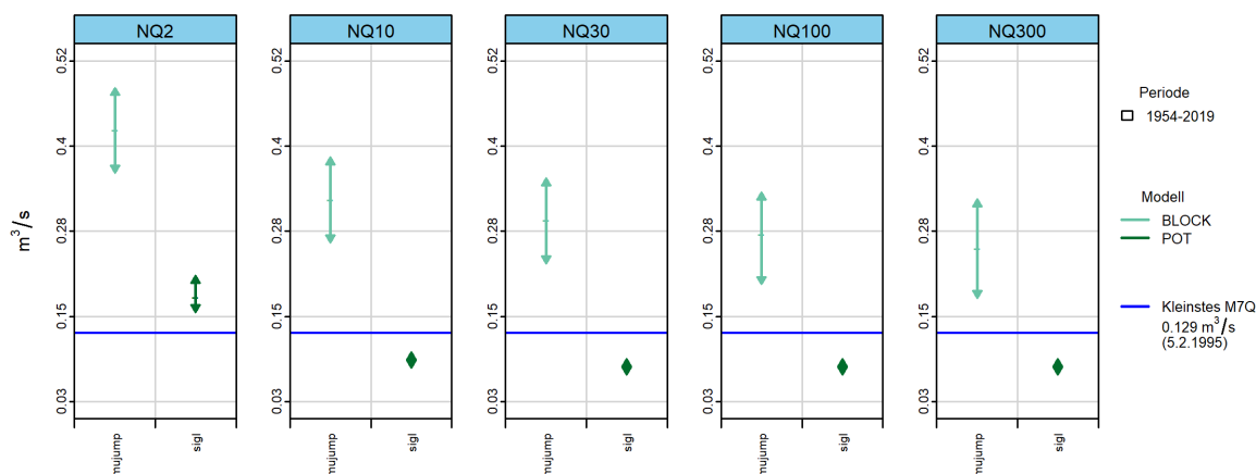
Abbildung 10: NQ_T [m³/s] inkl. 95%-Konfidenzintervalle, berechnet mit den jeweils bestangepassten Modellvarianten des BLOCK- und POT-Ansatzes
