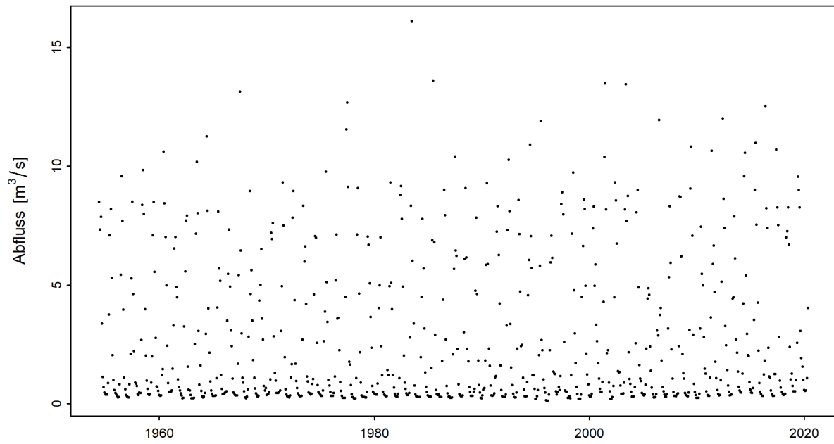
Abbildung 3: Zeitreihe der monatlichen Minima der M7Q [ \text{m}^3/\text{s} ] (01.06.1954 - 31.05.2020)
