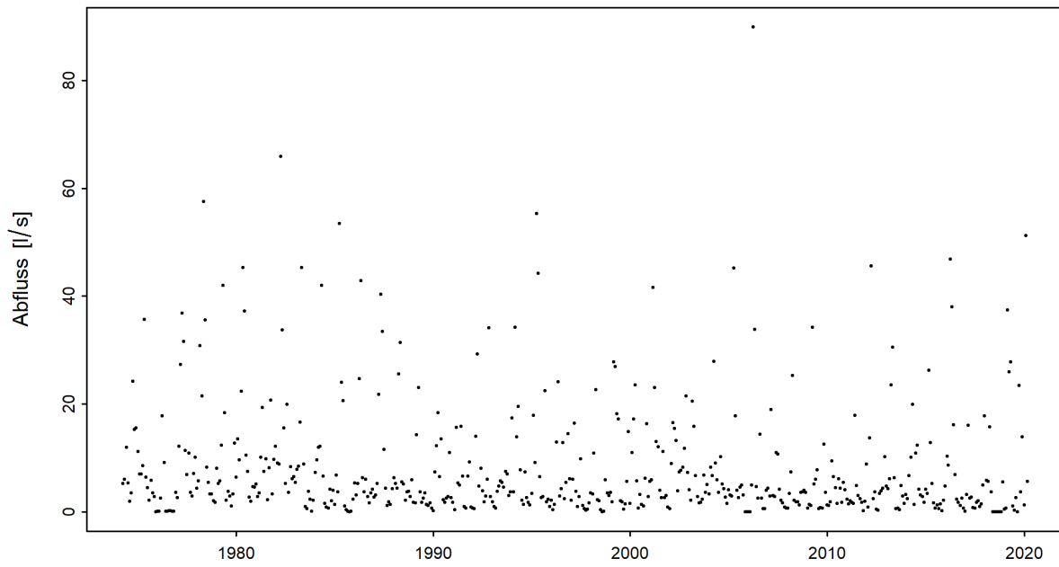
Abbildung 3: Zeitreihe der monatlichen Minima der M7Q [l/s] (01.04.1974 - 31.03.2020)
