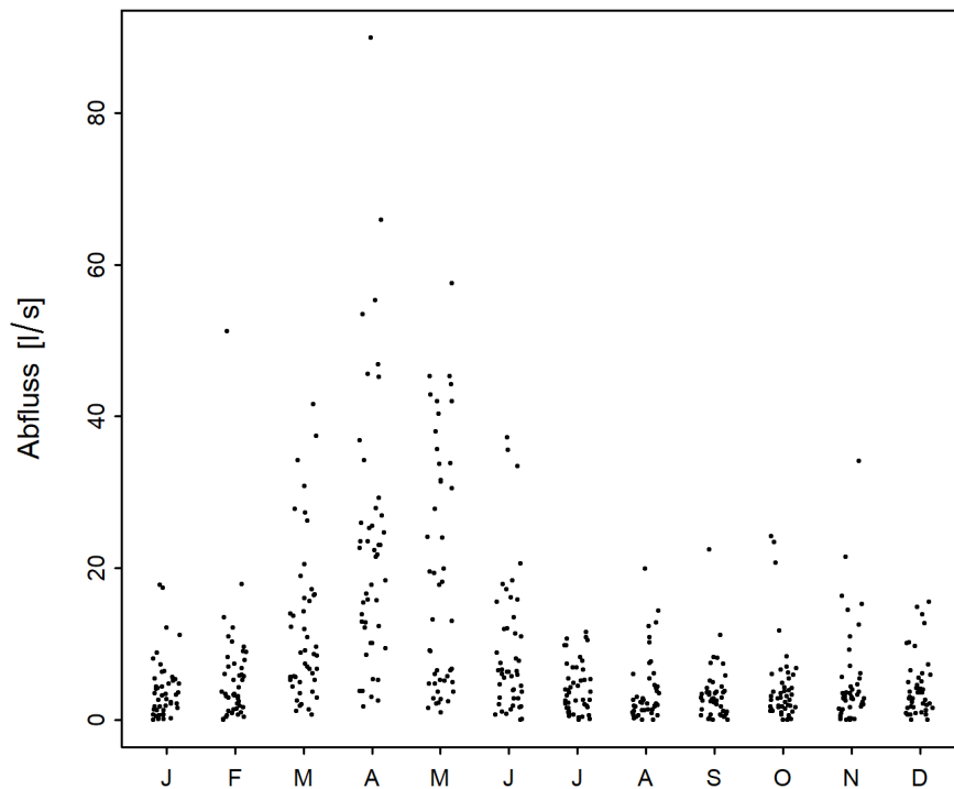
Abbildung 2: Saisonaler Verlauf der monatlichen Minima der M7Q [l/s] (01.04.1974 - 31.03.2020)
