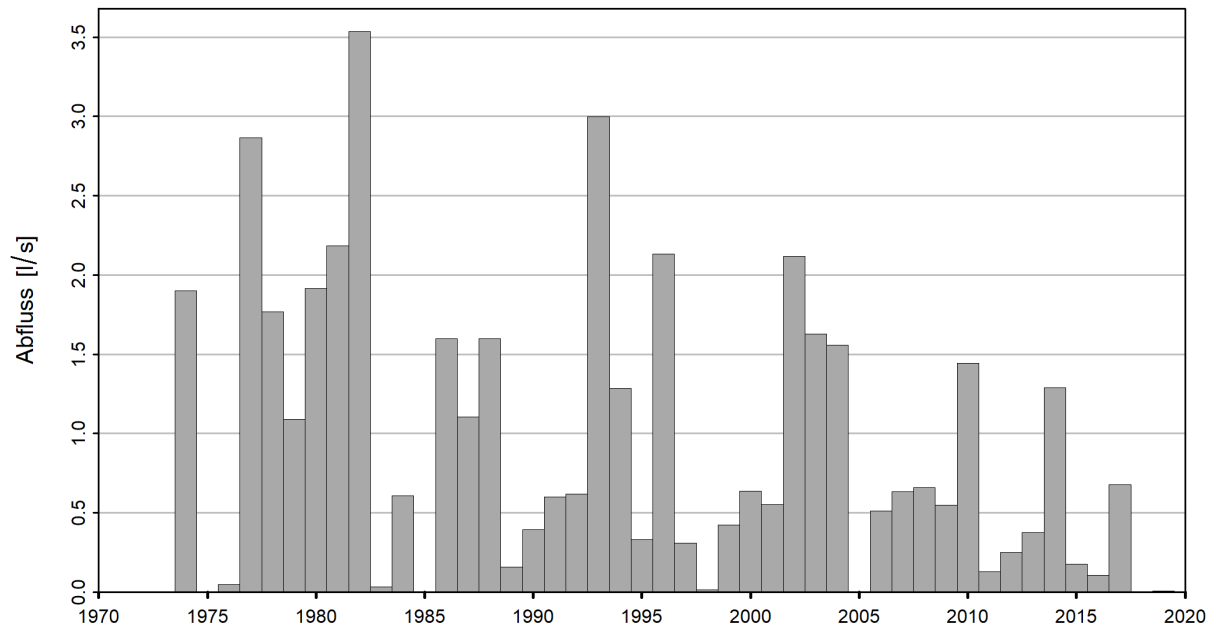
Abbildung 6: Zeitreihe der NM7Q [l/s] (01.04.1974 - 31.03.2020)
