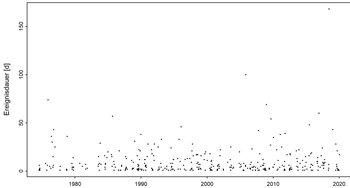
Abbildung 4: Zeitreihe der Niedrigwasserdauern [d] (01.04.1974 - 31.03.2020)
