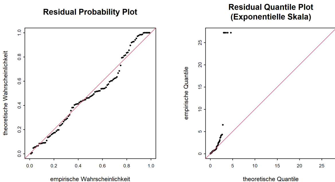
Abbildung 9: Diagnostikplots der Modellvariante "sigjump1983" des POT-Ansatzes (01.04.1974 - 31.03.2020)
