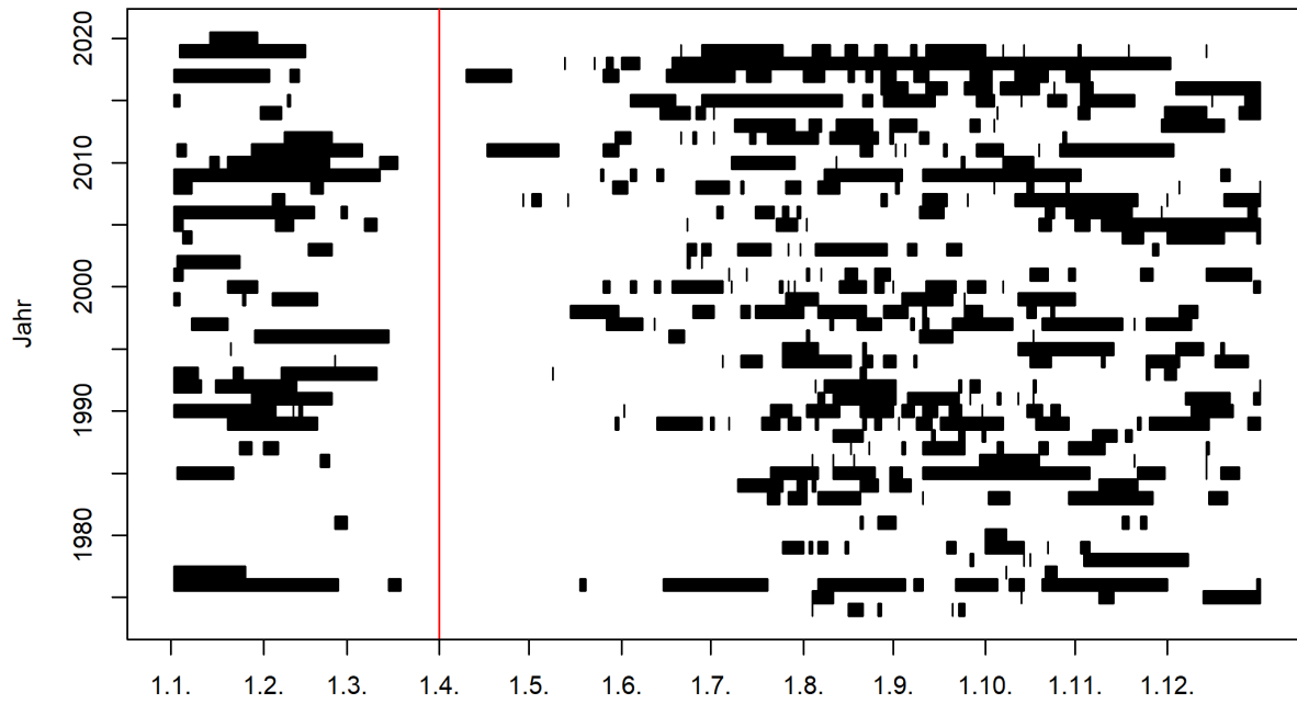
Abbildung 1: Zeitliches Auftreten der Niedrigwasserperioden im Jahresverlauf (01.04.1974 - 31.03.2020) und Startmonat des Niedrigwasserjahres (rote Linie) 1
