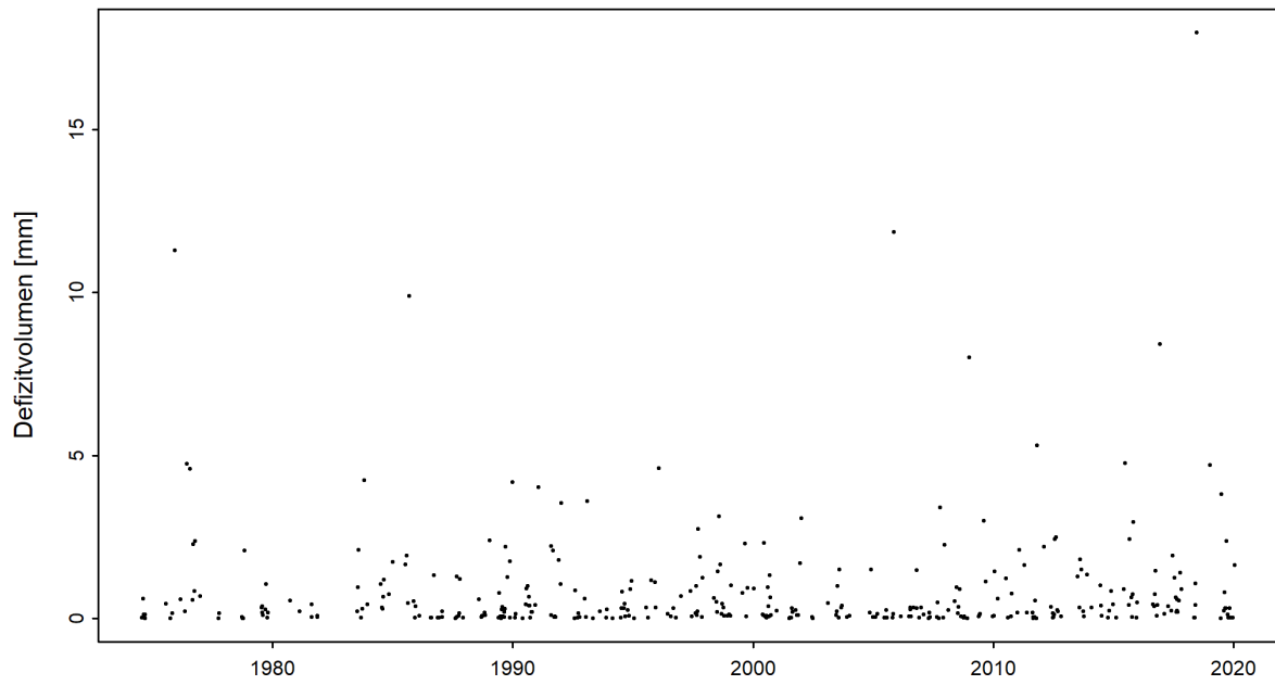
Abbildung 5: Zeitreihe der Defizitvolumen [mm] (01.04.1974 - 31.03.2020)
