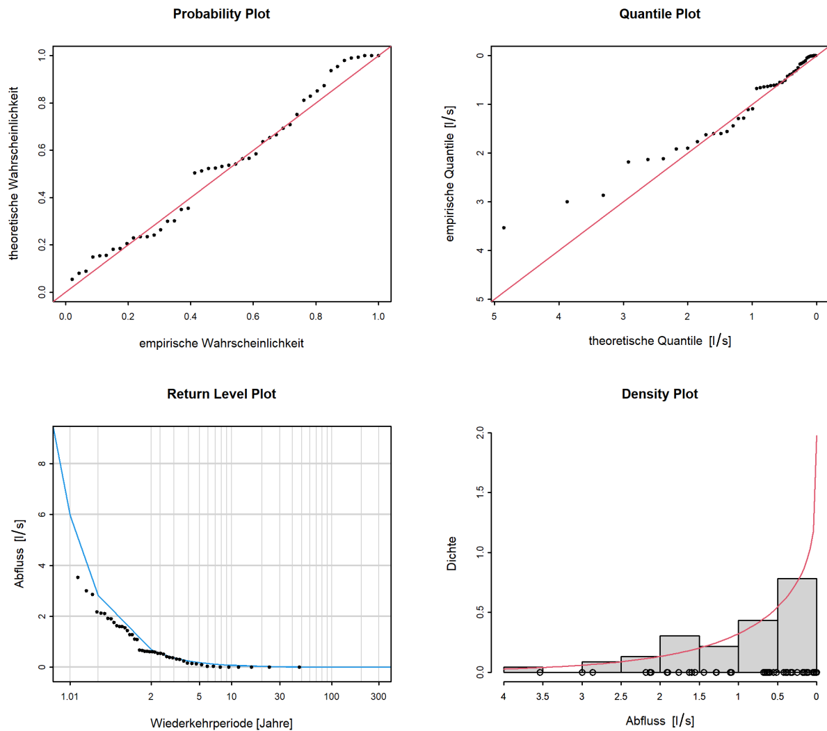
Abbildung 7: Diagnostikplots der Modellvariante “stat” des BLOCK-Ansatzes (01.04.1974 - 31.03.2020)
