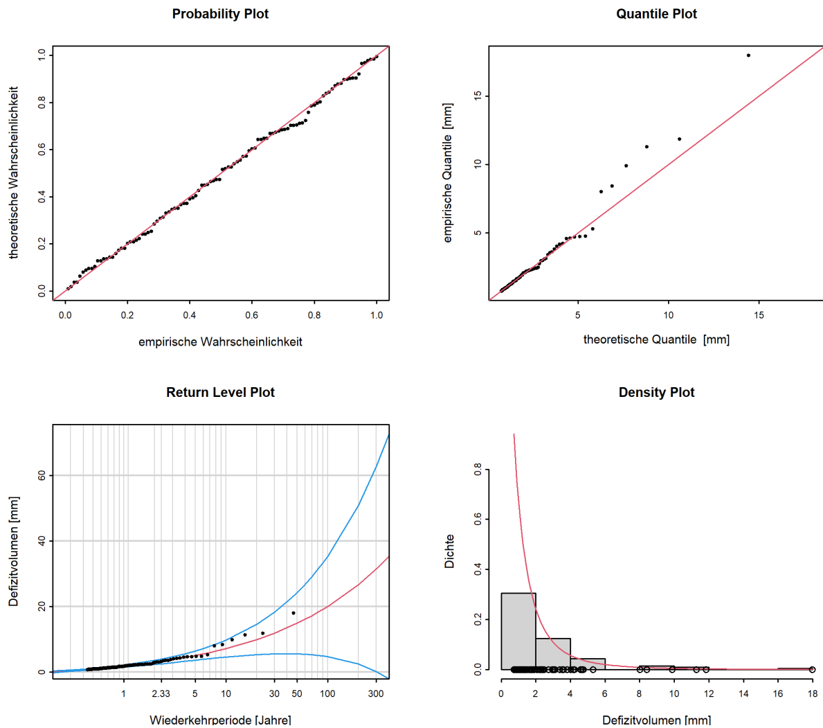
Abbildung 14: Diagnostikplots der Modellvariante “stat” des POT-Ansatzes (01.04.1974 - 31.03.2020)
