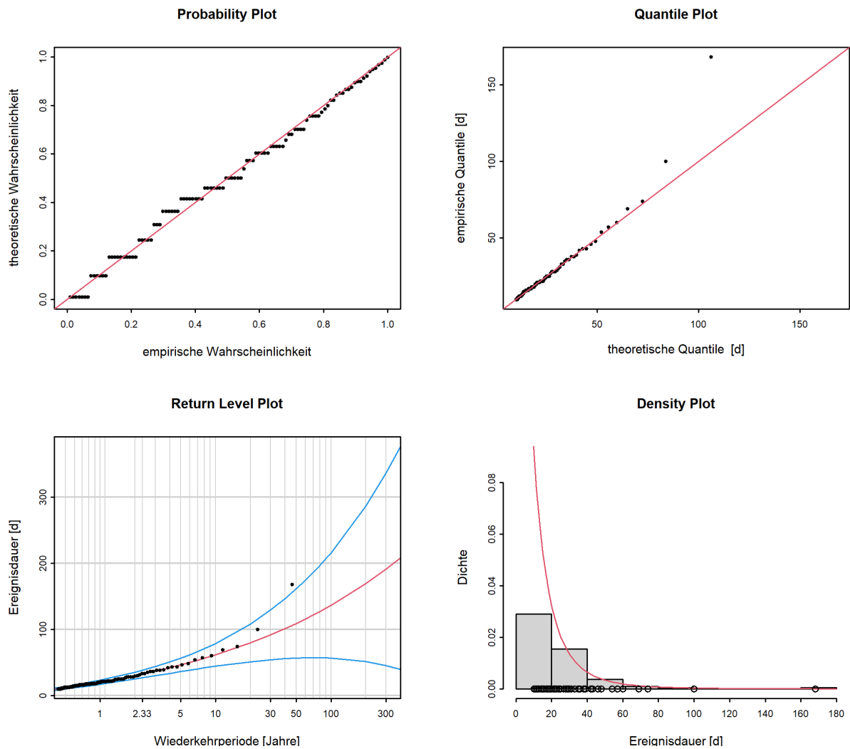
Abbildung 12: Diagnostikplots der Modellvariante "stat" des POT-Ansatzes (01.04.1974 - 31.03.2020)
