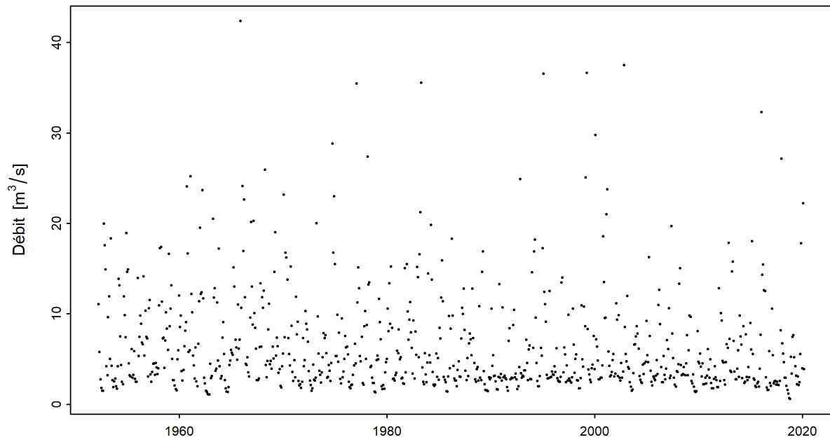
FIGURE 3 – Série temporelle du minimum mensuel de M7Q [m 3 /s] (01.04.1952 - 31.03.2020)
