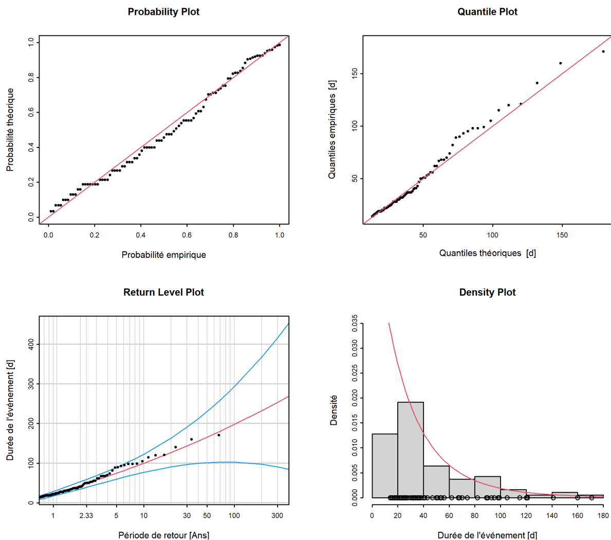
FIGURE 12 – Graphiques diagnostiques de la variante du modèle “ stat ” de la méthode POT (01.04.1953 - 31.03.2020)
