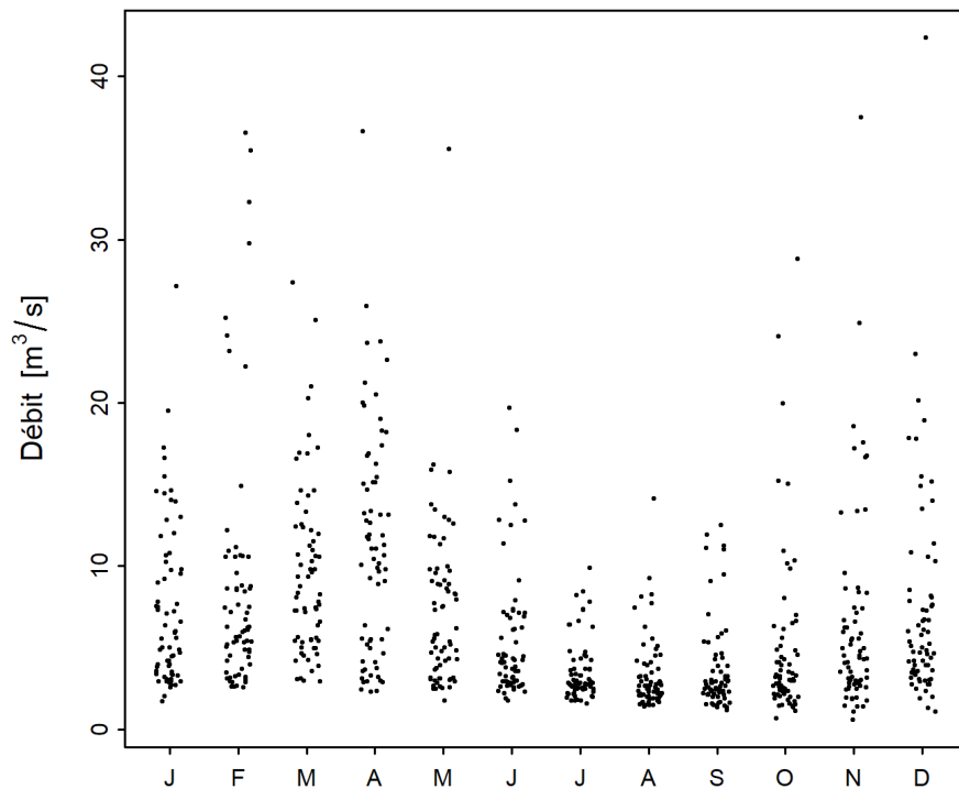
FIGURE 2 – Évolution saisonnière du minimum mensuel de M7Q [ \text{m}^3/\text{s} ] (01.04.1952 - 31.03.2020)
