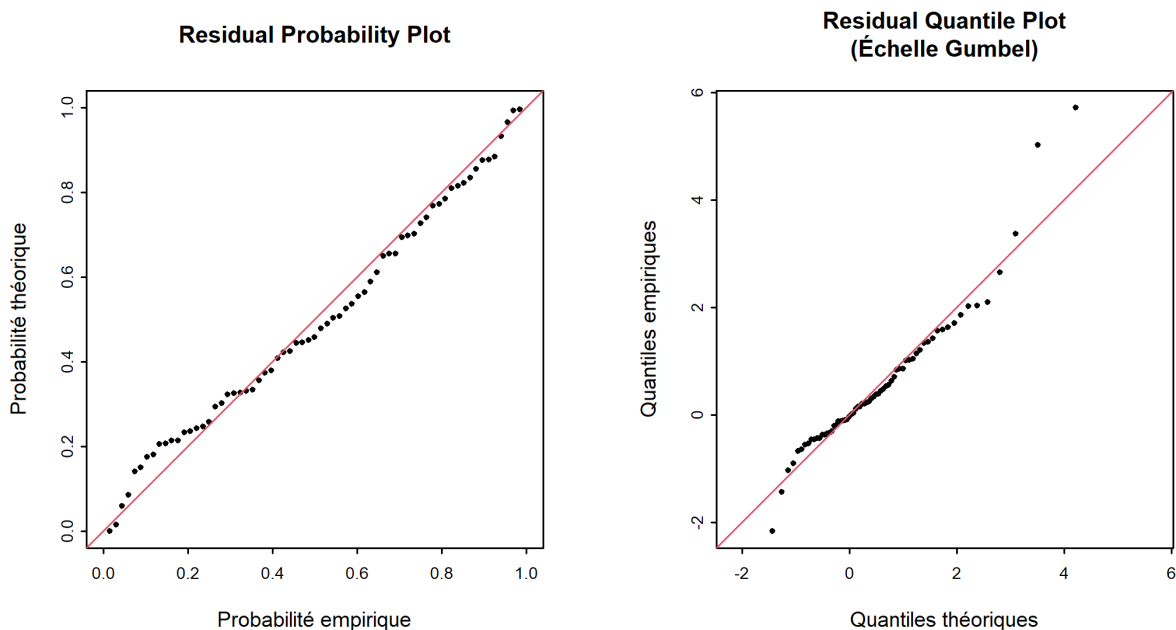
FIGURE 7 – Graphiques diagnostiques de la variante du modèle " mujump1969 " de la méthode BLOCK (01.04.1953 - 31.03.2020)
