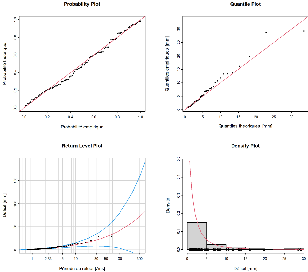
FIGURE 14 – Graphiques diagnostiques de la variante du modèle “ stat ” de la méthode POT (01.04.1953 - 31.03.2020)
