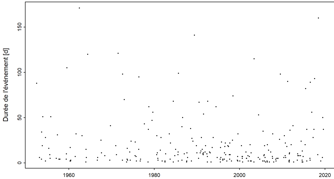
FIGURE 4 – Série temporelle des durées d'étéage [d] (01.04.1952 - 31.03.2020)
