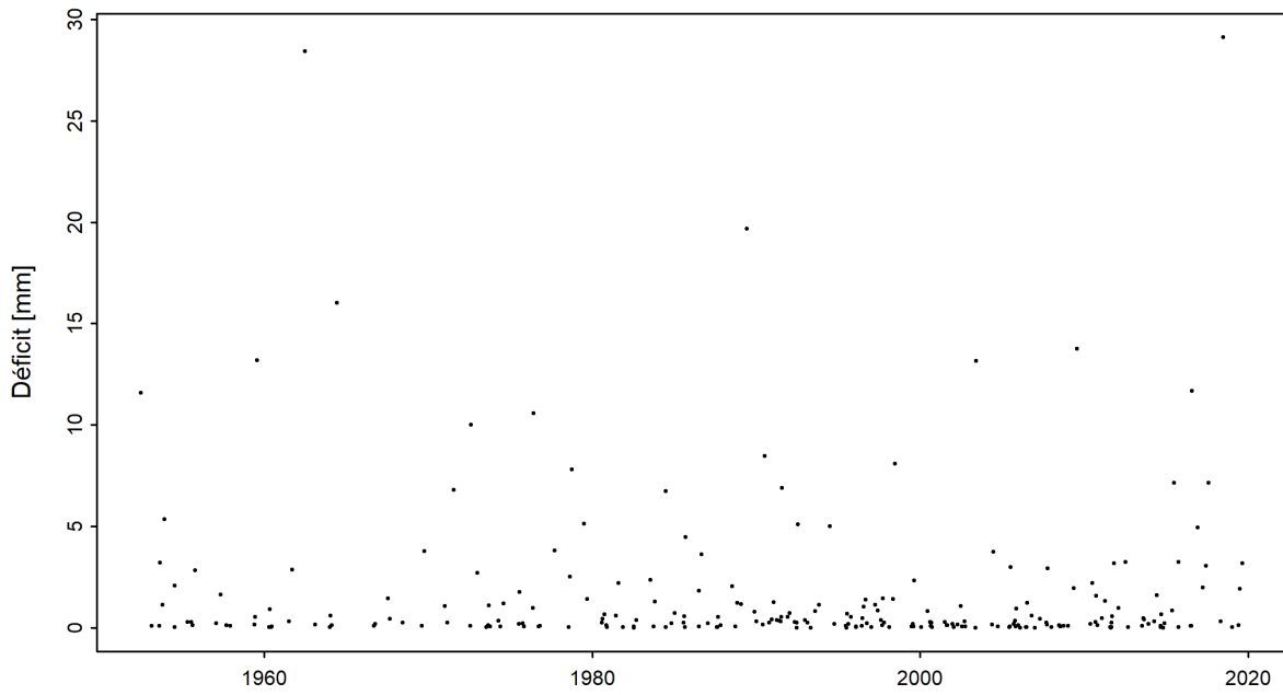
FIGURE 5 – Série temporelle du volume déficitaire [mm] (01.04.1952 - 31.03.2020)
