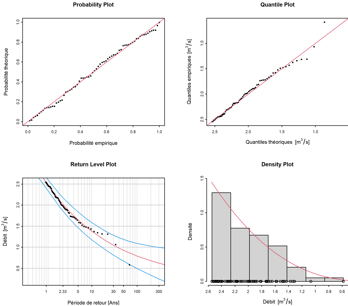
FIGURE 9 – Graphiques diagnostiques de la variante du modèle “ stat ” de la méthode POT (01.04.1953 - 31.03.2020)
