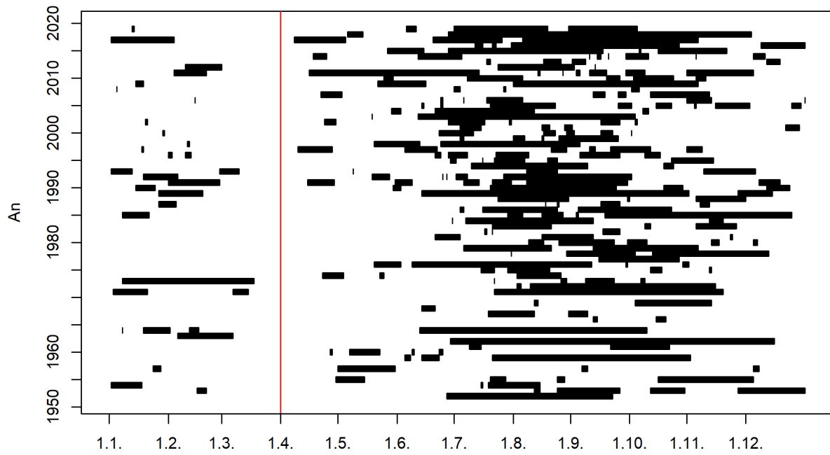
FIGURE 1 – Apparition temporelle des périodes d'étiage pendant l'année (01.04.1952 - 31.03.2020) et mois de début de l'année d'étiage (ligne rouge) 1
