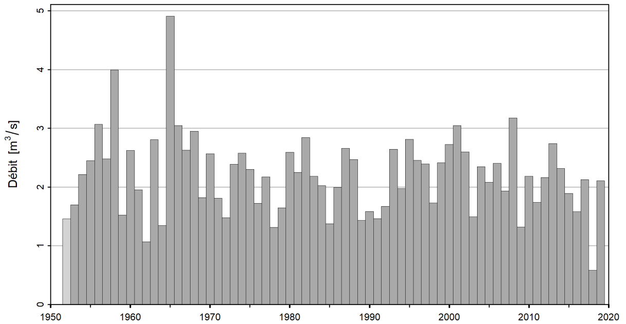
FIGURE 6 – Série temporelle de NM7Q [ \text{m}^3/\text{s} ] (01.04.1952 - 31.03.2020), gris clair : NM7Q non utilisés, gris foncé : NM7Q utilisés
