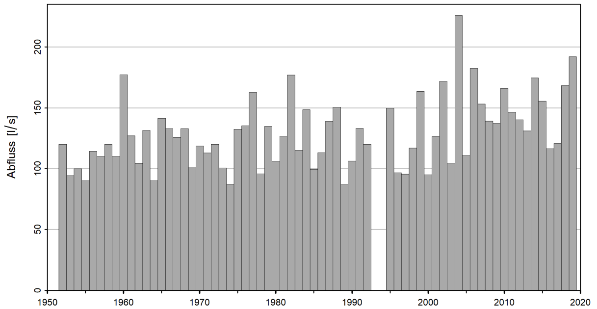
Abbildung 6: Zeitreihe der NM7Q [l/s] (01.06.1952 - 31.05.2020)
