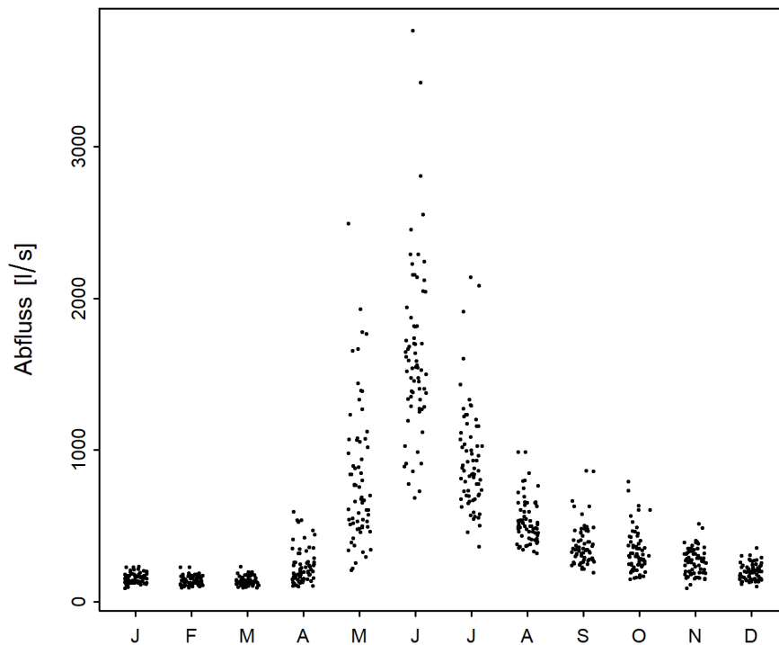
Abbildung 2: Saisonaler Verlauf der monatlichen Minima der M7Q [l/s] (01.06.1952 - 31.05.2020)
