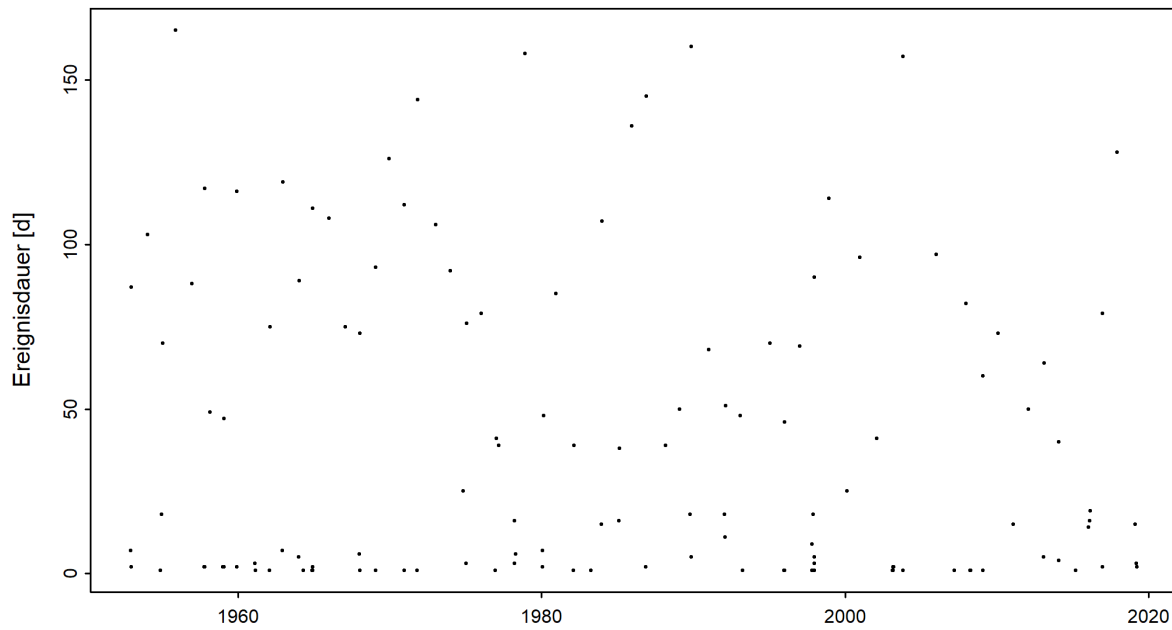
Abbildung 4: Zeitreihe der Niedrigwasserdauern [d] (01.06.1952 - 31.05.2020)
