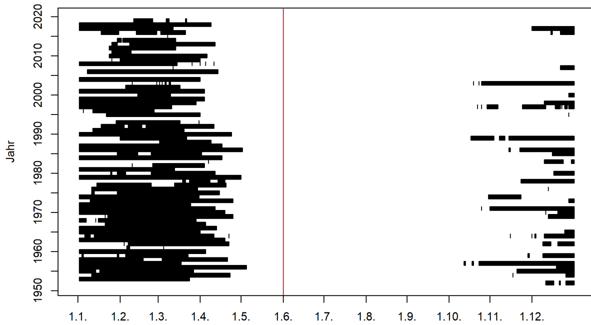
Abbildung 1: Zeitliches Auftreten der Niedrigwasserperioden im Jahresverlauf (01.06.1952 - 31.05.2020) und Startmonat des Niedrigwasserjahres (rote Linie) 1
