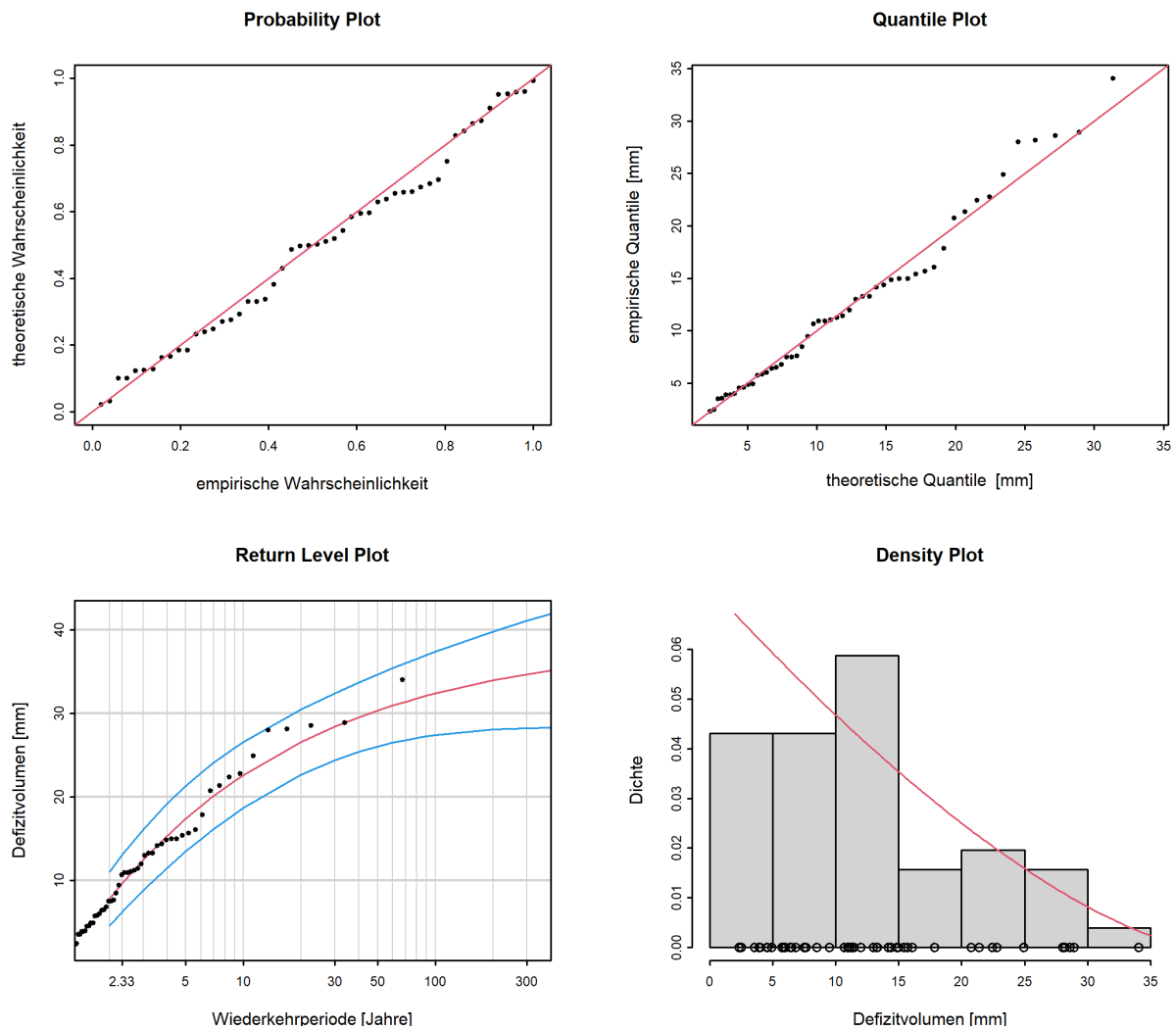
Abbildung 14: Diagnostikplots der Modellvariante “stat” des POT-Ansatzes (01.06.1952 - 31.05.2020)
