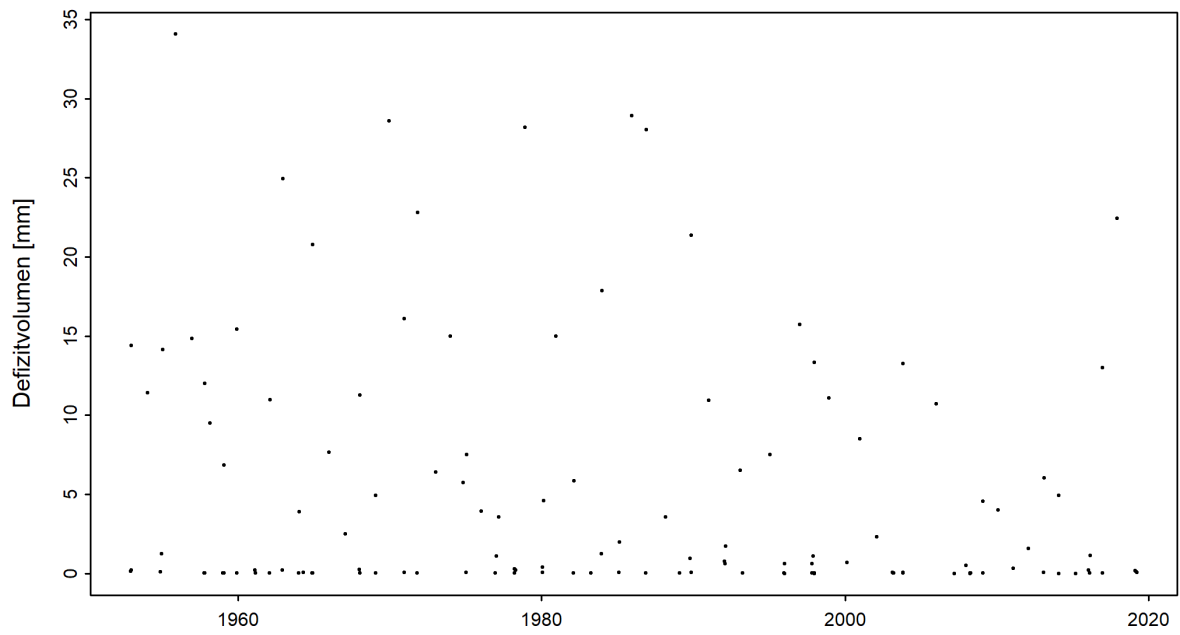
Abbildung 5: Zeitreihe der Defizitvolumen [mm] (01.06.1952 - 31.05.2020)
