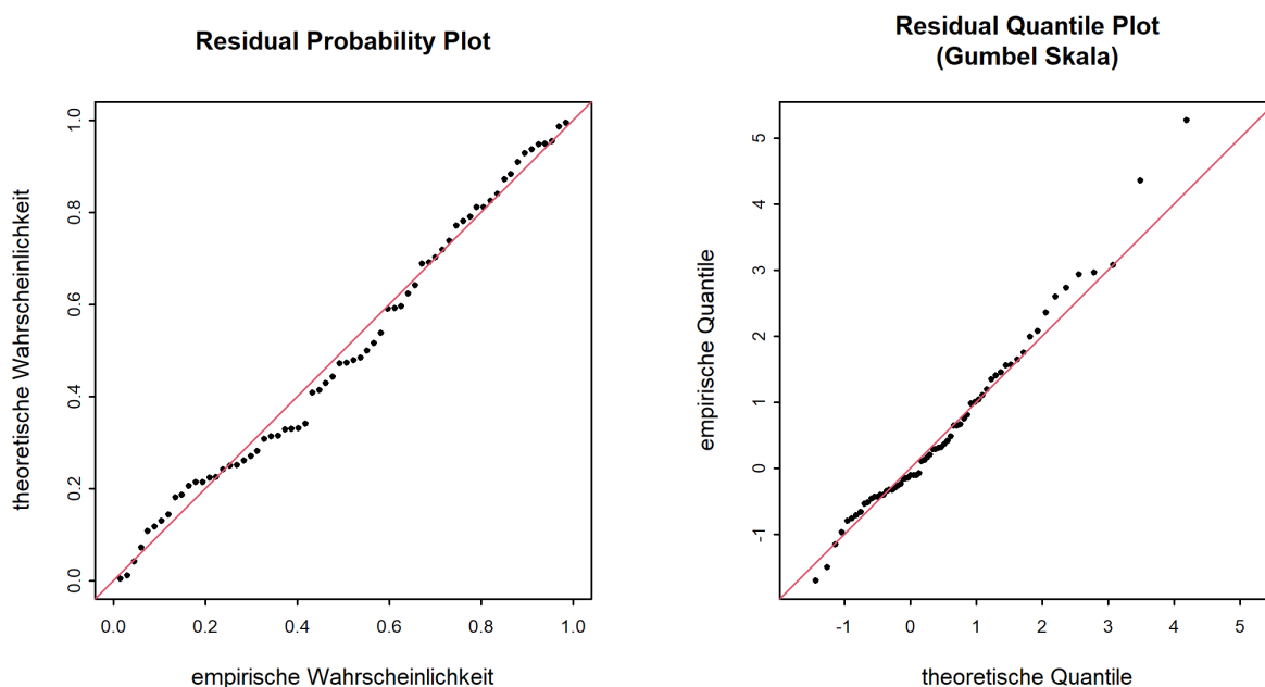
Abbildung 7: Diagnostikplots der Modellvariante "musigl" des BLOCK-Ansatzes (01.06.1952 - 31.05.2020)
