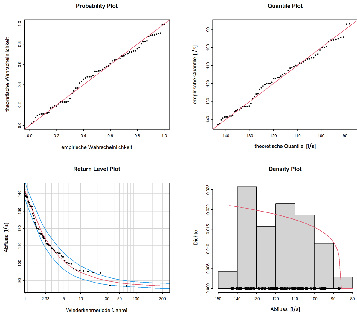
Abbildung 9: Diagnostikplots der Modellvariante “stat” des POT-Ansatzes (01.06.1952 - 31.05.2020)
