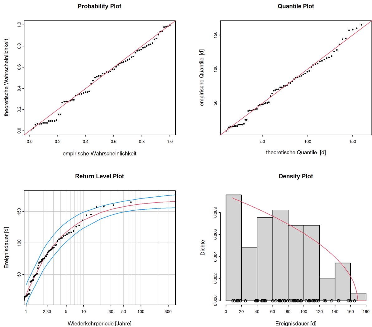
Abbildung 12: Diagnostikplots der Modellvariante “stat” des POT-Ansatzes (01.06.1952 - 31.05.2020)
