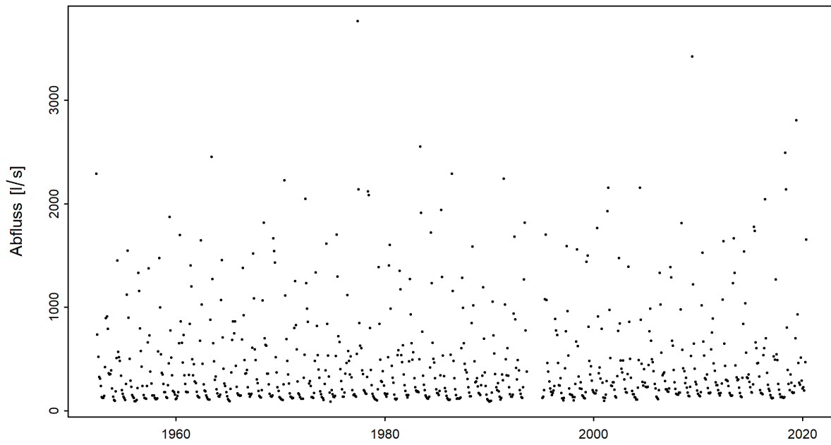
Abbildung 3: Zeitreihe der monatlichen Minima der M7Q [l/s] (01.06.1952 - 31.05.2020)
