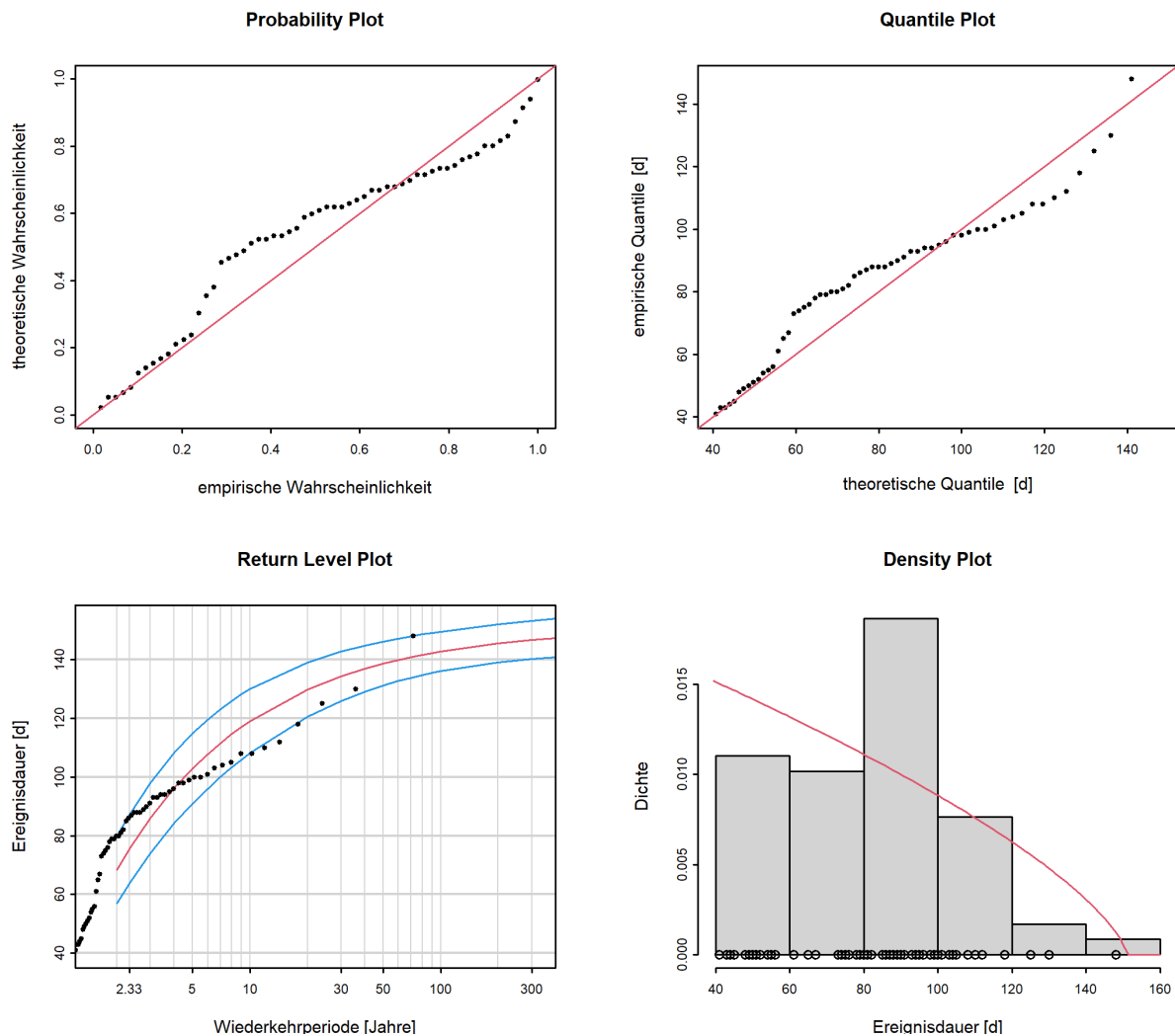
Abbildung 12: Diagnostikplots der Modellvariante “stat” des POT-Ansatzes (01.06.1949 - 31.05.2020)
