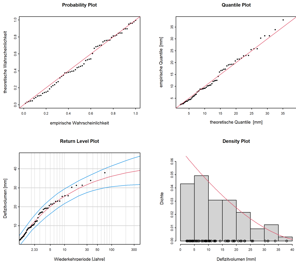
Abbildung 14: Diagnostikplots der Modellvariante “stat” des POT-Ansatzes (01.06.1949 - 31.05.2020)
