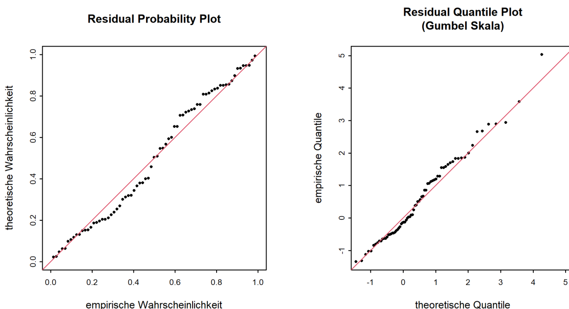
Abbildung 7: Diagnostikplots der Modellvariante “muq” des BLOCK-Ansatzes (01.06.1949 - 31.05.2020)
