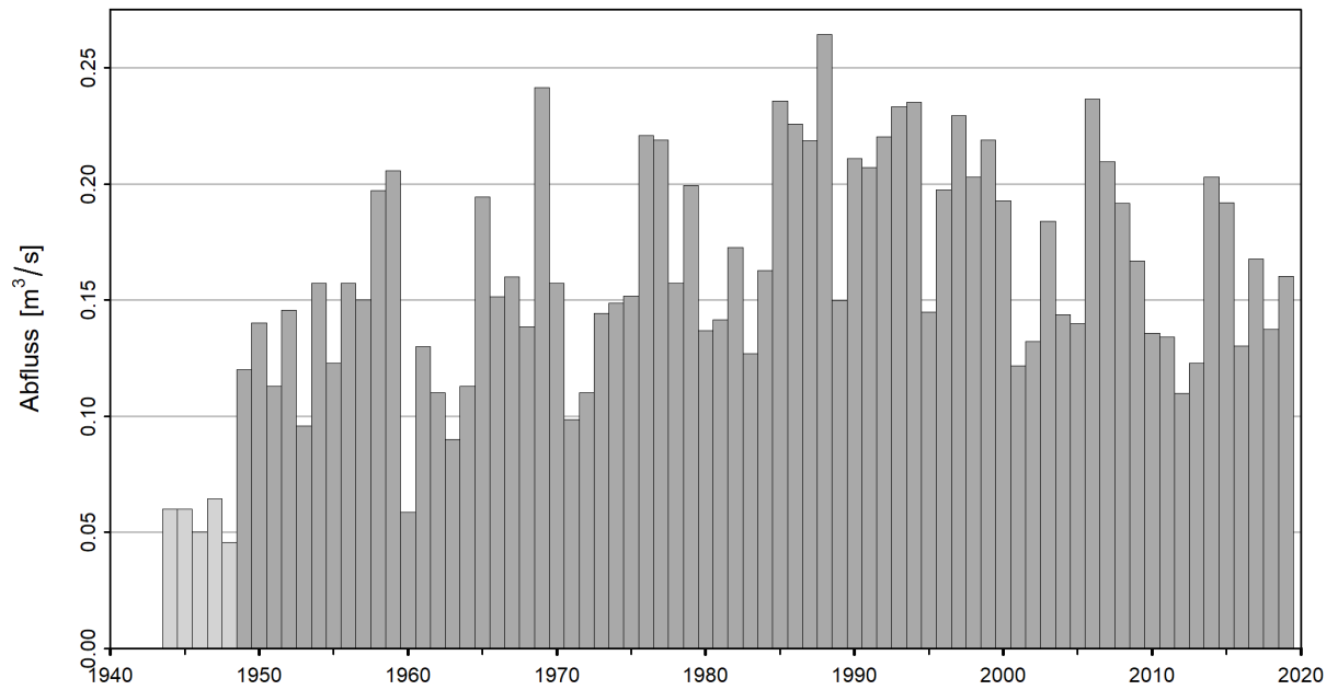
Abbildung 6: Zeitreihe der NM7Q [m³/s] (01.06.1944 - 31.05.2020), hellgrau: nicht verwendete NM7Q, dunkelgrau: verwendete NM7Q
