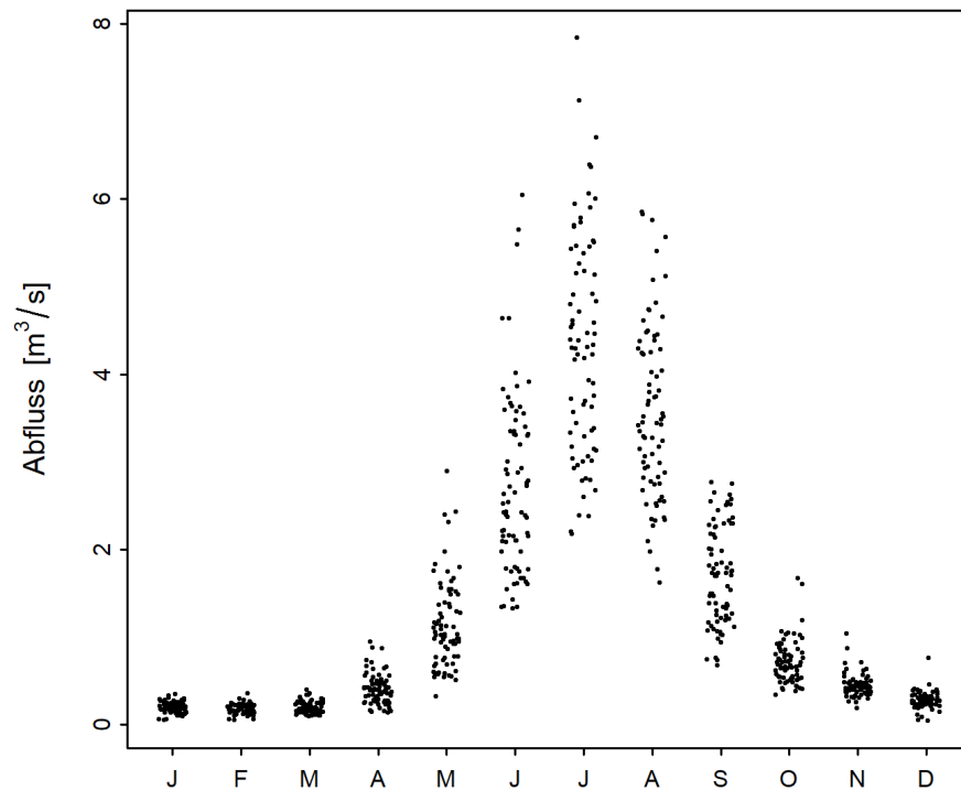
Abbildung 2: Saisonaler Verlauf der monatlichen Minima der M7Q [m³/s] (01.06.1944 - 31.05.2020)
