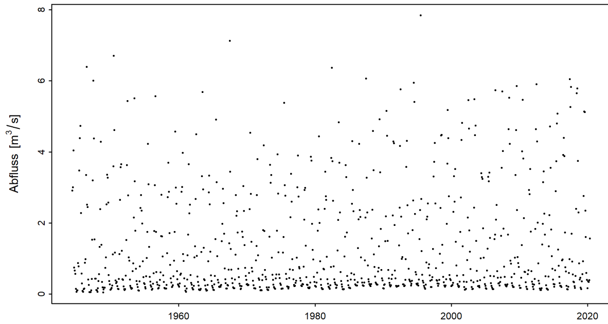
Abbildung 3: Zeitreihe der monatlichen Minima der M7Q [ \text{m}^3/\text{s} ] (01.06.1944 - 31.05.2020)
