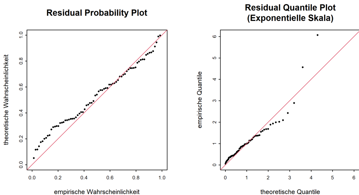
Abbildung 9: Diagnostikplots der Modellvariante “sigl” des POT-Ansatzes (01.06.1949 - 31.05.2020)
