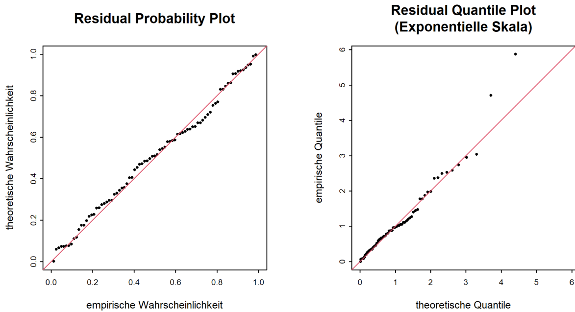
Abbildung 9: Diagnostikplots der Modellvariante “sigjump1981” des POT-Ansatzes (01.04.1958 - 31.03.2019)
