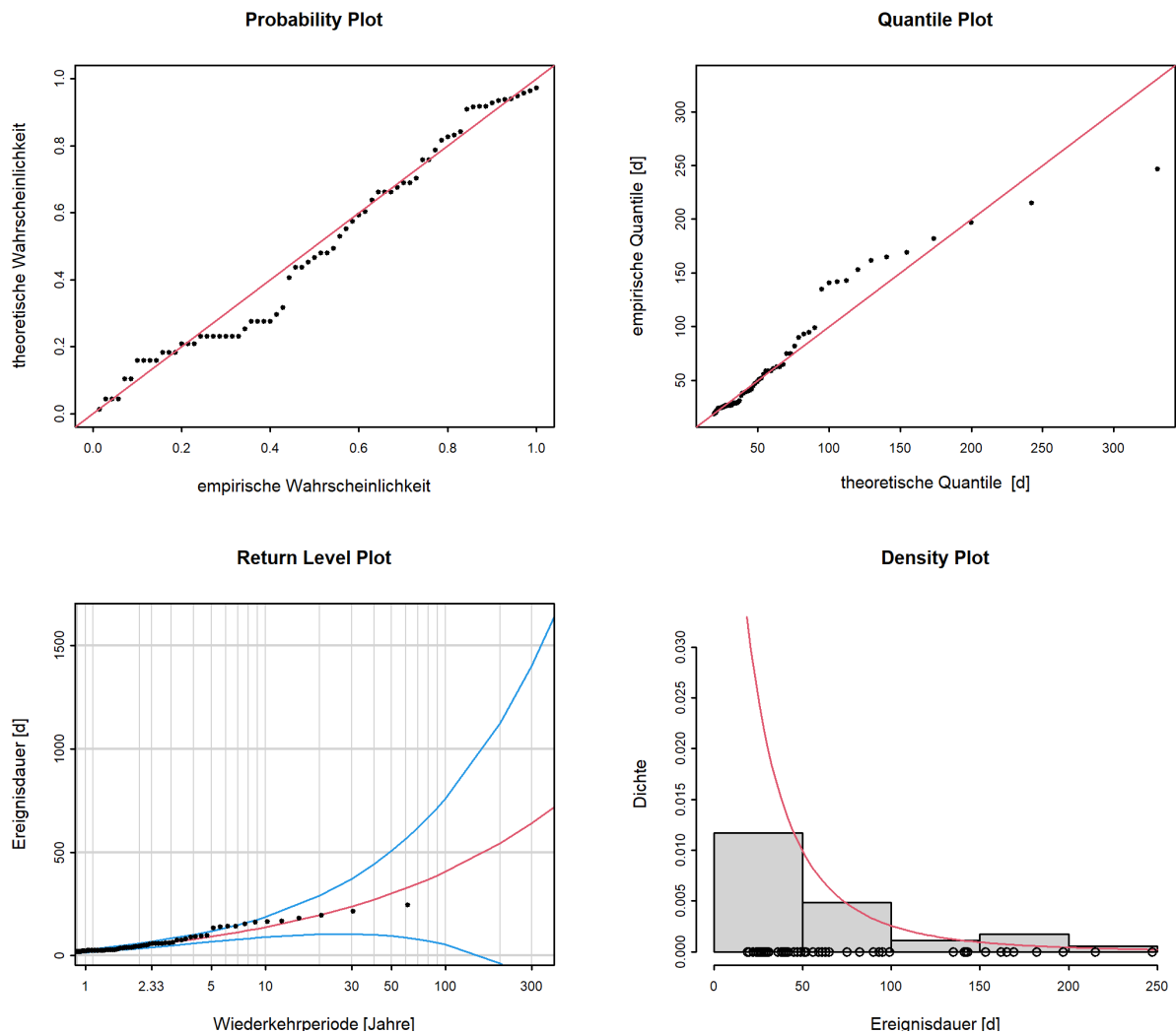
Abbildung 12: Diagnostikplots der Modellvariante “stat” des POT-Ansatzes (01.04.1958 - 31.03.2019)
