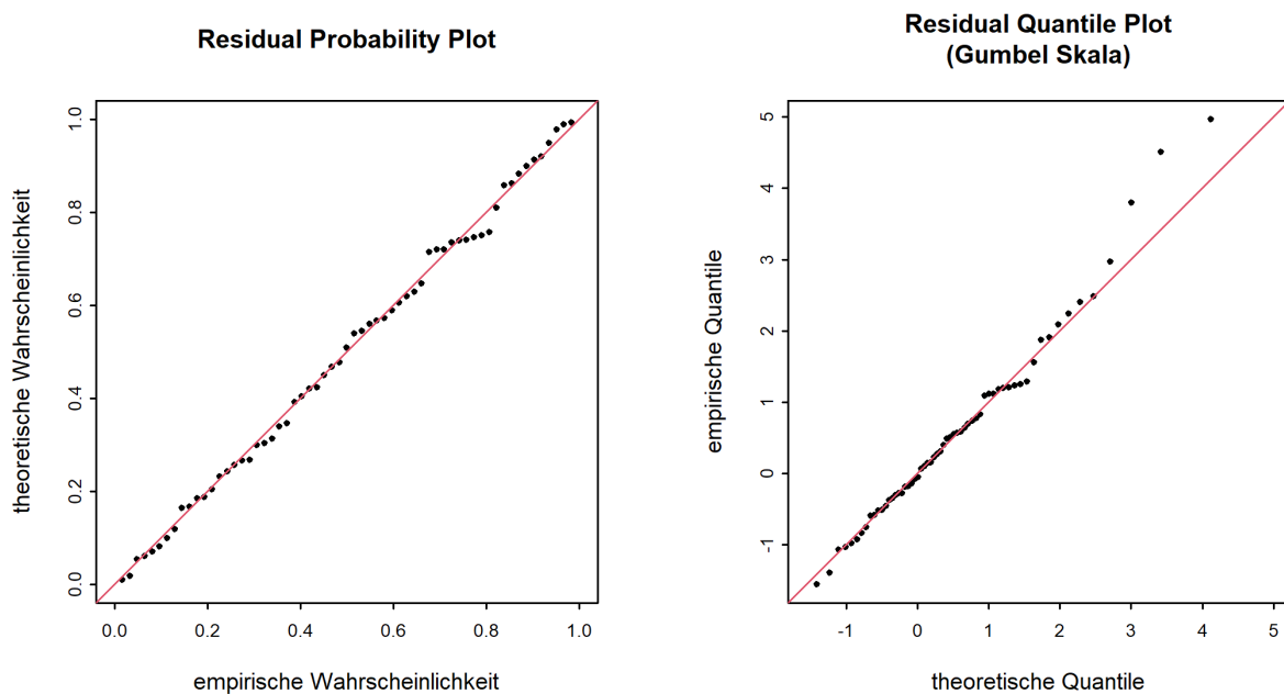
Abbildung 7: Diagnostikplots der Modellvariante "sigl" des BLOCK-Ansatzes (01.04.1958 - 31.03.2019)
