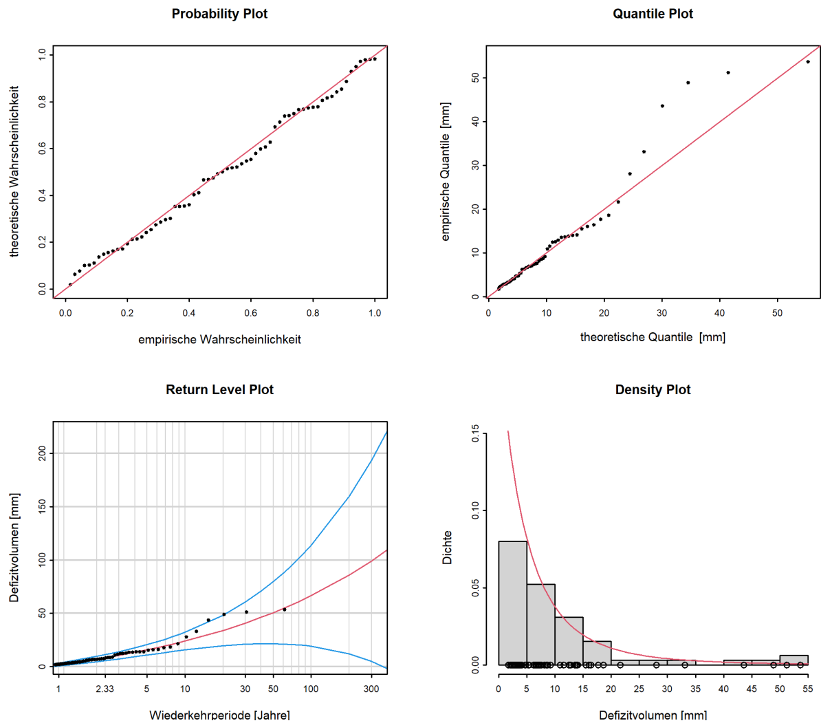
Abbildung 14: Diagnostikplots der Modellvariante “stat” des POT-Ansatzes (01.04.1958 - 31.03.2019)
