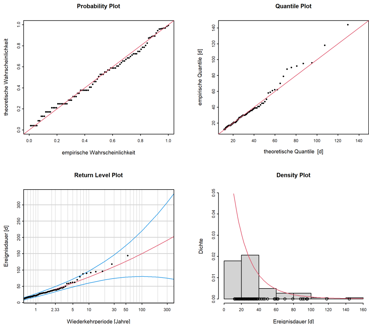
Abbildung 12: Diagnostikplots der Modellvariante "stat" des POT-Ansatzes (01.04.1965 - 31.03.2019)
