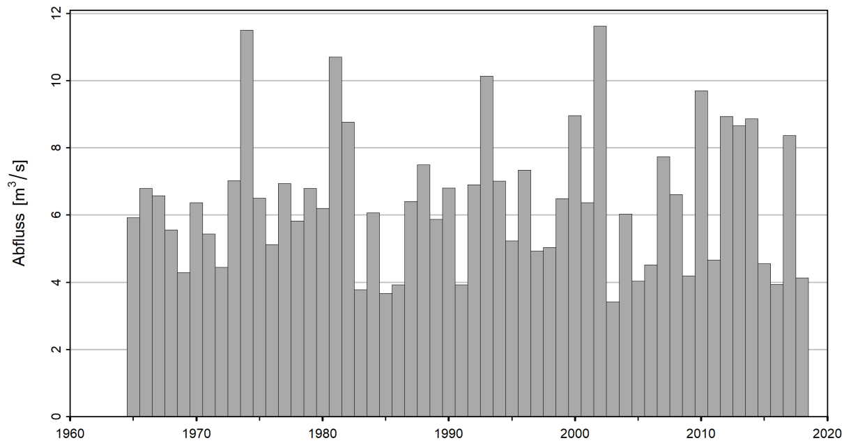
Abbildung 6: Zeitreihe der NM7Q [ \text{m}^3/\text{s} ] (01.04.1965 - 31.03.2019)
