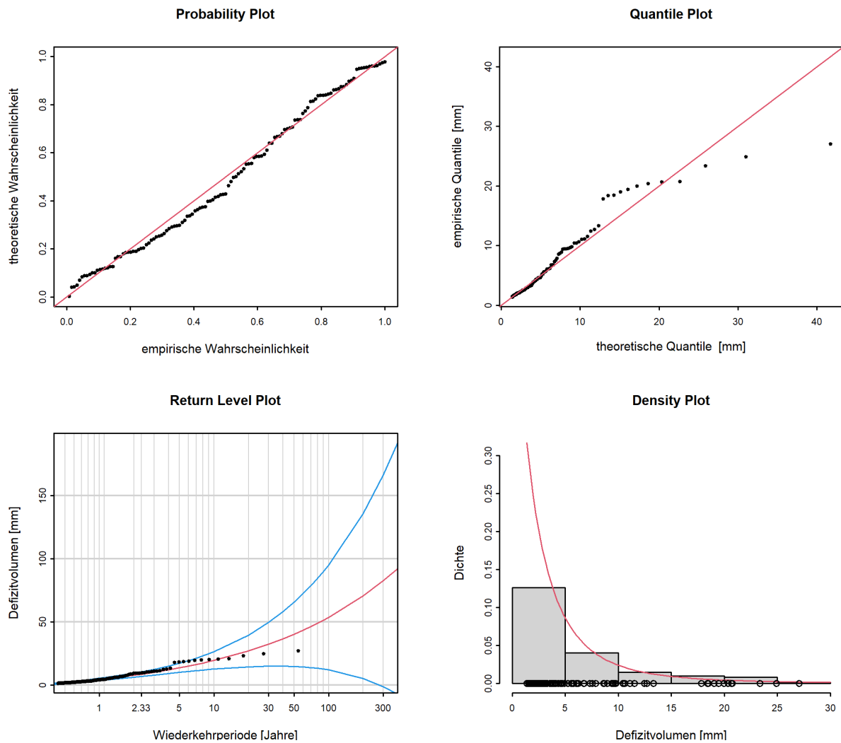
Abbildung 14: Diagnostikplots der Modellvariante "stat" des POT-Ansatzes (01.04.1965 - 31.03.2019)
