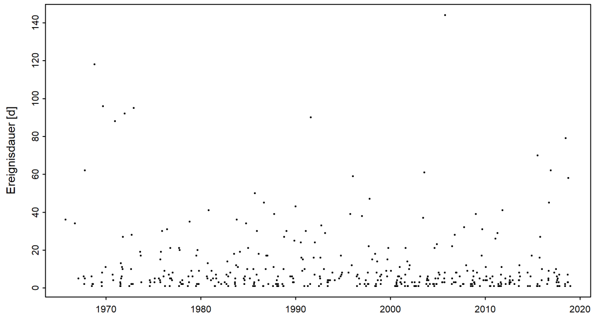
Abbildung 4: Zeitreihe der Niedrigwasserdauern [d] (01.04.1965 - 31.03.2019)
