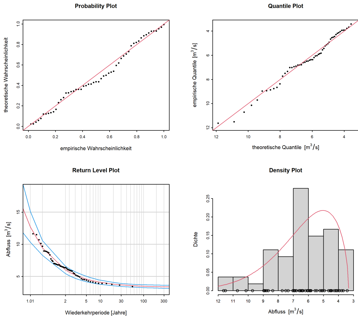
Abbildung 7: Diagnostikplots der Modellvariante “stat” des BLOCK-Ansatzes (01.04.1965 - 31.03.2019)
