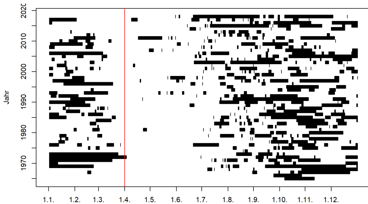
Abbildung 1: Zeitliches Auftreten der Niedrigwasserperioden im Jahresverlauf (01.04.1965 - 31.03.2019) und Startmonat des Niedrigwasserjahres (rote Linie) 1
