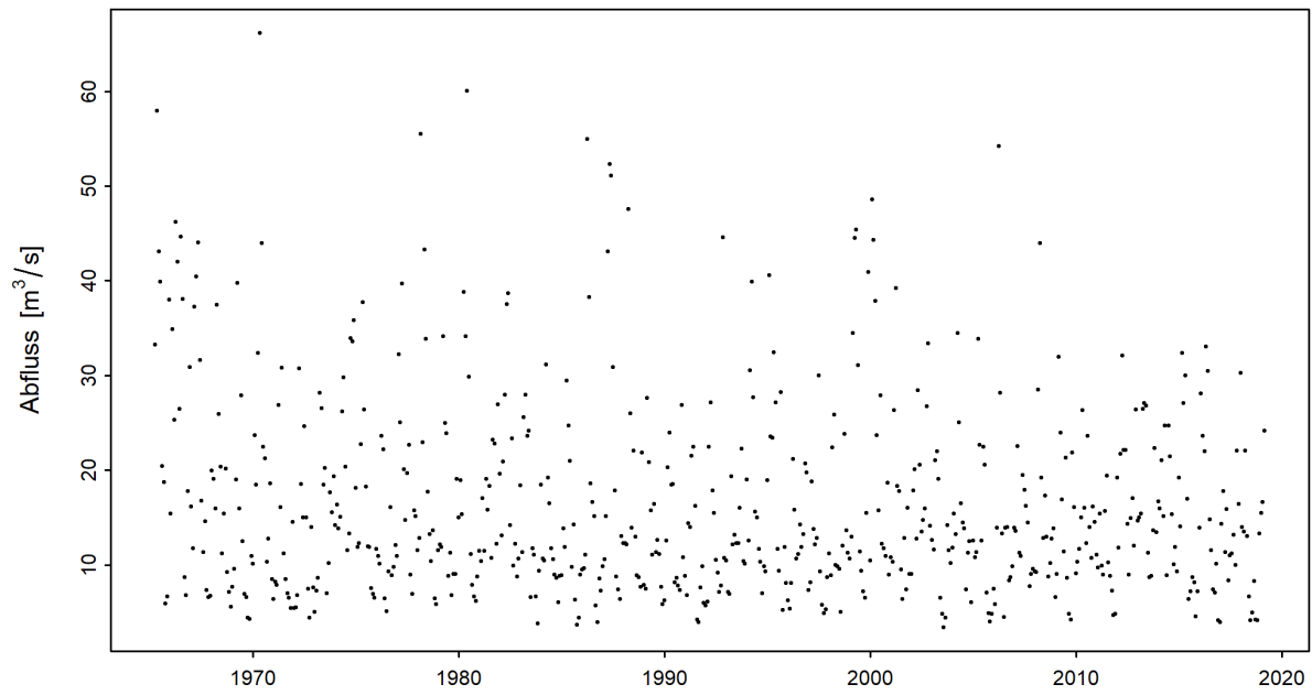
Abbildung 3: Zeitreihe der monatlichen Minima der M7Q [ \text{m}^3/\text{s} ] (01.04.1965 - 31.03.2019)
