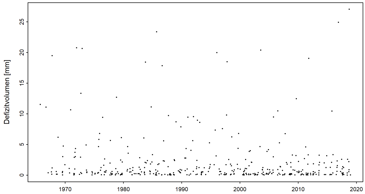
Abbildung 5: Zeitreihe der Defizitvolumen [mm] (01.04.1965 - 31.03.2019)
