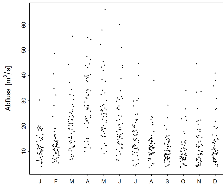
Abbildung 2: Saisonaler Verlauf der monatlichen Minima der M7Q [ \text{m}^3/\text{s} ] (01.04.1965 - 31.03.2019)
