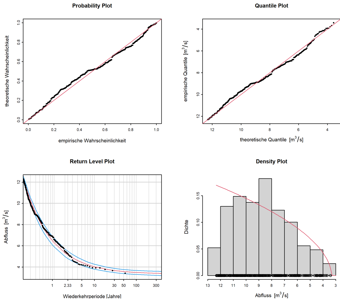
Abbildung 9: Diagnostikplots der Modellvariante “stat” des POT-Ansatzes (01.04.1965 - 31.03.2019)
