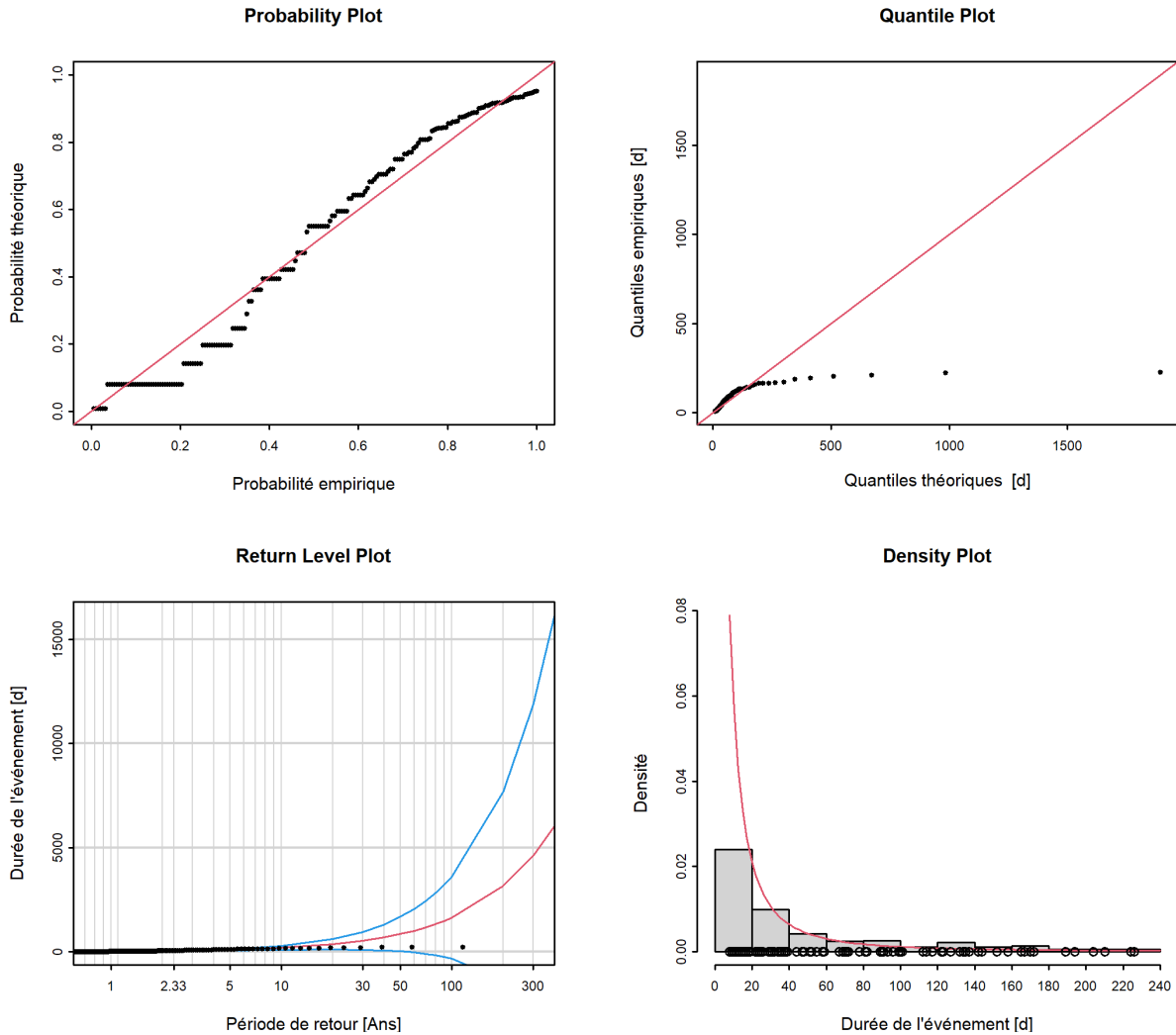
FIGURE 12 – Graphiques diagnostiques de la variante du modèle “ stat ” de la méthode POT (01.07.1904 - 30.06.2020)
