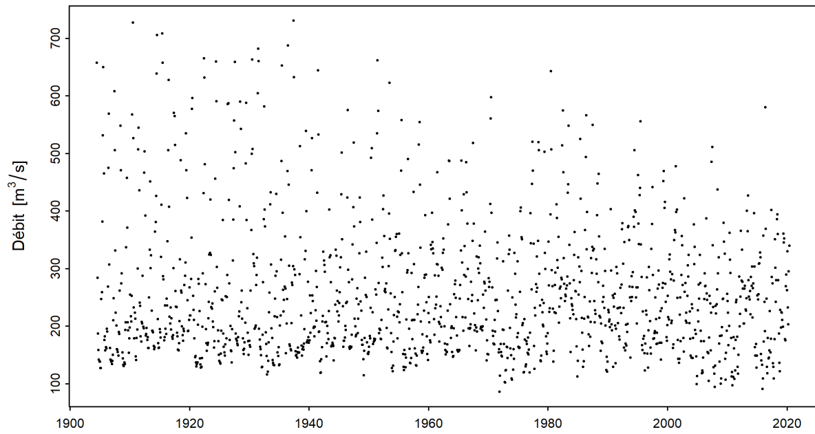
FIGURE 3 – Série temporelle du minimum mensuel de M7Q [m 3 /s] (01.07.1904 - 30.06.2020)
