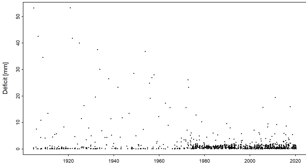
FIGURE 5 – Série temporelle du volume déficitaire [mm] (01.07.1904 - 30.06.2020)
