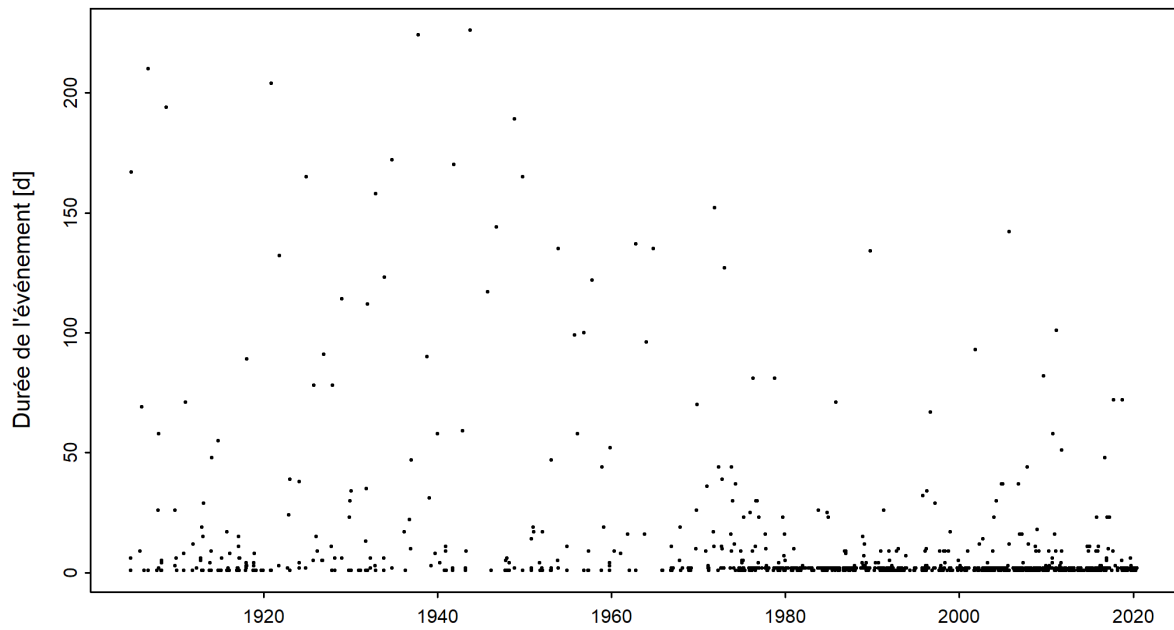
FIGURE 4 – Série temporelle des durées d'étiage [d] (01.07.1904 - 30.06.2020)
