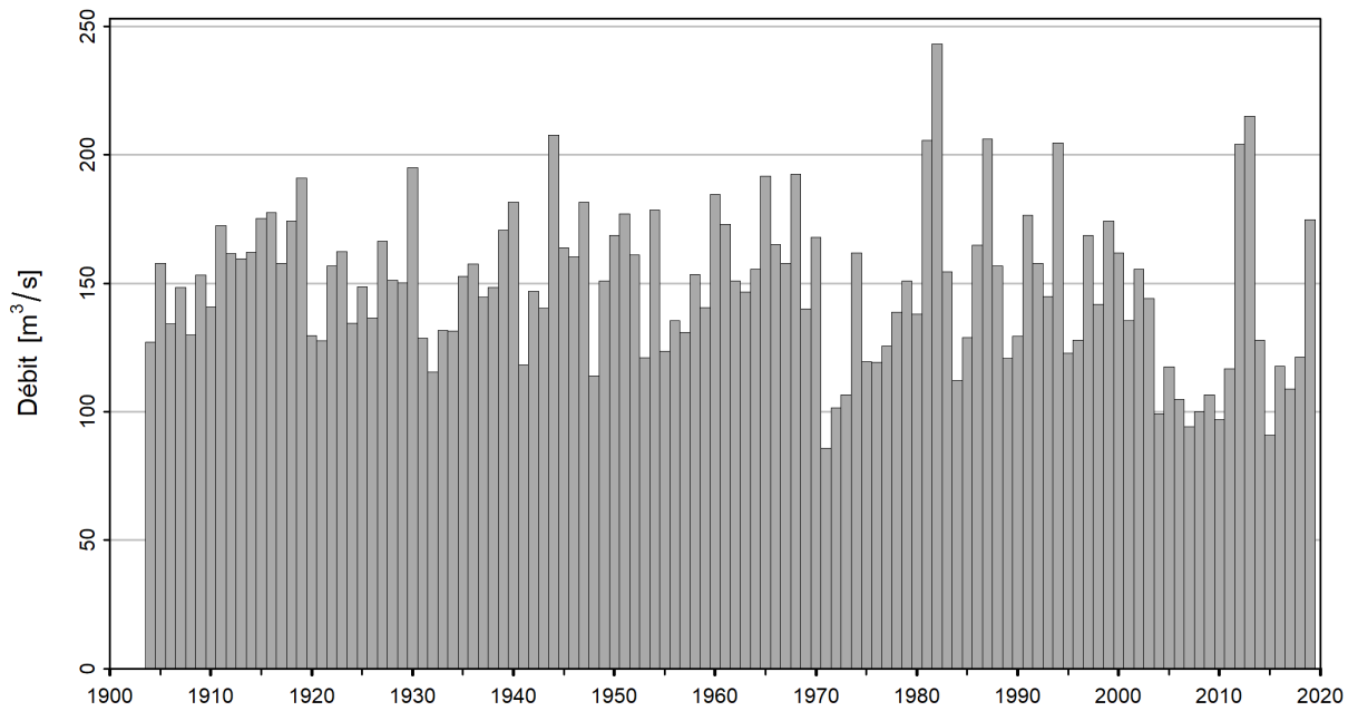
FIGURE 6 – Série temporelle de NM7Q [m 3 /s] (01.07.1904 - 30.06.2020)
