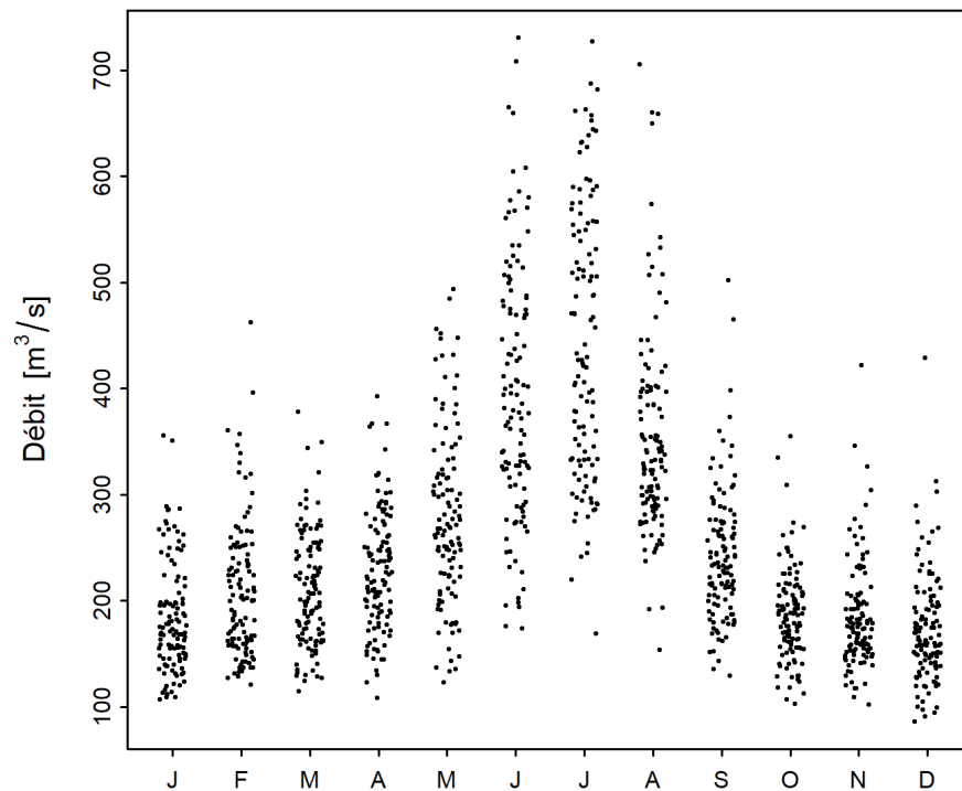
FIGURE 2 – Évolution saisonnière du minimum mensuel de M7Q [ \text{m}^3/\text{s} ] (01.07.1904 - 30.06.2020)
