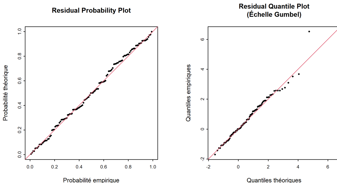
FIGURE 7 – Graphiques diagnostiques de la variante du modèle " sigl " de la méthode BLOCK (01.07.1904 - 30.06.2020)
