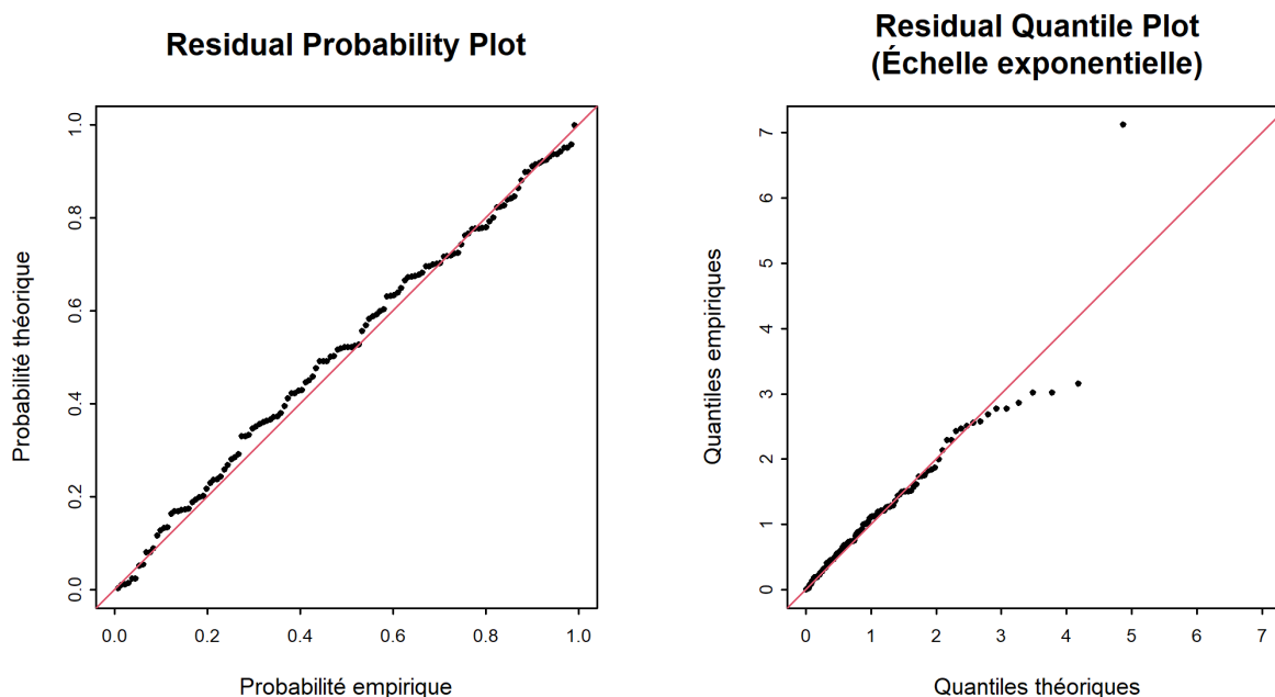
FIGURE 9 – Graphiques diagnostiques de la variante du modèle “ sigl ” de la méthode POT (01.07.1904 - 30.06.2020)
