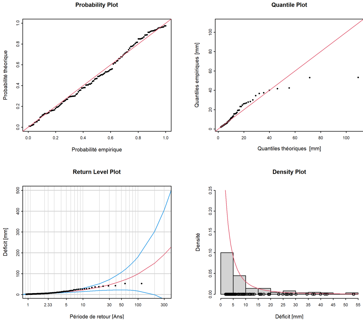
FIGURE 14 – Graphiques diagnostiques de la variante du modèle “ stat ” de la méthode POT (01.07.1904 - 30.06.2020)
