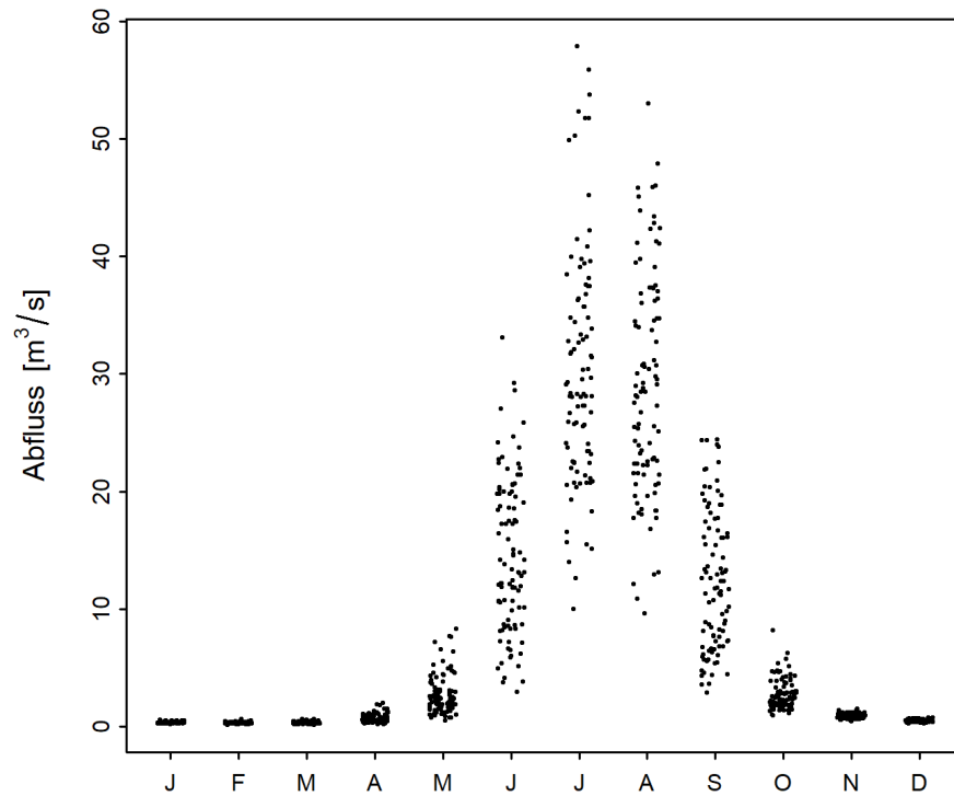
Abbildung 2: Saisonaler Verlauf der monatlichen Minima der M7Q [m³/s] (01.06.1922 - 31.05.2020)
