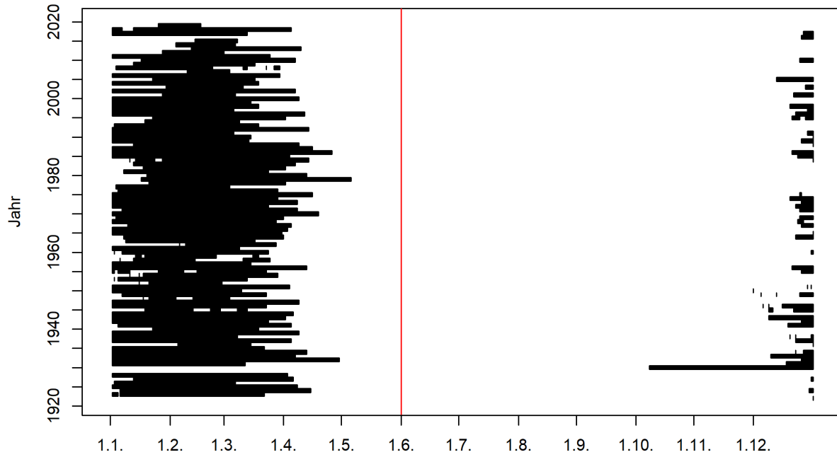
Abbildung 1: Zeitliches Auftreten der Niedrigwasserperioden im Jahresverlauf (01.06.1922 - 31.05.2020) und Startmonat des Niedrigwasserjahres (rote Linie) 1
