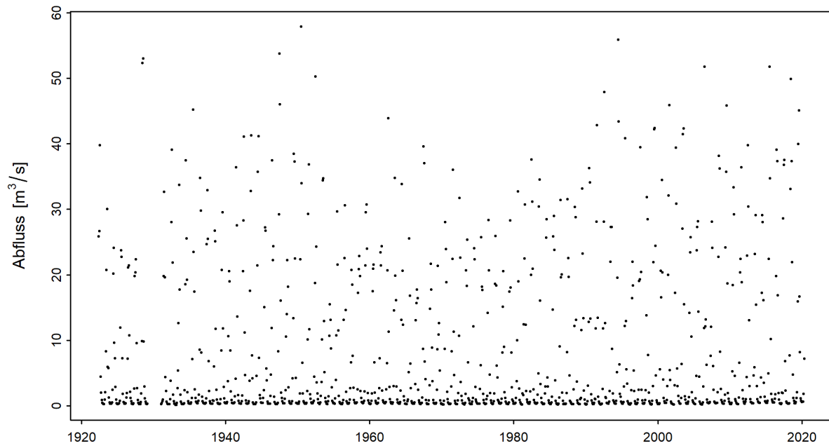
Abbildung 3: Zeitreihe der monatlichen Minima der M7Q [ \text{m}^3/\text{s} ] (01.06.1922 - 31.05.2020)
