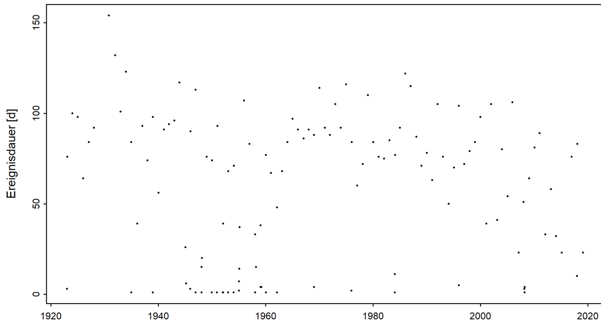
Abbildung 4: Zeitreihe der Niedrigwasserdauern [d] (01.06.1922 - 31.05.2020)
