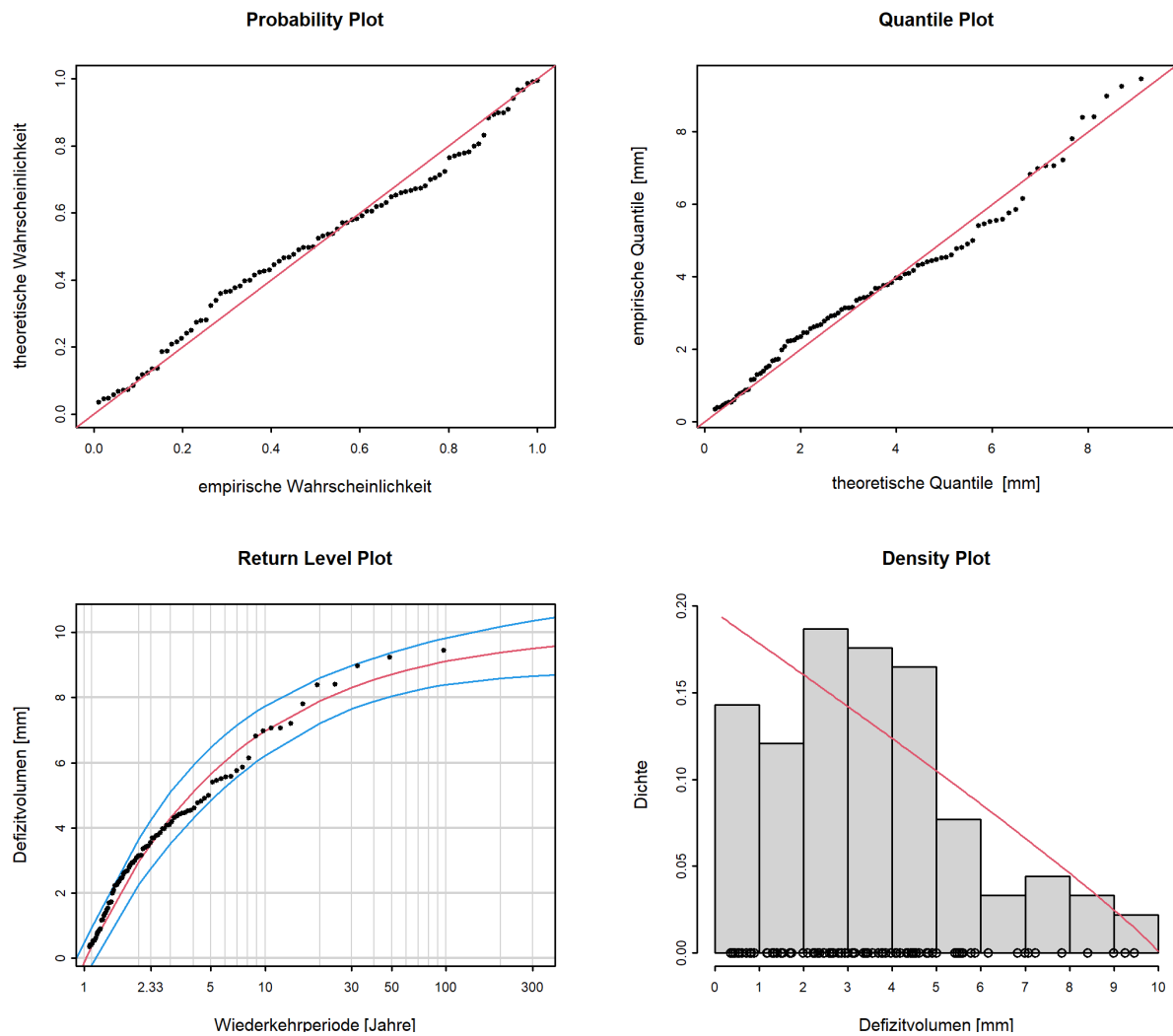
Abbildung 14: Diagnostikplots der Modellvariante "stat" des POT-Ansatzes (01.06.1922 - 31.05.2020)
