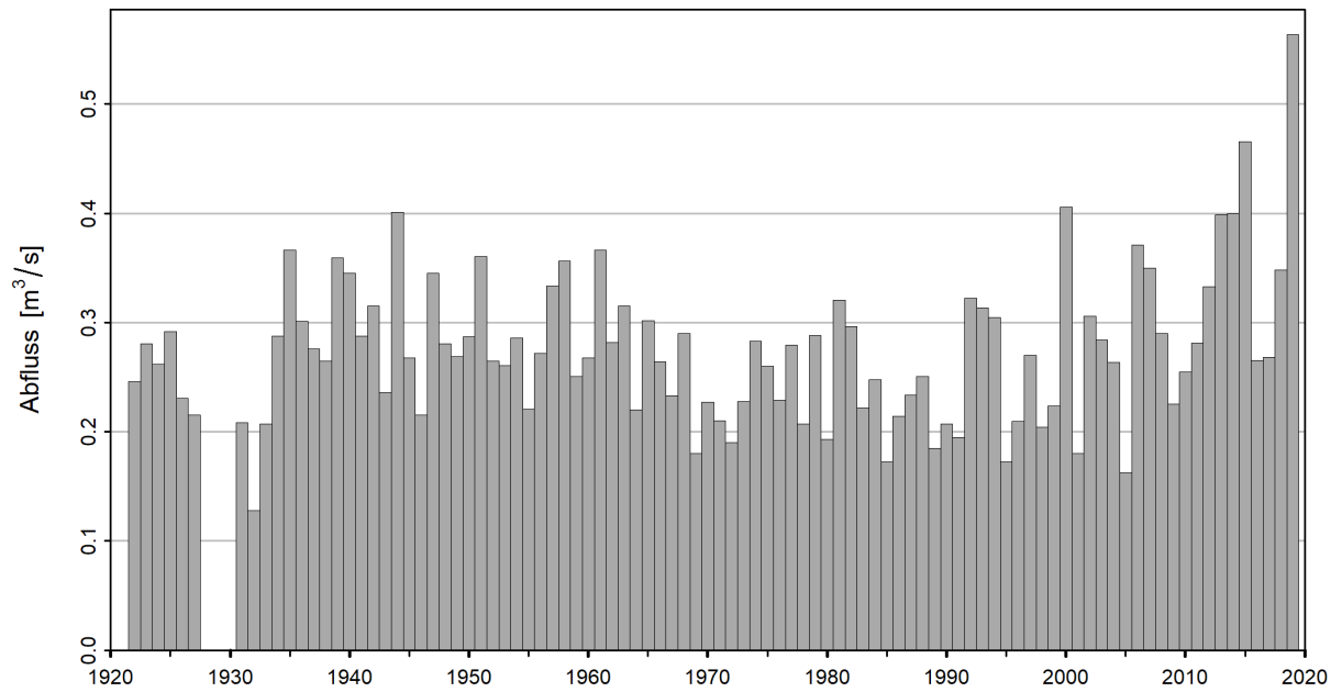
Abbildung 6: Zeitreihe der NM7Q [ \text{m}^3/\text{s} ] (01.06.1922 - 31.05.2020)
