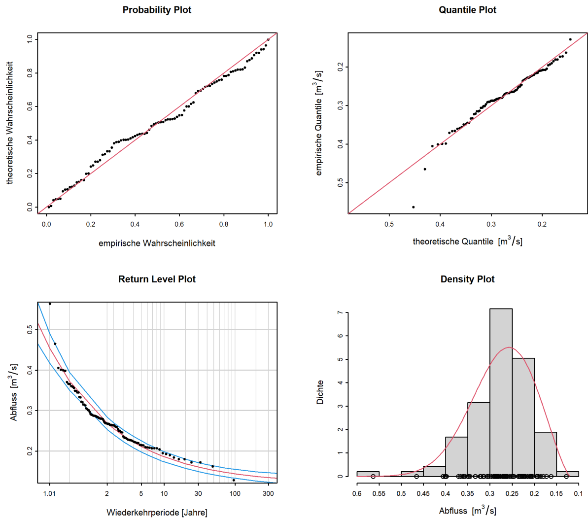
Abbildung 7: Diagnostikplots der Modellvariante “stat” des BLOCK-Ansatzes (01.06.1922 - 31.05.2020)
