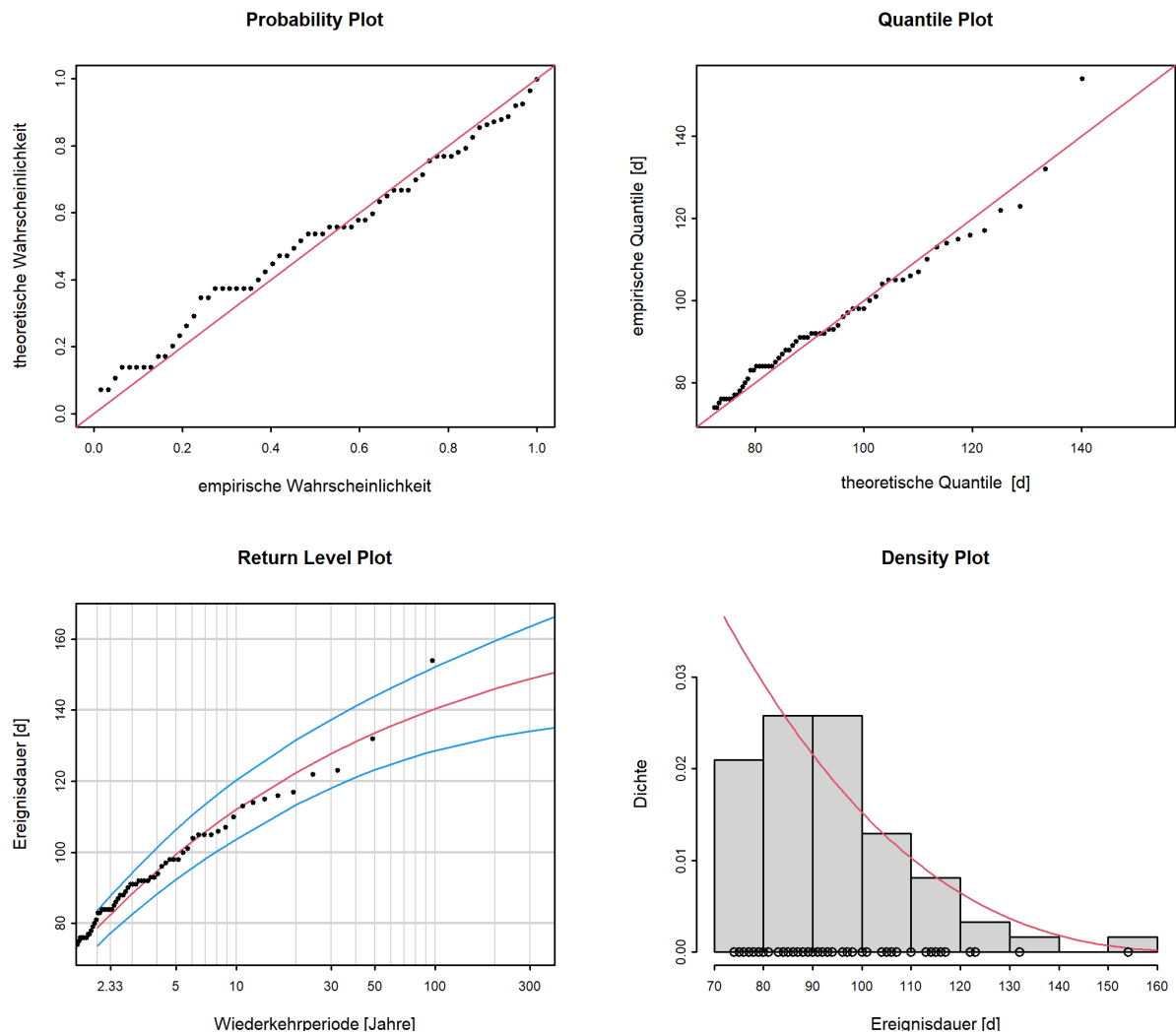
Abbildung 12: Diagnostikplots der Modellvariante “stat” des POT-Ansatzes (01.06.1922 - 31.05.2020)
