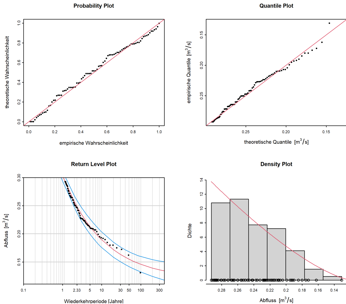
Abbildung 9: Diagnostikplots der Modellvariante “stat” des POT-Ansatzes (01.06.1922 - 31.05.2020)
