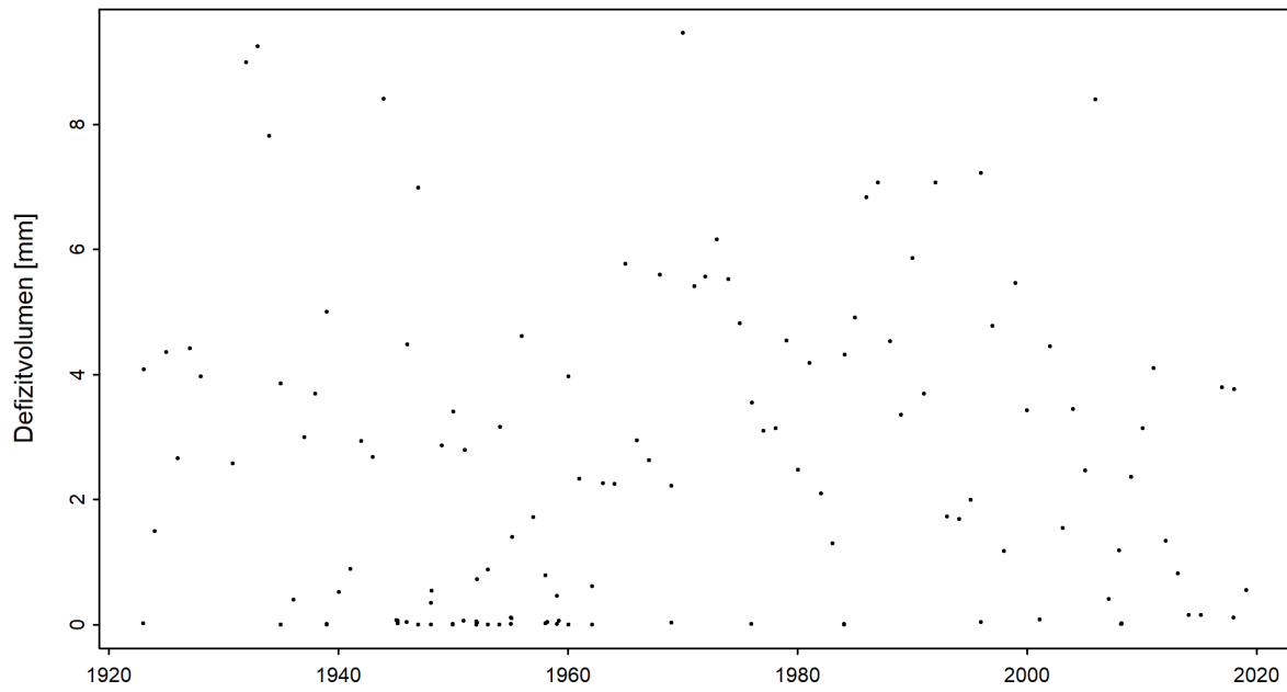
Abbildung 5: Zeitreihe der Defizitvolumen [mm] (01.06.1922 - 31.05.2020)
