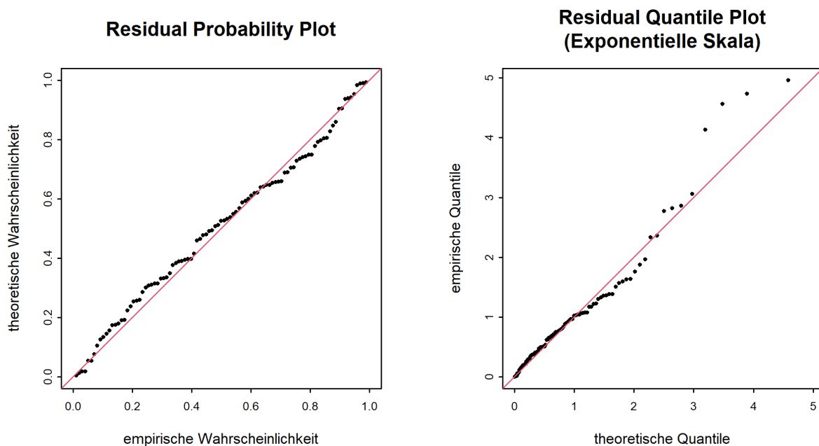
Abbildung 9: Diagnostikplots der Modellvariante “sigl” des POT-Ansatzes (01.06.1921 - 31.05.2020)
