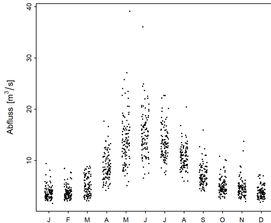
Abbildung 2: Saisonaler Verlauf der monatlichen Minima der M7Q [m³/s] (01.06.1921 - 31.05.2020)
