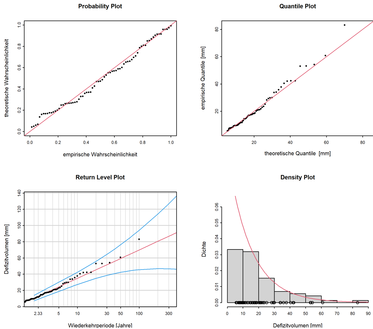
Abbildung 14: Diagnostikplots der Modellvariante “stat” des POT-Ansatzes (01.06.1921 - 31.05.2020)
