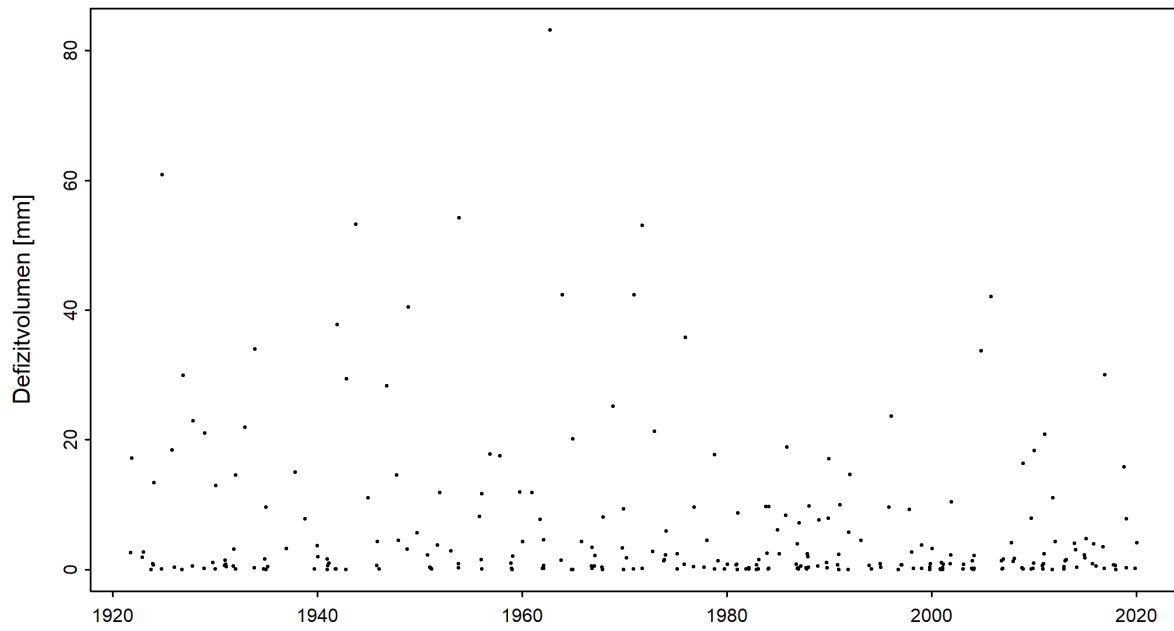
Abbildung 5: Zeitreihe der Defizitvolumen [mm] (01.06.1921 - 31.05.2020)
