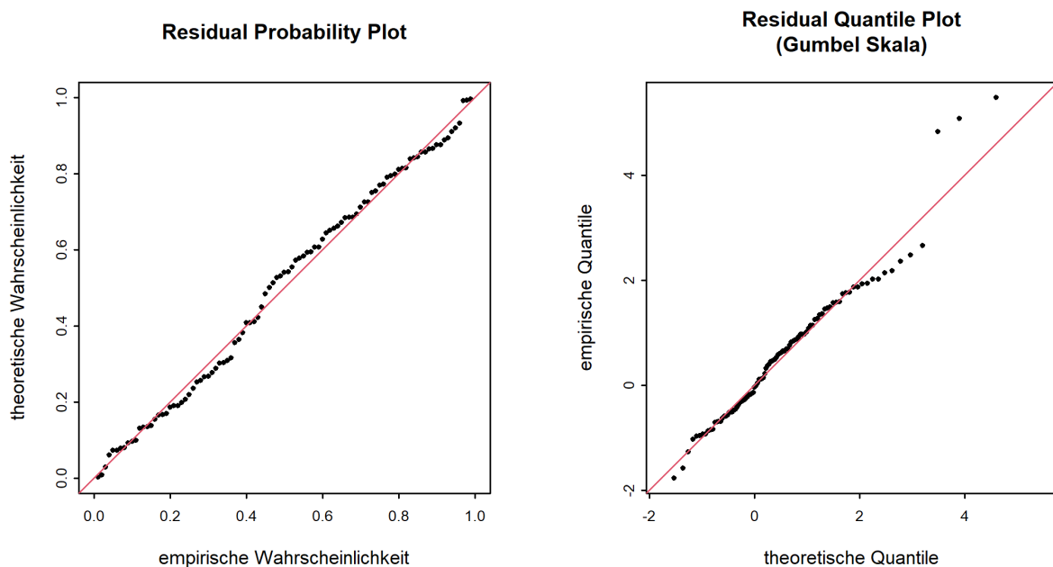
Abbildung 7: Diagnostikplots der Modellvariante “mul” des BLOCK-Ansatzes (01.06.1921 - 31.05.2020)
