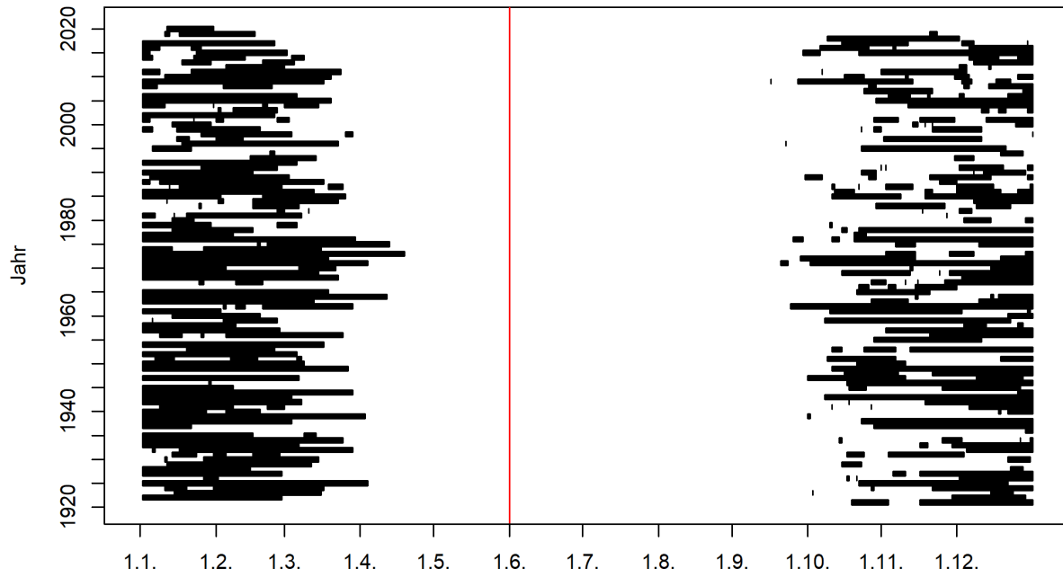
Abbildung 1: Zeitliches Auftreten der Niedrigwasserperioden im Jahresverlauf (01.06.1921 - 31.05.2020) und Startmonat des Niedrigwasserjahres (rote Linie) 1
