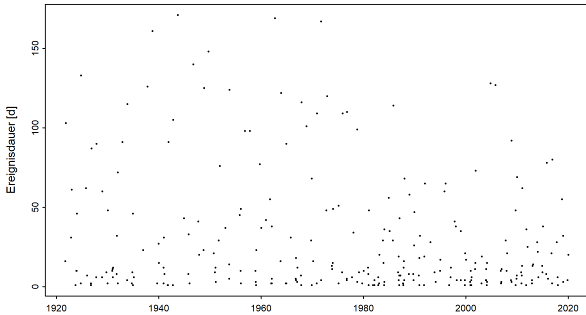
Abbildung 4: Zeitreihe der Niedrigwasserdauern [d] (01.06.1921 - 31.05.2020)
