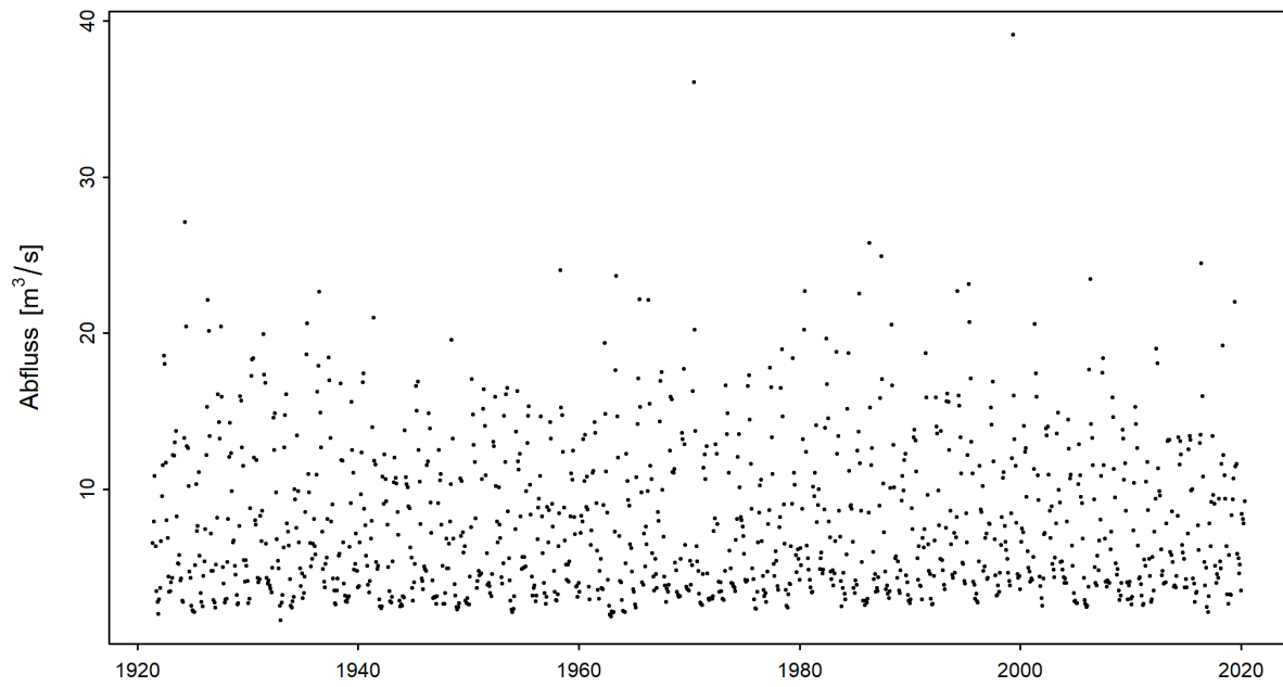
Abbildung 3: Zeitreihe der monatlichen Minima der M7Q [ \text{m}^3/\text{s} ] (01.06.1921 - 31.05.2020)
