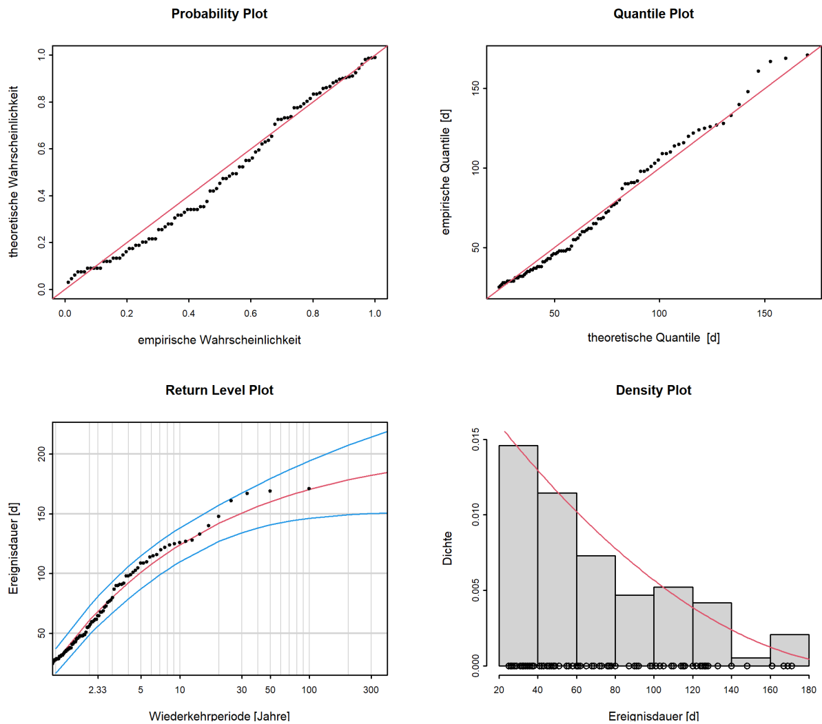
Abbildung 12: Diagnostikplots der Modellvariante "stat" des POT-Ansatzes (01.06.1921 - 31.05.2020)
