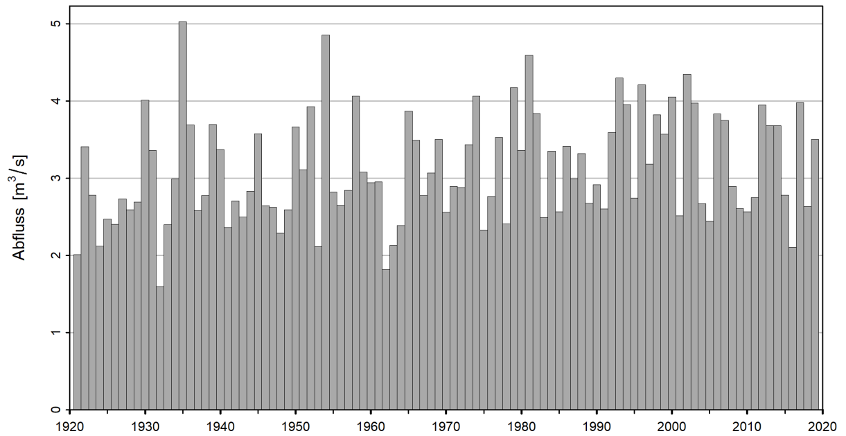
Abbildung 6: Zeitreihe der NM7Q [ \text{m}^3/\text{s} ] (01.06.1921 - 31.05.2020)
