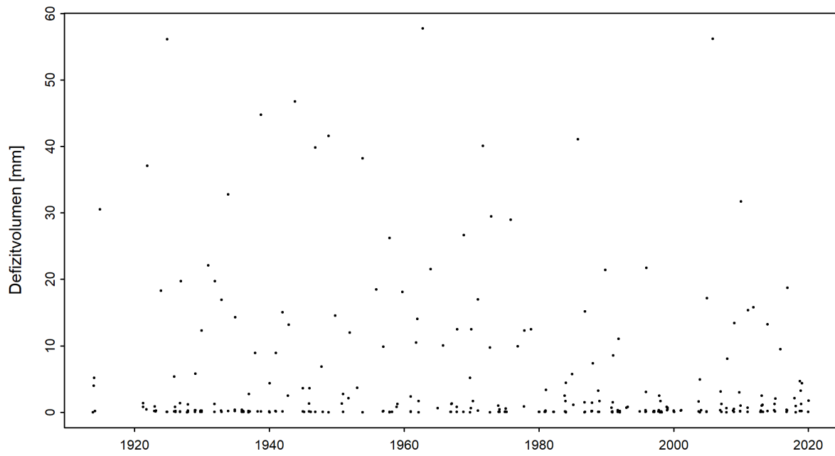
Abbildung 5: Zeitreihe der Defizitvolumen [mm] (01.06.1913 - 31.05.2020)
