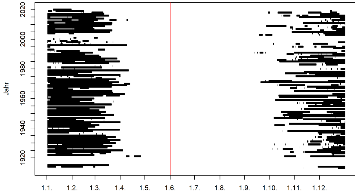
Abbildung 1: Zeitliches Auftreten der Niedrigwasserperioden im Jahresverlauf (01.06.1913 - 31.05.2020) und Startmonat des Niedrigwasserjahres (rote Linie) 1
