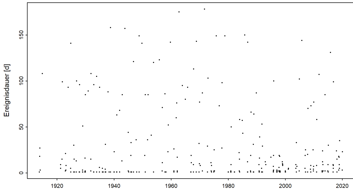
Abbildung 4: Zeitreihe der Niedrigwasserdauern [d] (01.06.1913 - 31.05.2020)
