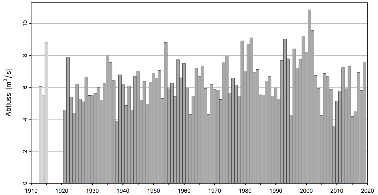
Abbildung 6: Zeitreihe der NM7Q [m³/s] (01.06.1913 - 31.05.2020), hellgrau: nicht verwendete NM7Q, dunkelgrau: verwendete NM7Q
