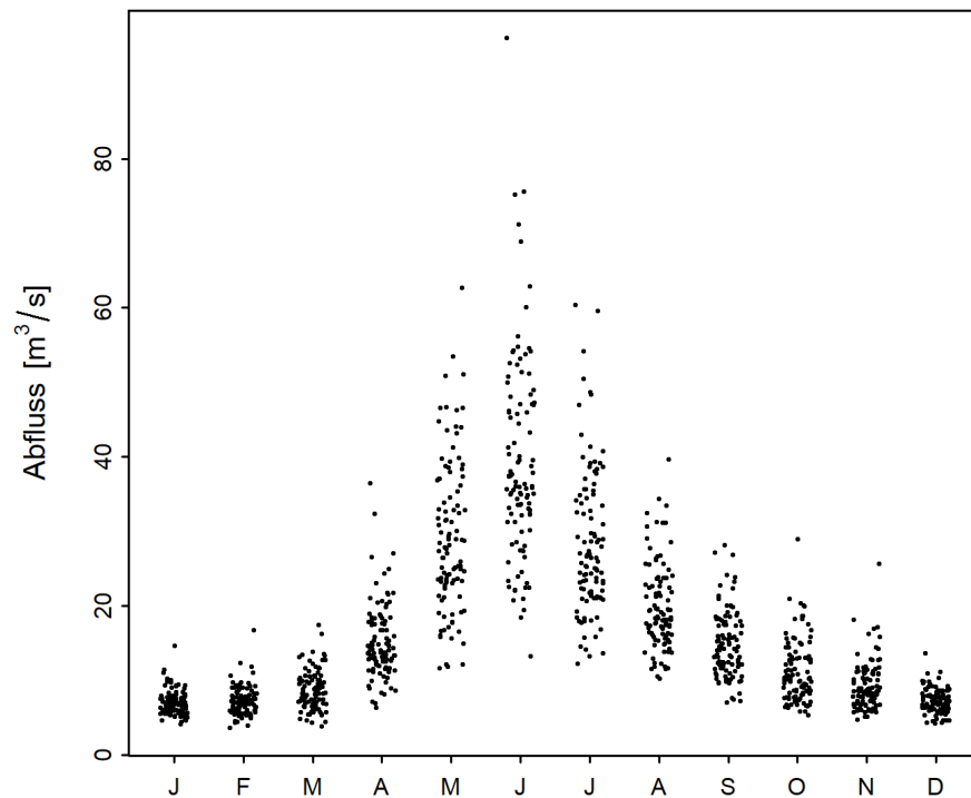
Abbildung 2: Saisonaler Verlauf der monatlichen Minima der M7Q [ \text{m}^3/\text{s} ] (01.06.1913 - 31.05.2020)
