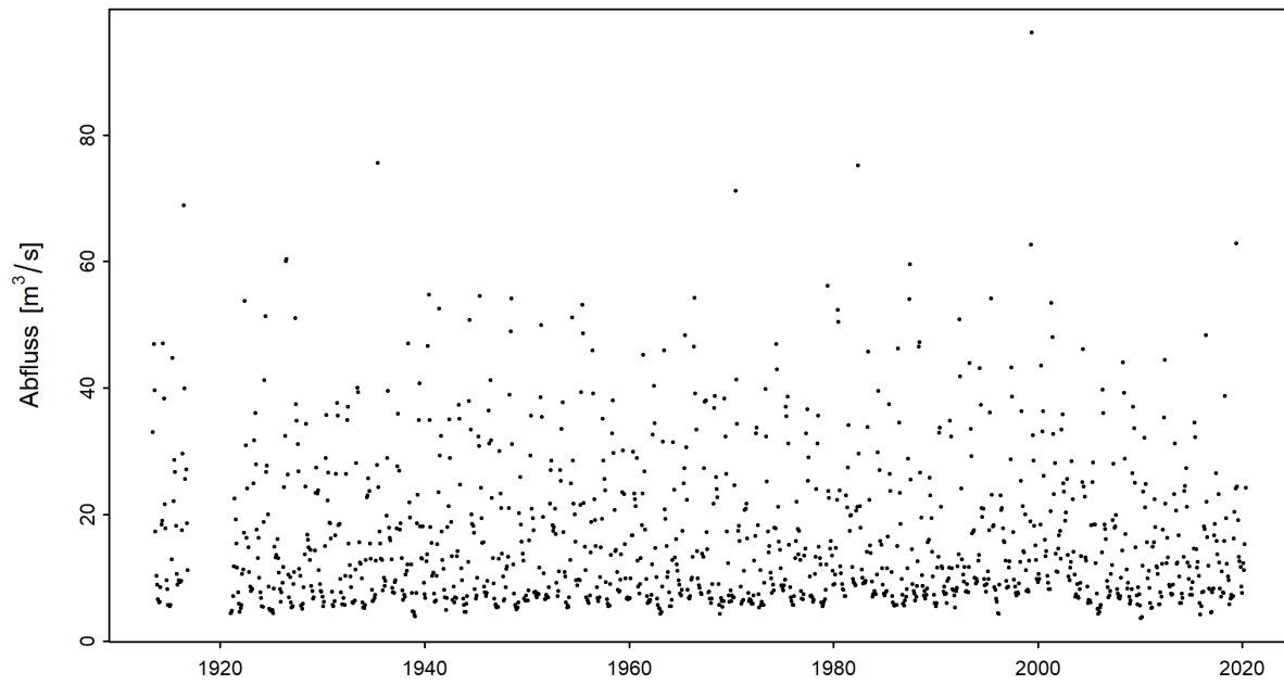
Abbildung 3: Zeitreihe der monatlichen Minima der M7Q [ \text{m}^3/\text{s} ] (01.06.1913 - 31.05.2020)
