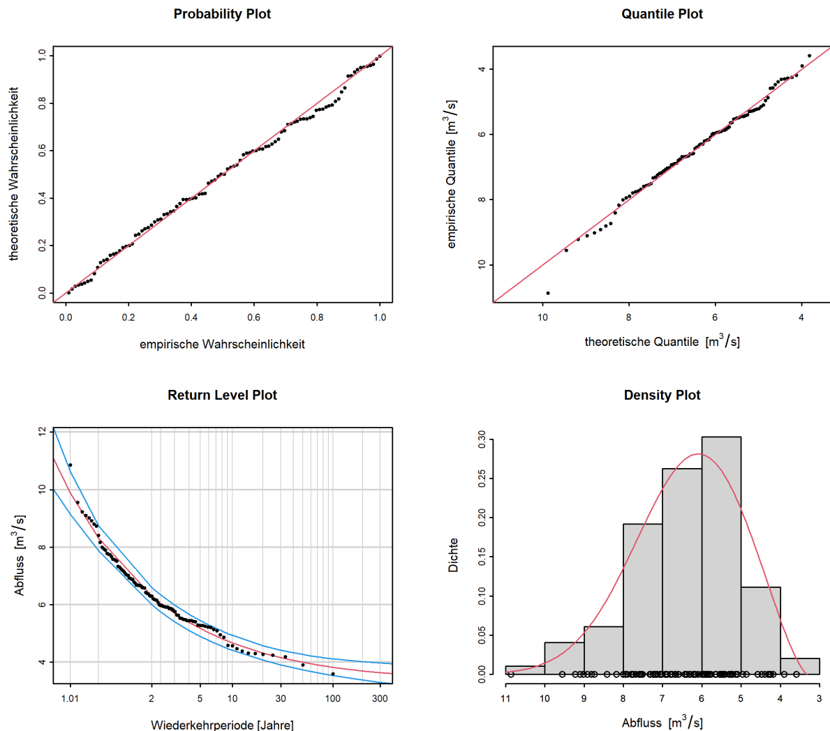
Abbildung 7: Diagnostikplots der Modellvariante “stat” des BLOCK-Ansatzes (01.06.1921 - 31.05.2020)
