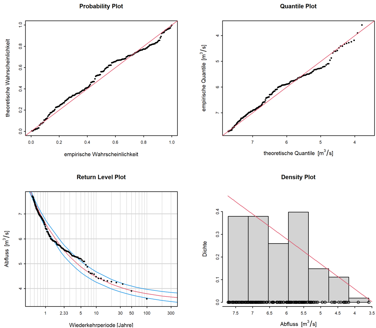
Abbildung 9: Diagnostikplots der Modellvariante “stat” des POT-Ansatzes (01.06.1921 - 31.05.2020)
