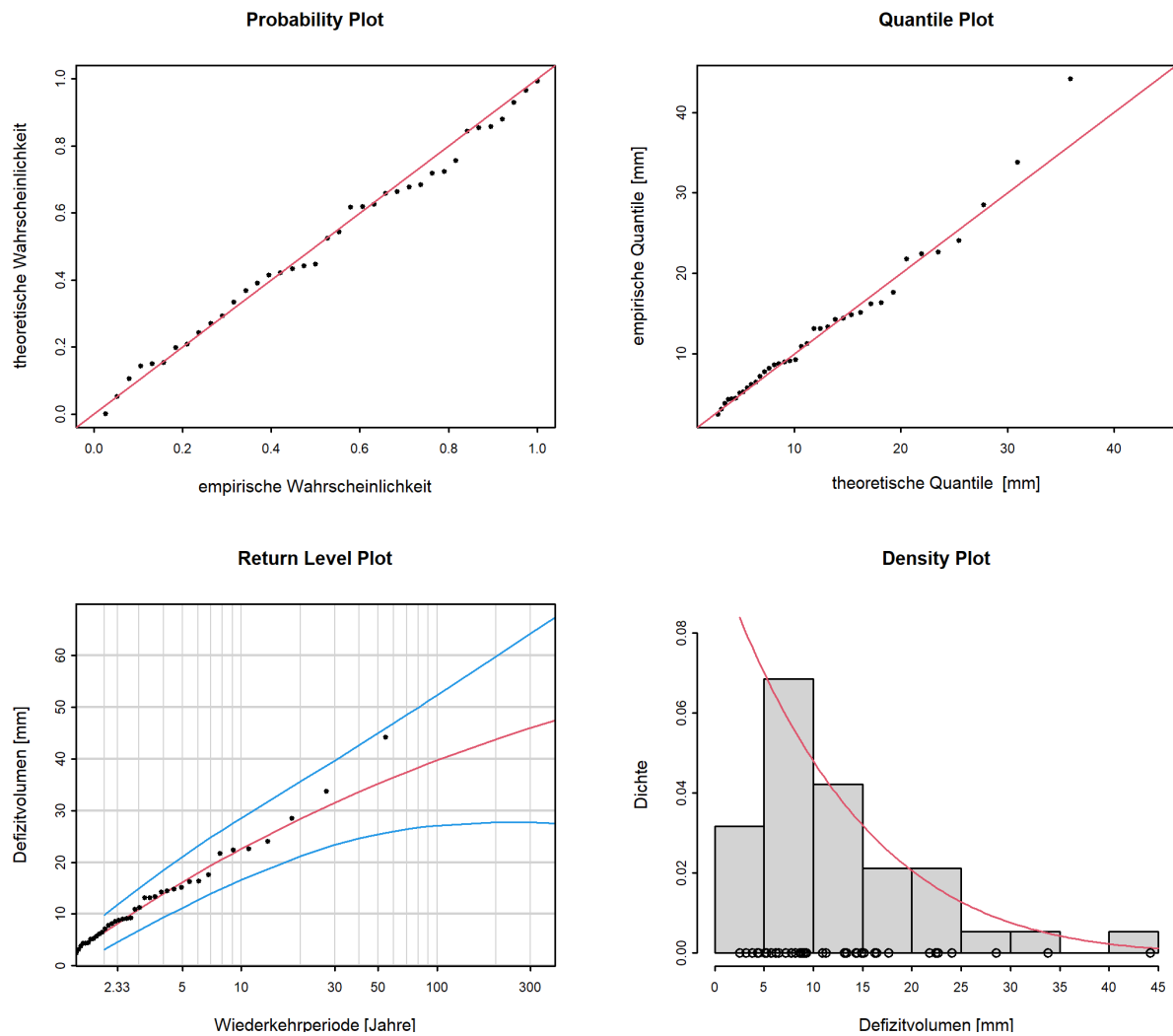
Abbildung 14: Diagnostikplots der Modellvariante “stat” des POT-Ansatzes (01.06.1966 - 31.05.2020)
