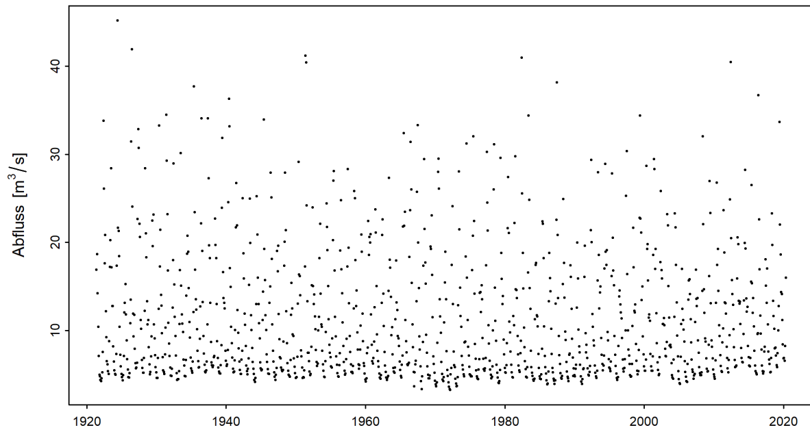
Abbildung 3: Zeitreihe der monatlichen Minima der M7Q [ \text{m}^3/\text{s} ] (01.06.1920 - 31.05.2020)
