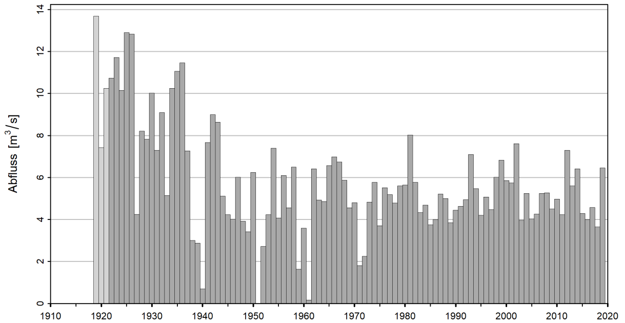
Abbildung 6: Zeitreihe der NM7Q [ \text{m}^3/\text{s} ] (01.06.1919 - 31.05.2020), hellgrau: nicht verwendete NM7Q, dunkelgrau: verwendete NM7Q
