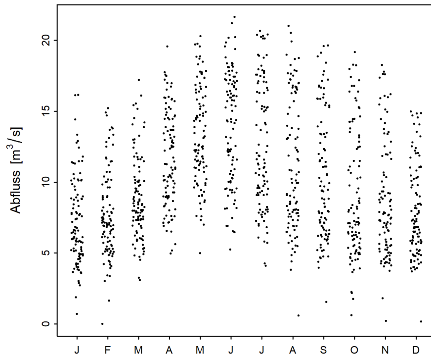
Abbildung 2: Saisonaler Verlauf der monatlichen Minima der M7Q [m 3 /s] (01.06.1919 - 31.05.2020)
