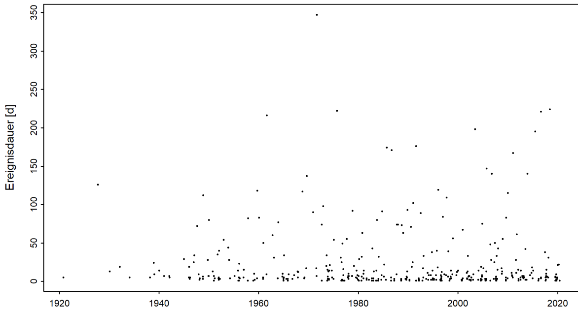
Abbildung 4: Zeitreihe der Niedrigwasserdauern [d] (01.06.1919 - 31.05.2020)
