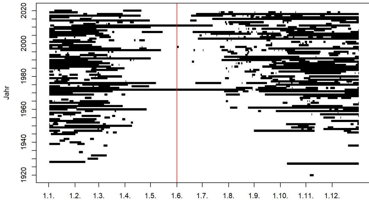
Abbildung 1: Zeitliches Auftreten der Niedrigwasserperioden im Jahresverlauf (01.06.1919 - 31.05.2020) und Startmonat des Niedrigwasserjahres (rote Linie) 1
