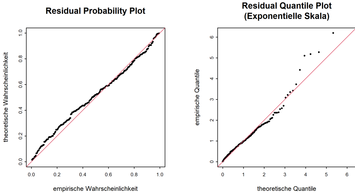
Abbildung 9: Diagnostikplots der Modellvariante “sigl” des POT-Ansatzes (01.06.1922 - 31.05.2020)
