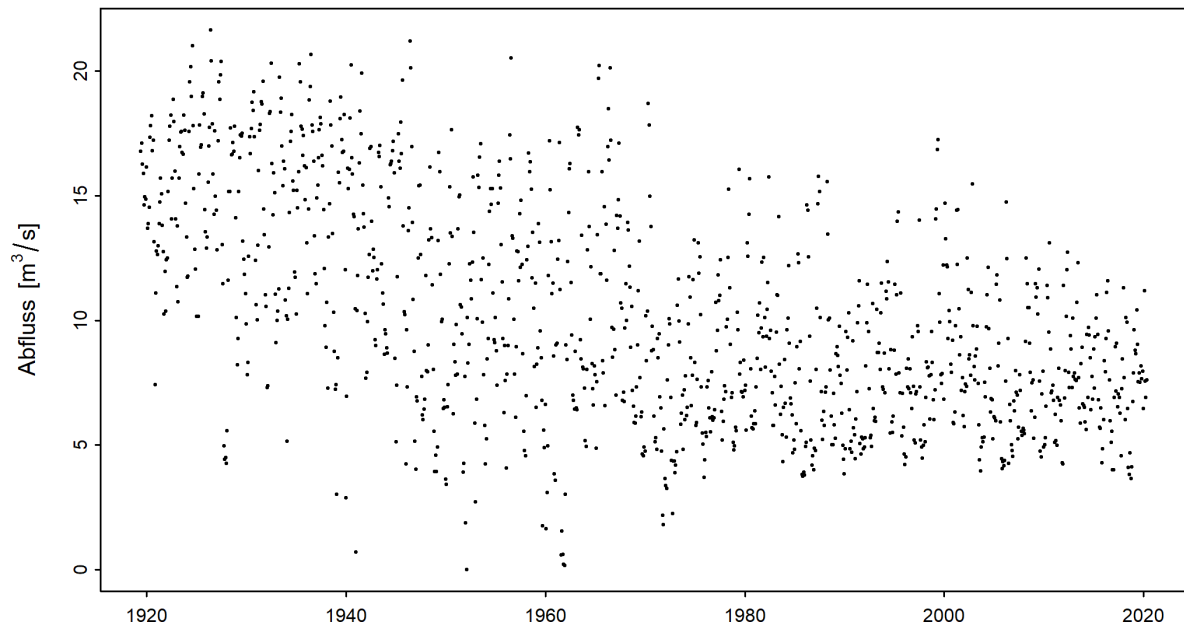
Abbildung 3: Zeitreihe der monatlichen Minima der M7Q [m³/s] (01.06.1919 - 31.05.2020)
