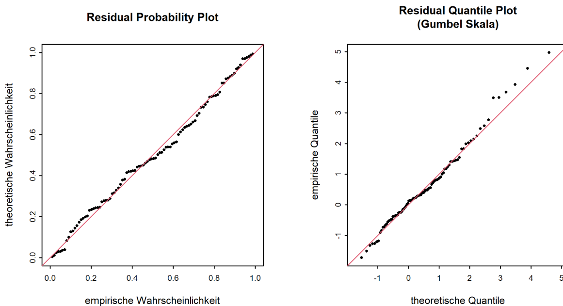
Abbildung 7: Diagnostikplots der Modellvariante "muq" des BLOCK-Ansatzes (01.06.1922 - 31.05.2020)
