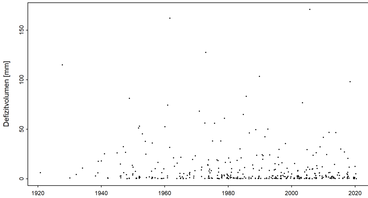
Abbildung 5: Zeitreihe der Defizitvolumen [mm] (01.06.1919 - 31.05.2020)
