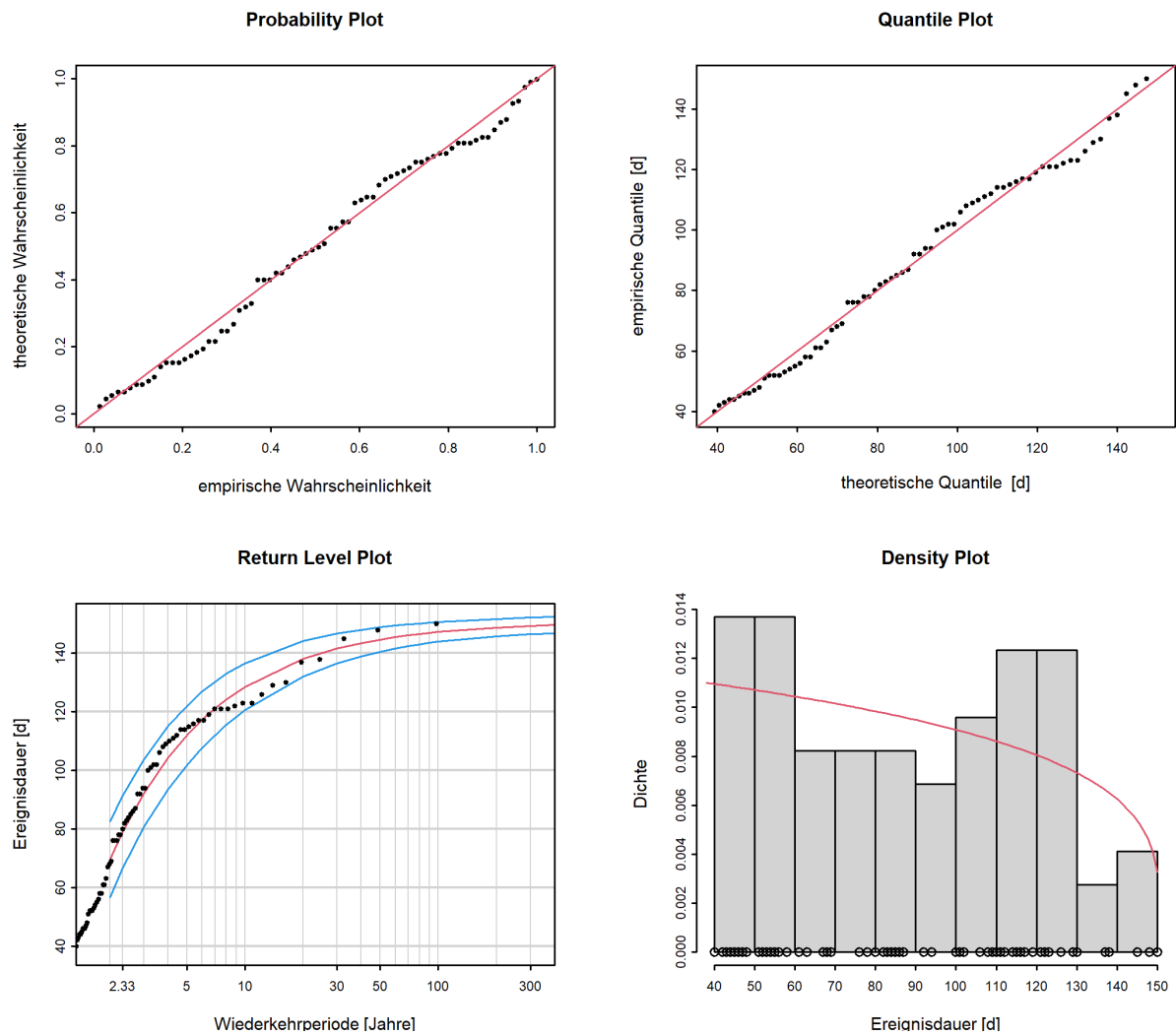
Abbildung 12: Diagnostikplots der Modellvariante “stat” des POT-Ansatzes (01.06.1923 - 31.05.2020)
