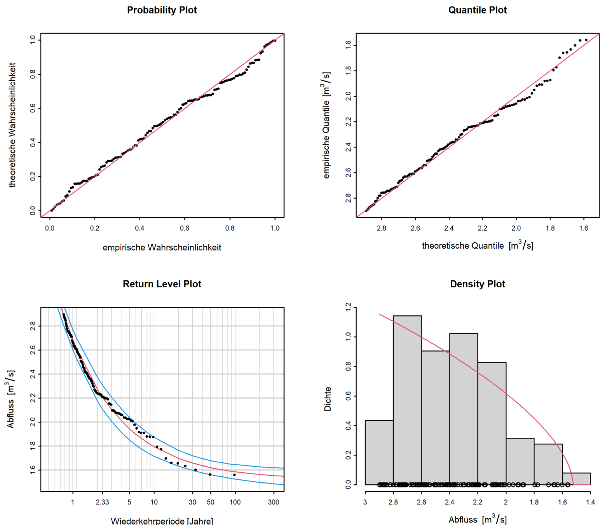
Abbildung 9: Diagnostikplots der Modellvariante “stat” des POT-Ansatzes (01.06.1923 - 31.05.2020)
