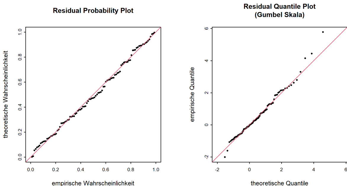
Abbildung 7: Diagnostikplots der Modellvariante "mujump1944" des BLOCK-Ansatzes (01.06.1923 - 31.05.2020)
