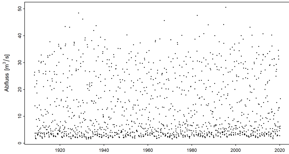
Abbildung 3: Zeitreihe der monatlichen Minima der M7Q [ \text{m}^3/\text{s} ] (01.06.1908 - 31.05.2020)
