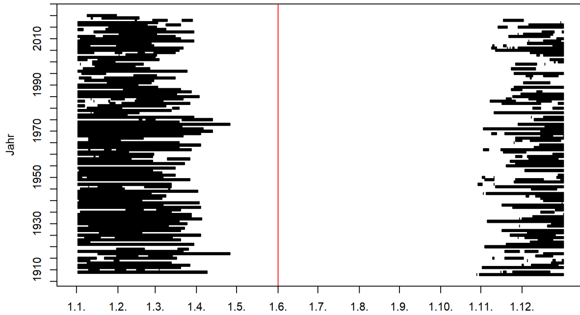
Abbildung 1: Zeitliches Auftreten der Niedrigwasserperioden im Jahresverlauf (01.06.1908 - 31.05.2020) und Startmonat des Niedrigwasserjahres (rote Linie) 1
