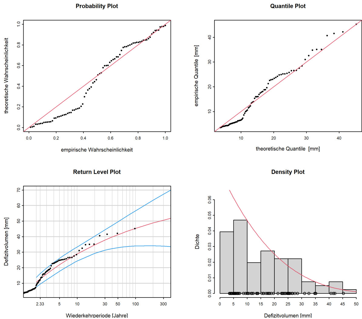
Abbildung 14: Diagnostikplots der Modellvariante “stat” des POT-Ansatzes (01.06.1923 - 31.05.2020)
