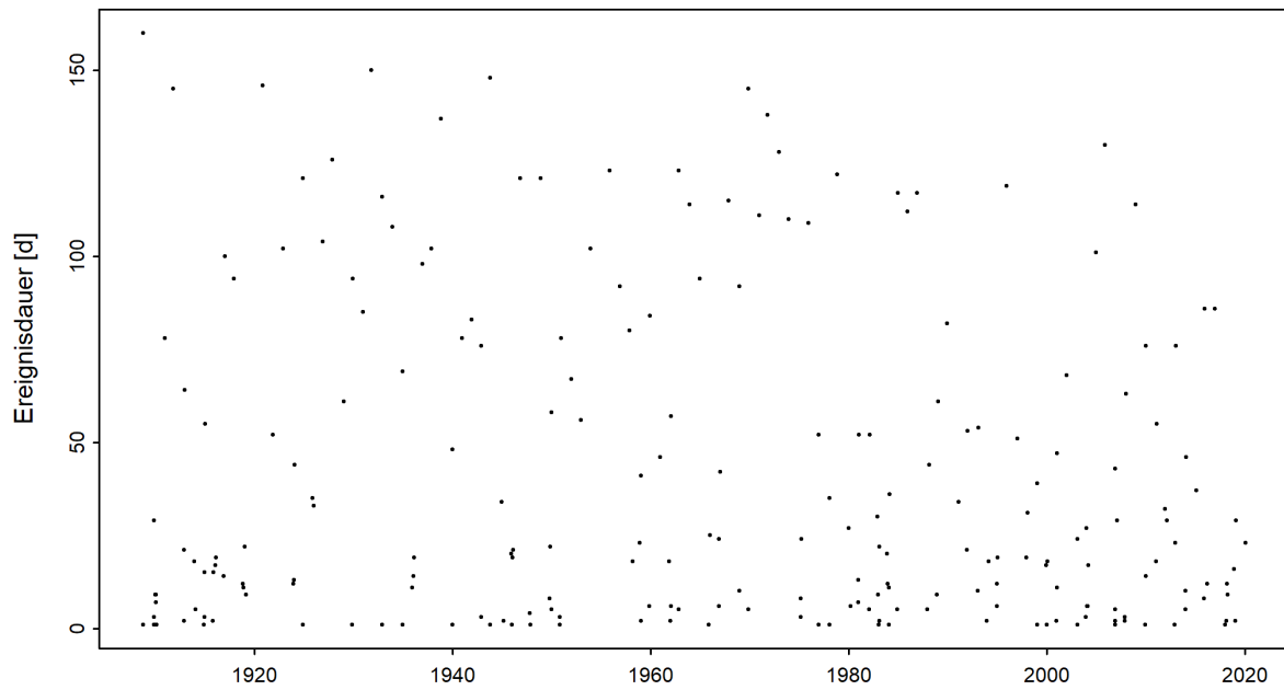
Abbildung 4: Zeitreihe der Niedrigwasserdauern [d] (01.06.1908 - 31.05.2020)
