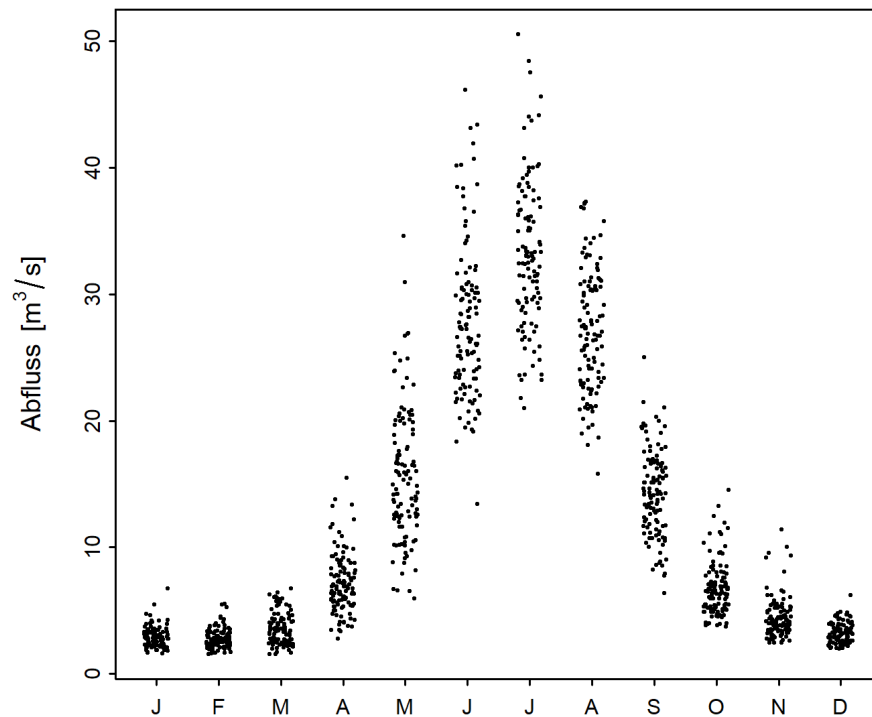
Abbildung 2: Saisonaler Verlauf der monatlichen Minima der M7Q [m³/s] (01.06.1908 - 31.05.2020)
