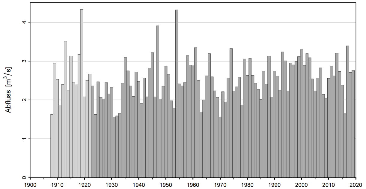
Abbildung 6: Zeitreihe der NM7Q [ \text{m}^3/\text{s} ] (01.06.1908 - 31.05.2020), hellgrau: nicht verwendete NM7Q, dunkelgrau: verwendete NM7Q
