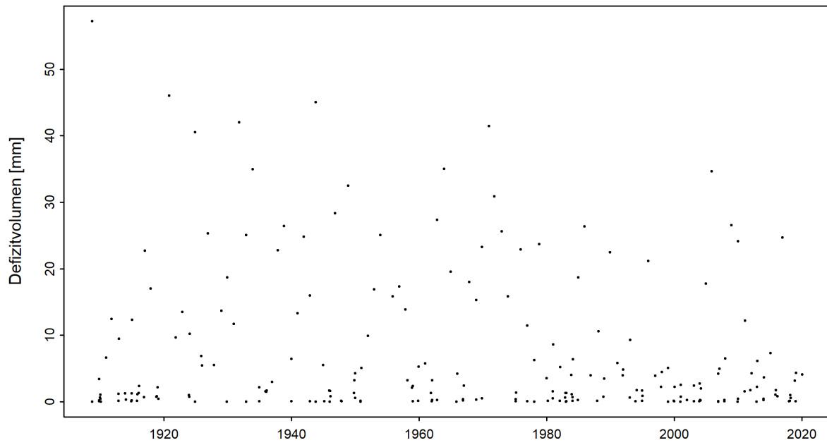
Abbildung 5: Zeitreihe der Defizitvolumen [mm] (01.06.1908 - 31.05.2020)
