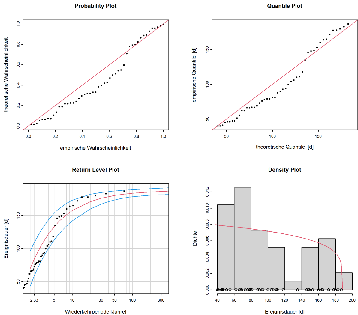
Abbildung 12: Diagnostikplots der Modellvariante “stat” des POT-Ansatzes (01.06.1948 - 31.05.2020)
