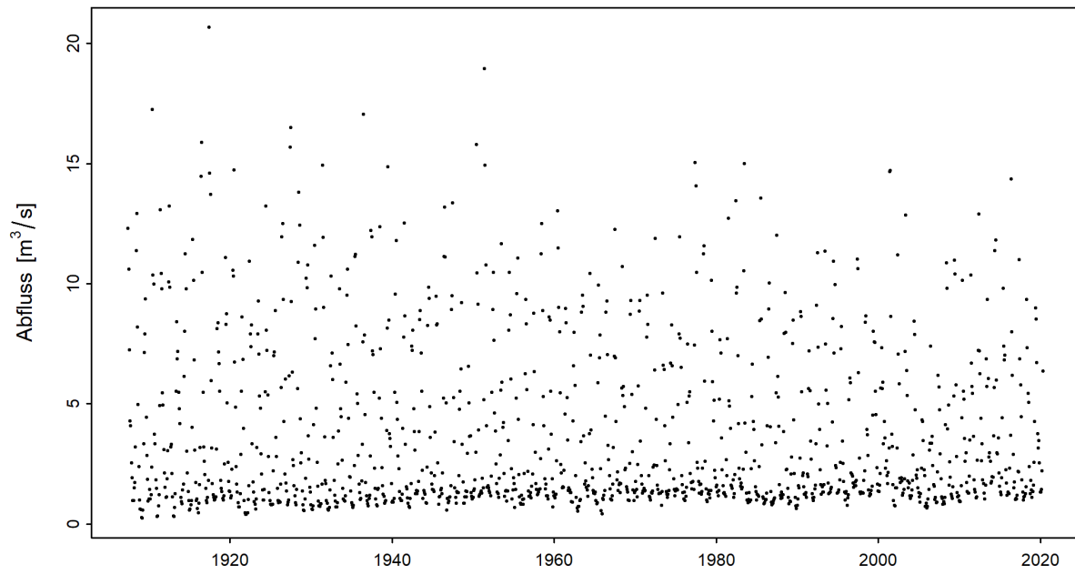
Abbildung 3: Zeitreihe der monatlichen Minima der M7Q [ \text{m}^3/\text{s} ] (01.06.1907 - 31.05.2020)
