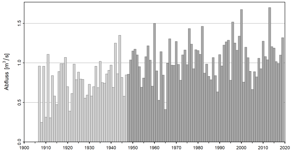
Abbildung 6: Zeitreihe der NM7Q [m³/s] (01.06.1907 - 31.05.2020), hellgrau: nicht verwendete NM7Q, dunkelgrau: verwendete NM7Q
