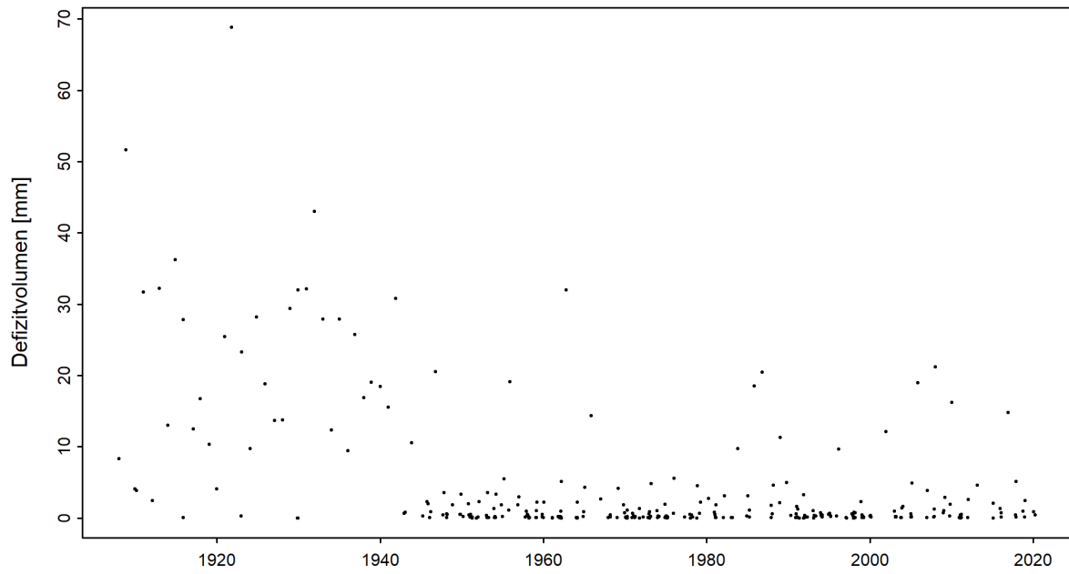
Abbildung 5: Zeitreihe der Defizitvolumen [mm] (01.06.1907 - 31.05.2020)
