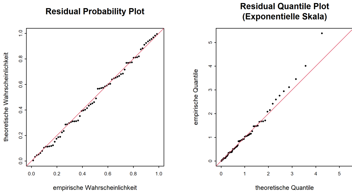
Abbildung 9: Diagnostikplots der Modellvariante “sigl” des POT-Ansatzes (01.06.1948 - 31.05.2020)
