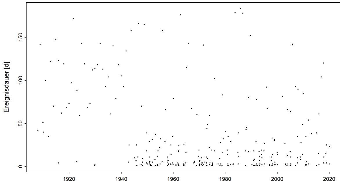
Abbildung 4: Zeitreihe der Niedrigwasserdauern [d] (01.06.1907 - 31.05.2020)
