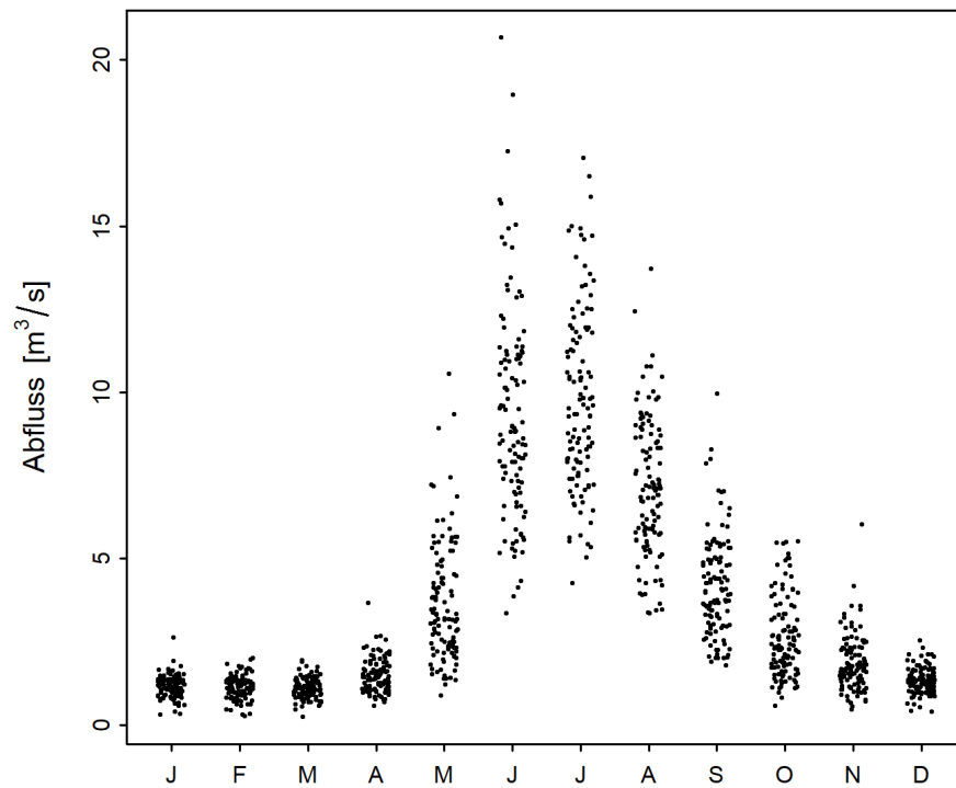
Abbildung 2: Saisonaler Verlauf der monatlichen Minima der M7Q [m³/s] (01.06.1907 - 31.05.2020)
