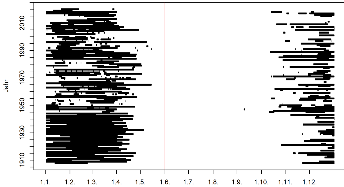
Abbildung 1: Zeitliches Auftreten der Niedrigwasserperioden im Jahresverlauf (01.06.1907 - 31.05.2020) und Startmonat des Niedrigwasserjahres (rote Linie) 1
