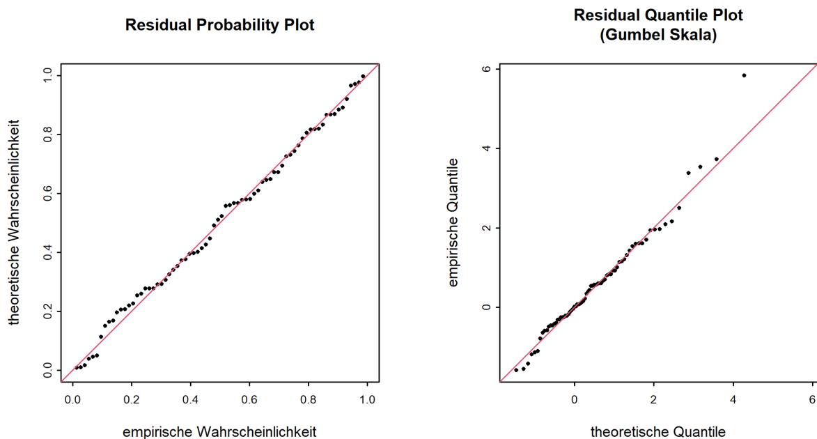
Abbildung 7: Diagnostikplots der Modellvariante “mul” des BLOCK-Ansatzes (01.06.1948 - 31.05.2020)
