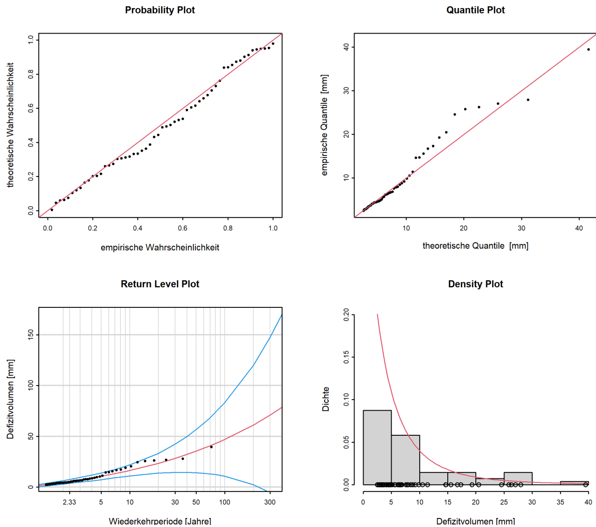
Abbildung 14: Diagnostikplots der Modellvariante “stat” des POT-Ansatzes (01.06.1948 - 31.05.2020)
