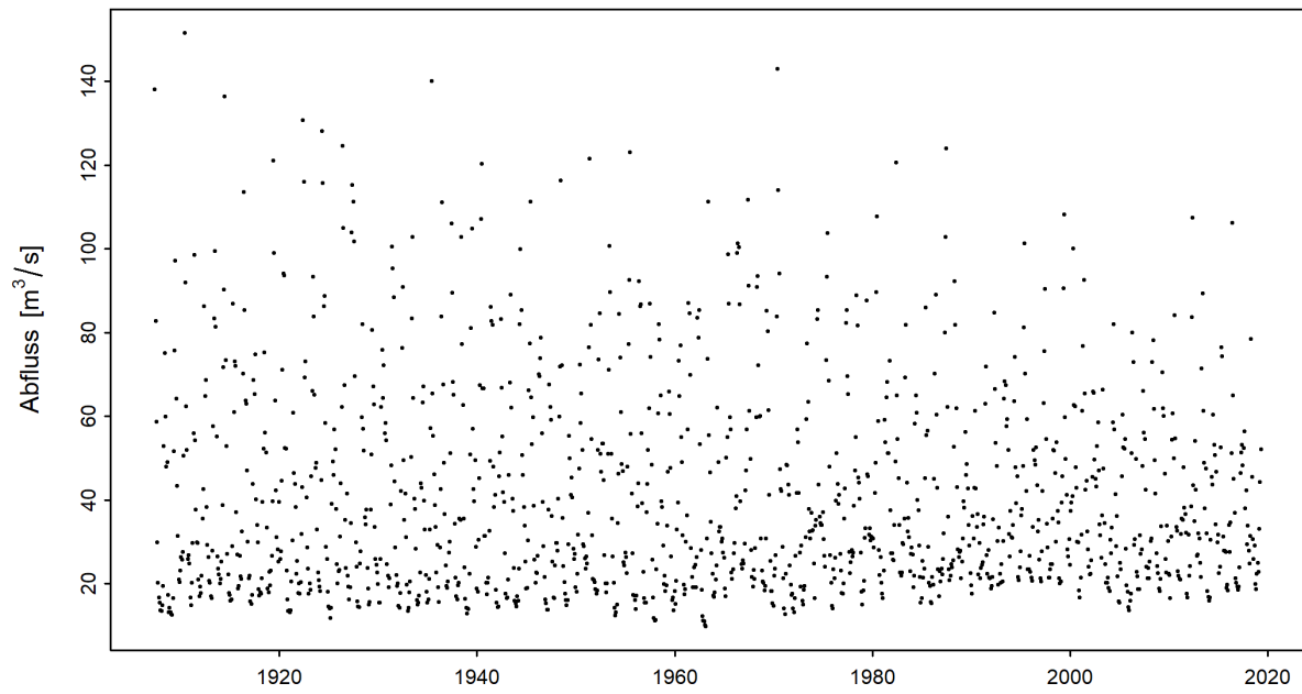
Abbildung 3: Zeitreihe der monatlichen Minima der M7Q [ \text{m}^3/\text{s} ] (01.06.1907 - 31.05.2019)
