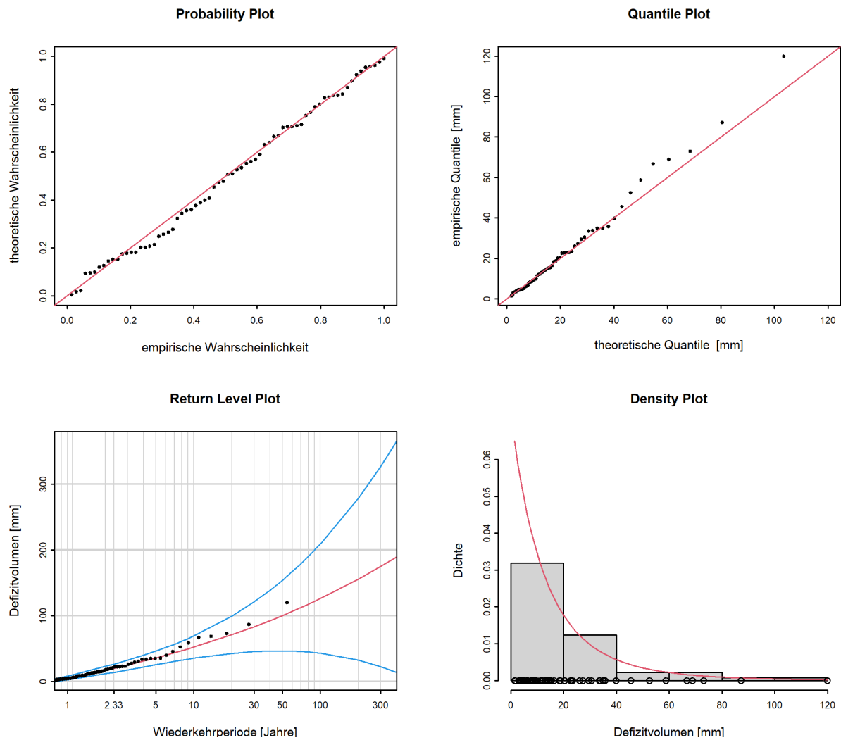
Abbildung 14: Diagnostikplots der Modellvariante “stat” des POT-Ansatzes (01.06.1965 - 31.05.2019)
