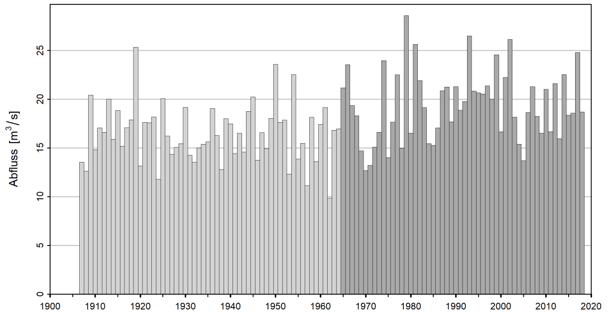
Abbildung 6: Zeitreihe der NM7Q [ \text{m}^3/\text{s} ] (01.06.1907 - 31.05.2019), hellgrau: nicht verwendete NM7Q, dunkelgrau: verwendete NM7Q
