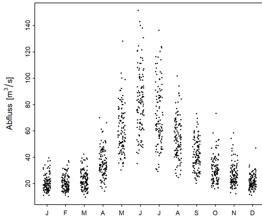
Abbildung 2: Saisonaler Verlauf der monatlichen Minima der M7Q [m³/s] (01.06.1907 - 31.05.2019)
