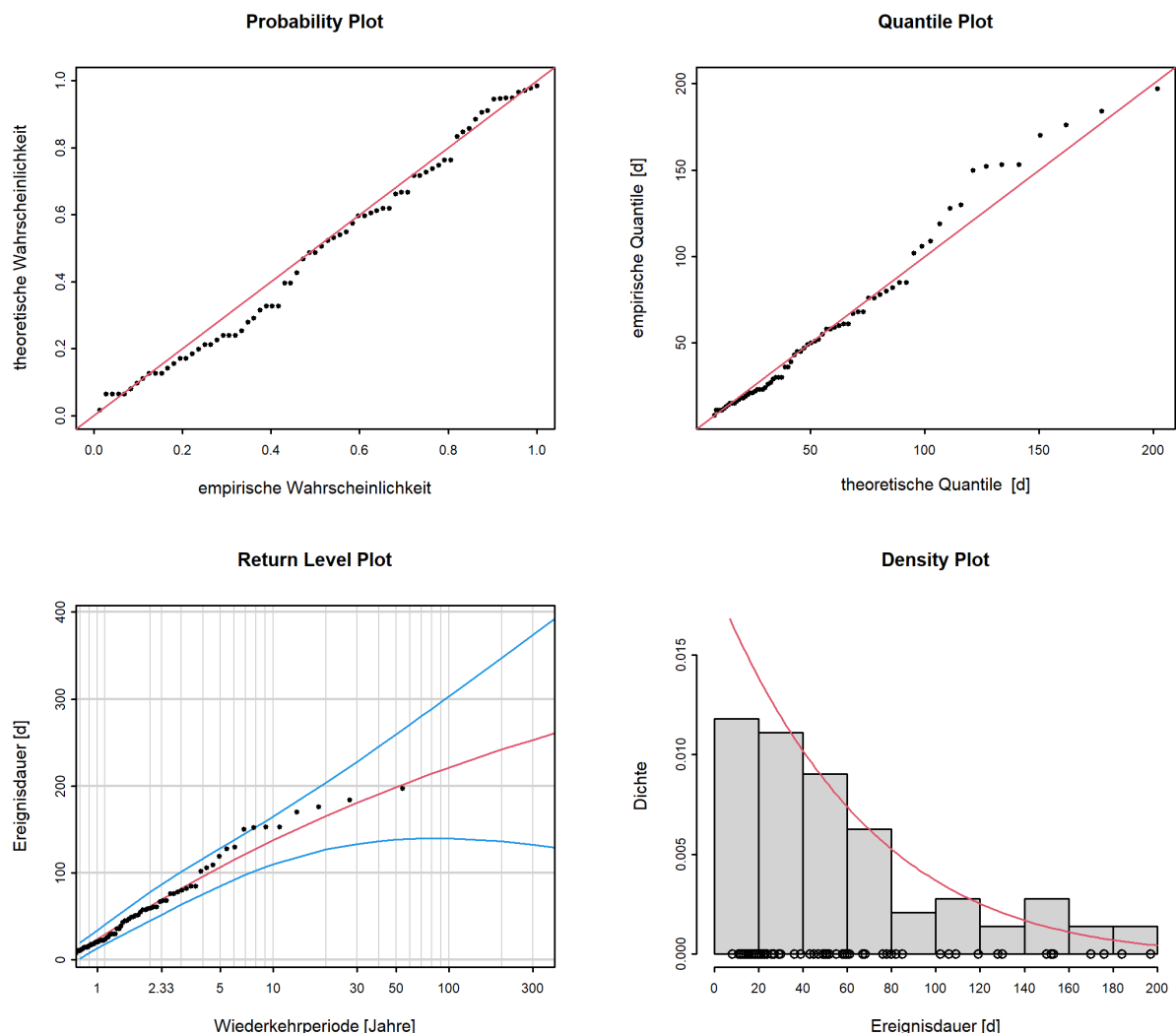
Abbildung 12: Diagnostikplots der Modellvariante “stat” des POT-Ansatzes (01.06.1965 - 31.05.2019)
