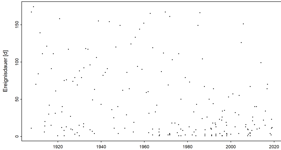
Abbildung 4: Zeitreihe der Niedrigwasserdauern [d] (01.06.1907 - 31.05.2019)
