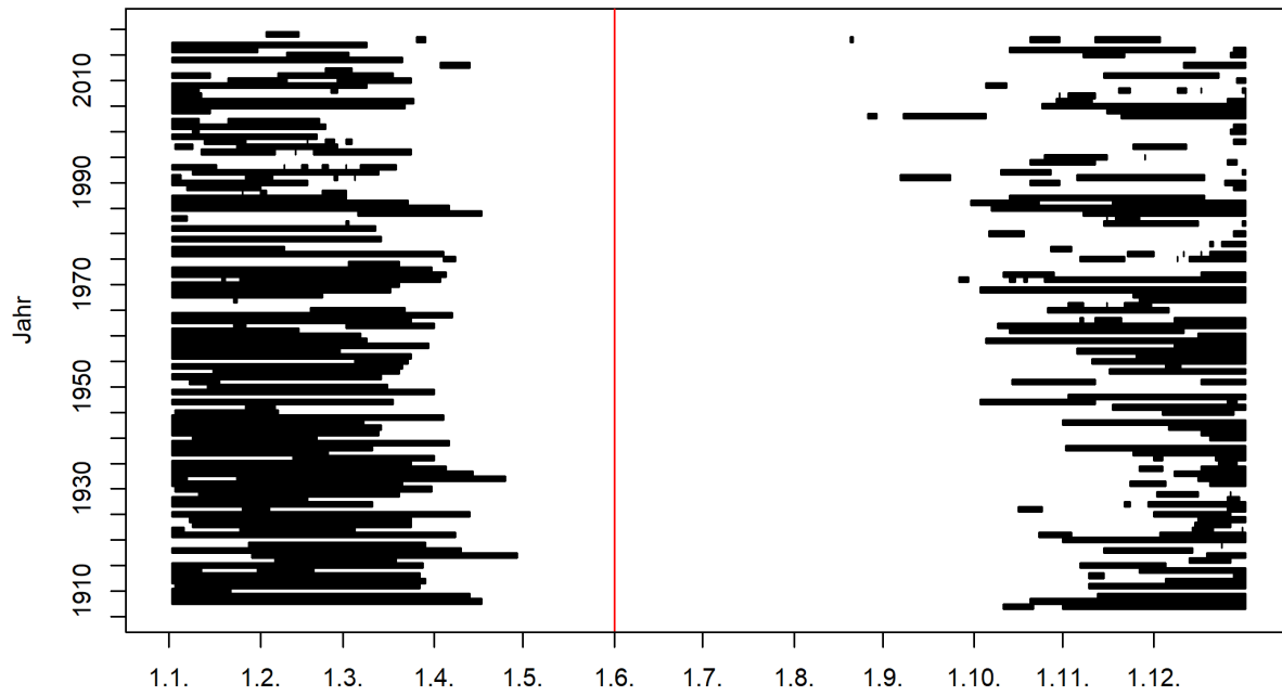
Abbildung 1: Zeitliches Auftreten der Niedrigwasserperioden im Jahresverlauf (01.06.1907 - 31.05.2019) und Startmonat des Niedrigwasserjahres (rote Linie) 1
