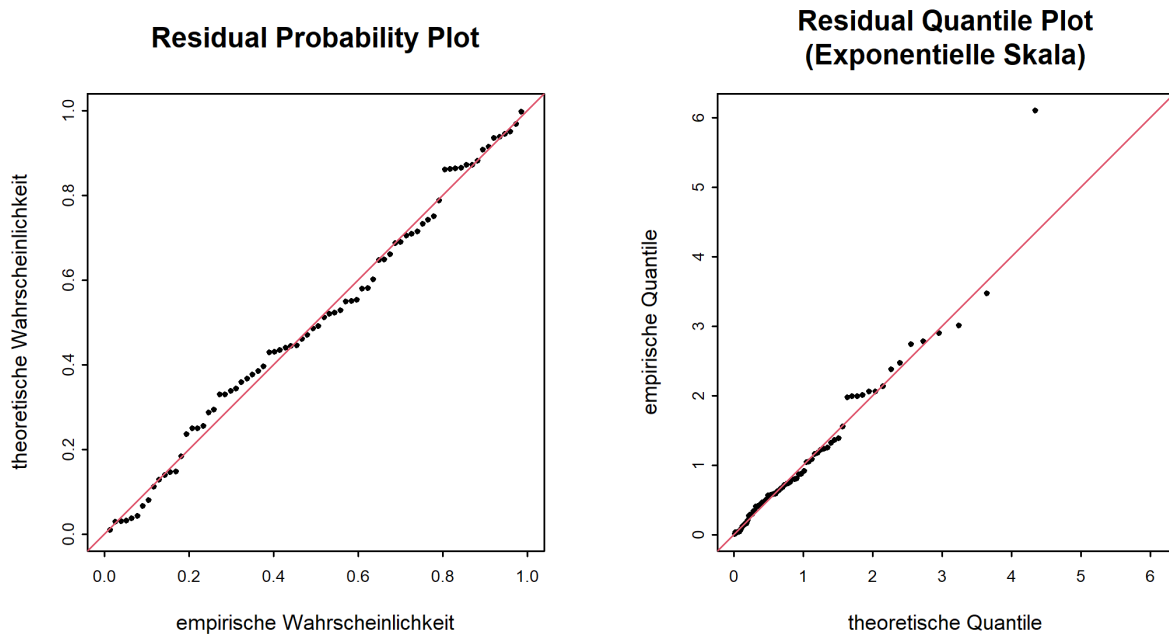
Abbildung 9: Diagnostikplots der Modellvariante “sigjump1979” des POT-Ansatzes (01.06.1965 - 31.05.2019)
