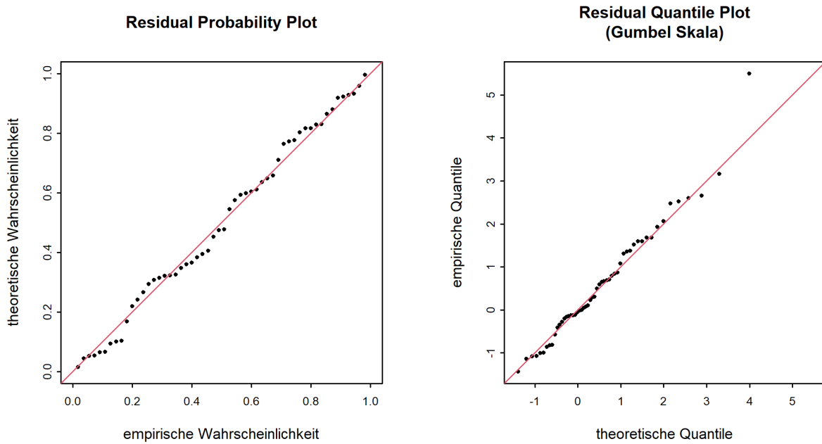
Abbildung 7: Diagnostikplots der Modellvariante "mujump1979" des BLOCK-Ansatzes (01.06.1965 - 31.05.2019)
