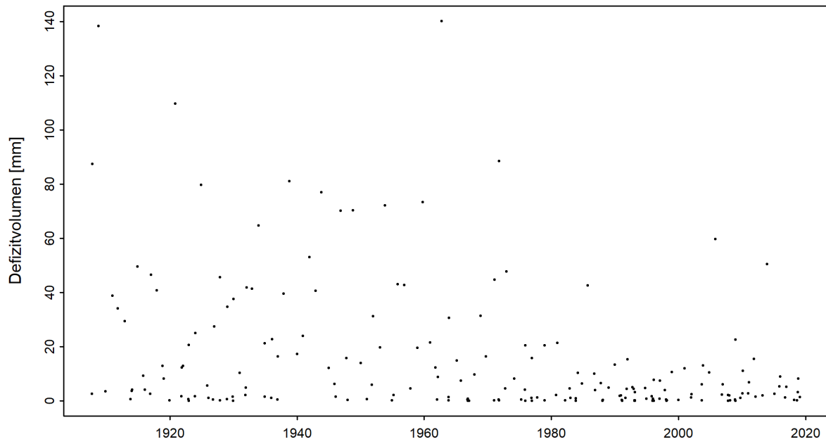
Abbildung 5: Zeitreihe der Defizitvolumen [mm] (01.06.1907 - 31.05.2019)
