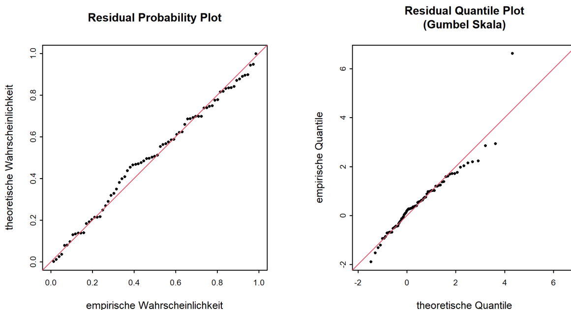
Abbildung 7: Diagnostikplots der Modellvariante “mujump1994” des BLOCK-Ansatzes (01.06.1945 - 31.05.2020)
