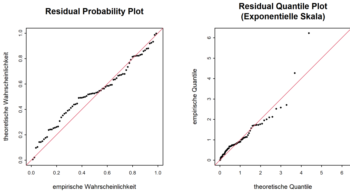
Abbildung 9: Diagnostikplots der Modellvariante "sigjump1994" des POT-Ansatzes (01.06.1945 - 31.05.2020)
