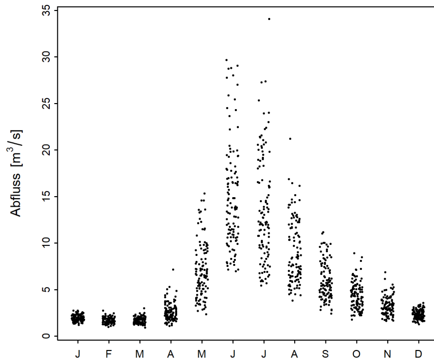
Abbildung 2: Saisonaler Verlauf der monatlichen Minima der M7Q [m³/s] (01.06.1910 - 31.05.2020)
