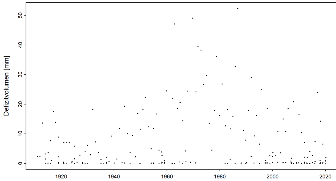
Abbildung 5: Zeitreihe der Defizitvolumen [mm] (01.06.1910 - 31.05.2020)
