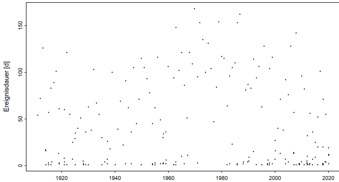
Abbildung 4: Zeitreihe der Niedrigwasserdauern [d] (01.06.1910 - 31.05.2020)
