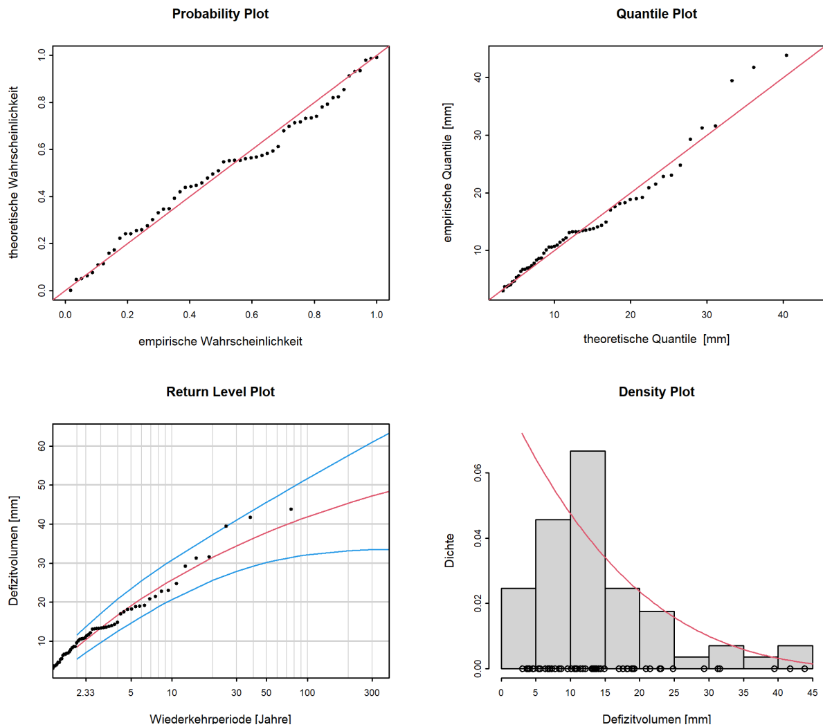
Abbildung 14: Diagnostikplots der Modellvariante “stat” des POT-Ansatzes (01.06.1945 - 31.05.2020)
