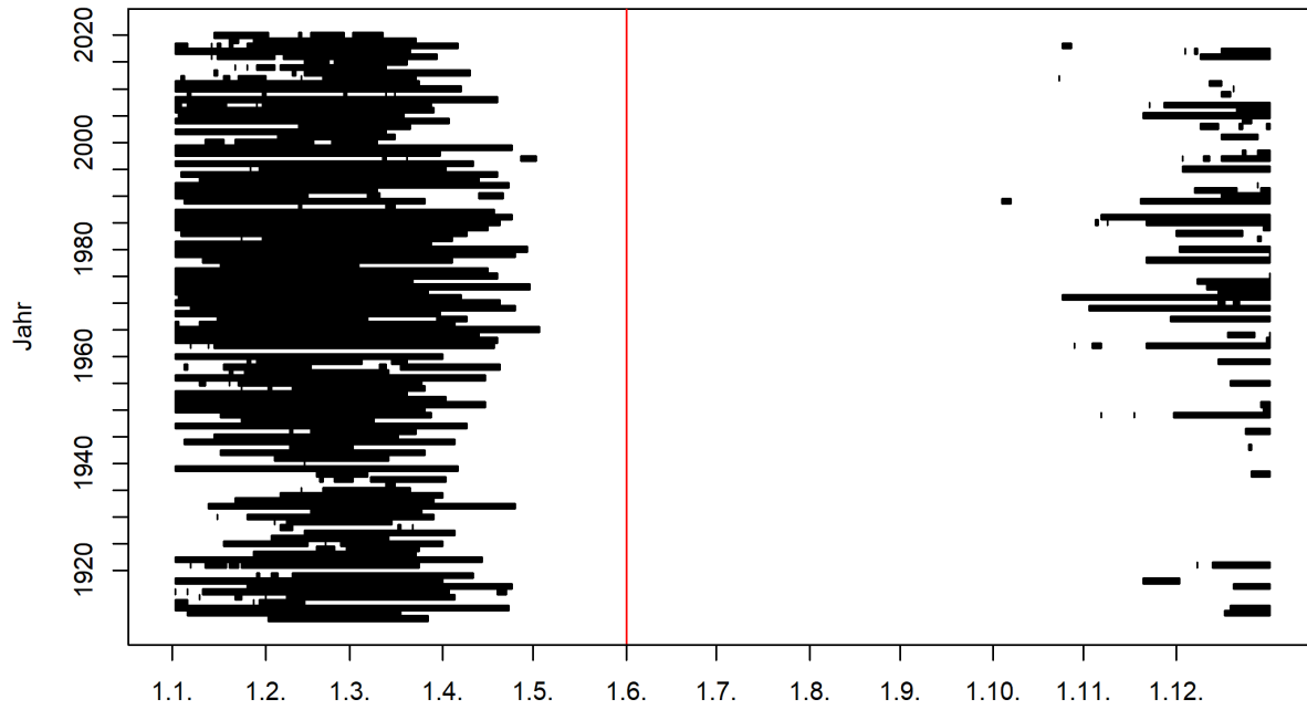
Abbildung 1: Zeitliches Auftreten der Niedrigwasserperioden im Jahresverlauf (01.06.1910 - 31.05.2020) und Startmonat des Niedrigwasserjahres (rote Linie) 1
