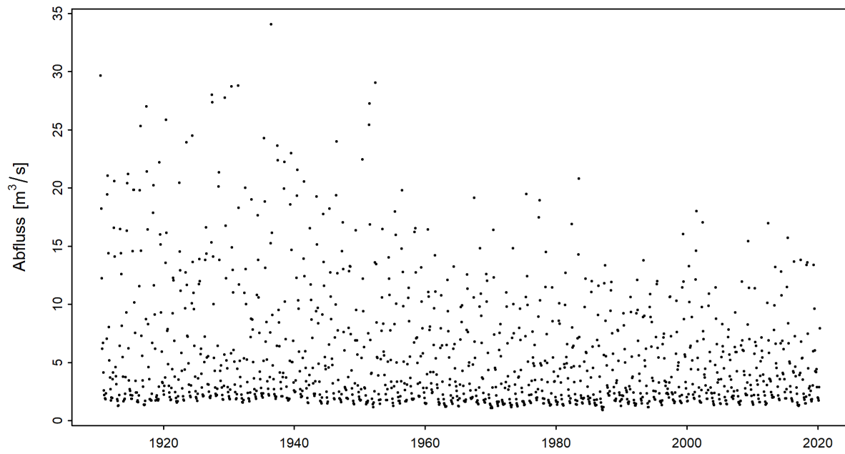
Abbildung 3: Zeitreihe der monatlichen Minima der M7Q [m³/s] (01.06.1910 - 31.05.2020)
