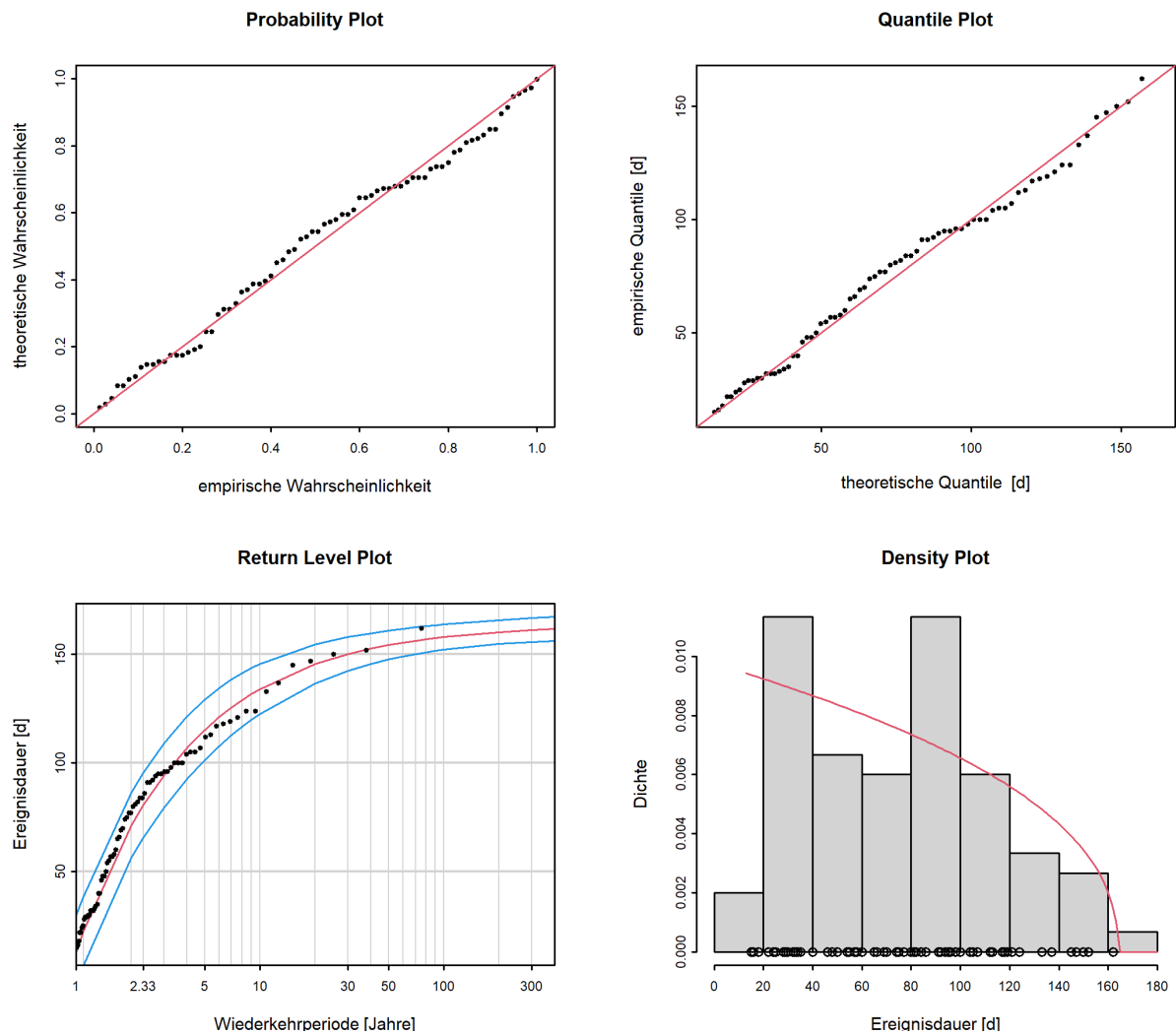
Abbildung 12: Diagnostikplots der Modellvariante “stat” des POT-Ansatzes (01.06.1945 - 31.05.2020)
