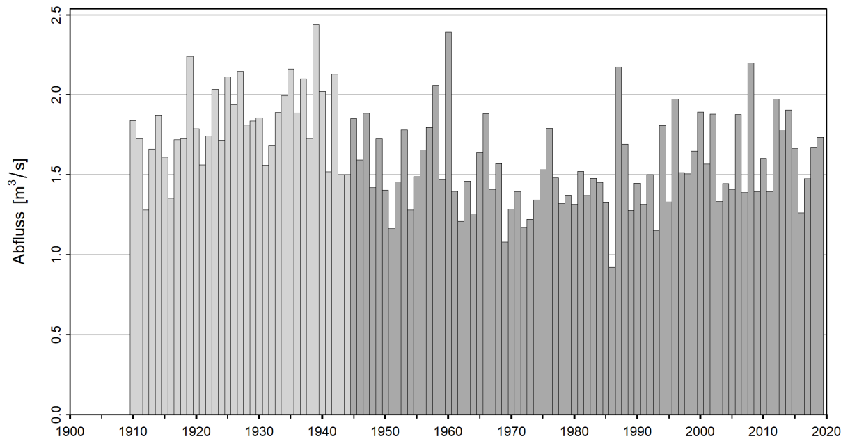
Abbildung 6: Zeitreihe der NM7Q [m³/s] (01.06.1910 - 31.05.2020), hellgrau: nicht verwendete NM7Q, dunkelgrau: verwendete NM7Q
