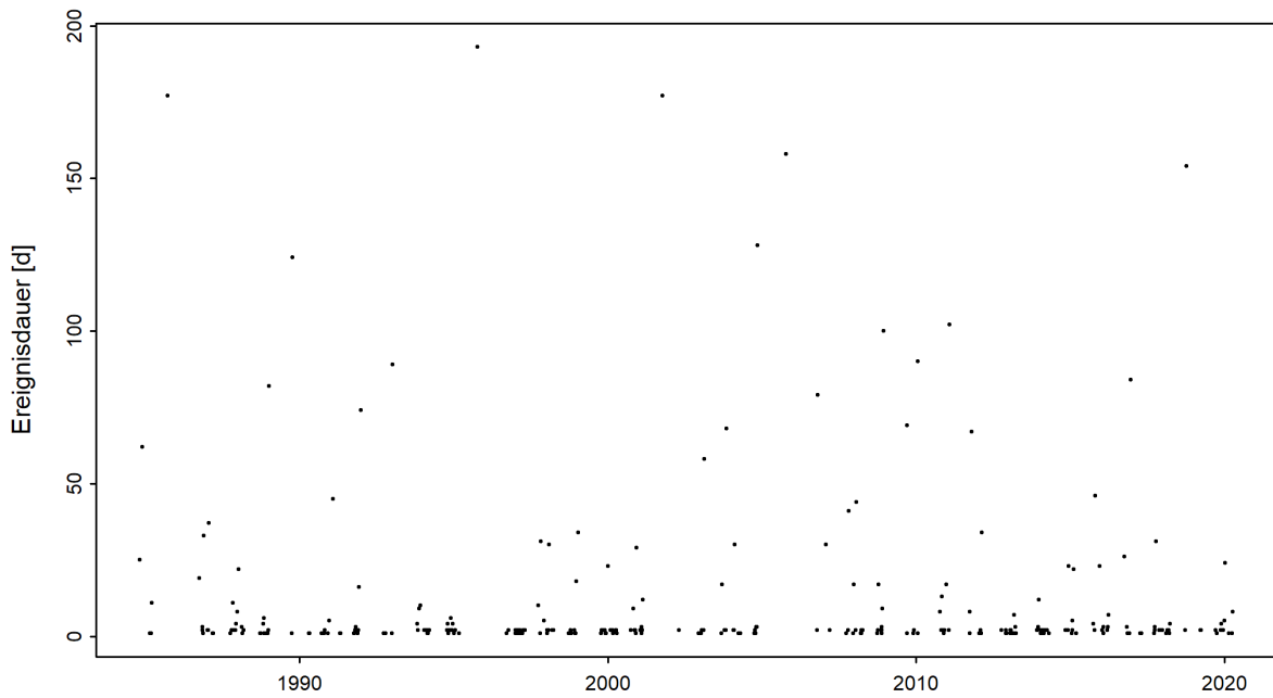
Abbildung 4: Zeitreihe der Niedrigwasserdauern [d] (01.06.1984 - 31.05.2020)
