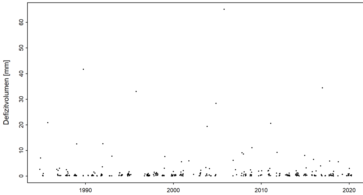
Abbildung 5: Zeitreihe der Defizitvolumen [mm] (01.06.1984 - 31.05.2020)
