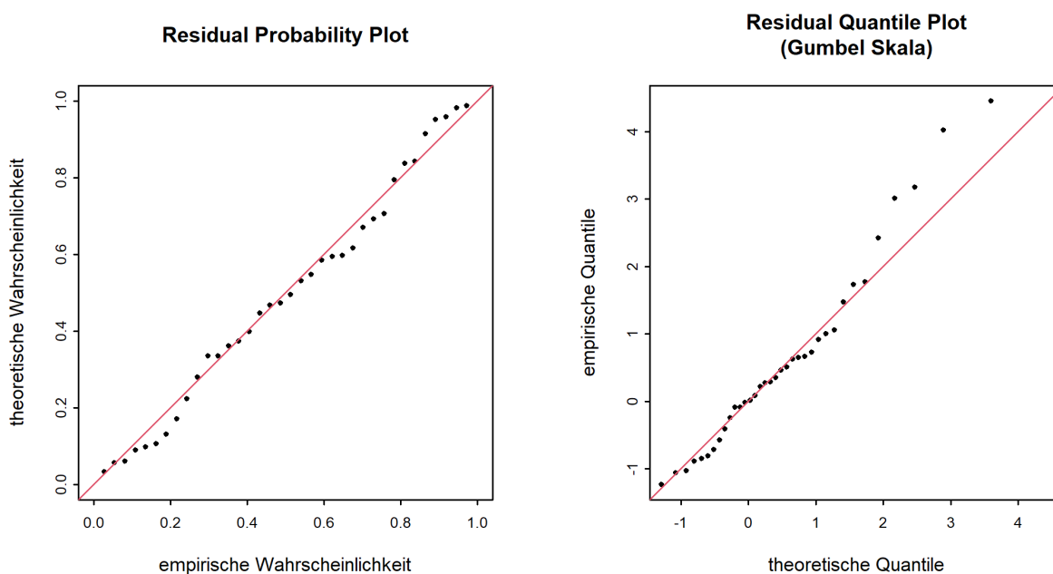
Abbildung 7: Diagnostikplots der Modellvariante “mul” des BLOCK-Ansatzes (01.06.1984 - 31.05.2020)
