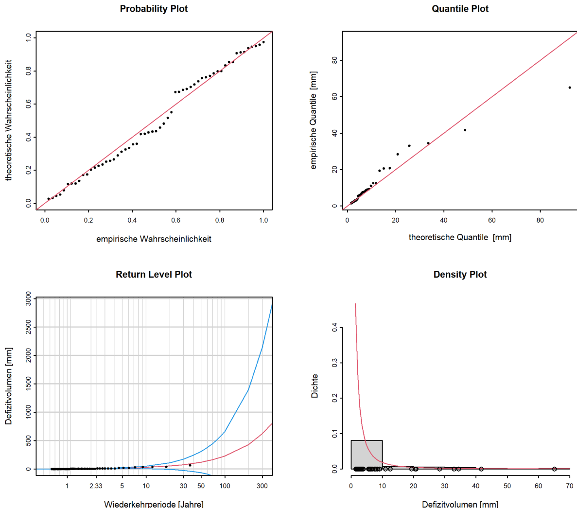
Abbildung 14: Diagnostikplots der Modellvariante "stat" des POT-Ansatzes (01.06.1984 - 31.05.2020)
