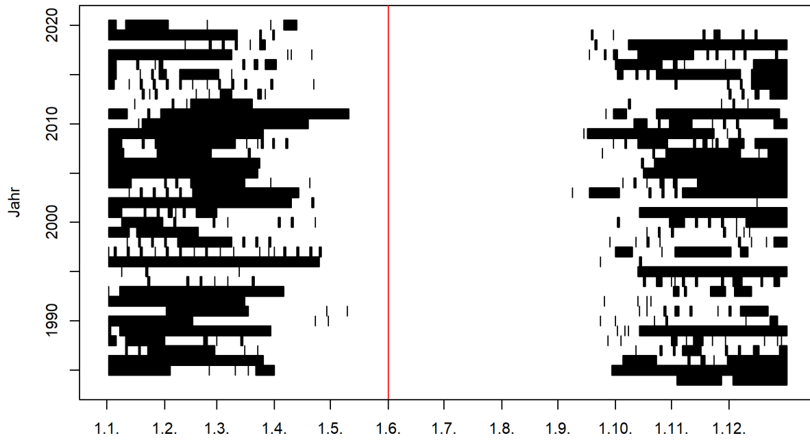
Abbildung 1: Zeitliches Auftreten der Niedrigwasserperioden im Jahresverlauf (01.06.1984 - 31.05.2020) und Startmonat des Niedrigwasserjahres (rote Linie) 1
