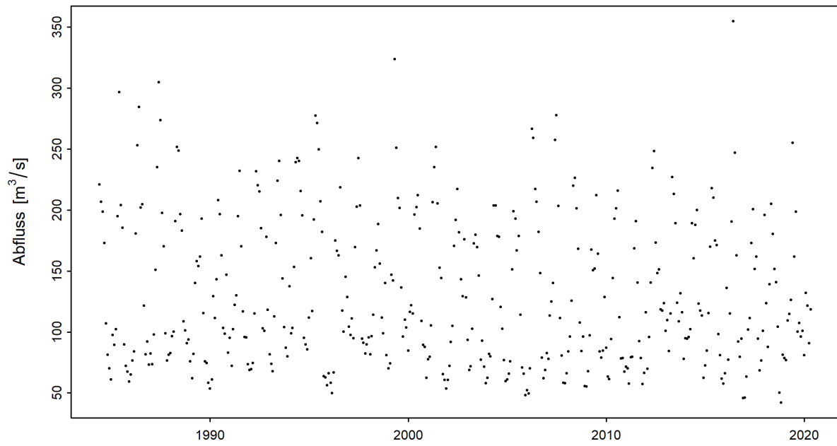
Abbildung 3: Zeitreihe der monatlichen Minima der M7Q [m 3 /s] (01.06.1984 - 31.05.2020)
