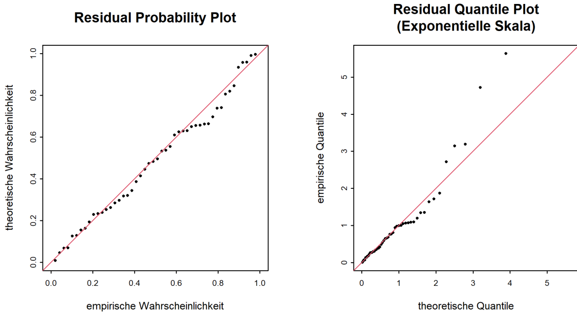
Abbildung 9: Diagnostikplots der Modellvariante “sigl” des POT-Ansatzes (01.06.1984 - 31.05.2020)
