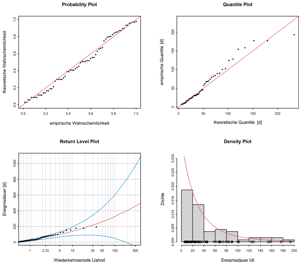
Abbildung 12: Diagnostikplots der Modellvariante “stat” des POT-Ansatzes (01.06.1984 - 31.05.2020)
