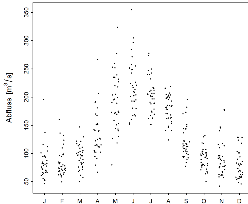
Abbildung 2: Saisonaler Verlauf der monatlichen Minima der M7Q [ \text{m}^3/\text{s} ] (01.06.1984 - 31.05.2020)
