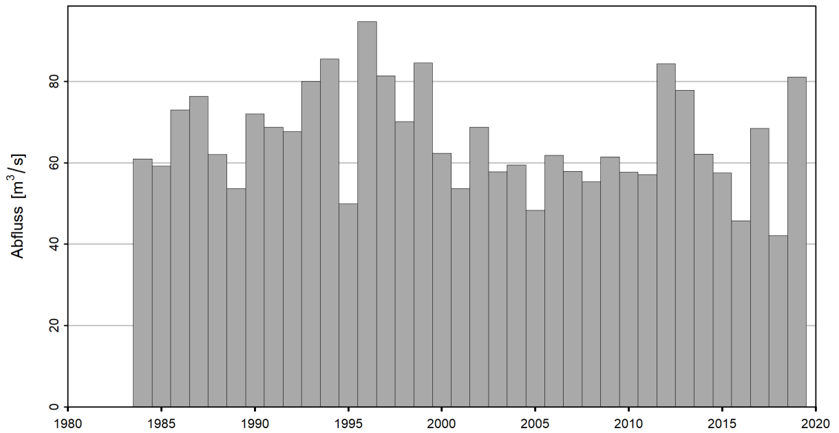
Abbildung 6: Zeitreihe der NM7Q [m 3 /s] (01.06.1984 - 31.05.2020)
