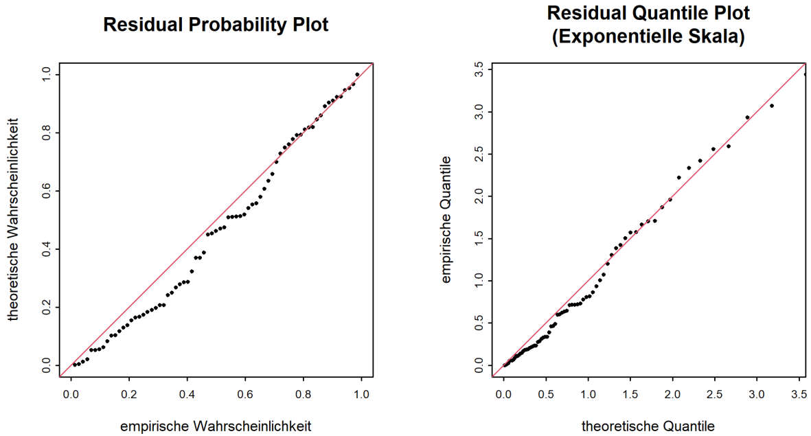
Abbildung 9: Diagnostikplots der Modellvariante “sigjump1983” des POT-Ansatzes (01.06.1969 - 31.05.2020)
