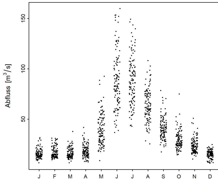
Abbildung 2: Saisonaler Verlauf der monatlichen Minima der M7Q [ \text{m}^3/\text{s} ] (01.06.1904 - 31.05.2020)
