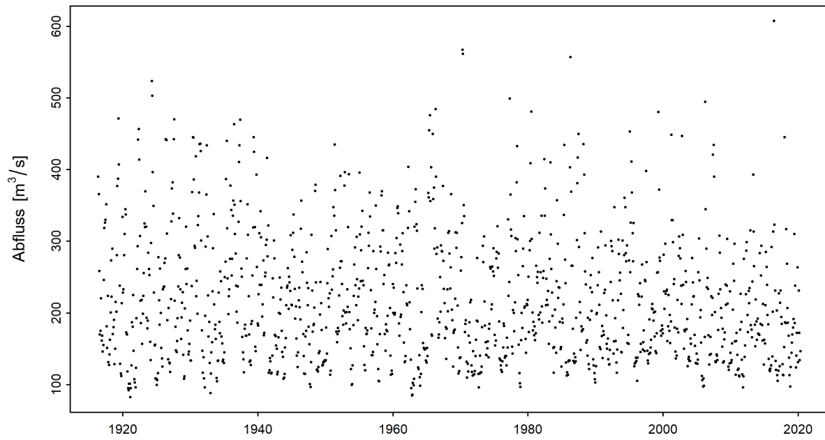
Abbildung 3: Zeitreihe der monatlichen Minima der M7Q [ \text{m}^3/\text{s} ] (01.06.1916 - 31.05.2020)
