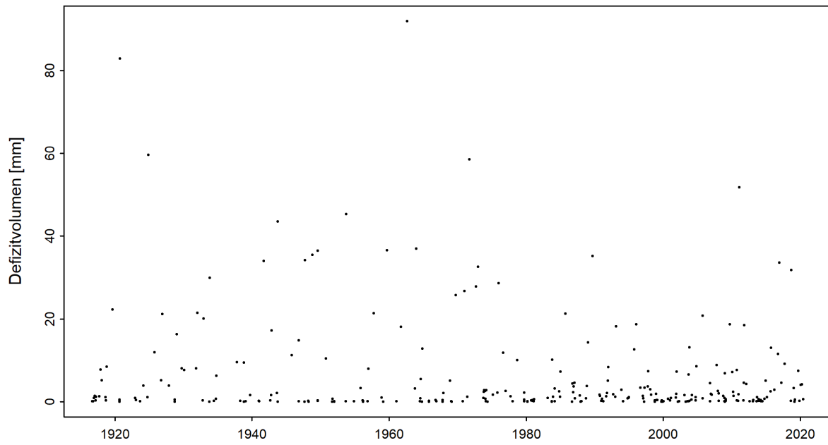
Abbildung 5: Zeitreihe der Defizitvolumen [mm] (01.06.1916 - 31.05.2020)
