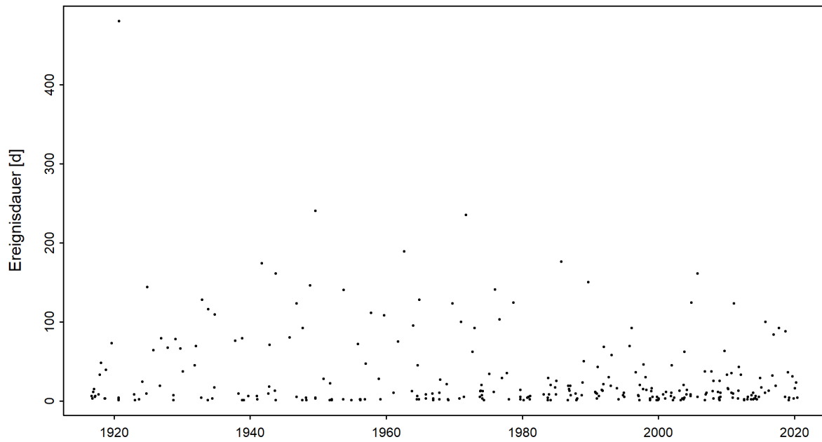
Abbildung 4: Zeitreihe der Niedrigwasserdauern [d] (01.06.1916 - 31.05.2020)
