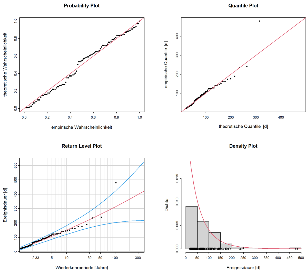
Abbildung 12: Diagnostikplots der Modellvariante “stat” des POT-Ansatzes (01.06.1916 - 31.05.2020)
