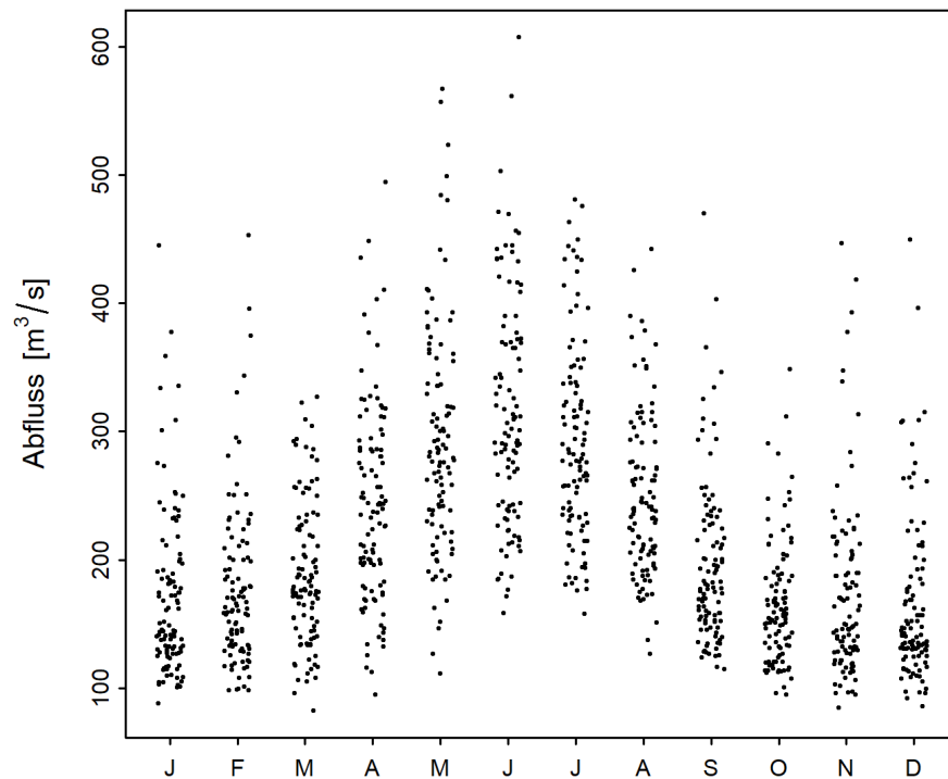
Abbildung 2: Saisonaler Verlauf der monatlichen Minima der M7Q [m³/s] (01.06.1916 - 31.05.2020)
