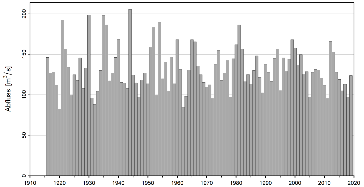
Abbildung 6: Zeitreihe der NM7Q [m³/s] (01.06.1916 - 31.05.2020)
