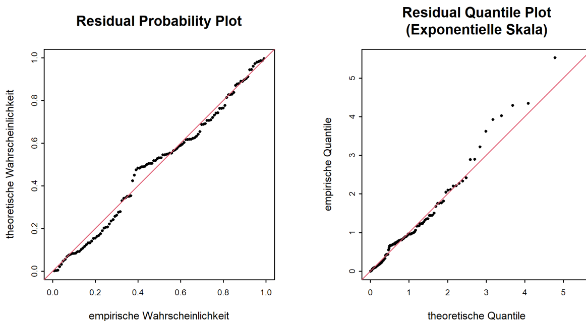
Abbildung 9: Diagnostikplots der Modellvariante “sigl” des POT-Ansatzes (01.06.1916 - 31.05.2020)
