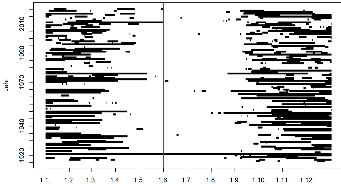
Abbildung 1: Zeitliches Auftreten der Niedrigwasserperioden im Jahresverlauf (01.06.1916 - 31.05.2020) und Startmonat des Niedrigwasserjahres (rote Linie) 1
