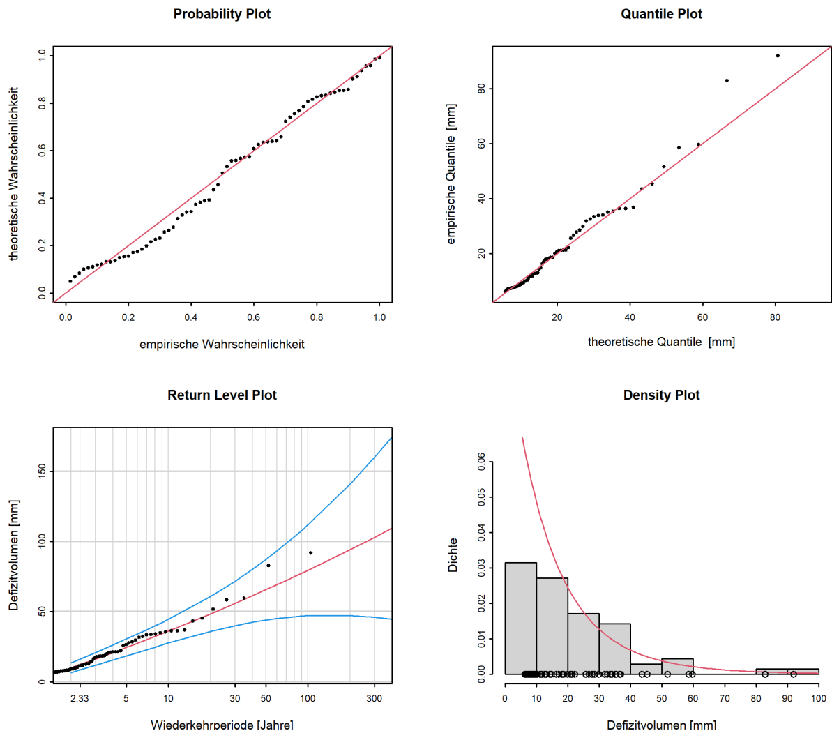
Abbildung 14: Diagnostikplots der Modellvariante “stat” des POT-Ansatzes (01.06.1916 - 31.05.2020)
