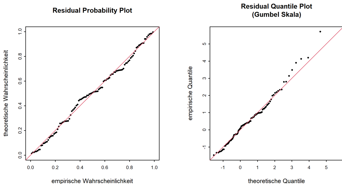
Abbildung 7: Diagnostikplots der Modellvariante "sigl" des BLOCK-Ansatzes (01.06.1916 - 31.05.2020)
