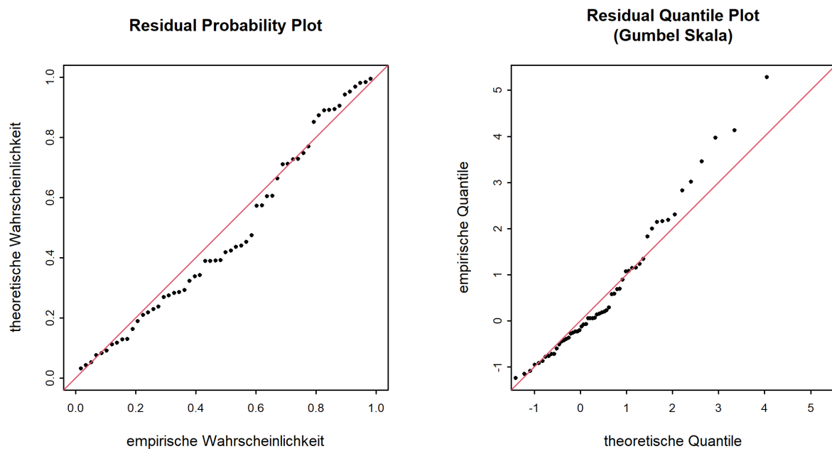
Abbildung 7: Diagnostikplots der Modellvariante "sigl" des BLOCK-Ansatzes (01.06.1963 - 31.05.2020)
