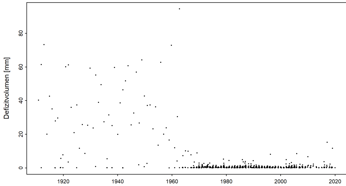
Abbildung 5: Zeitreihe der Defizitvolumen [mm] (01.06.1910 - 31.05.2020)
