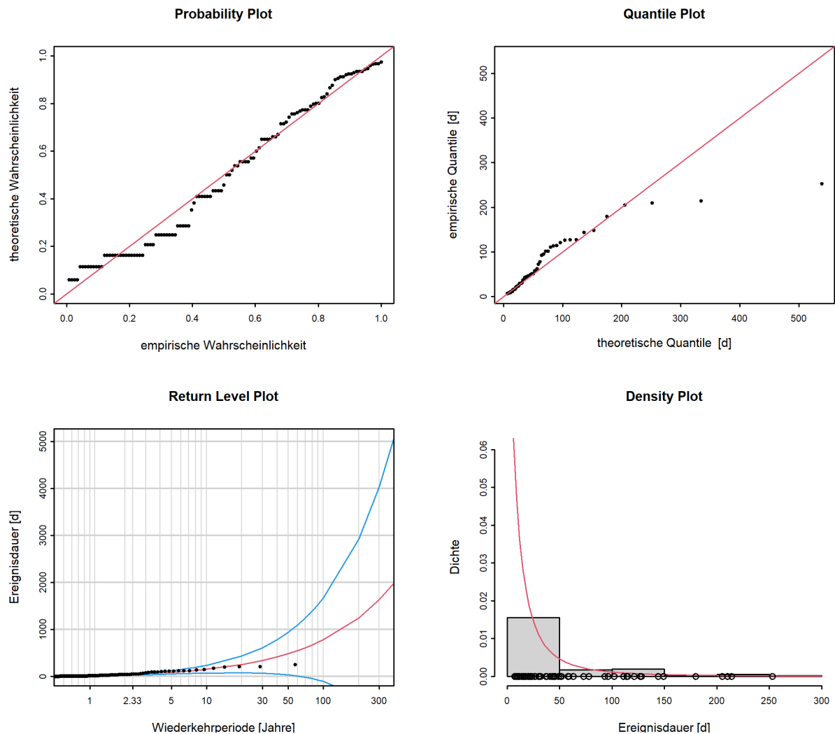
Abbildung 12: Diagnostikplots der Modellvariante “stat” des POT-Ansatzes (01.06.1963 - 31.05.2020)
