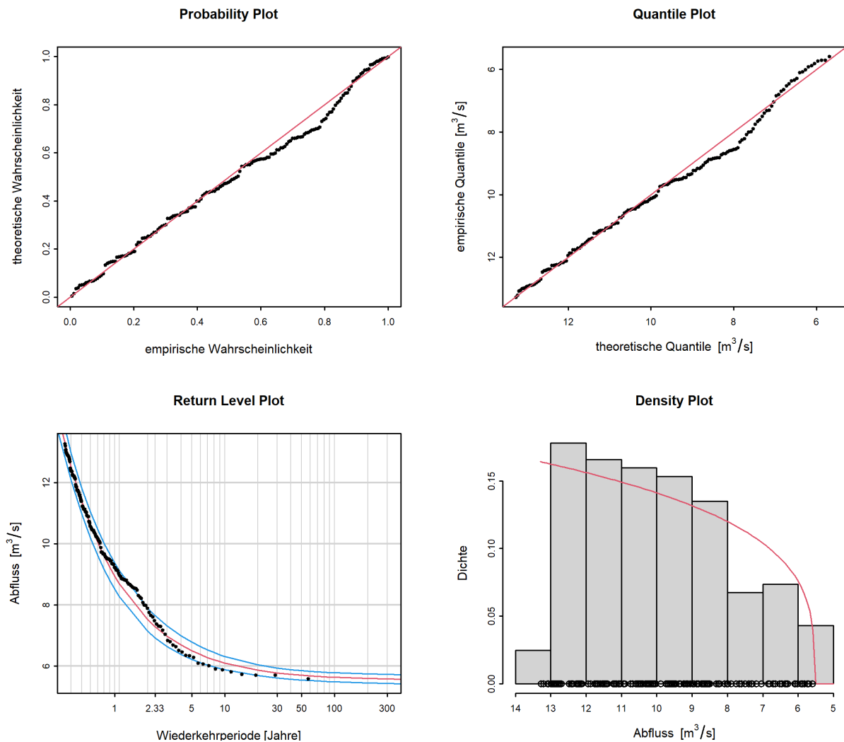
Abbildung 9: Diagnostikplots der Modellvariante “stat” des POT-Ansatzes (01.06.1963 - 31.05.2020)
