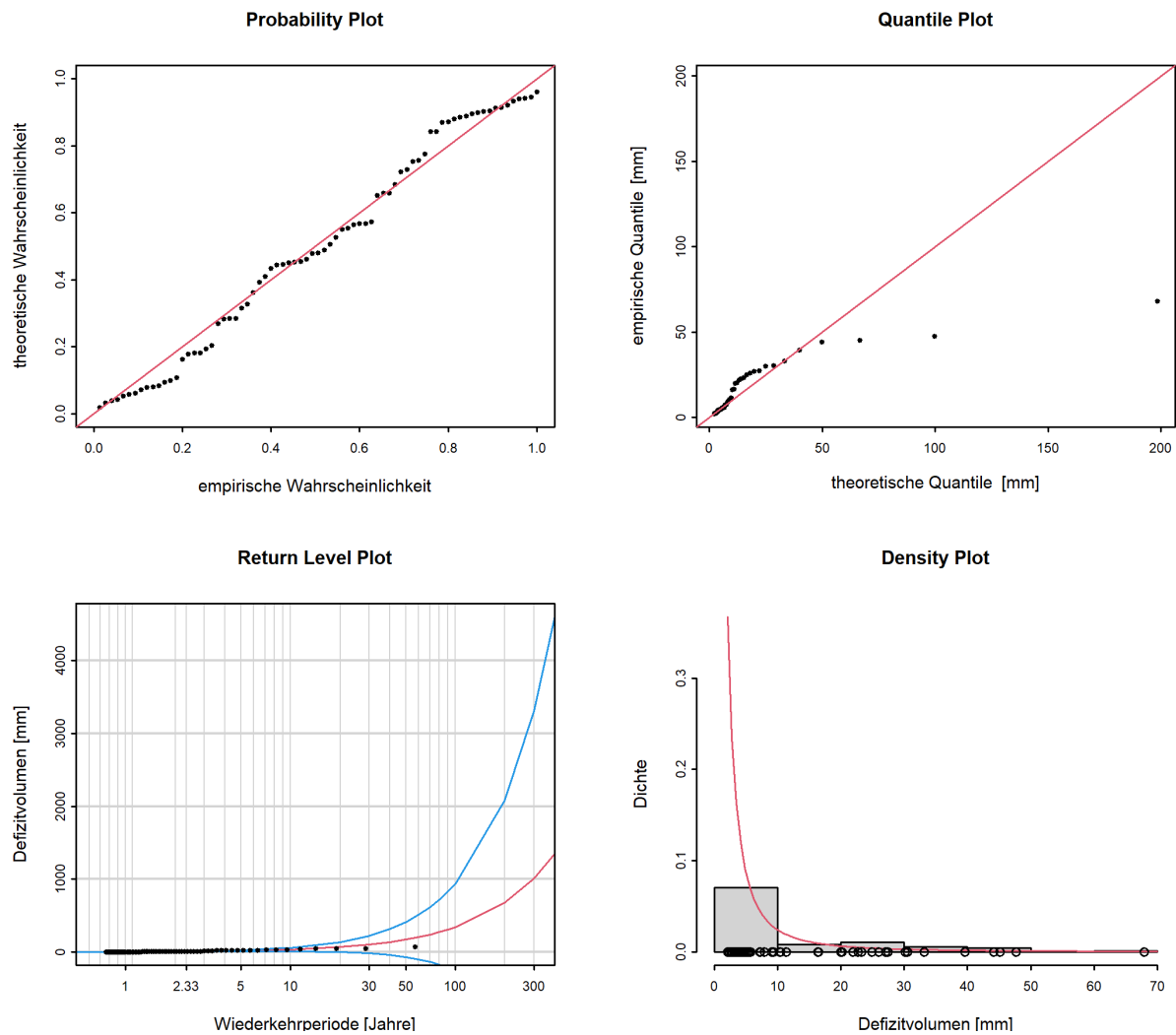
Abbildung 14: Diagnostikplots der Modellvariante “stat” des POT-Ansatzes (01.06.1963 - 31.05.2020)
