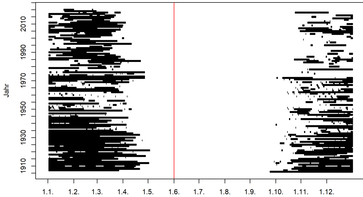
Abbildung 1: Zeitliches Auftreten der Niedrigwasserperioden im Jahresverlauf (01.06.1906 - 31.05.2020) und Startmonat des Niedrigwasserjahres (rote Linie) 1
