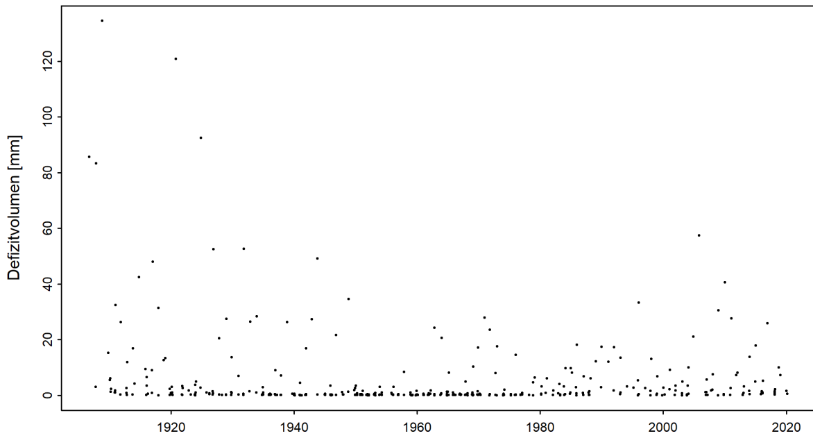
Abbildung 5: Zeitreihe der Defizitvolumen [mm] (01.06.1906 - 31.05.2020)
