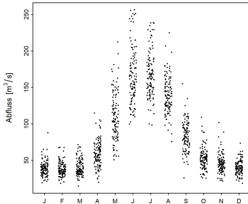
Abbildung 2: Saisonaler Verlauf der monatlichen Minima der M7Q [ \text{m}^3/\text{s} ] (01.06.1906 - 31.05.2020)
