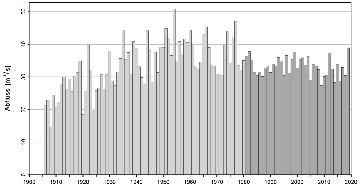
Abbildung 6: Zeitreihe der NM7Q [ \text{m}^3/\text{s} ] (01.06.1906 - 31.05.2020), hellgrau: nicht verwendete NM7Q, dunkelgrau: verwendete NM7Q
