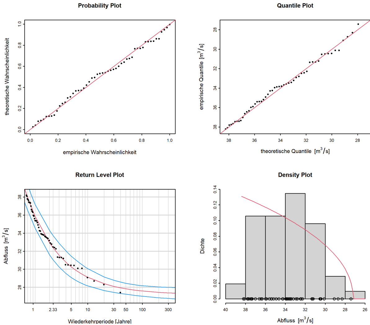
Abbildung 9: Diagnostikplots der Modellvariante "stat" des POT-Ansatzes (01.06.1981 - 31.05.2020)
