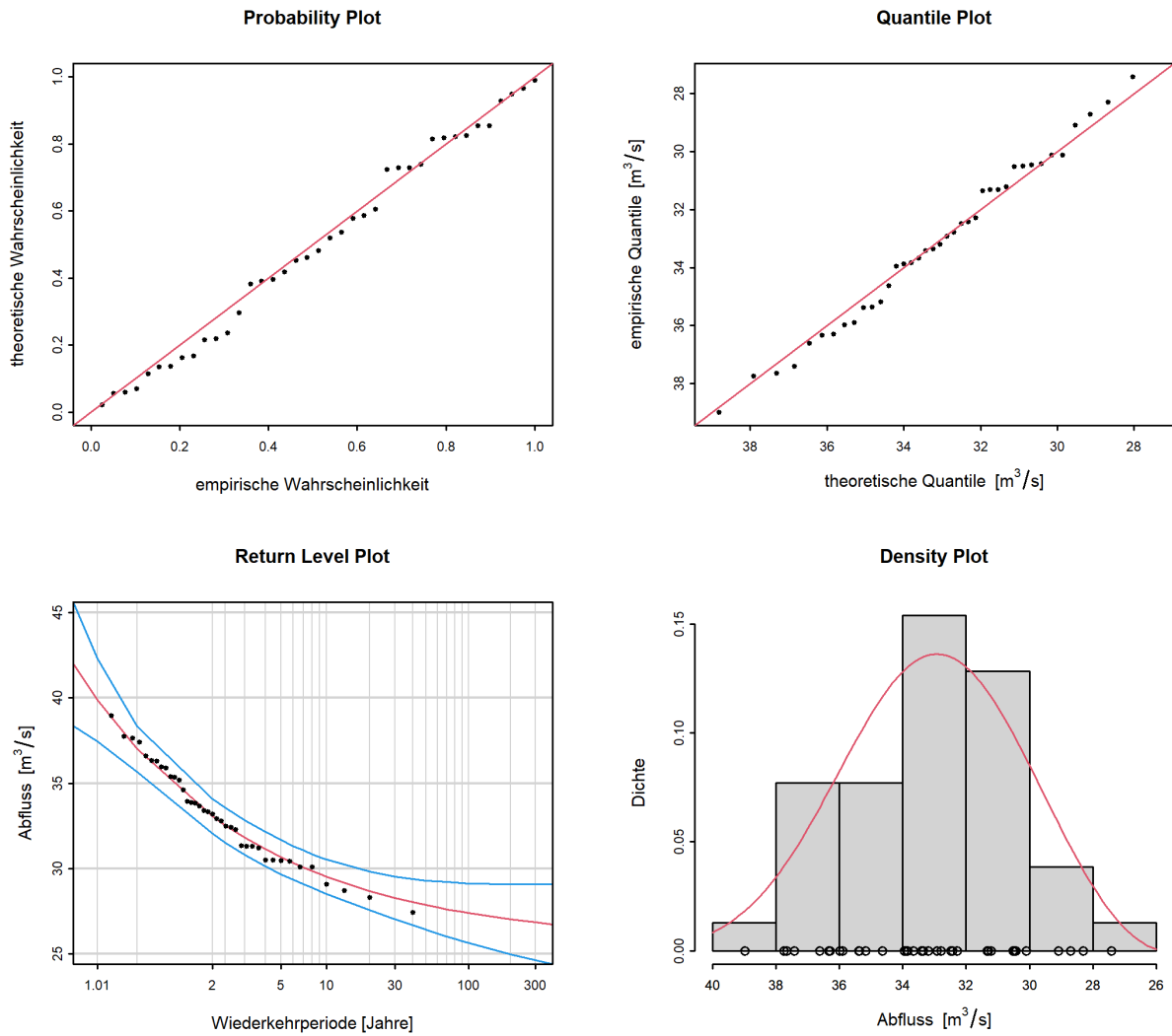
Abbildung 7: Diagnostikplots der Modellvariante “stat” des BLOCK-Ansatzes (01.06.1981 - 31.05.2020)
