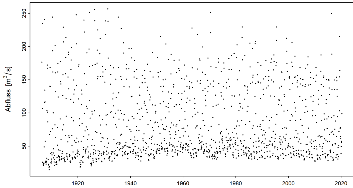
Abbildung 3: Zeitreihe der monatlichen Minima der M7Q [ \text{m}^3/\text{s} ] (01.06.1906 - 31.05.2020)
