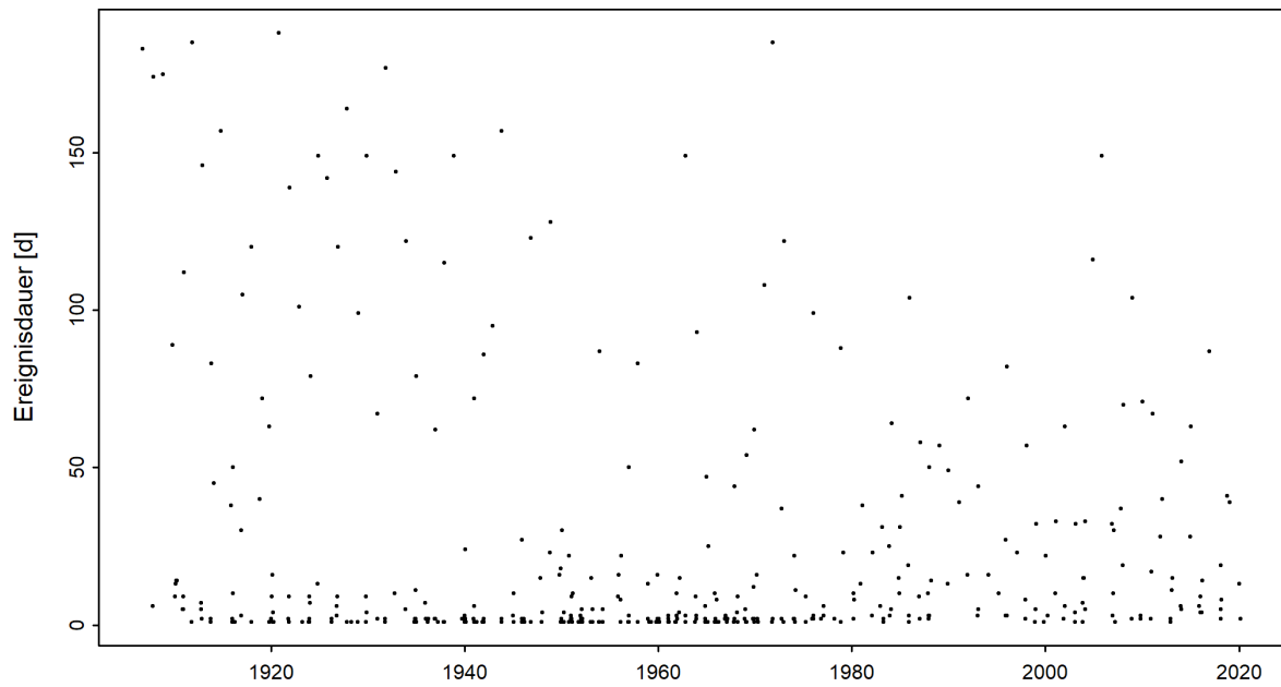
Abbildung 4: Zeitreihe der Niedrigwasserdauern [d] (01.06.1906 - 31.05.2020)
