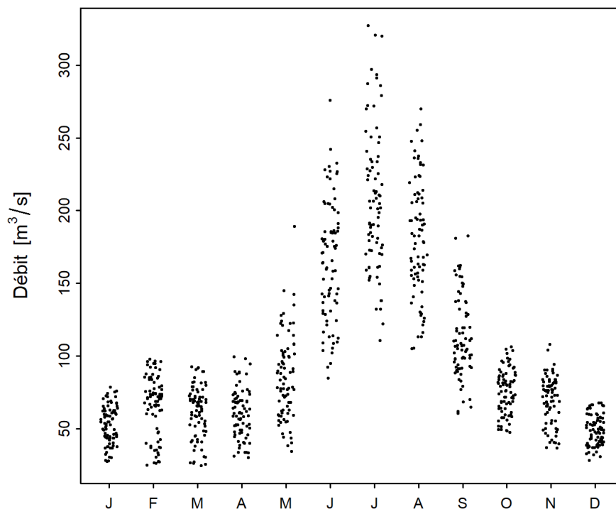
FIGURE 2 – Évolution saisonnière du minimum mensuel de M7Q [ \text{m}^3/\text{s} ] (01.06.1941 - 31.05.2020)
