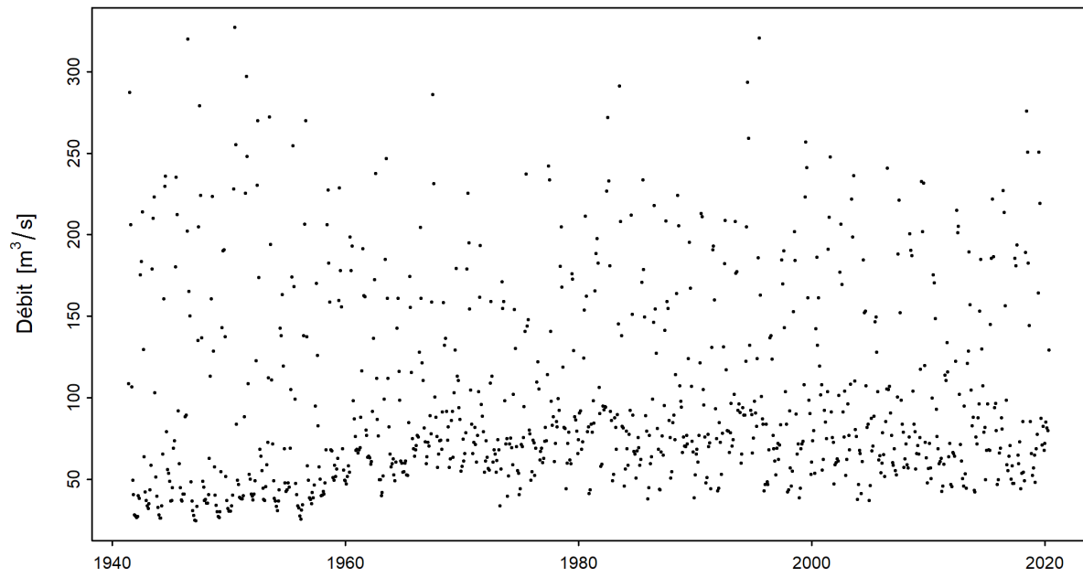
FIGURE 3 – Série temporelle du minimum mensuel de M7Q [ \text{m}^3/\text{s} ] (01.06.1941 - 31.05.2020)
