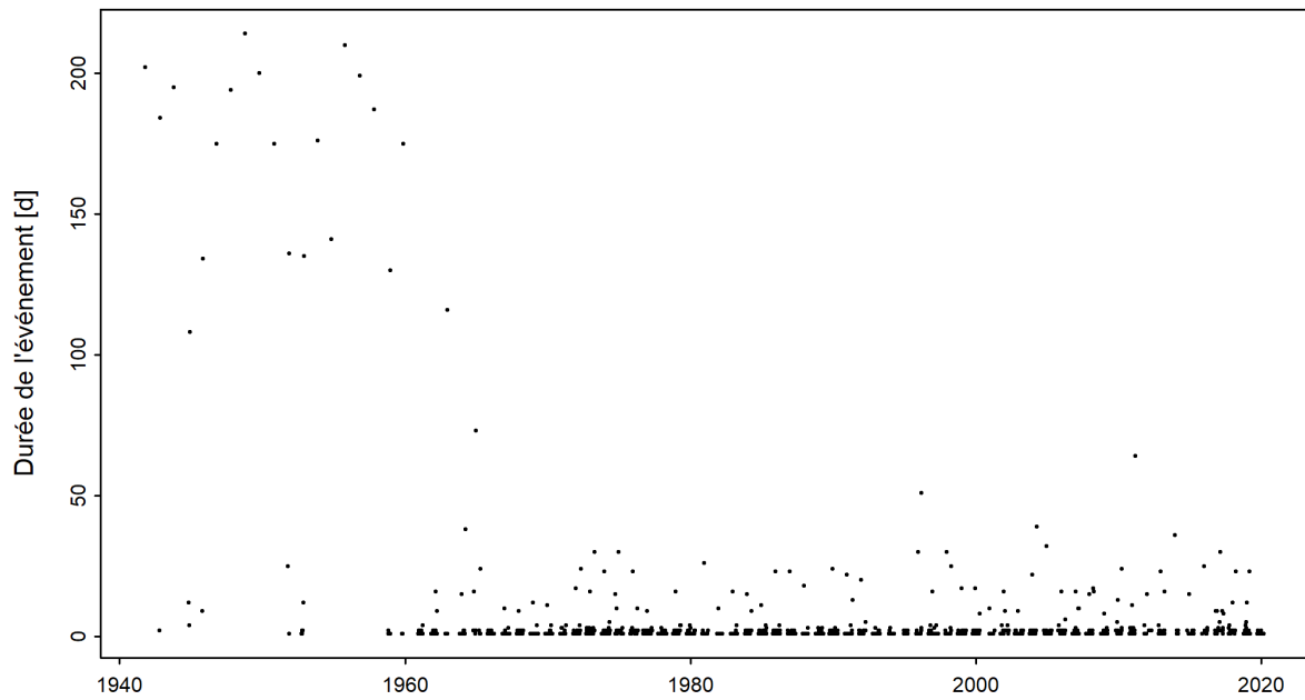
FIGURE 4 – Série temporelle des durées d'étéage [d] (01.06.1941 - 31.05.2020)
