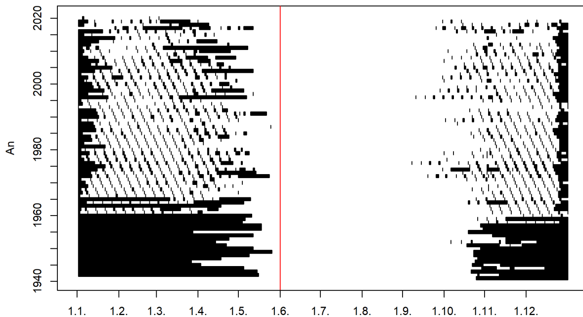
FIGURE 1 – Apparition temporelle des périodes d’étéage pendant l’année (01.06.1941 - 31.05.2020) et mois de début de l’année d’étéage (ligne rouge) 1
