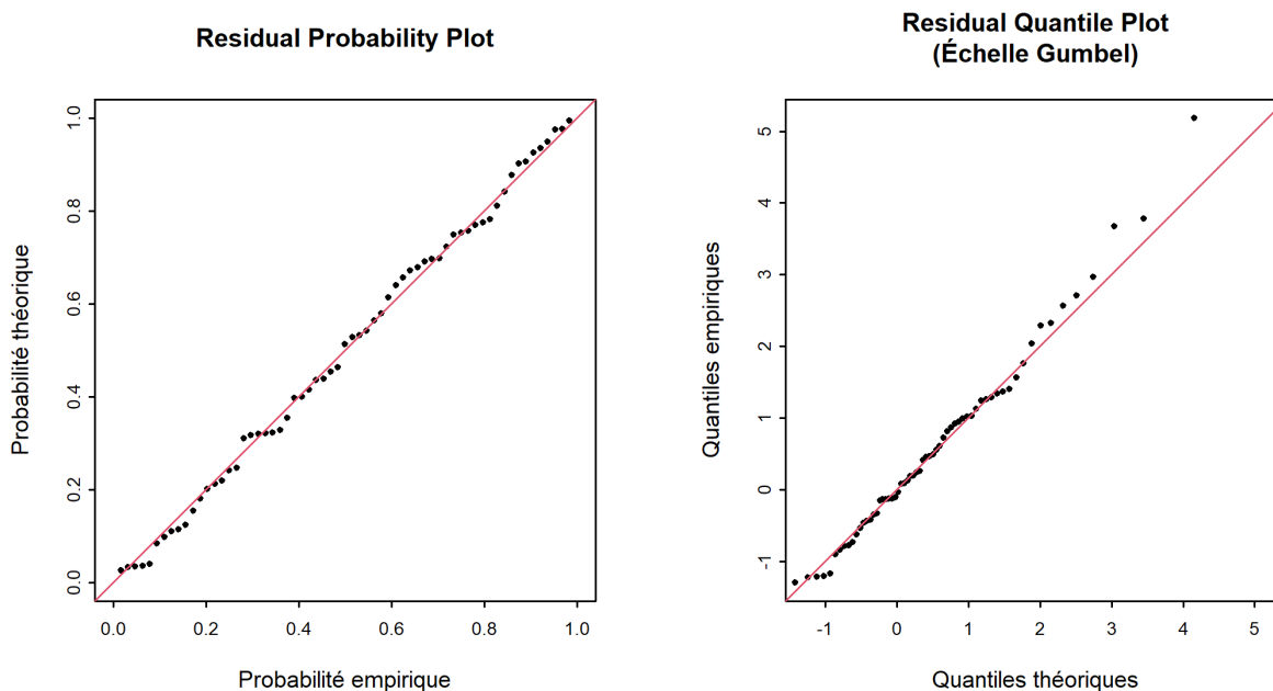
FIGURE 7 – Graphiques diagnostiques de la variante du modèle " mujump1972 " de la méthode BLOCK (01.06.1957 - 31.05.2020)
