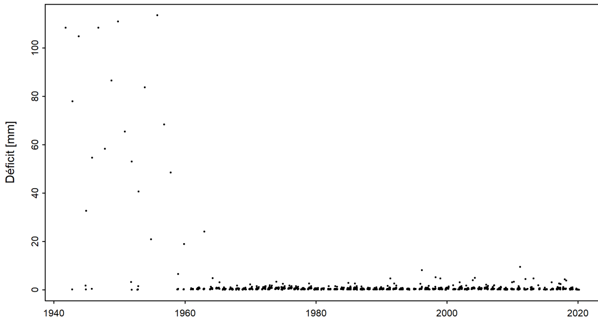
FIGURE 5 – Série temporelle du volume déficitaire [mm] (01.06.1941 - 31.05.2020)
