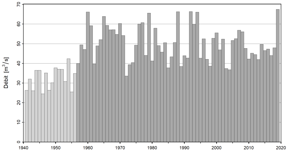
FIGURE 6 – Série temporelle de NM7Q [ \text{m}^3/\text{s} ] (01.06.1941 - 31.05.2020), gris clair : NM7Q non utilisés, gris foncé : NM7Q utilisés
