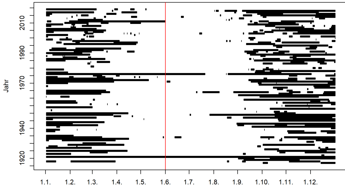
Abbildung 1: Zeitliches Auftreten der Niedrigwasserperioden im Jahresverlauf (01.06.1916 - 31.05.2019) und Startmonat des Niedrigwasserjahres (rote Linie) 1
