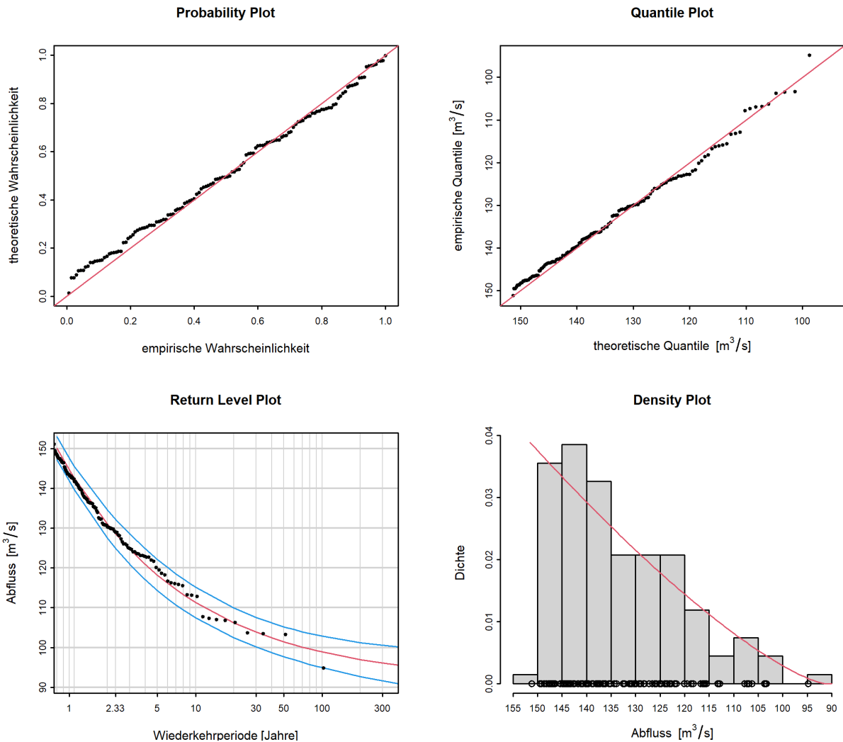
Abbildung 9: Diagnostikplots der Modellvariante "stat" des POT-Ansatzes (01.06.1917 - 31.05.2019)
