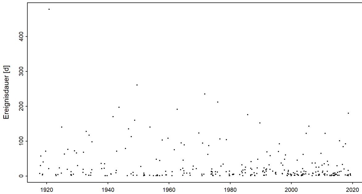
Abbildung 4: Zeitreihe der Niedrigwasserdauern [d] (01.06.1916 - 31.05.2019)
