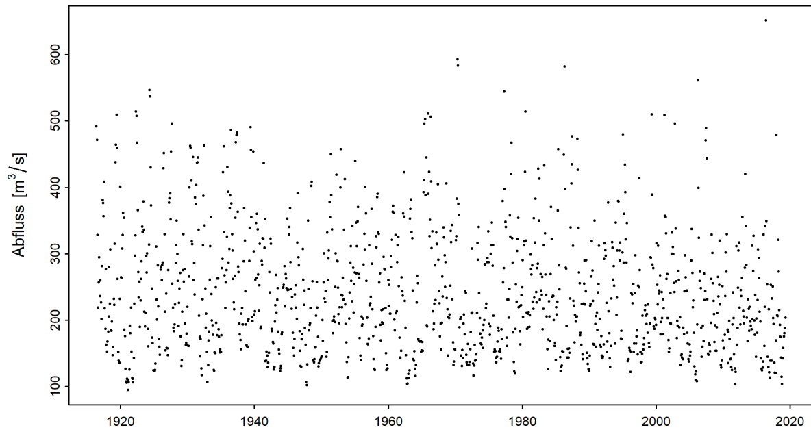
Abbildung 3: Zeitreihe der monatlichen Minima der M7Q [m 3 /s] (01.06.1916 - 31.05.2019)
