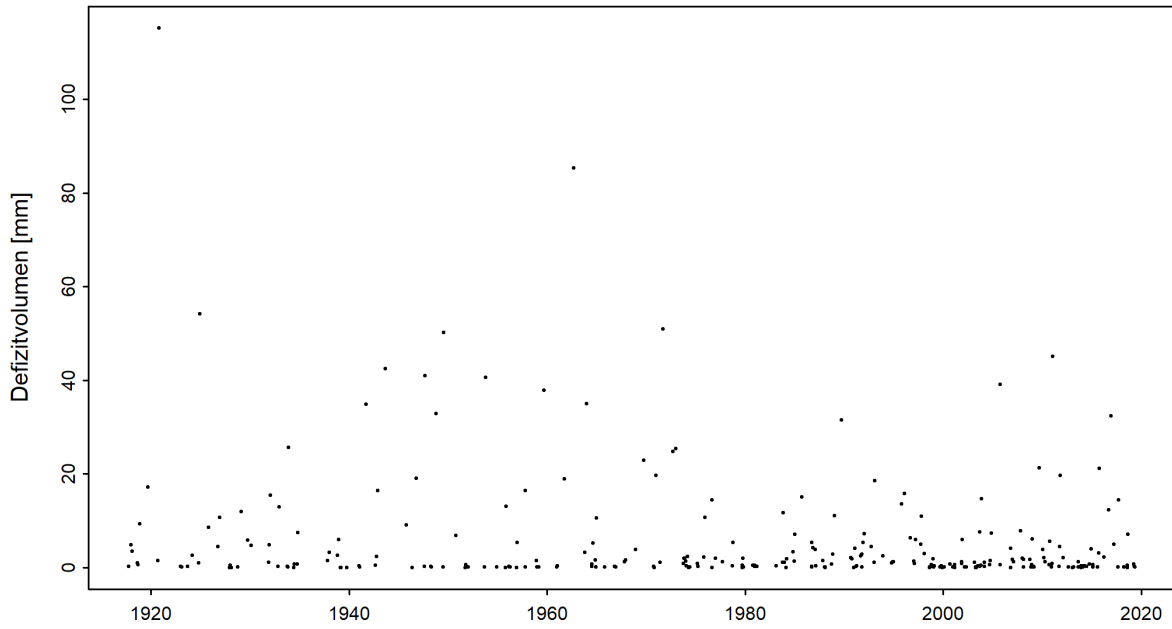
Abbildung 5: Zeitreihe der Defizitvolumen [mm] (01.06.1916 - 31.05.2019)
