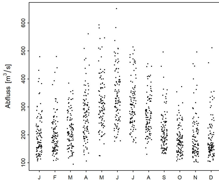
Abbildung 2: Saisonaler Verlauf der monatlichen Minima der M7Q [ \text{m}^3/\text{s} ] (01.06.1916 - 31.05.2019)
