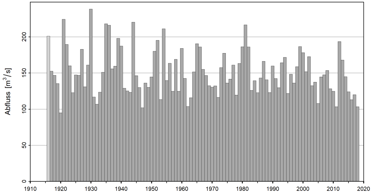
Abbildung 6: Zeitreihe der NM7Q [ \text{m}^3/\text{s} ] (01.06.1916 - 31.05.2019), hellgrau: nicht verwendete NM7Q, dunkelgrau: verwendete NM7Q
