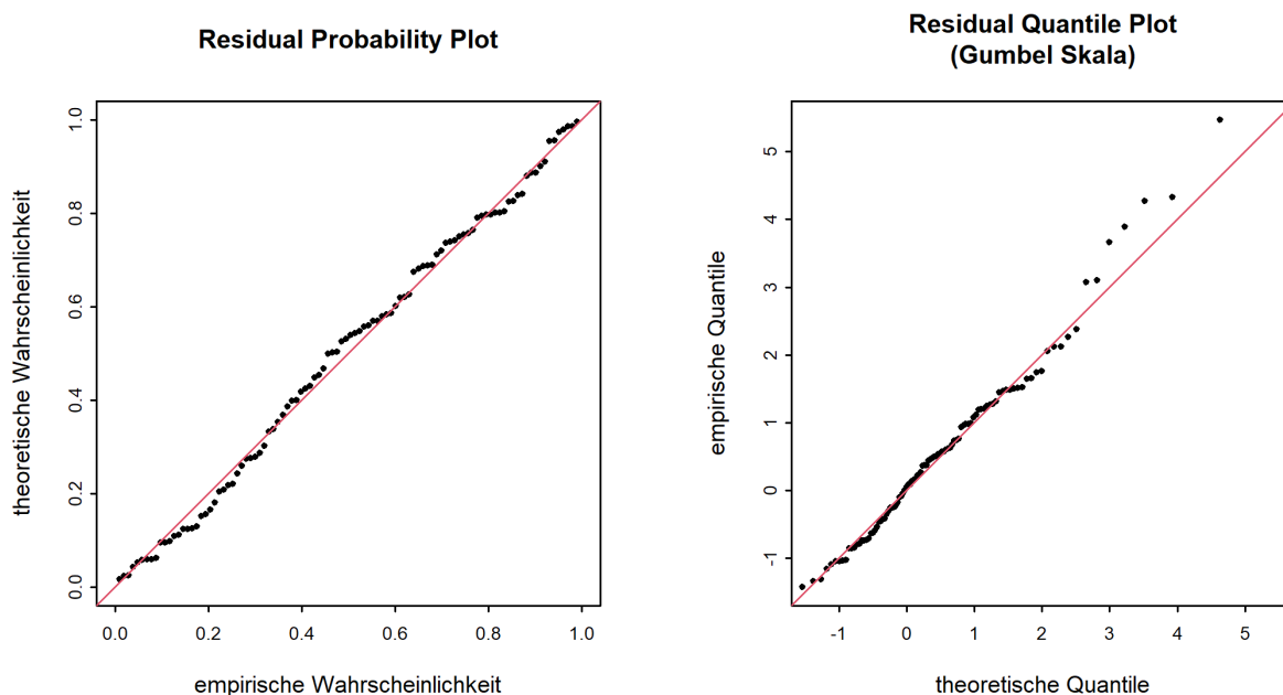
Abbildung 7: Diagnostikplots der Modellvariante "musigl" des BLOCK-Ansatzes (01.06.1917 - 31.05.2019)
