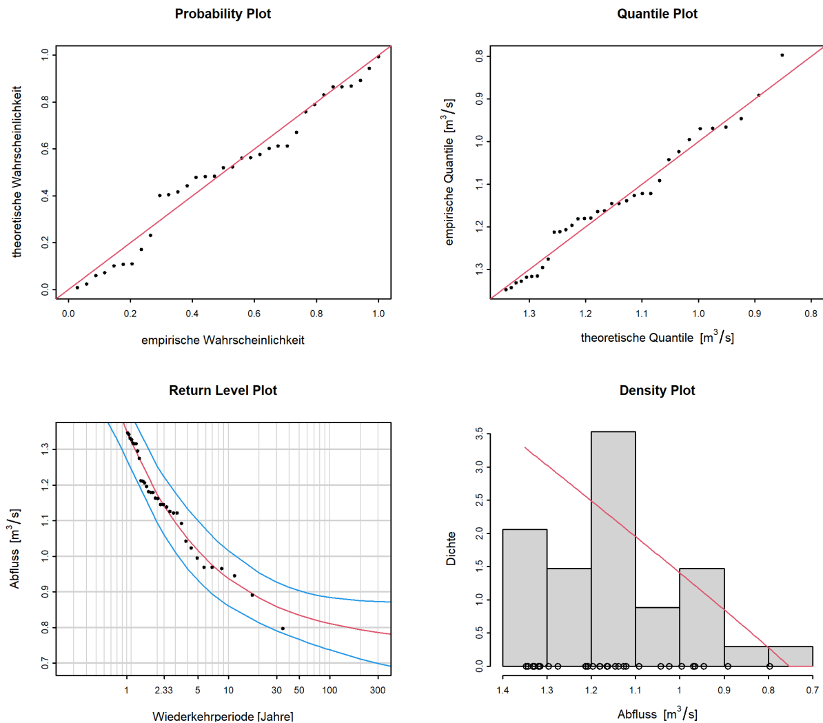
Abbildung 9: Diagnostikplots der Modellvariante “stat” des POT-Ansatzes (01.06.1986 - 31.05.2020)
