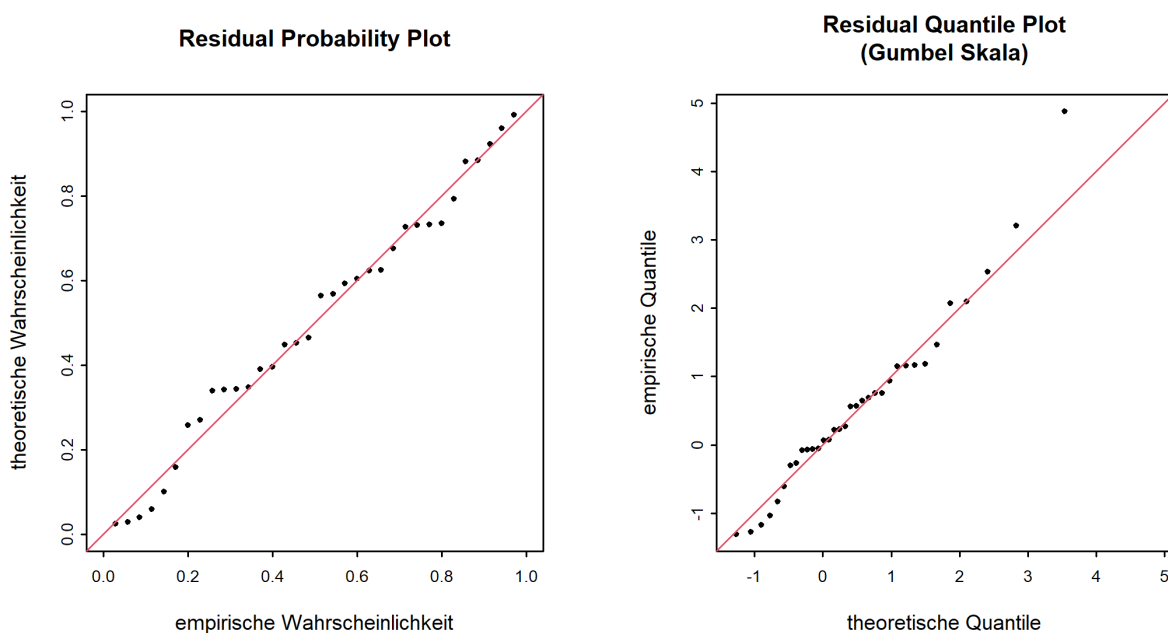
Abbildung 7: Diagnostikplots der Modellvariante “muq” des BLOCK-Ansatzes (01.06.1986 - 31.05.2020)
