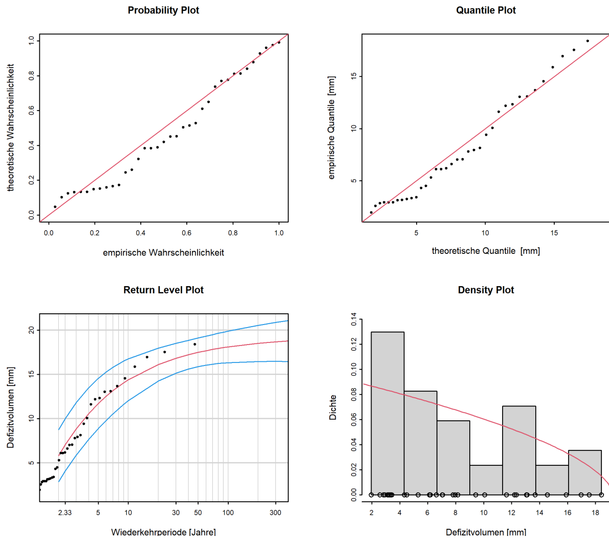
Abbildung 14: Diagnostikplots der Modellvariante "stat" des POT-Ansatzes (01.06.1974 - 31.05.2020)
