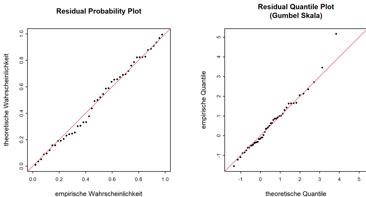
Abbildung 7: Diagnostikplots der Modellvariante "sigl" des BLOCK-Ansatzes (01.06.1974 - 31.05.2020)
