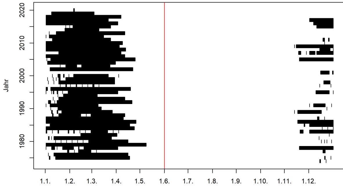
Abbildung 1: Zeitliches Auftreten der Niedrigwasserperioden im Jahresverlauf (01.06.1974 - 31.05.2020) und Startmonat des Niedrigwasserjahres (rote Linie) 1
