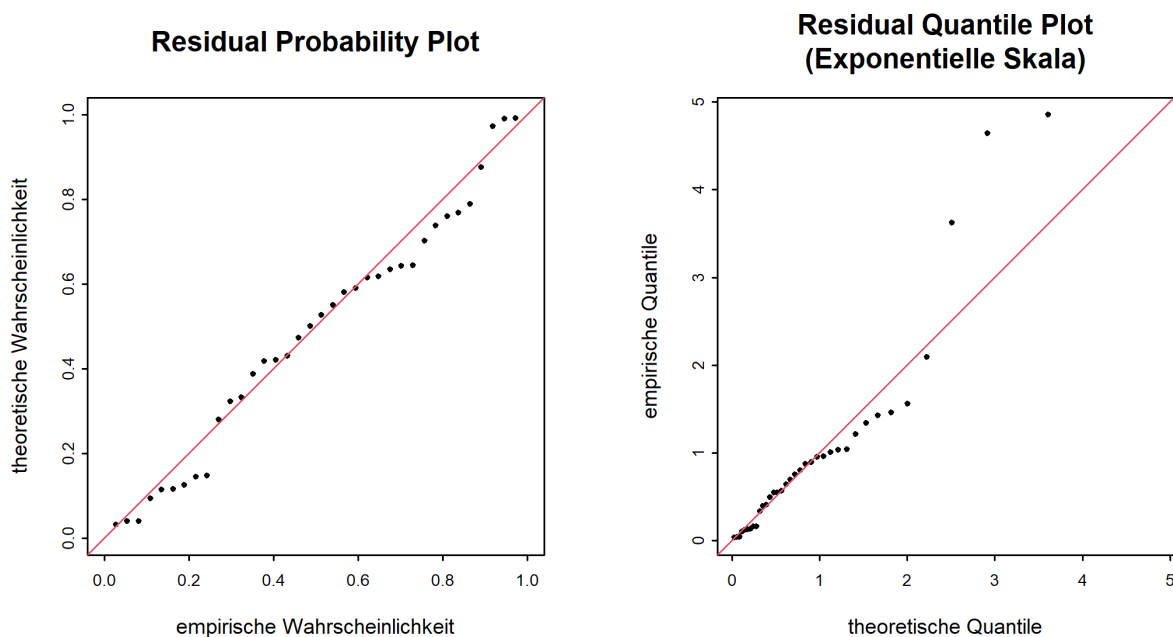
Abbildung 9: Diagnostikplots der Modellvariante “sigjump2004” des POT-Ansatzes (01.06.1974 - 31.05.2020)
