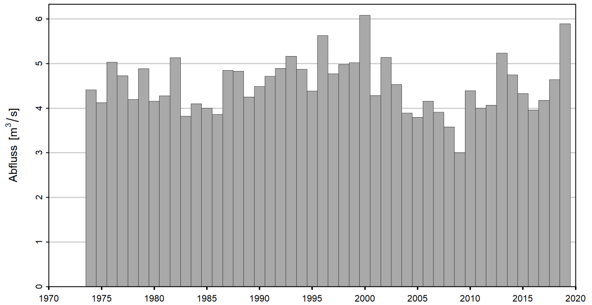
Abbildung 6: Zeitreihe der NM7Q [m³/s] (01.06.1974 - 31.05.2020)
