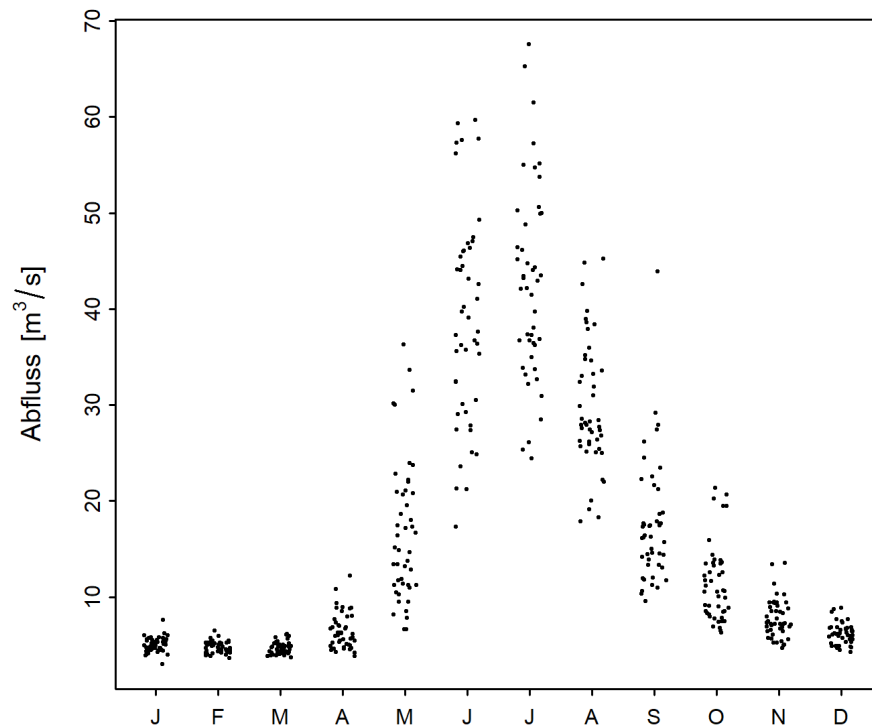
Abbildung 2: Saisonaler Verlauf der monatlichen Minima der M7Q [m³/s] (01.06.1974 - 31.05.2020)
