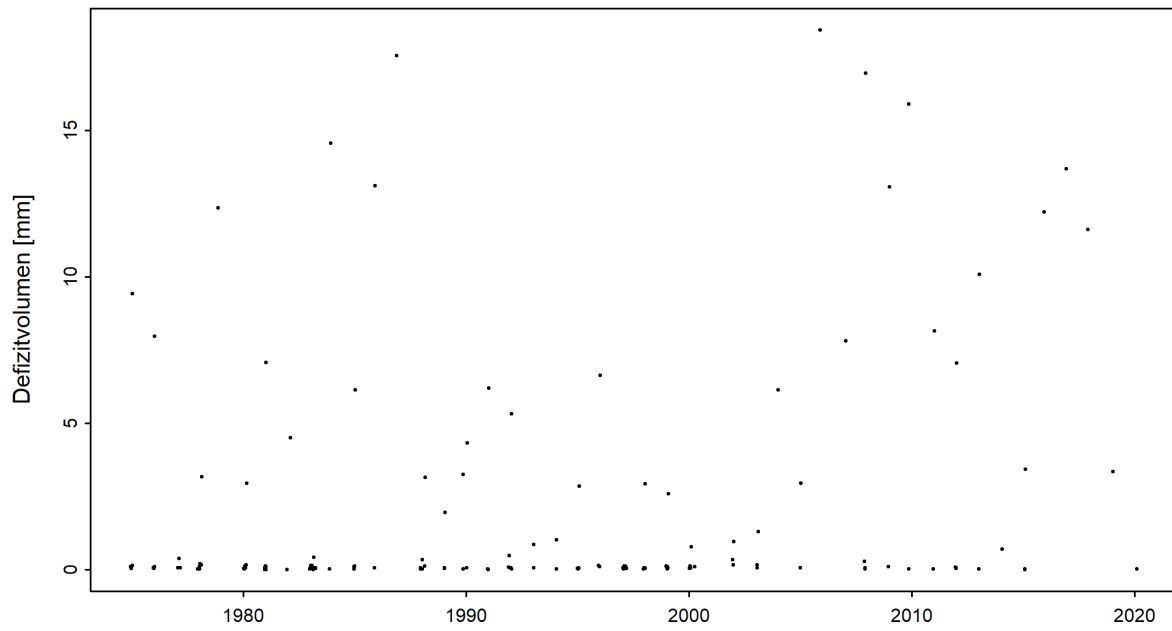
Abbildung 5: Zeitreihe der Defizitvolumen [mm] (01.06.1974 - 31.05.2020)
