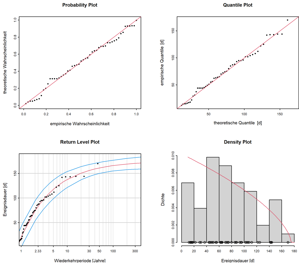
Abbildung 12: Diagnostikplots der Modellvariante “stat” des POT-Ansatzes (01.06.1974 - 31.05.2020)
