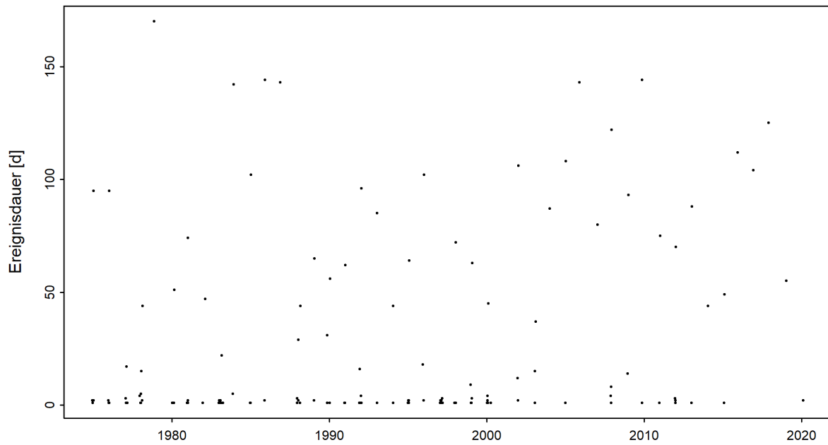
Abbildung 4: Zeitreihe der Niedrigwasserdauern [d] (01.06.1974 - 31.05.2020)
