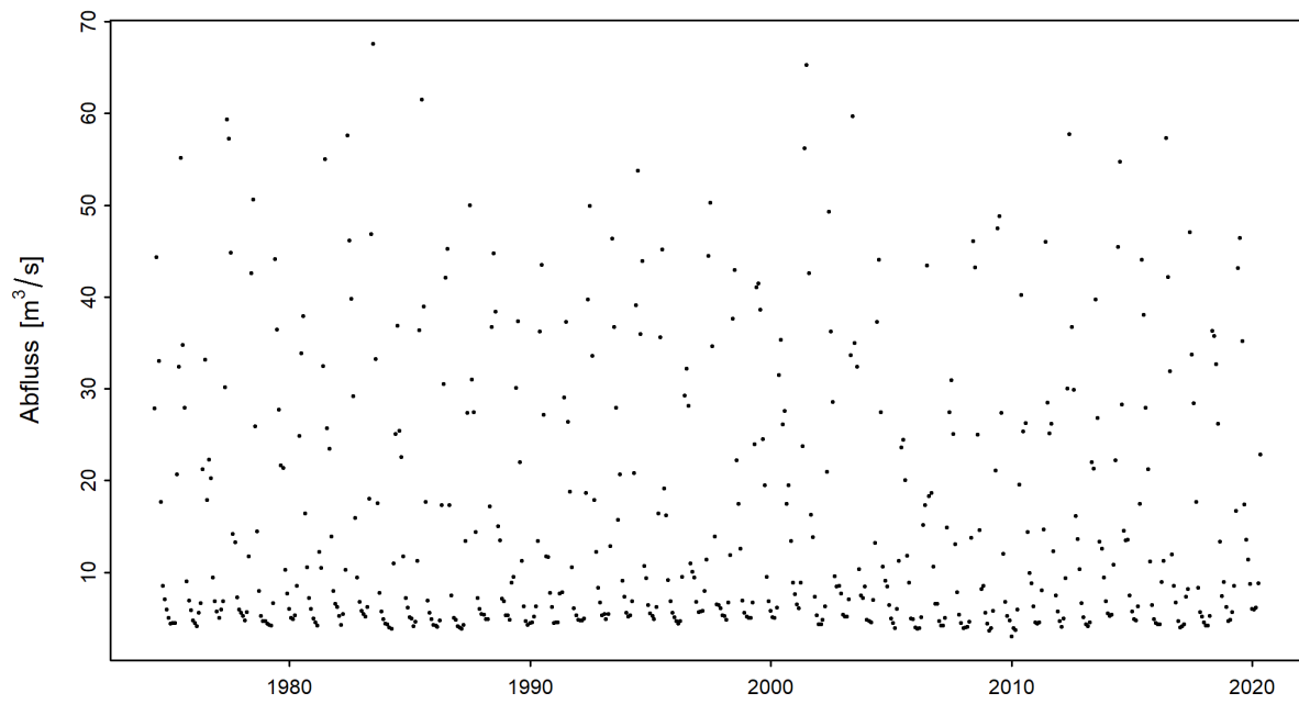
Abbildung 3: Zeitreihe der monatlichen Minima der M7Q [m³/s] (01.06.1974 - 31.05.2020)
