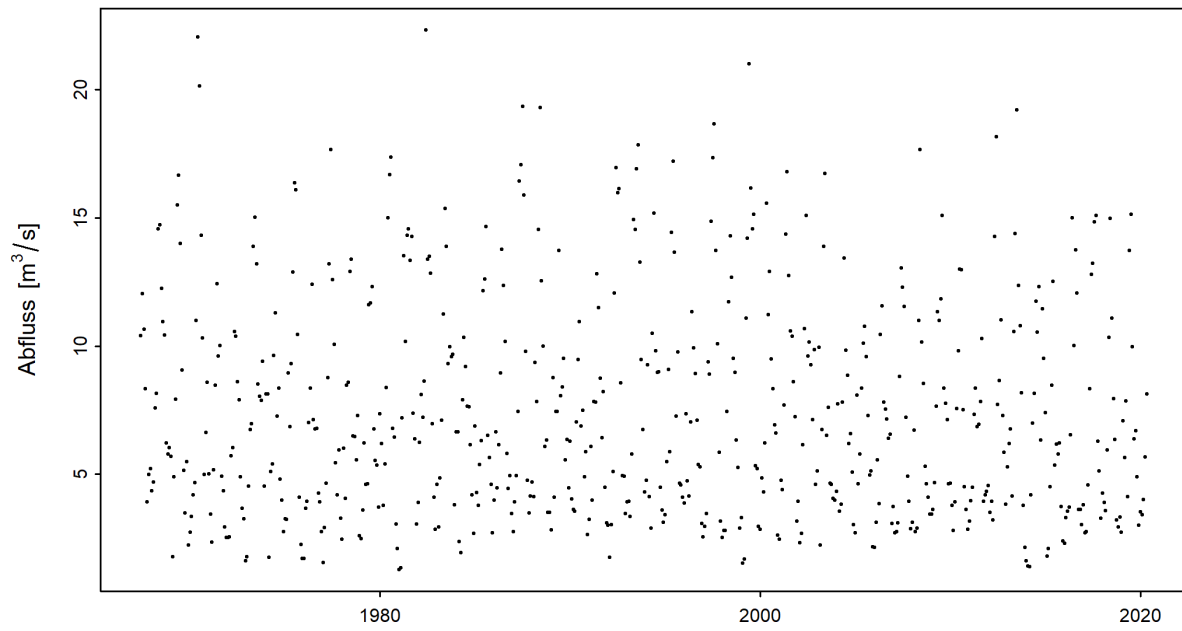
Abbildung 3: Zeitreihe der monatlichen Minima der M7Q [ \text{m}^3/\text{s} ] (01.06.1967 - 31.05.2020)
