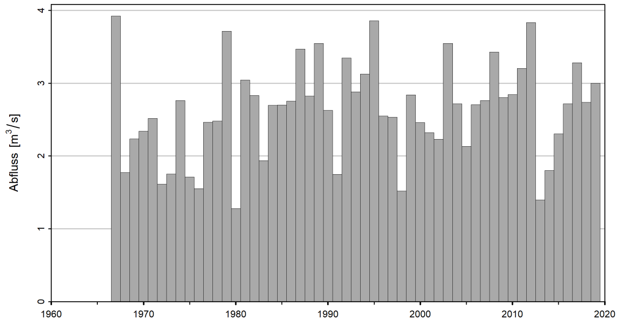
Abbildung 6: Zeitreihe der NM7Q [m³/s] (01.06.1967 - 31.05.2020)
