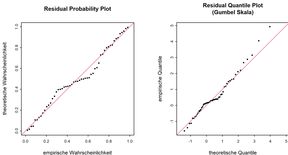
Abbildung 7: Diagnostikplots der Modellvariante “mujump1981” des BLOCK-Ansatzes (01.06.1967 - 31.05.2020)
