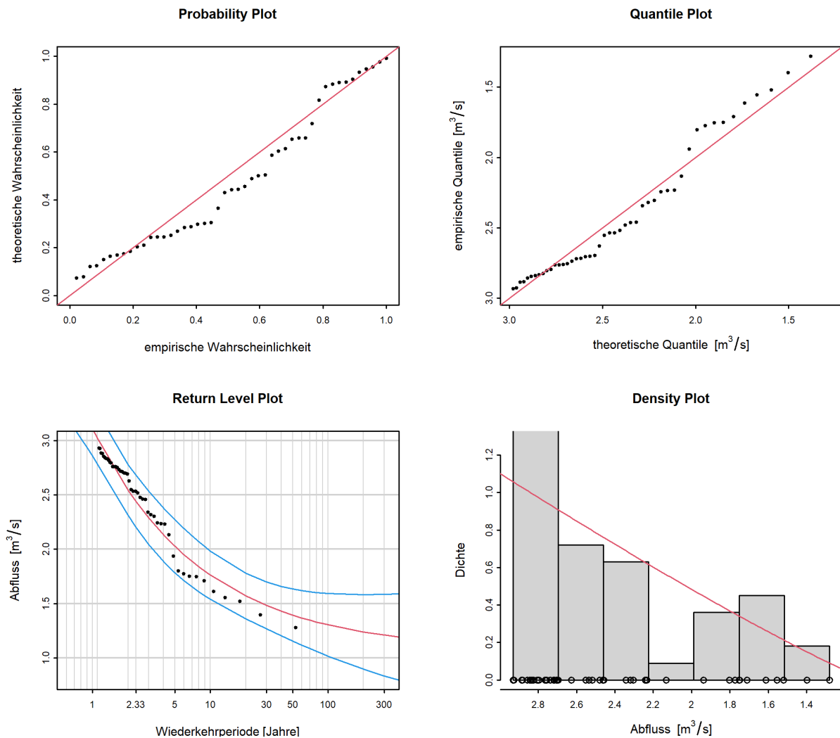
Abbildung 9: Diagnostikplots der Modellvariante “stat” des POT-Ansatzes (01.06.1967 - 31.05.2020)
