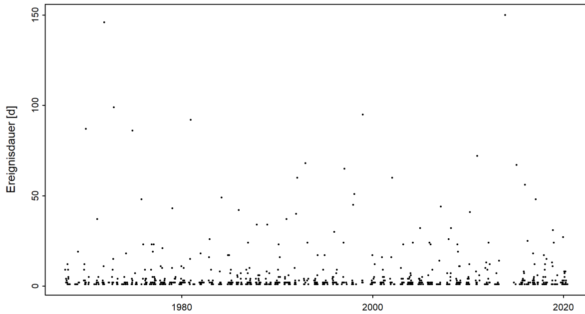
Abbildung 4: Zeitreihe der Niedrigwasserdauern [d] (01.06.1967 - 31.05.2020)
