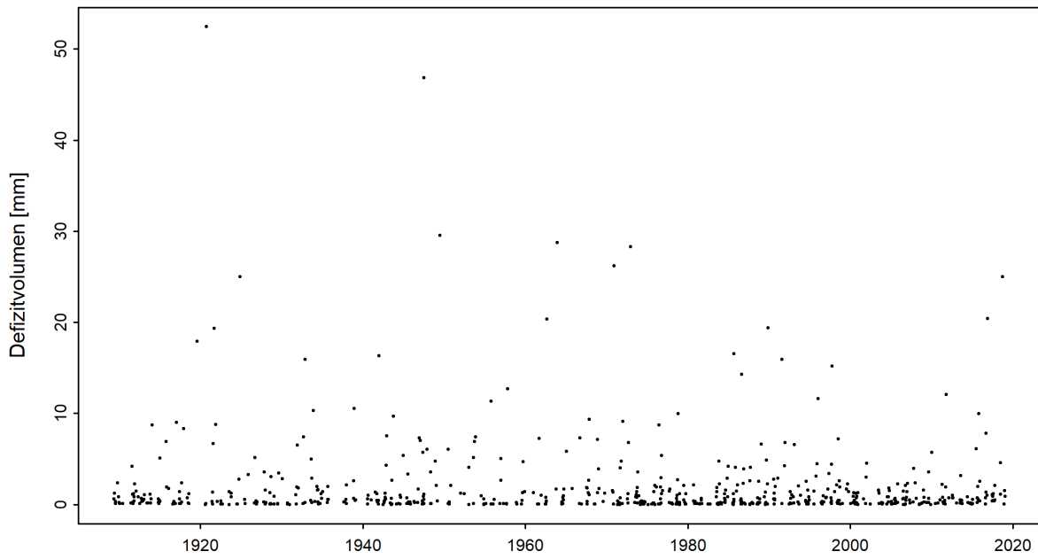
Abbildung 5: Zeitreihe der Defizitvolumen [mm] (01.04.1909 - 31.03.2019)
