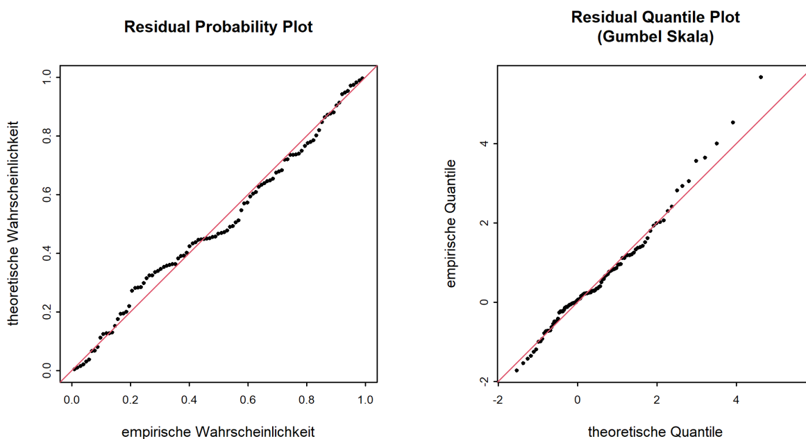
Abbildung 7: Diagnostikplots der Modellvariante "sigl" des BLOCK-Ansatzes (01.04.1918 - 31.03.2019)
