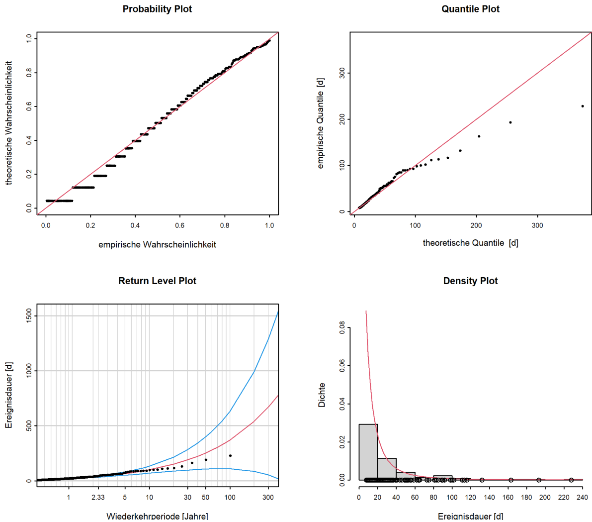
Abbildung 12: Diagnostikplots der Modellvariante "stat" des POT-Ansatzes (01.04.1918 - 31.03.2019)
