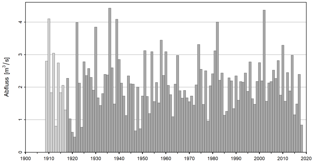
Abbildung 6: Zeitreihe der NM7Q [ \text{m}^3/\text{s} ] (01.04.1909 - 31.03.2019), hellgrau: nicht verwendete NM7Q, dunkelgrau: verwendete NM7Q
