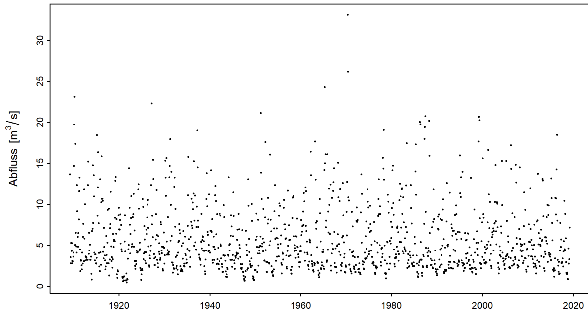
Abbildung 3: Zeitreihe der monatlichen Minima der M7Q [m 3 /s] (01.04.1909 - 31.03.2019)
