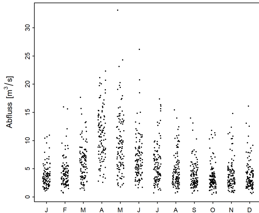
Abbildung 2: Saisonaler Verlauf der monatlichen Minima der M7Q [ \text{m}^3/\text{s} ] (01.04.1909 - 31.03.2019)
