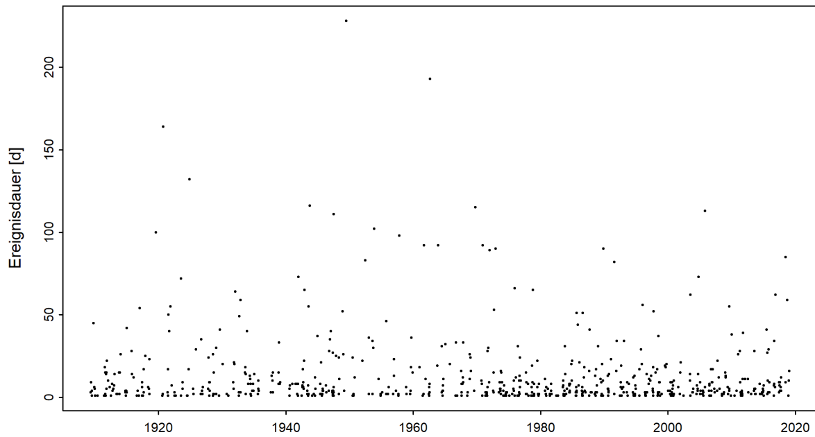
Abbildung 4: Zeitreihe der Niedrigwasserdauern [d] (01.04.1909 - 31.03.2019)
