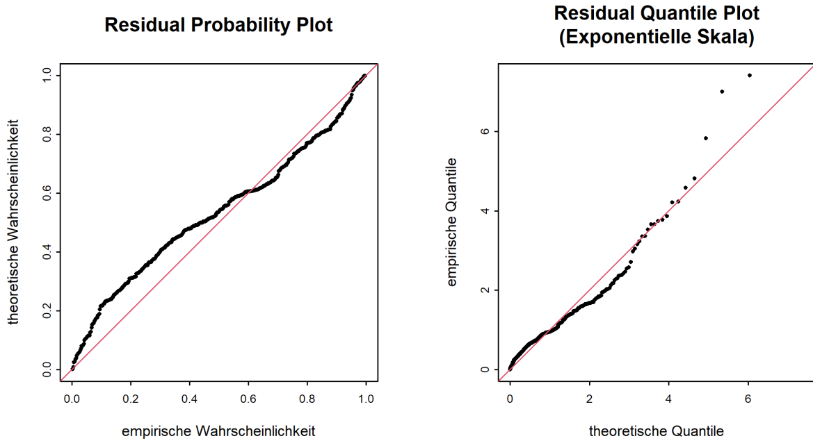
Abbildung 9: Diagnostikplots der Modellvariante “sigl” des POT-Ansatzes (01.04.1918 - 31.03.2019)
