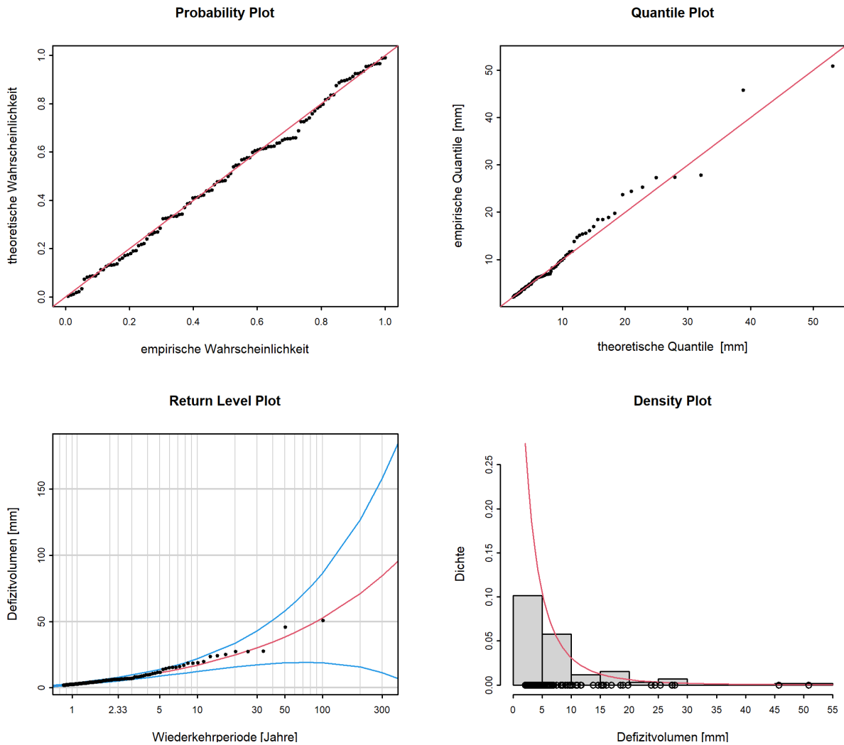
Abbildung 14: Diagnostikplots der Modellvariante “stat” des POT-Ansatzes (01.04.1918 - 31.03.2019)
